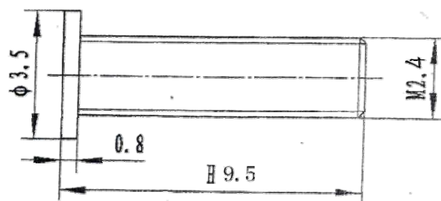
帽钉螺钉
