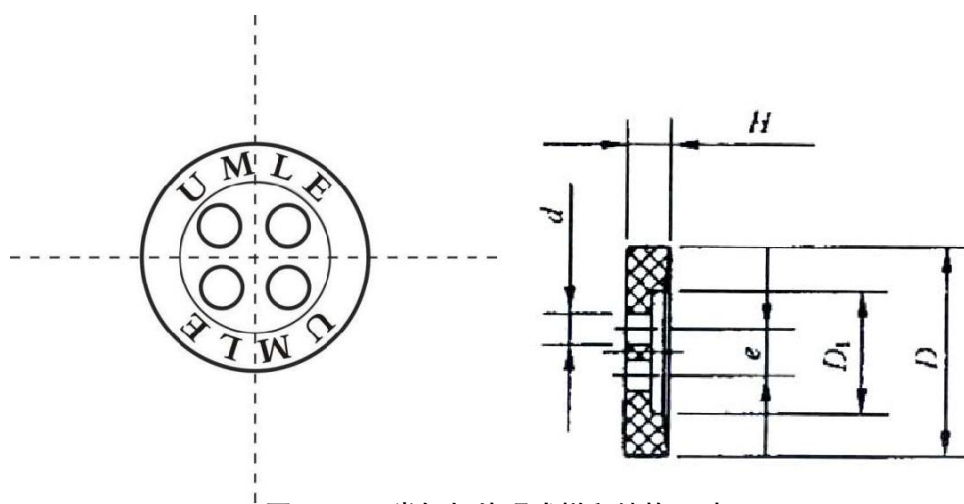
图 70 II 类钮扣外观式样和结构尺寸
