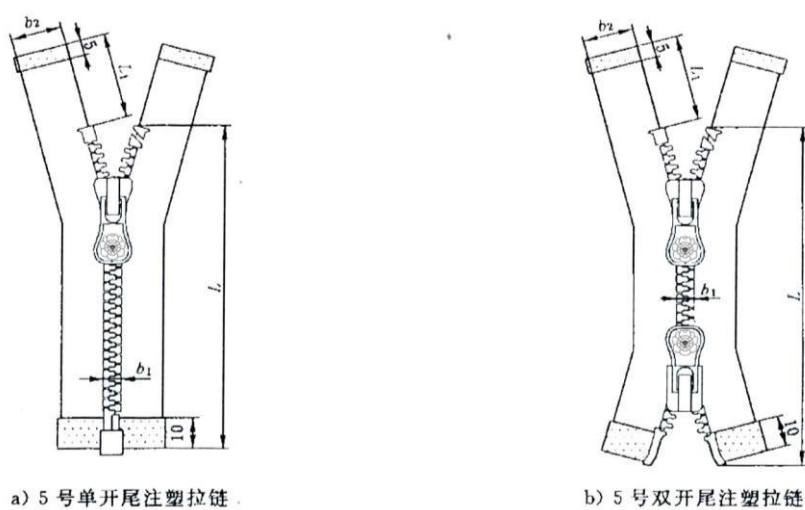
图 76 注塑拉链
