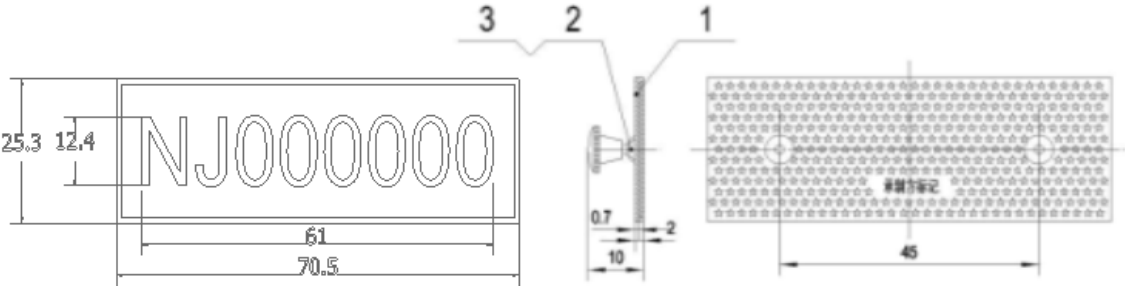
1-主体；2-螺钉；3-螺母
