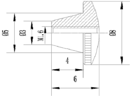
图 59b 螺钉结构及主要尺寸
