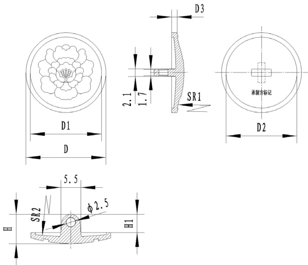
图 68 金属扣结构和主要尺寸
