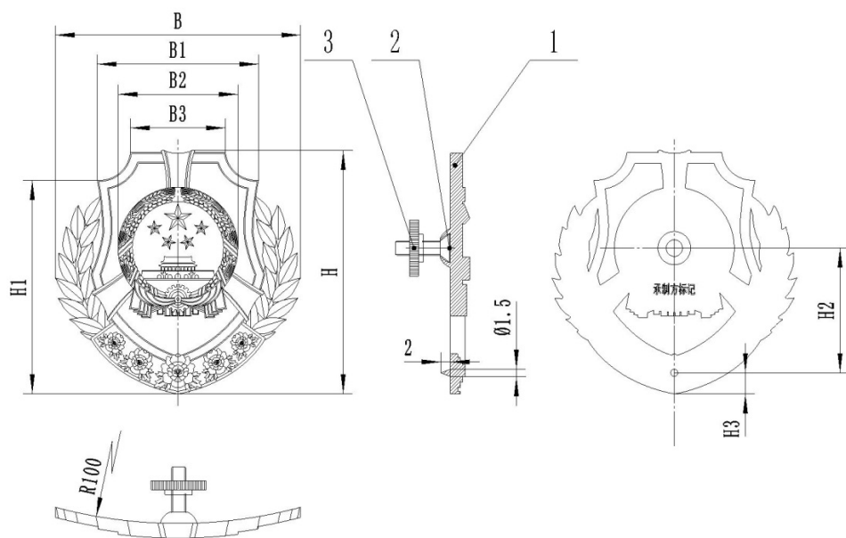
1-徽体;2-螺钉;3-螺母
