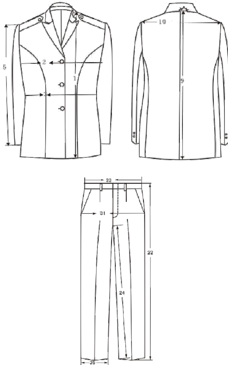
图 6 测量图
