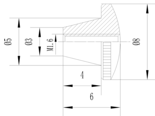
图 5 螺母结构及主要尺寸
