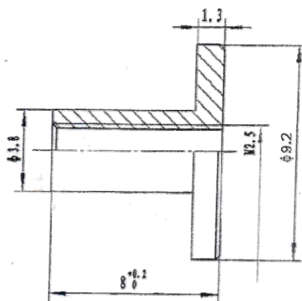
帽钉螺母
