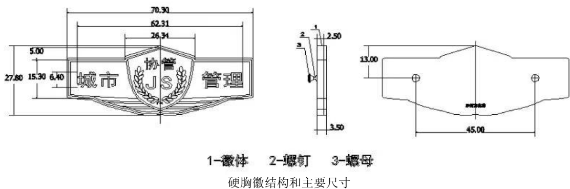
图 1 硬胸徽样式
