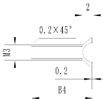
图 53c 螺母结构及主要尺寸
