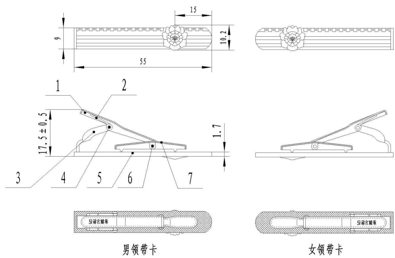
1-手柄;2-压簧;3-支架;4-销轴 1;5-骨架;6-销轴 2;7-压柄
