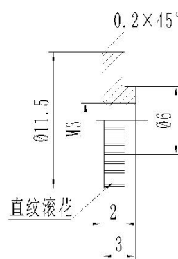
图 53b 螺钉结构及主要尺寸
