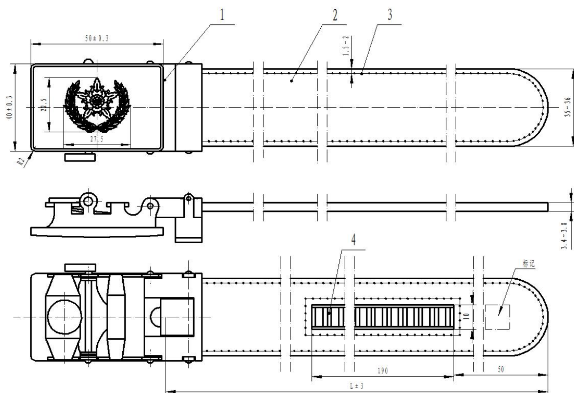
图 73 男腰带结构及主要尺寸
