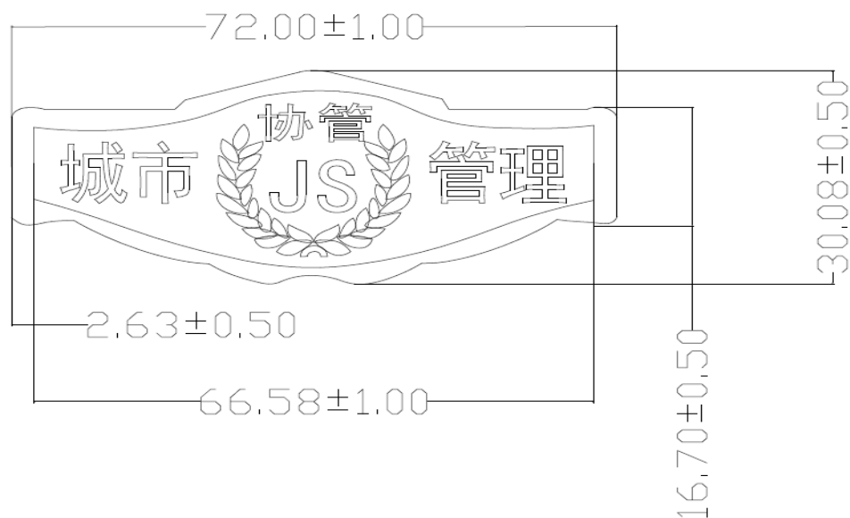
图 2 软胸徽结构和主要尺寸
