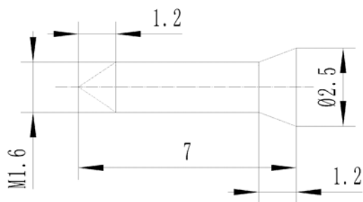
图 4 螺钉结构及主要尺寸
