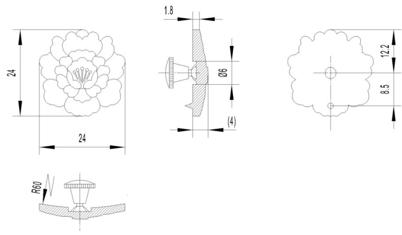
图 55a 金属牡丹花结构尺寸
