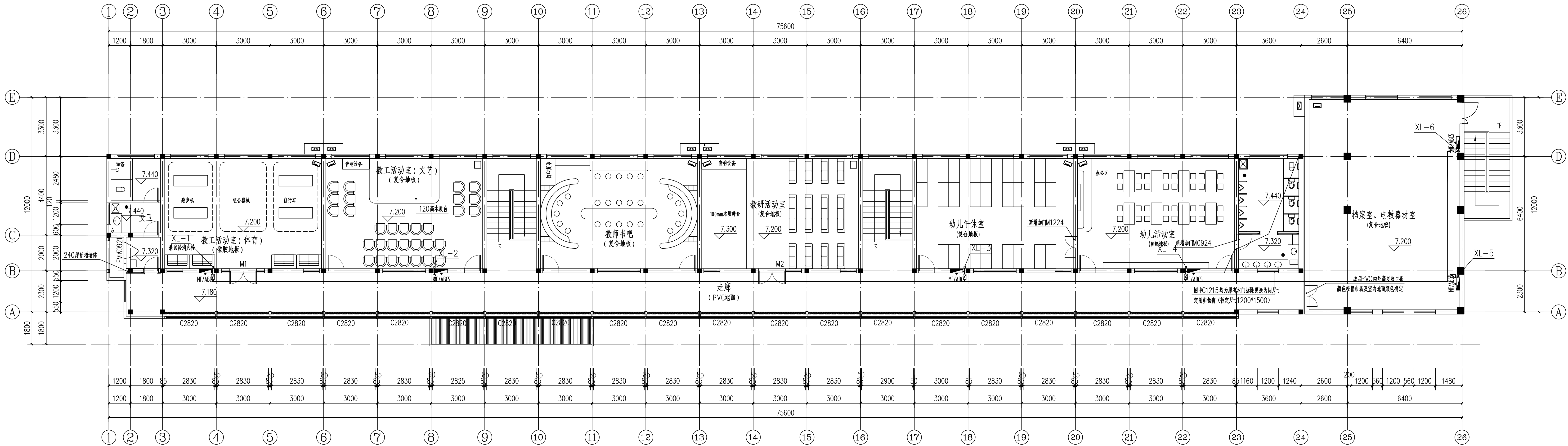
三层消火栓平面图 1:100
