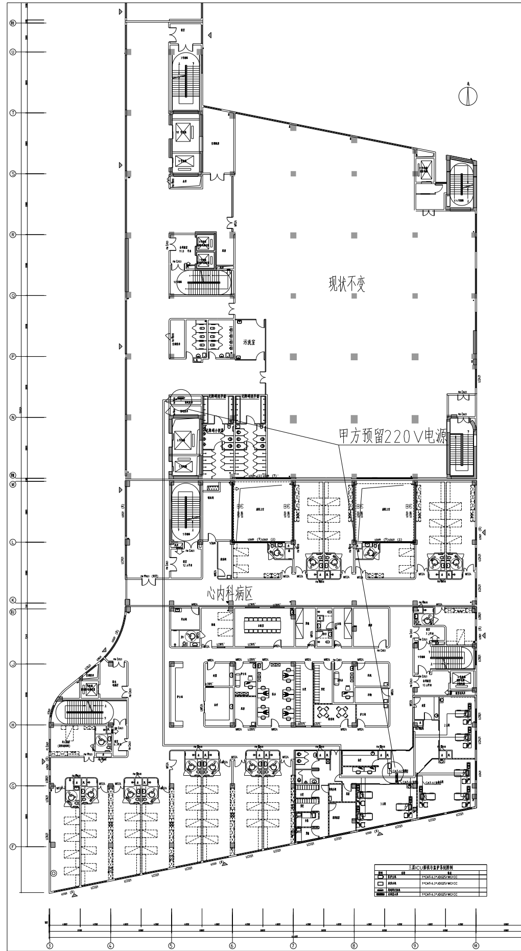
三层呼叫平面图
