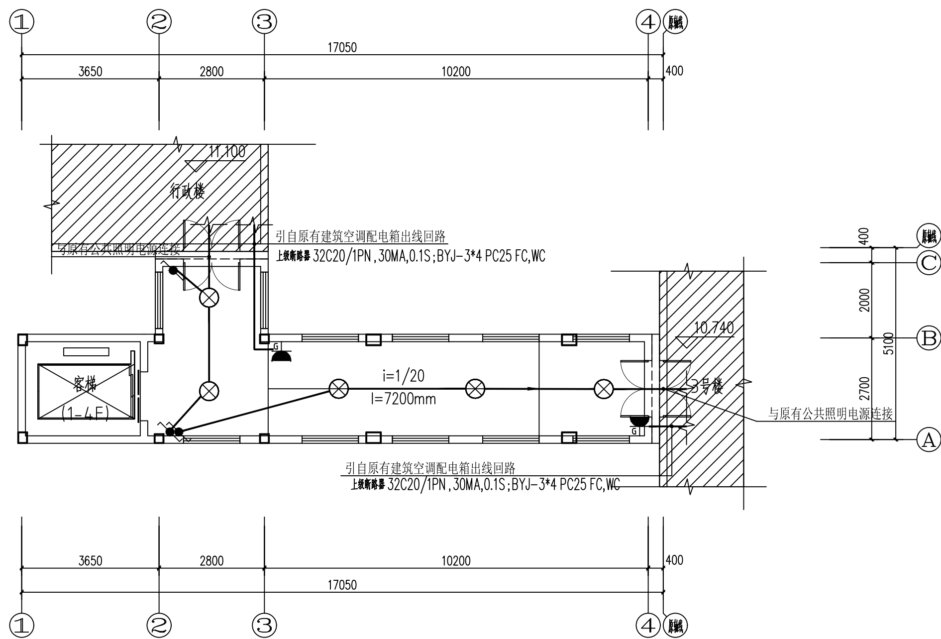
电梯四层照明平面图 1:100
