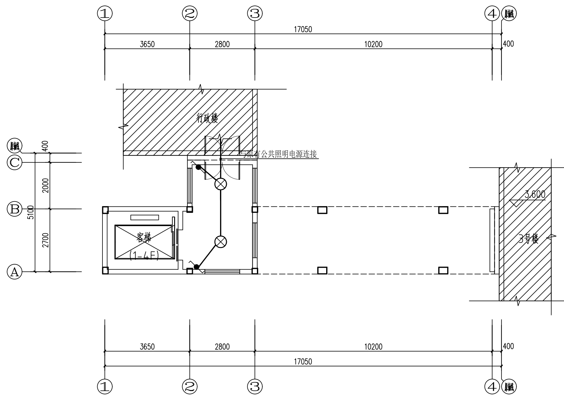
电梯二层照明平面图 1:100
