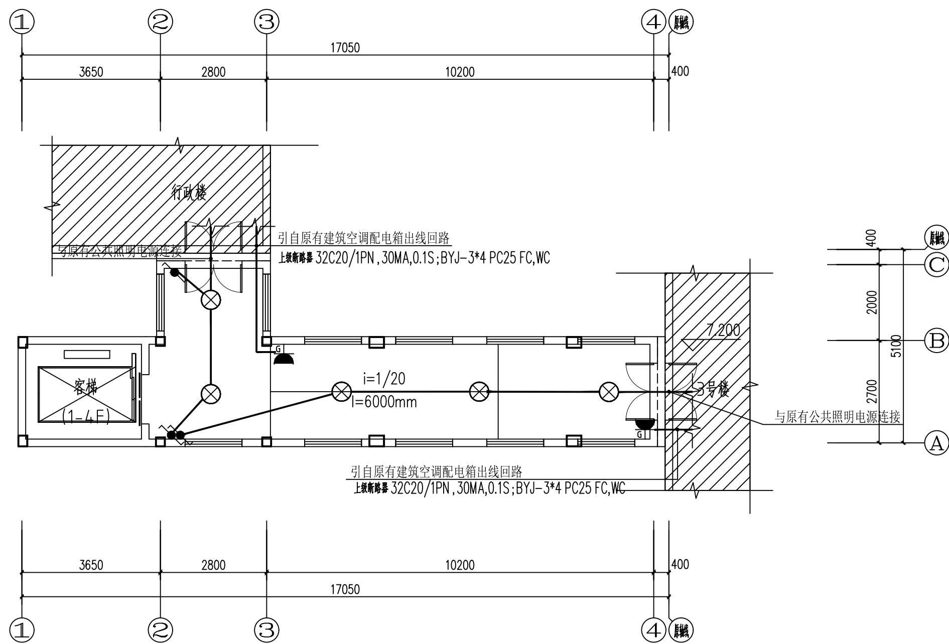
电梯三层照明平面图 1:100
