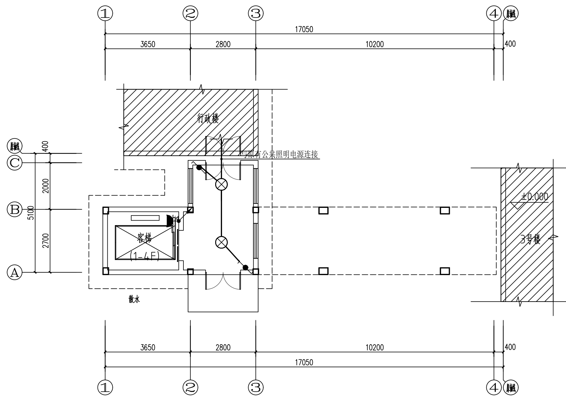
电梯一层照明平面图 1:100
