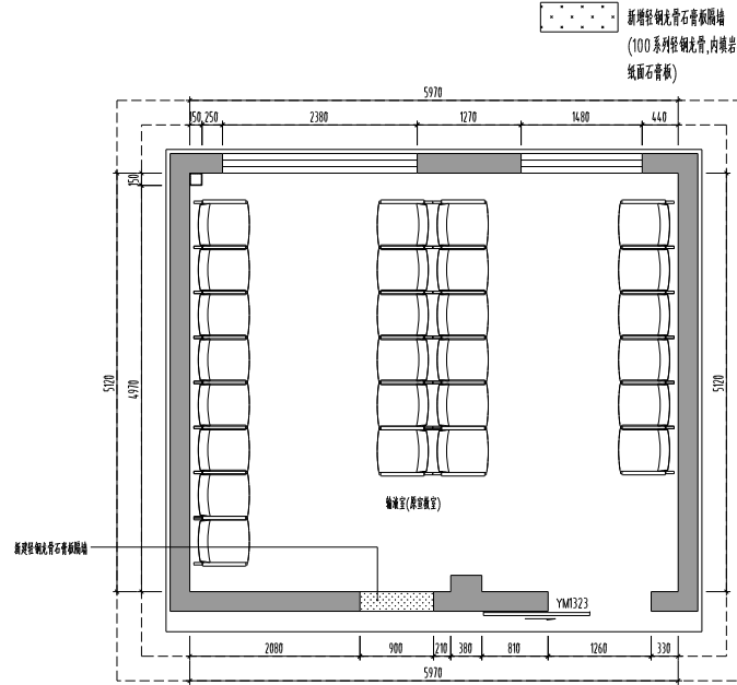
二层宣教室(原宣教室)改造后平面布置图 1:50
