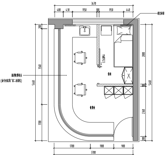
一层改造后收费处平面布置图 1:50
