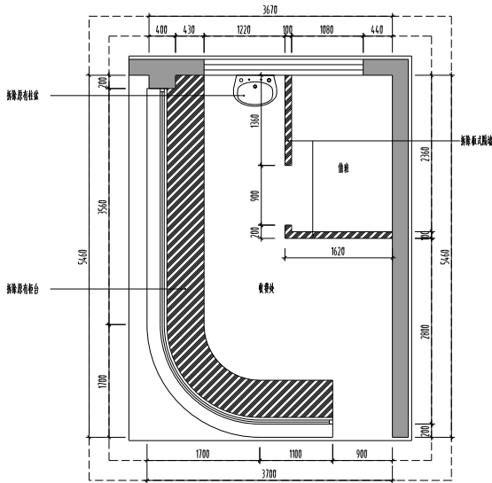
一层收费处拆除墙体图 1:50
