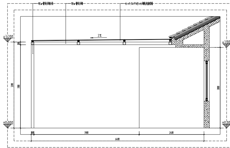
一层晒晒区A立面图 1:40
