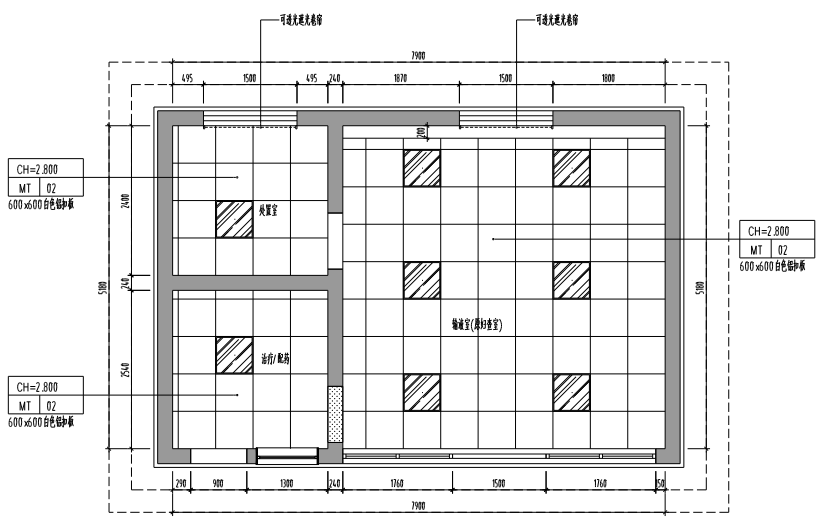
二层输液室(原实验室)改造后天花布置图 1:60
