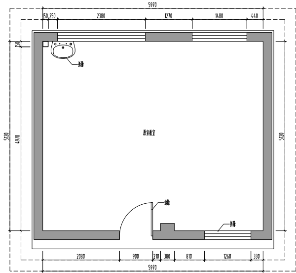
二层宣教室(原宣教室)现状平面图 1:50
