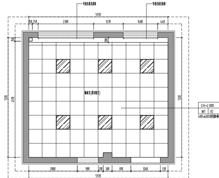
二层宣教室(原宣教室)改造后天花布置图 1:50
