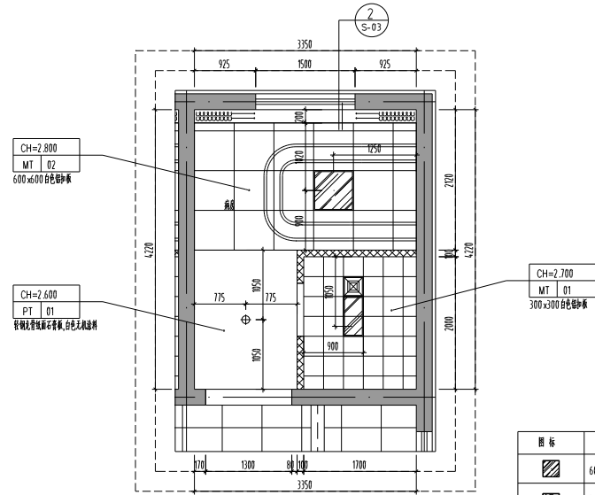
一层改造后病房(2)天花布置图 1:50
