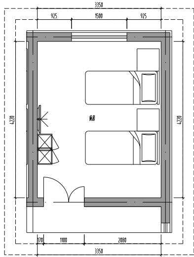
一层病房(2)现状平面图 1:50
