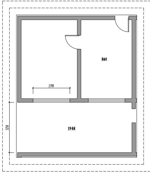
一层抽血处和室外通道现状平面图 1:75
