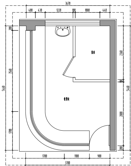
一层收费处现状平面图 1:50
