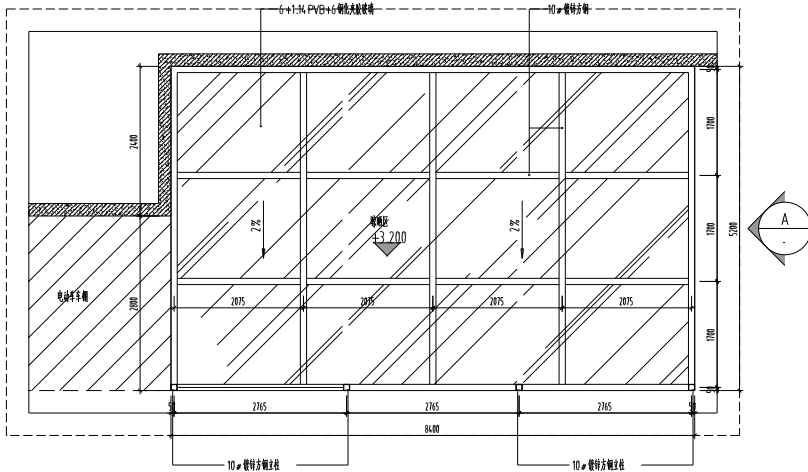
一层晒晒区天花布置图 1:60
