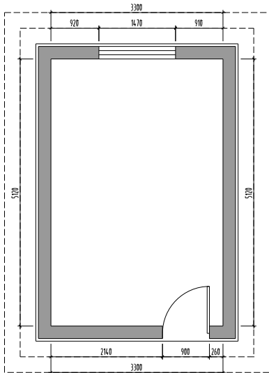
一层抢救室(原内科2东侧)现状平面图 1:50
