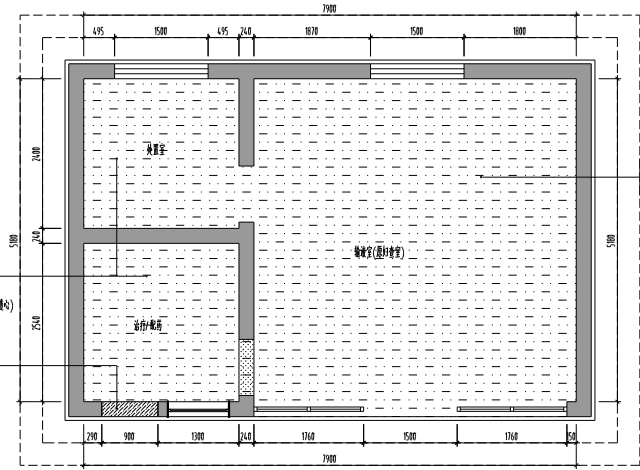
二层输液室(原实验室)改造后地面铺装图 1:60
