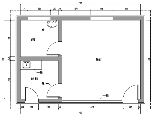
二层输液室(原实验室)现状平面图 1:60
