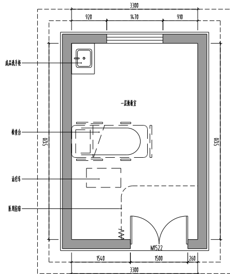
一层抢救室(原内科2东侧)改造后平面布置图 1:50
