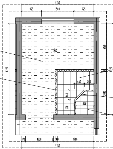
一层改造后病房(2)地面铺装图 1:50
