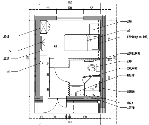
一层改造后病房(2)平面布置图 1:50
