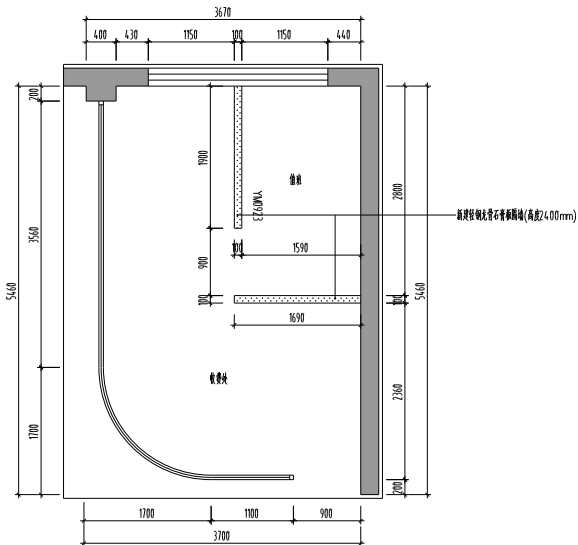
一层改造后收费处新增隔墙图 1:50
