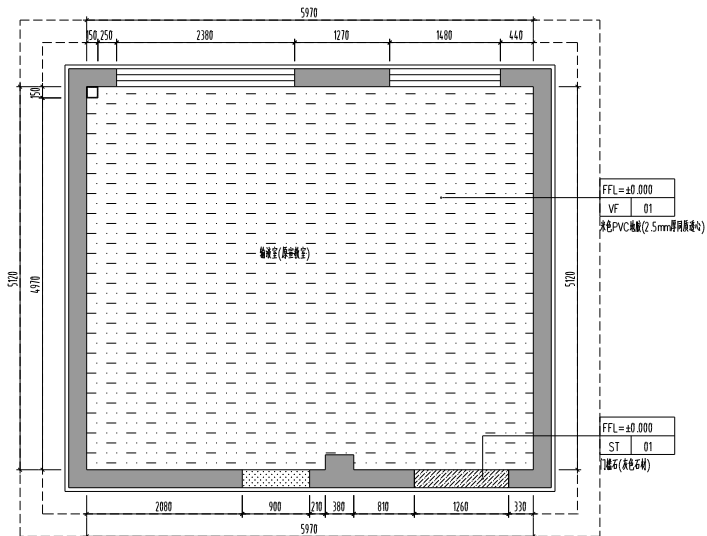
二层宣教室(原宣教室)改造后地面铺装图 1:50
