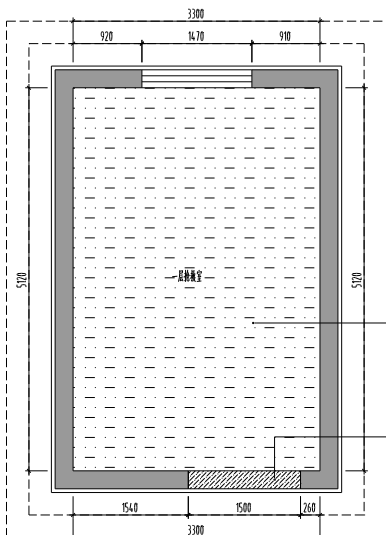
一层抢救室(原内科2东侧)改造后地面铺装图 1:50
