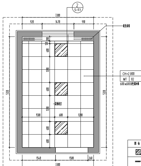
一层抢救室(原内科2东侧)改造后天花布置图 1:50
