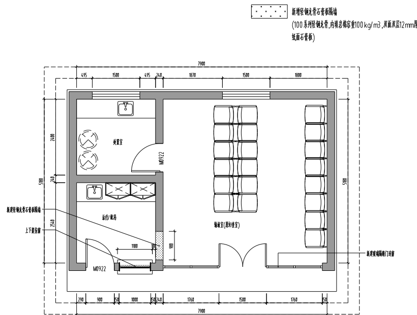
二层输液室(原实验室)改造后平面布置图 1:60
