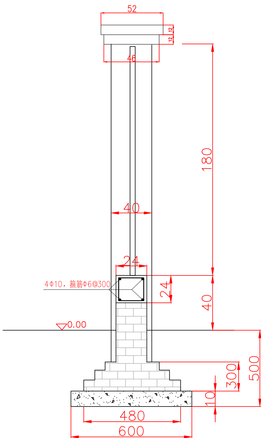
基础大样图
