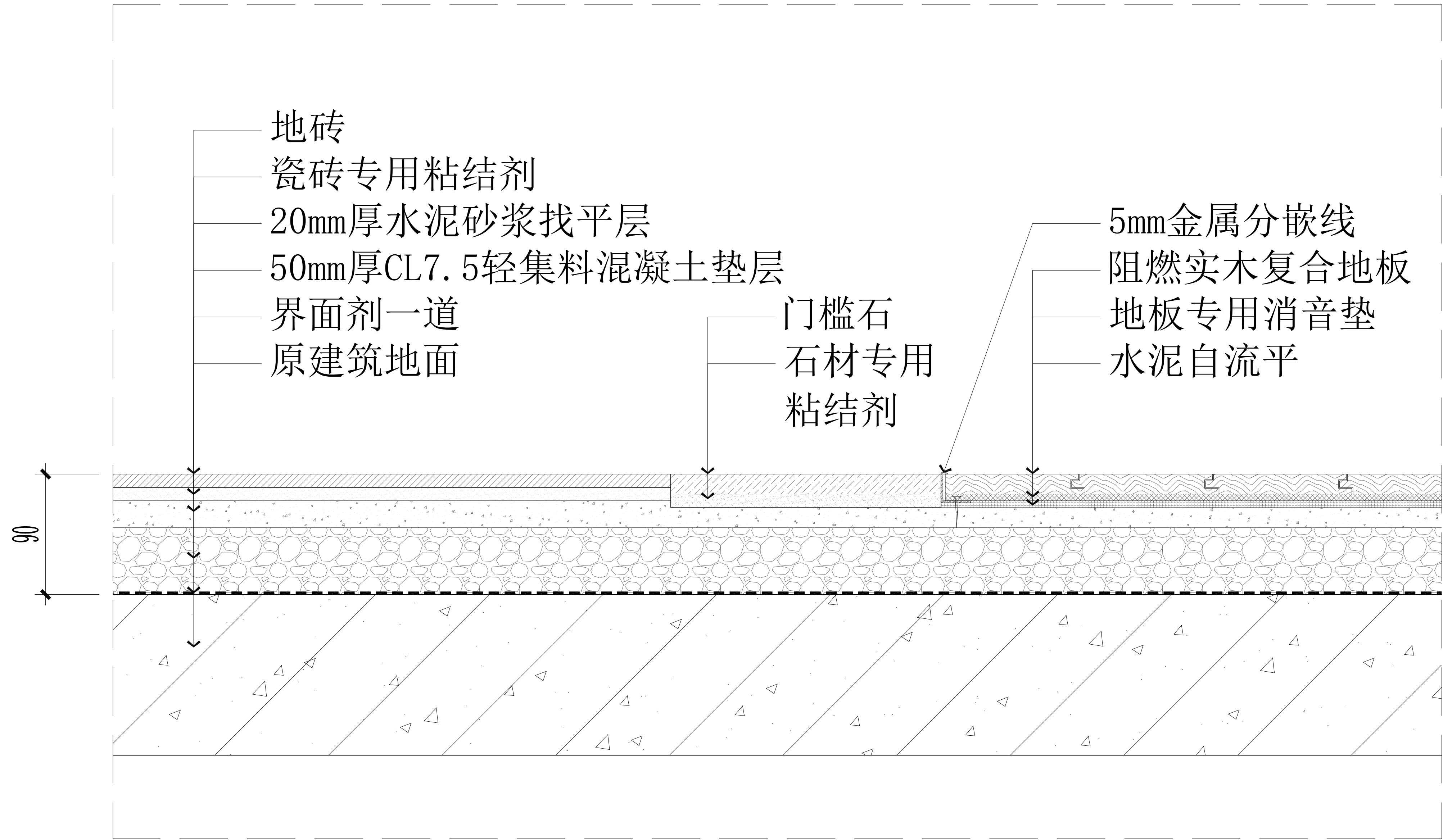
04 ELEVATION 04-P-09 地砖门槛石地板节点 SCALE 1:4
