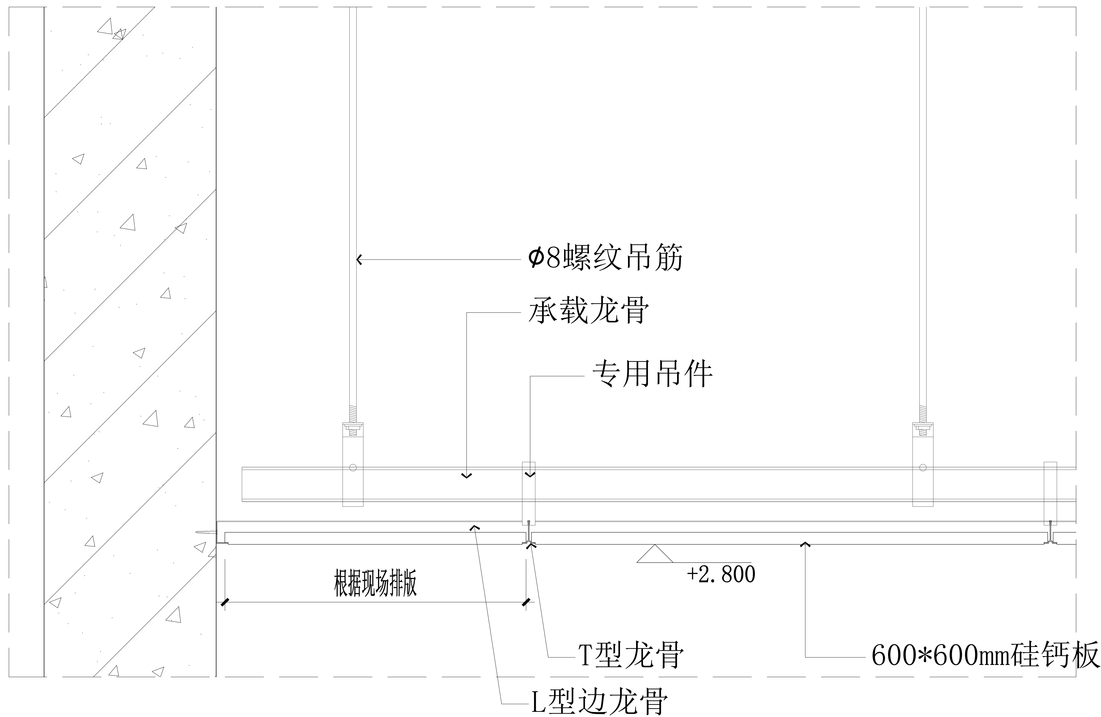
01 40-P-04 ELEVATION 硅酸钙板吊节点图 SCALE 1:5
