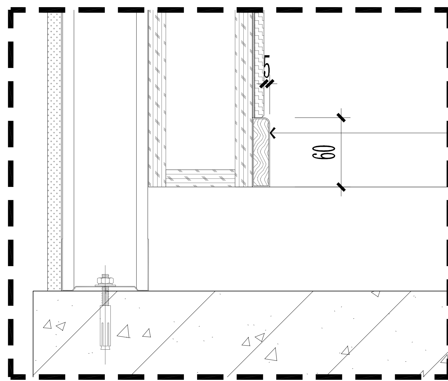
D2 大样图 SCALE 1:4
