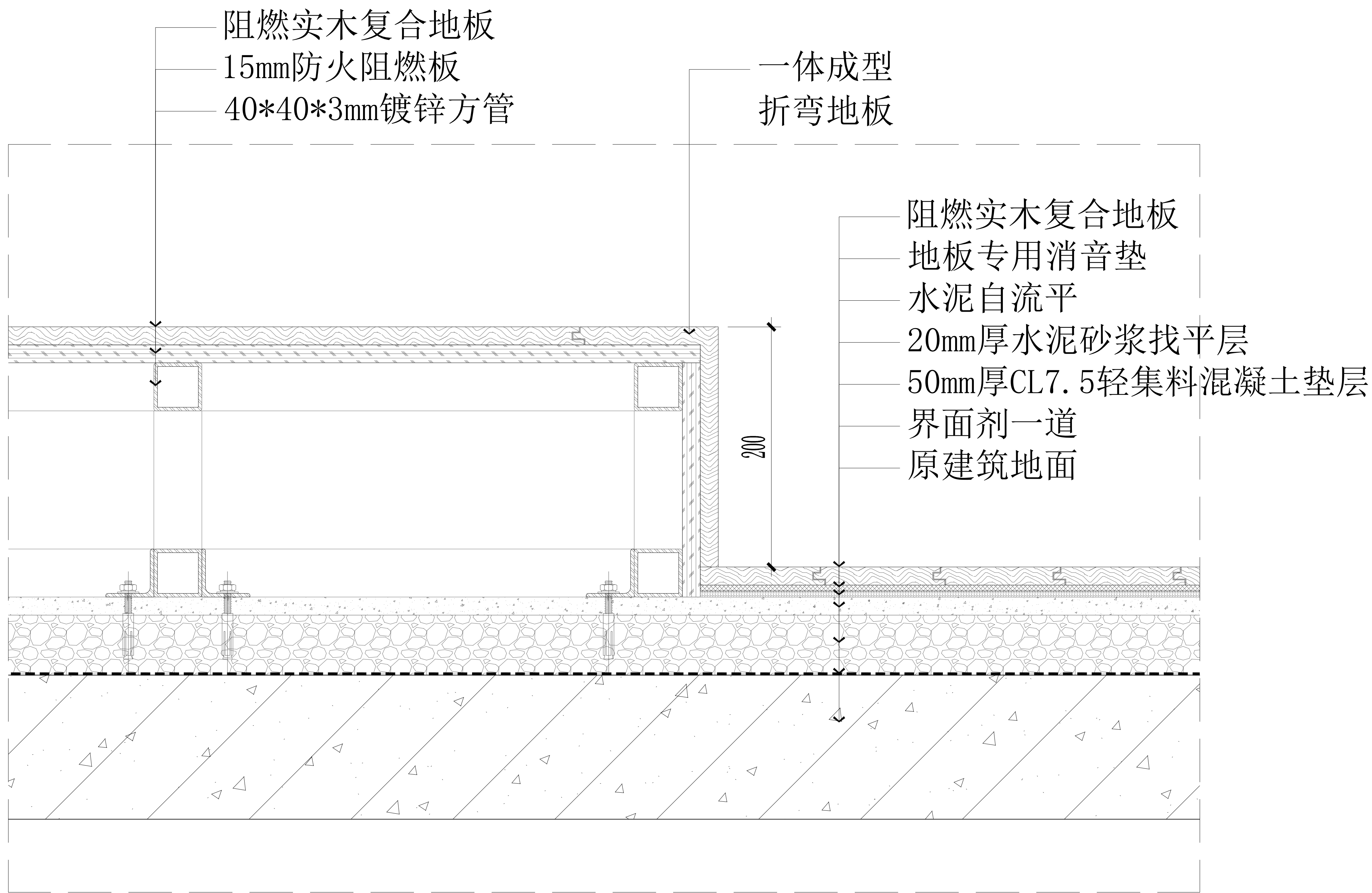
05 ELEVATION 05-P-09 地板地台节点 SCALE 1:4
