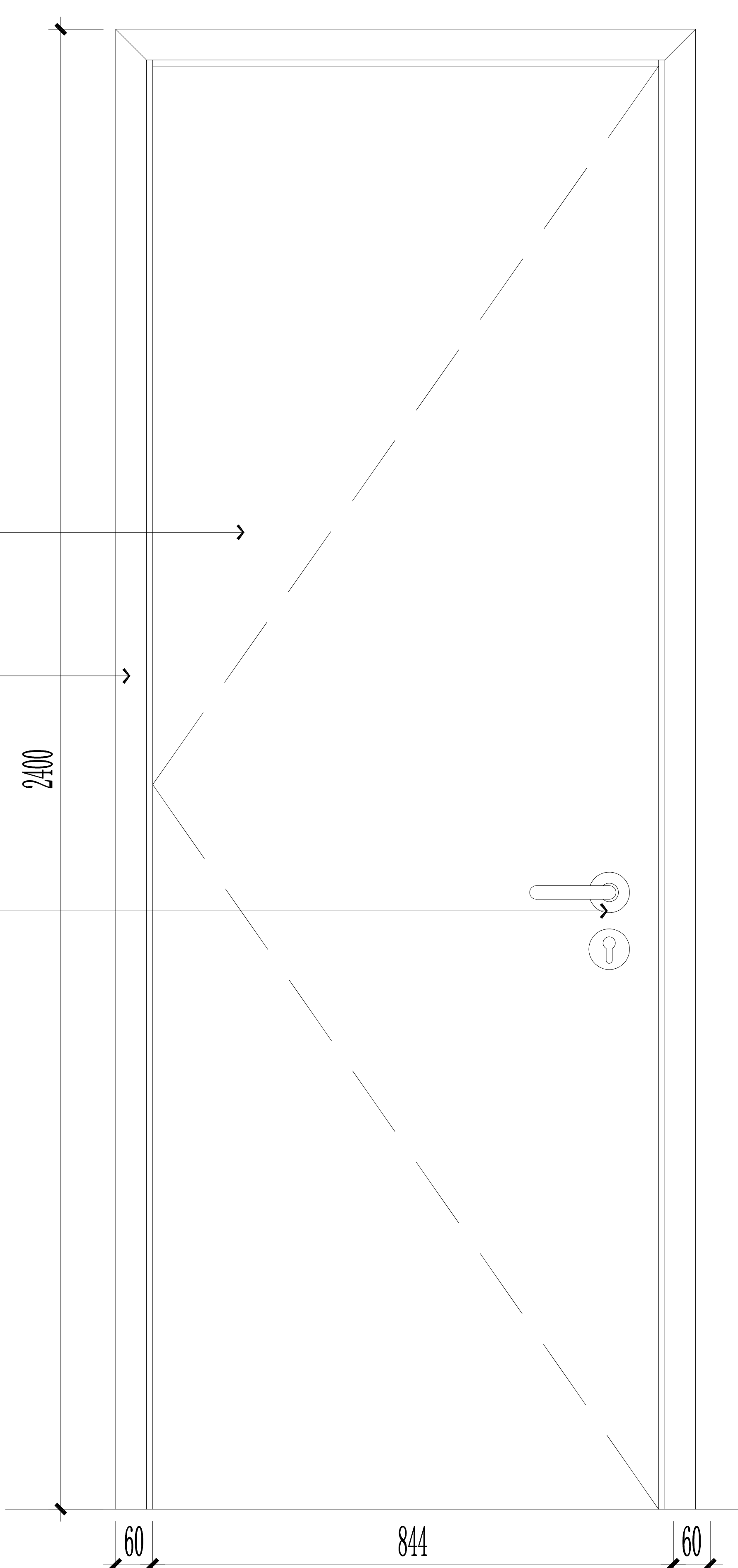
多功能教室门外立面 SCALE 1:10
