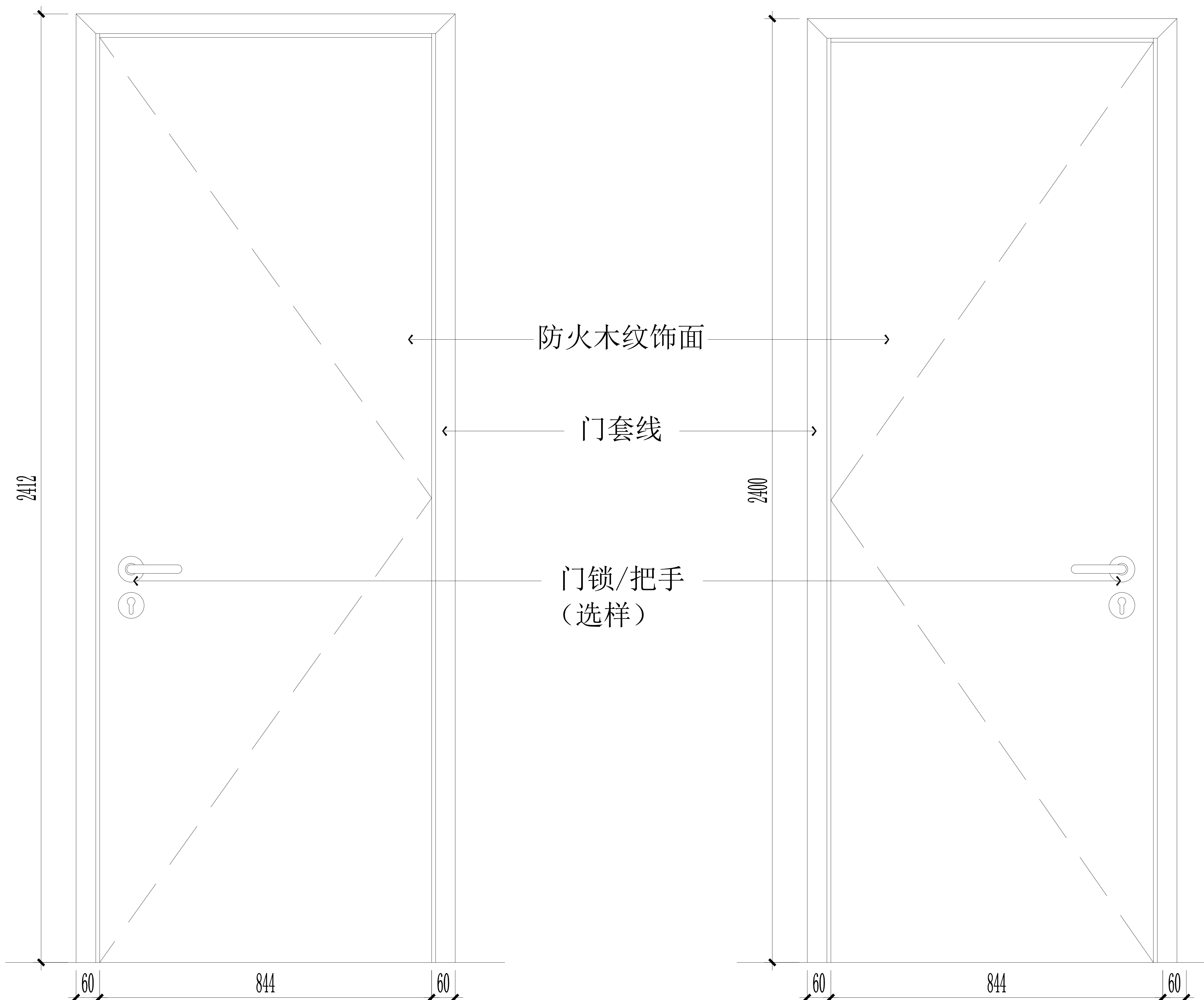
多功能教室门内立面 SCALE 1:10
