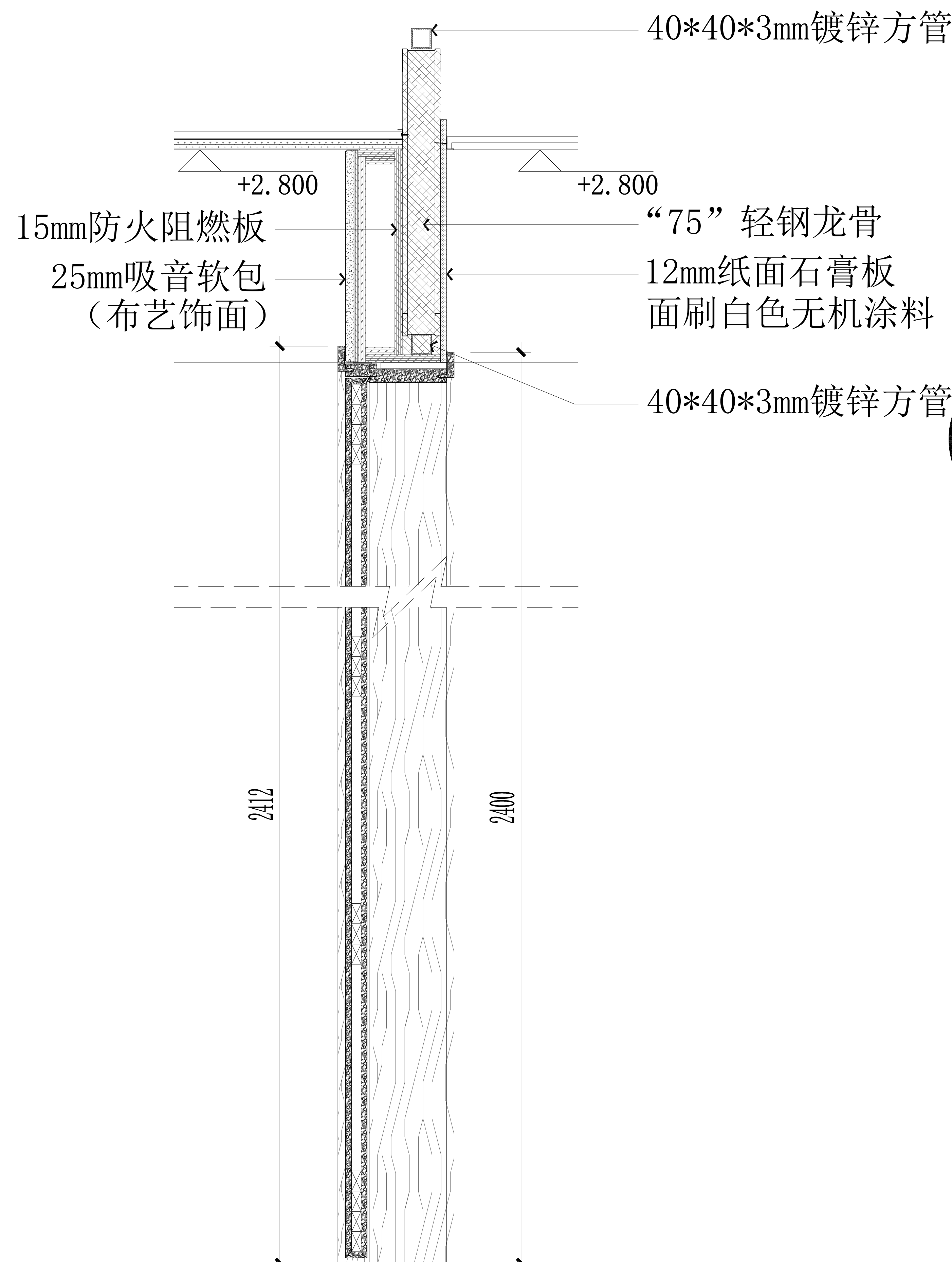
多功能教室门剖面 SCALE 1:10
