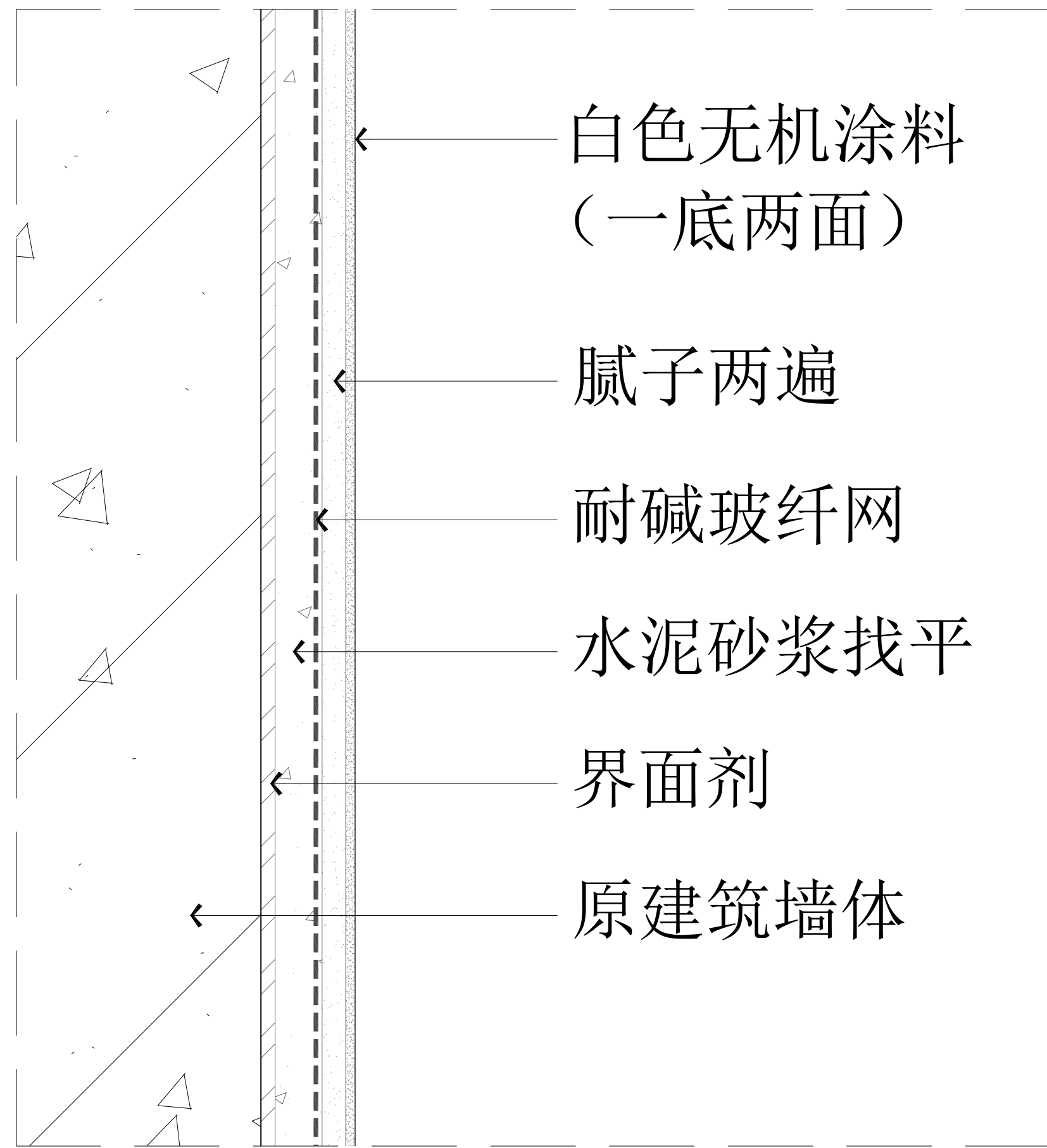
05b ELEVATION 05b-P-09 原建筑墙体涂料节点 SCALE 1:2
