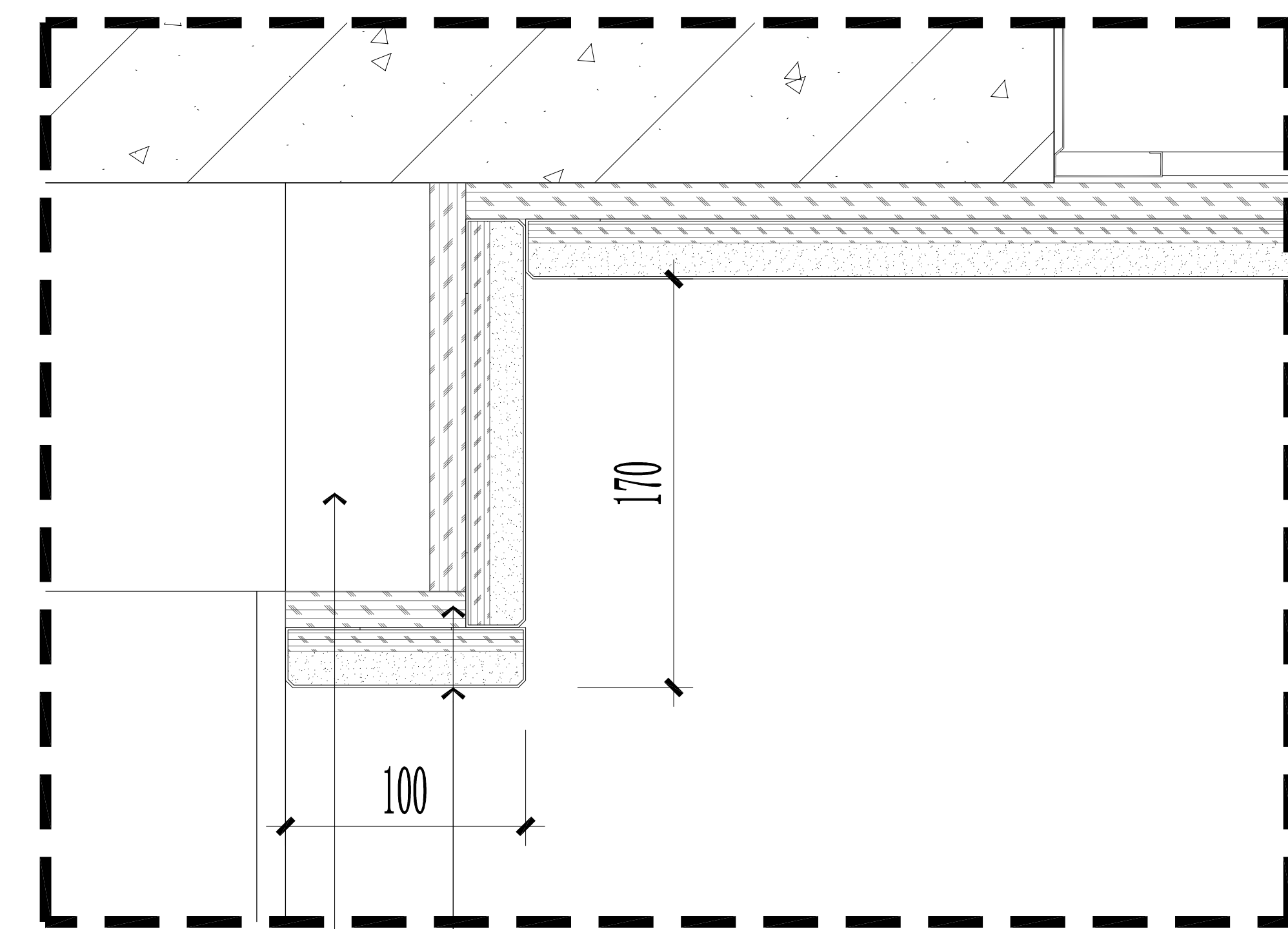
D3 大样图 SCALE 1:4
