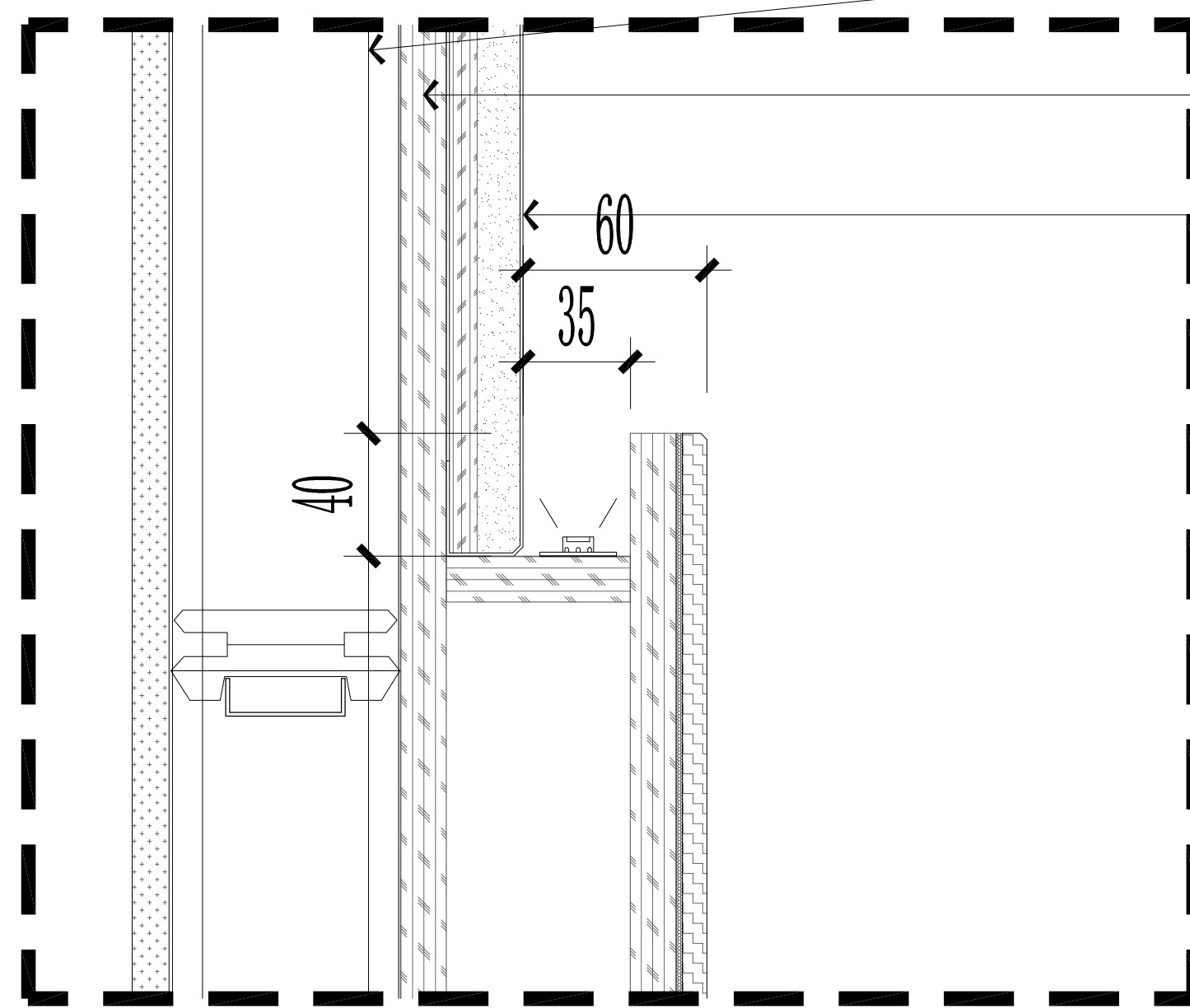
D1 大样图 SCALE 1:4
