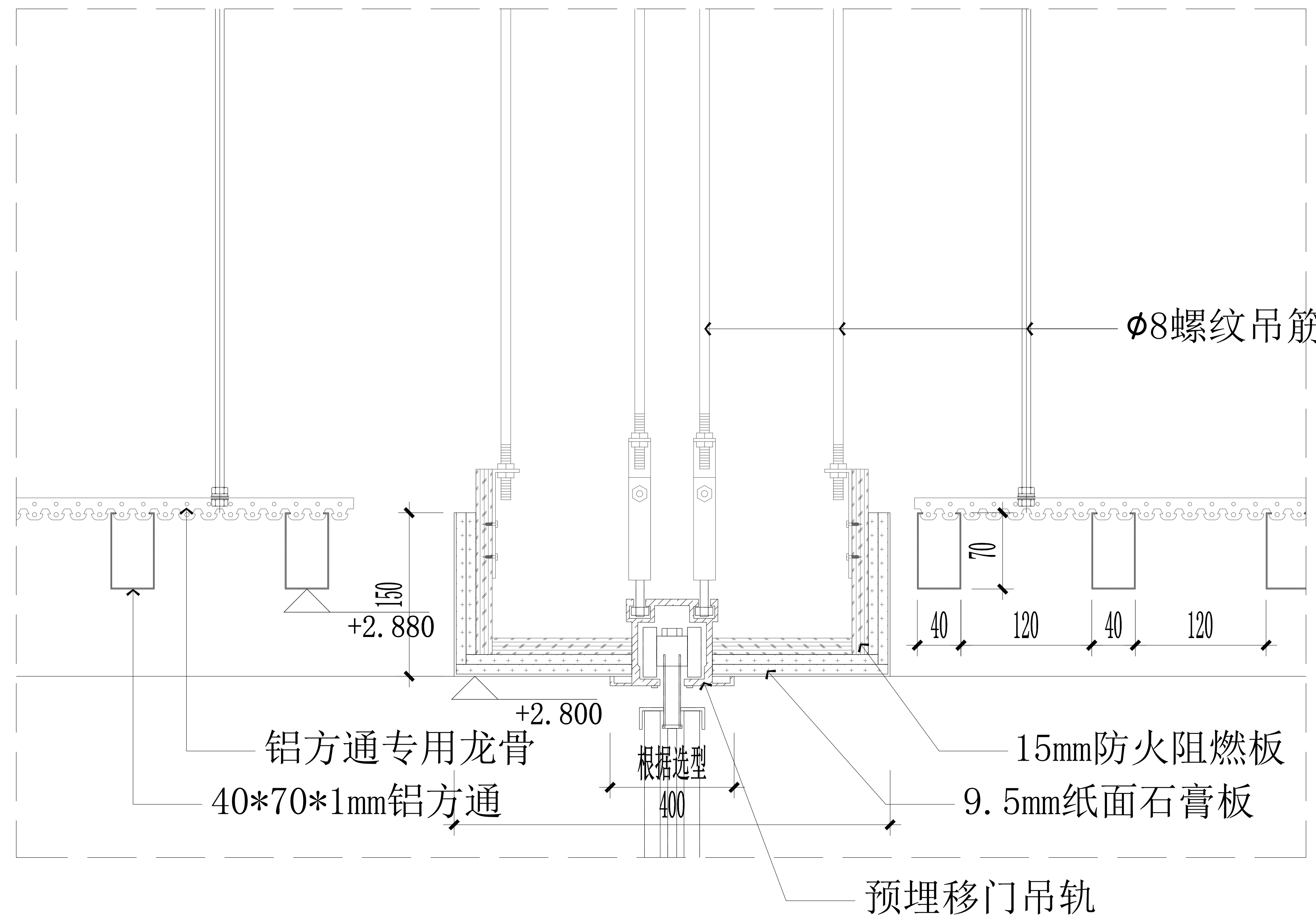
02 40-P-04 ELEVATION 移门轨道节点图 SCALE 1:5
