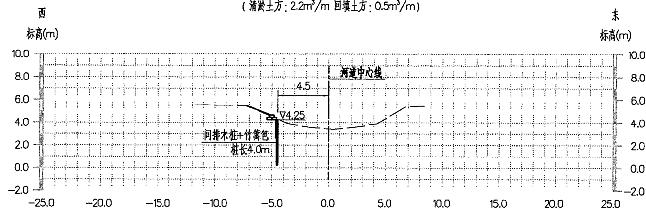
K0+247 (回填土方: 0.0m³/m)
