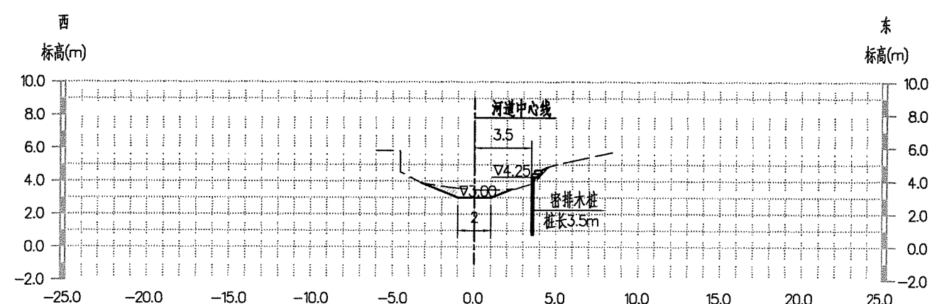
K0+120 (清淤土方: 2.0m³/m 回填土方: 0.5m³/m)
