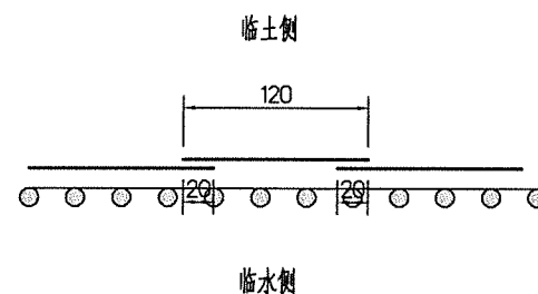
竹篱笆搭接平面示意图
