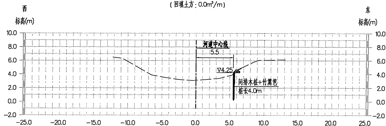
K1+547 (回填土方: 0.0m³/m)
