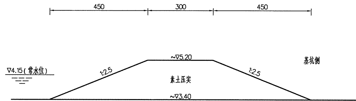
头甲河施工围堰结构图
