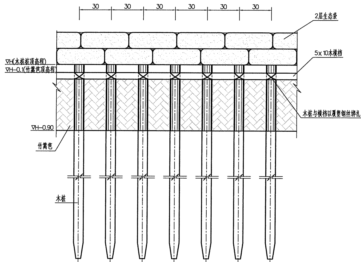
间排木桩+篱笆桩立面图
