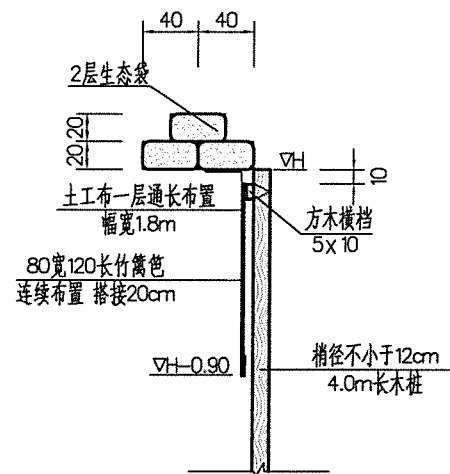
间排木桩+篱笆桩结构图
