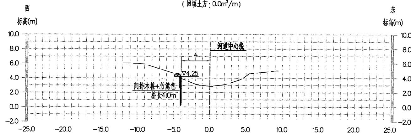
K1+067 (回填土方: 0.0m³/m)
