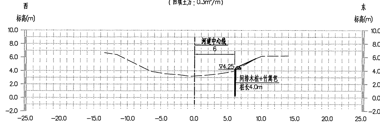
K2+067 (回填土方: 0.5m³/m)
