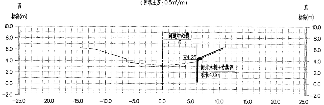
K2+147 (回填土方: 0.8m³/m)
