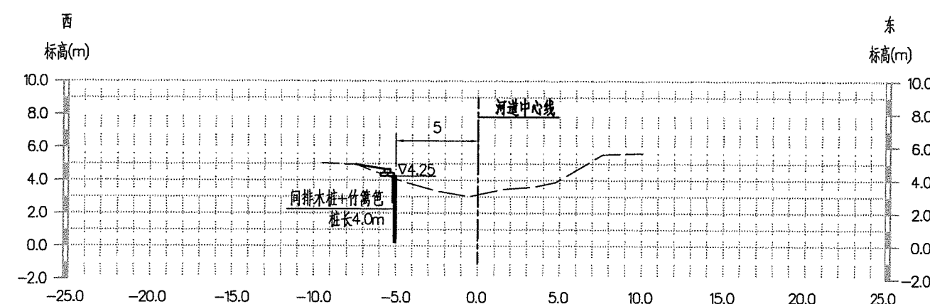
K0+747 (回填土方: 0.2m³/m)
