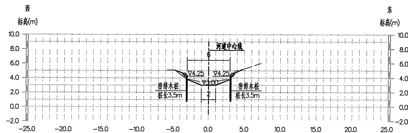
K0+060 (清淤土方: 2.2m³/m 回填土方: 0.5m³/m)
