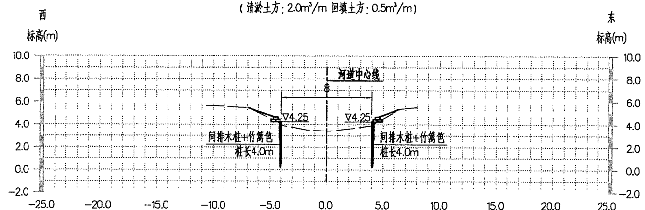
K0+347 (回填土方: 0.5m³/m)
