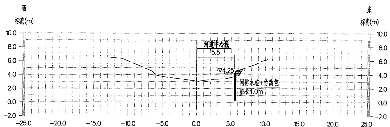
K1+947 (回填土方: 0.5m³/m)
