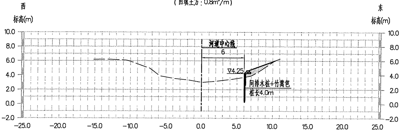
K2+347 (回填土方: 2.1m³/m)
