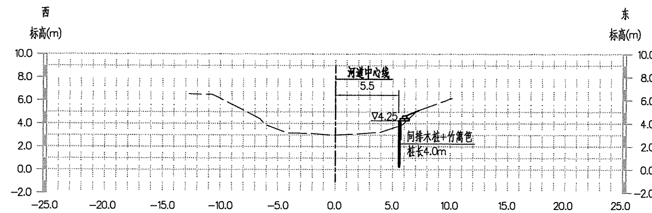
K1+847 (回填土方: 0.3m³/m)
