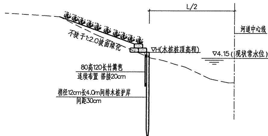
间排木桩+篱笆桩护岸标准断面图
