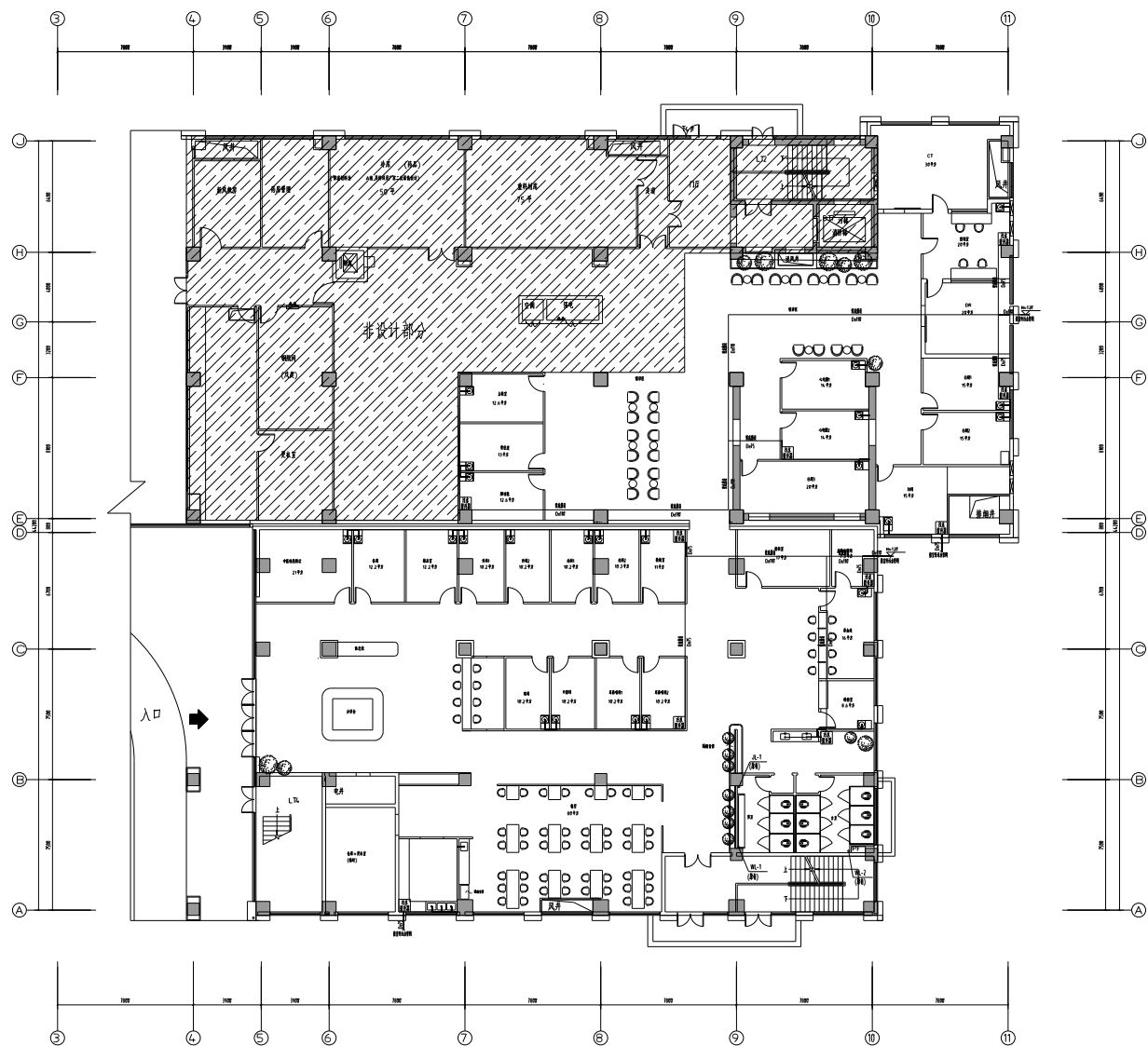
排水平面图 1:100
