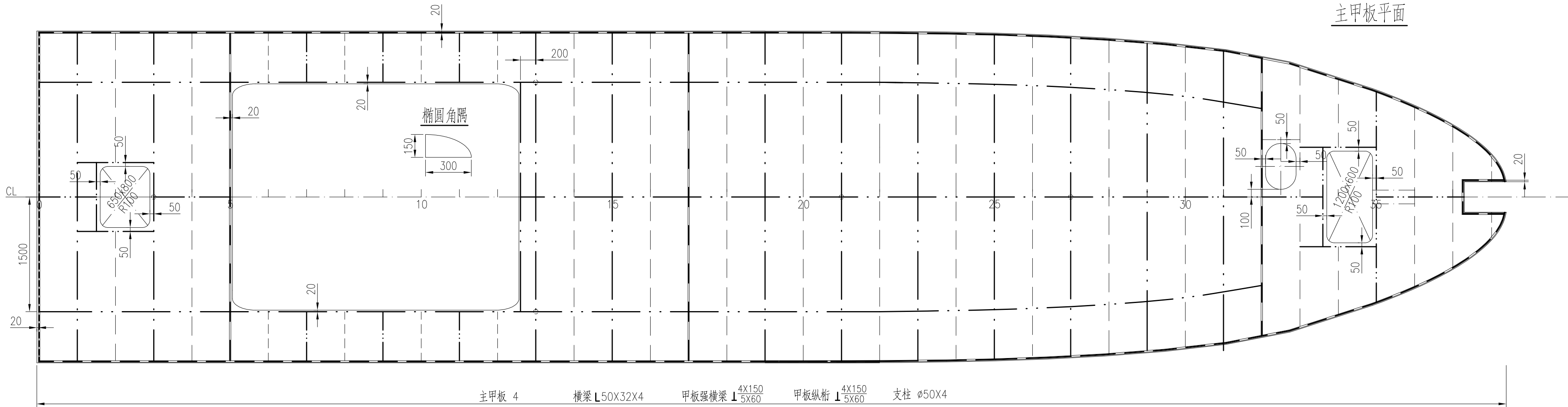
主甲板平面
