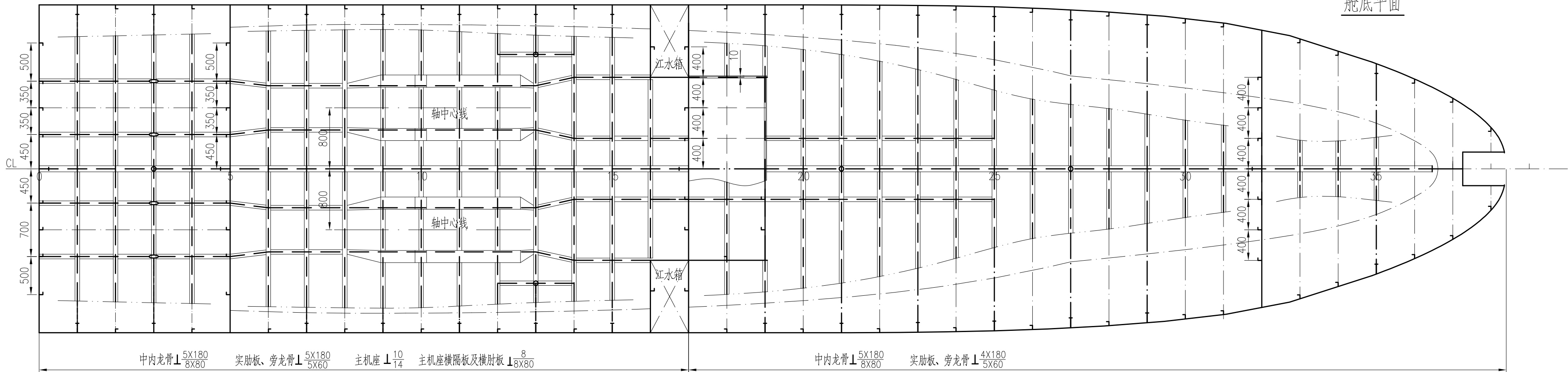
舱底平面
