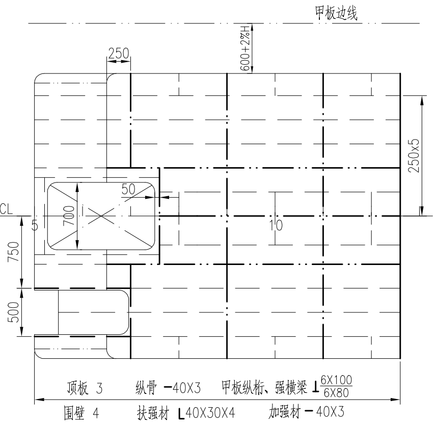
机舱顶棚
