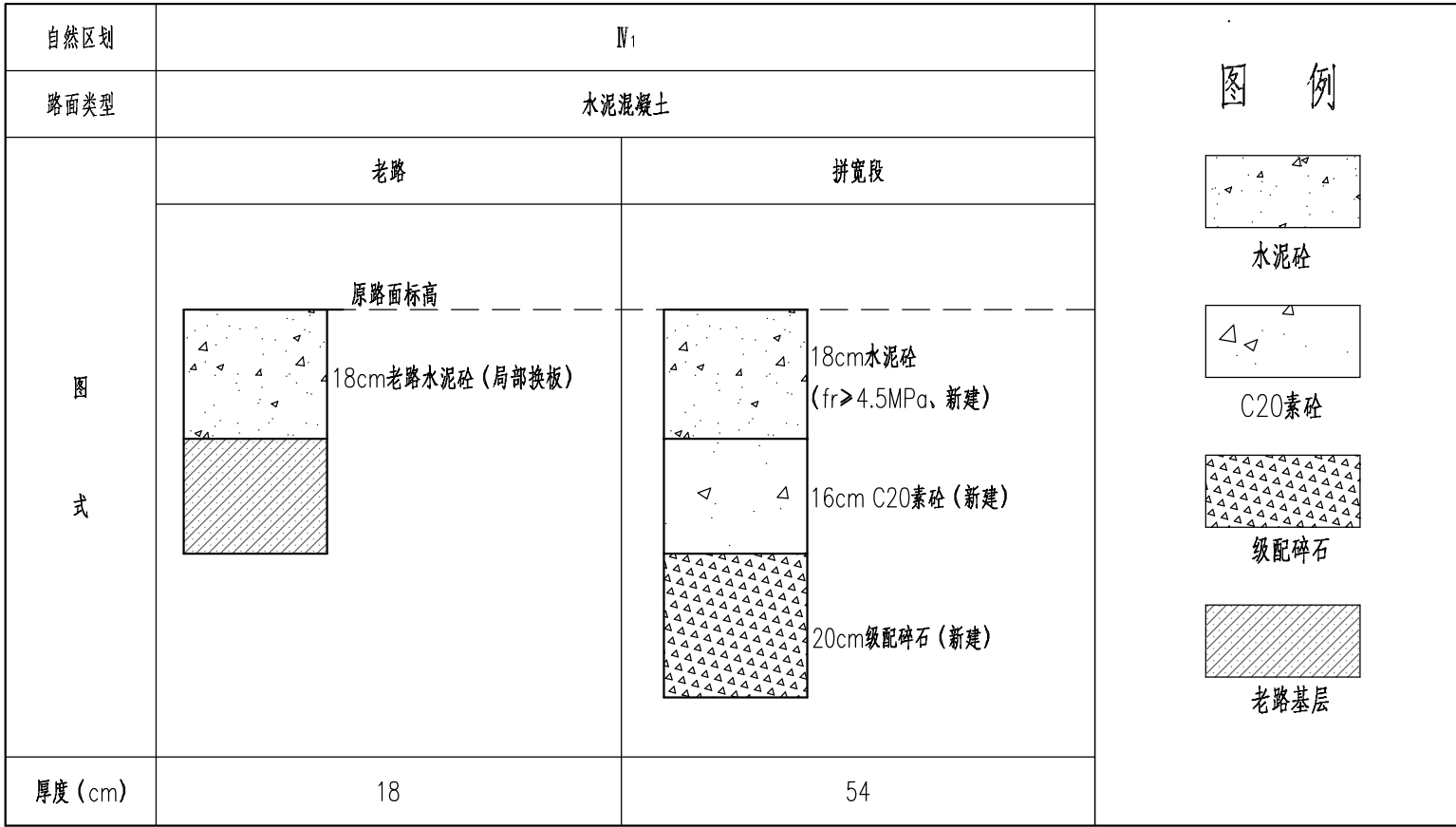
路面结构图
