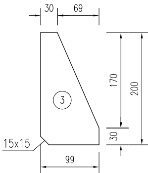
立柱法兰肋板
