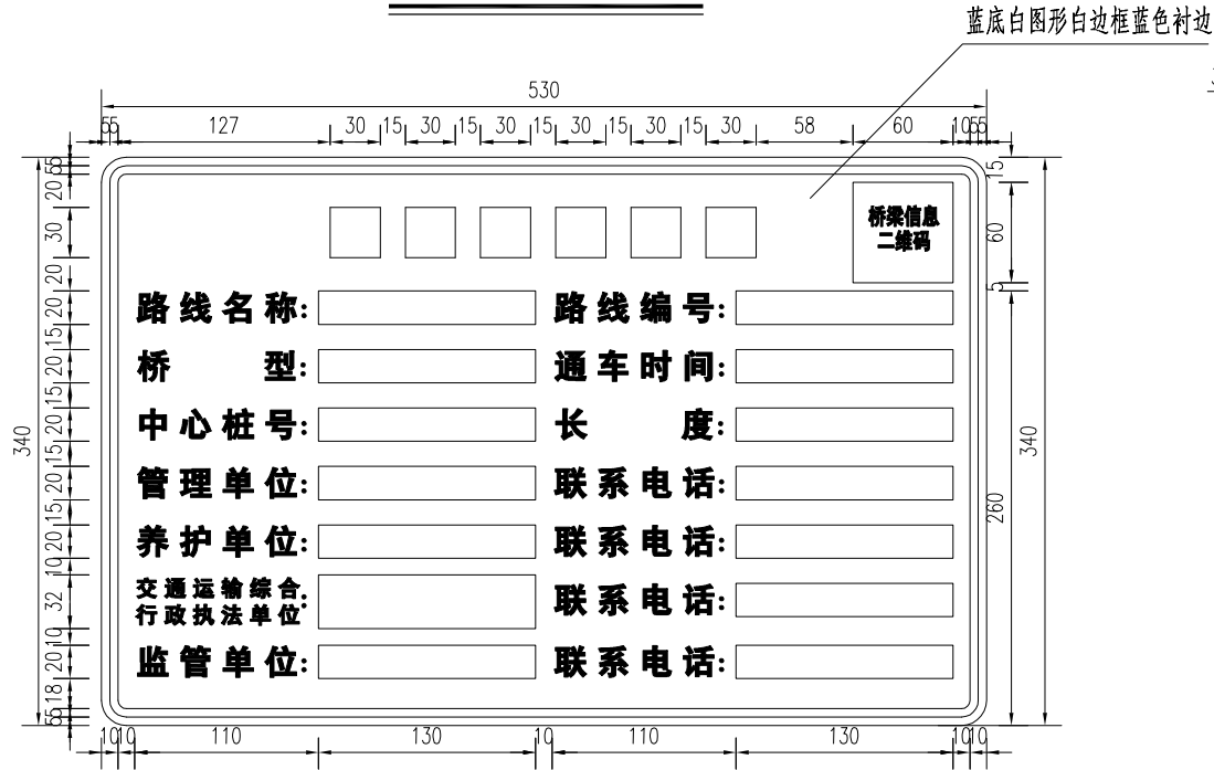
桥梁信息公示牌
