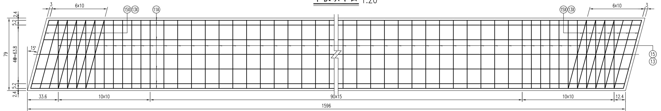
中板底平面 1:20
