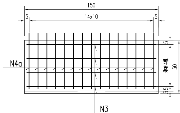
上挡板钢筋平面图
