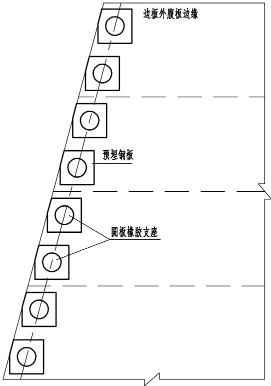
支座安装大样
