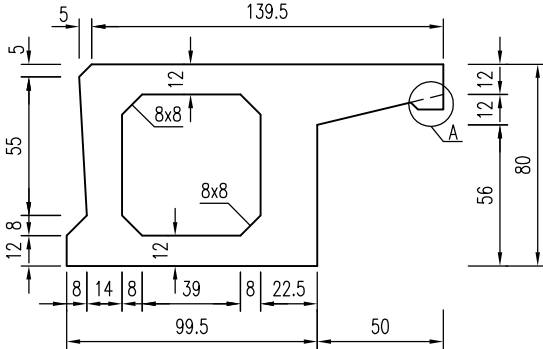
边板断面 1:30
