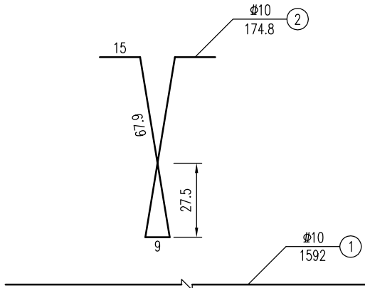
一道铰缝数量表
