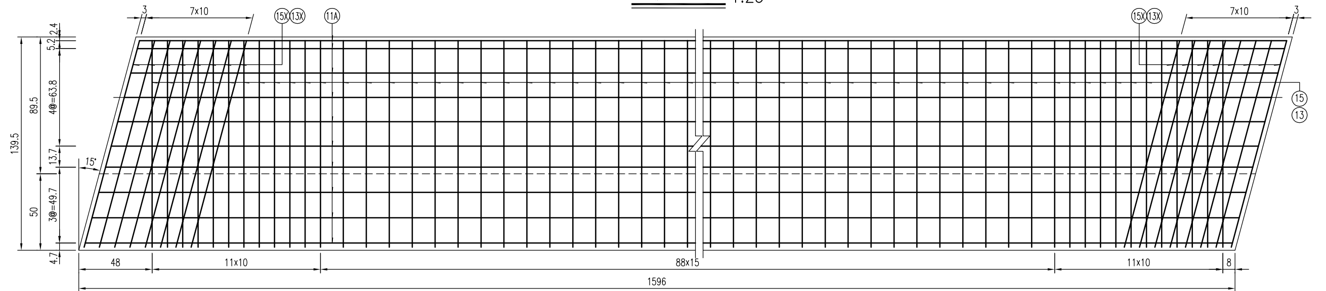
边板底平面 1:25
