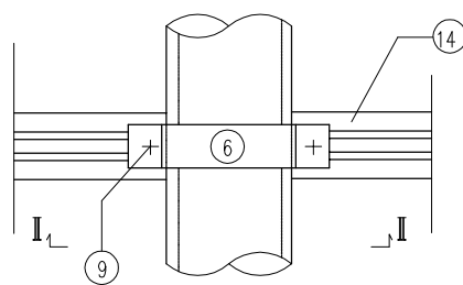
A大样
