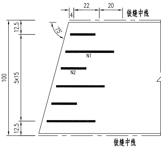
中板梁顶面伸缩缝钢筋预埋平面
