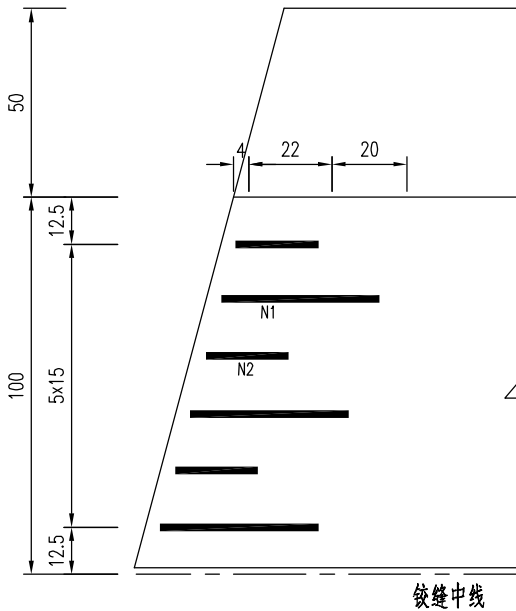
边板梁顶面伸缩缝钢筋预埋平面
