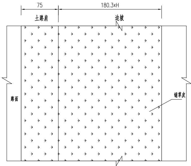
铺草皮护坡平面
