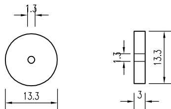
混凝土定位块大样
