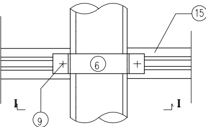
A大样
