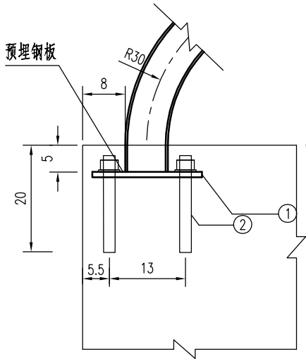
A大样
