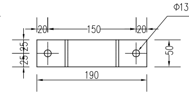
铝合金龙骨截面
