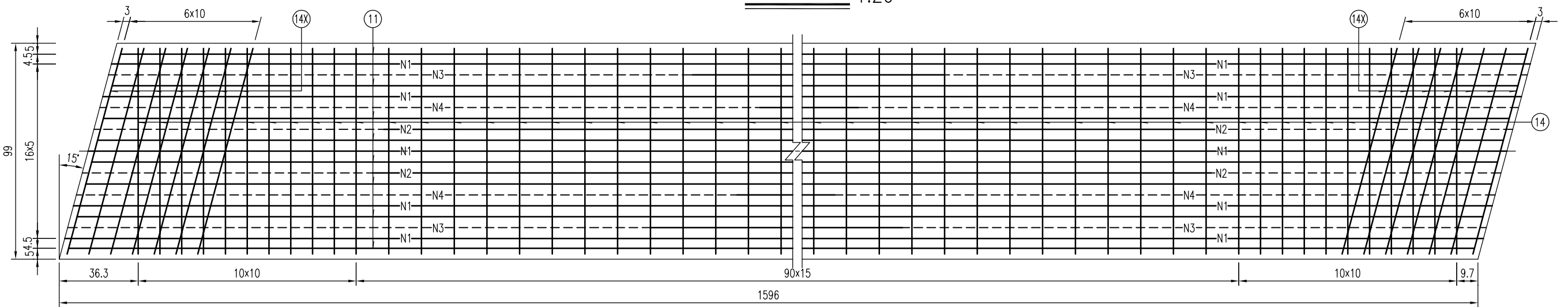
中板底平面 1:20
