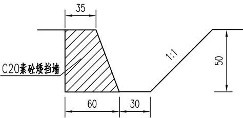
台背回填示意 1:100
