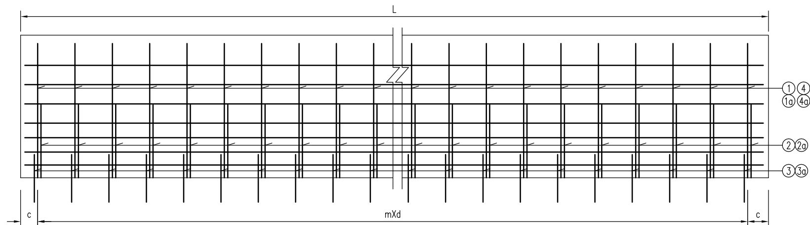
组合式护栏钢筋平面 1:20
