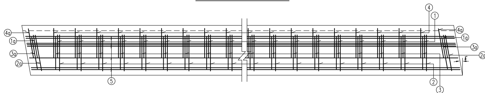
组合式护栏钢筋平面 1:20
