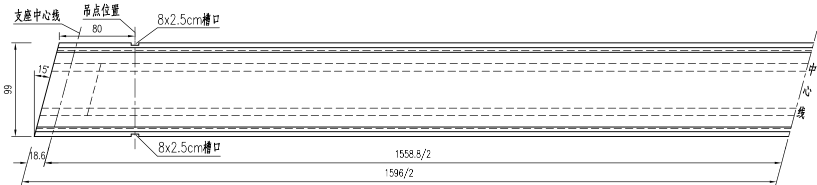
1/2中板平面 1:40
