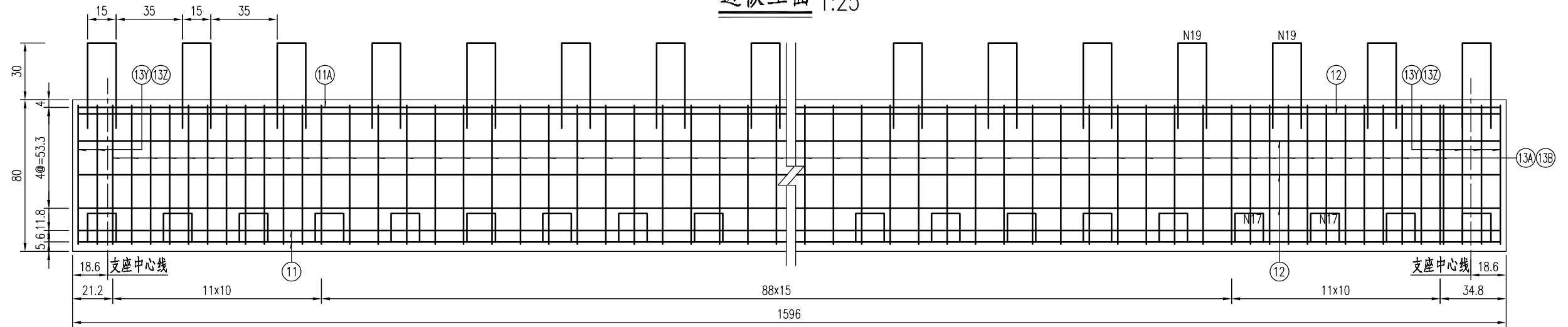
边板顶平面 1:25
