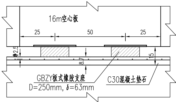
支座垫石布置示意（16m）
