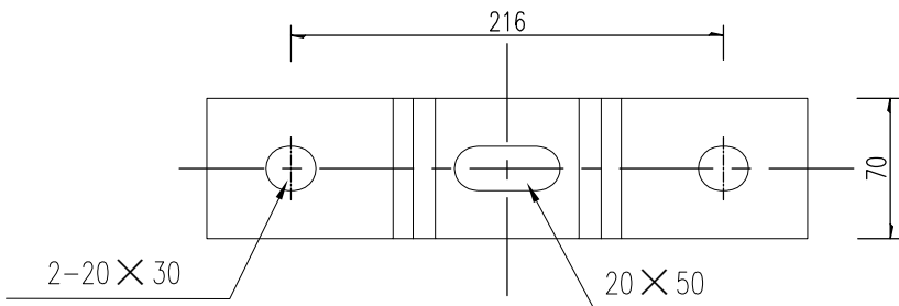
托架平面图 1:4
