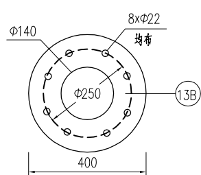
基础锚板平面
