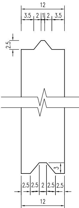
挡板齿口大样图
