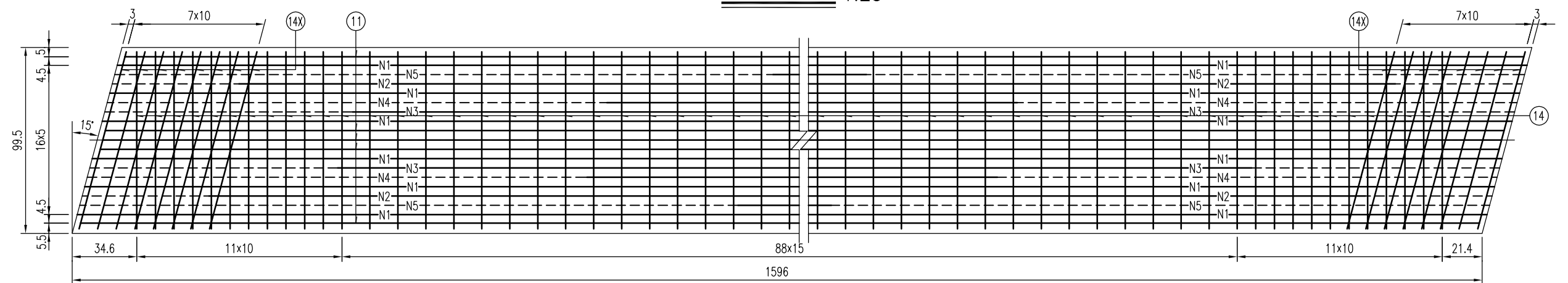
边板底平面 1:25
