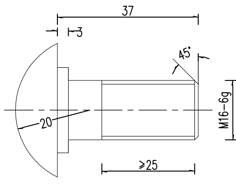
拼接螺栓JI-3 1:1
