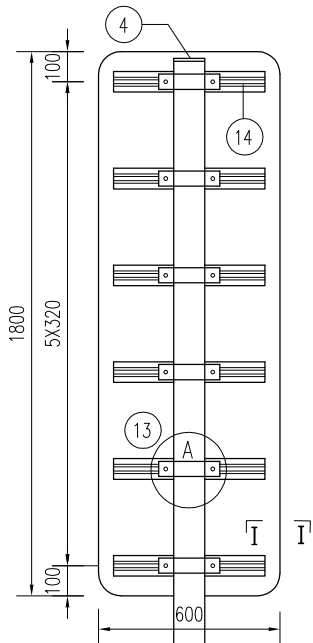
A大样
