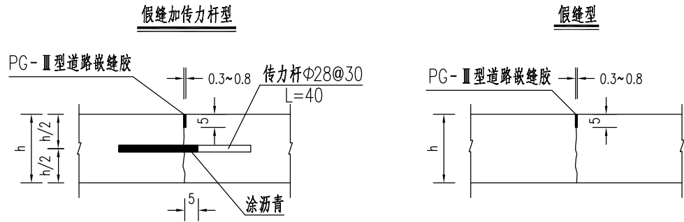
灌缝示意图
