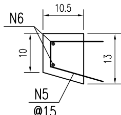
牛腿钢筋立面图
