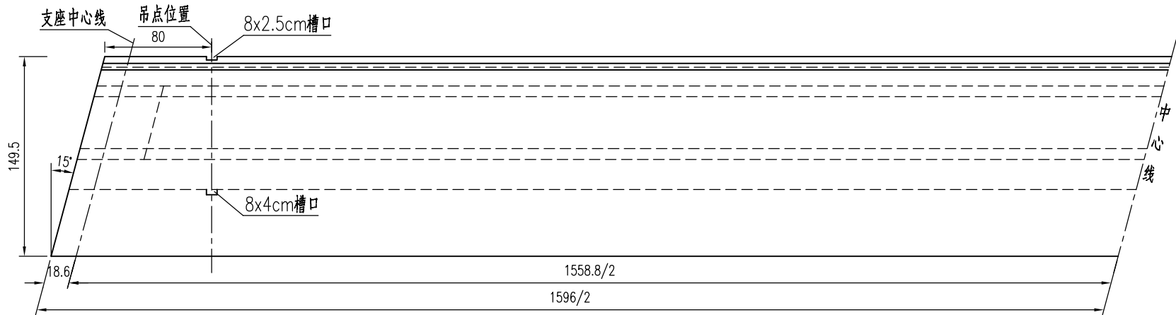
1/2边板平面 1:40
