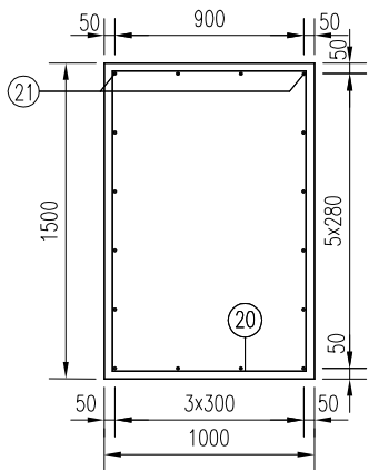
基础钢筋平面
