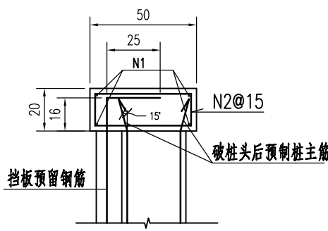
桩顶与挡墙压顶连接构造图
