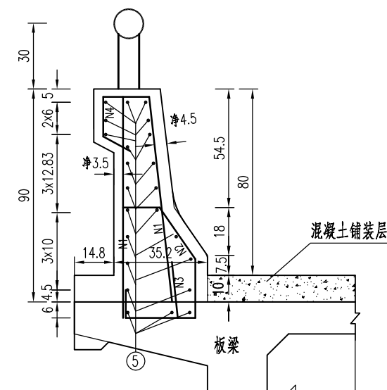
组合式护栏钢筋横断面 1:20
