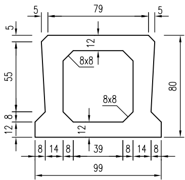
中板断面 1:30
