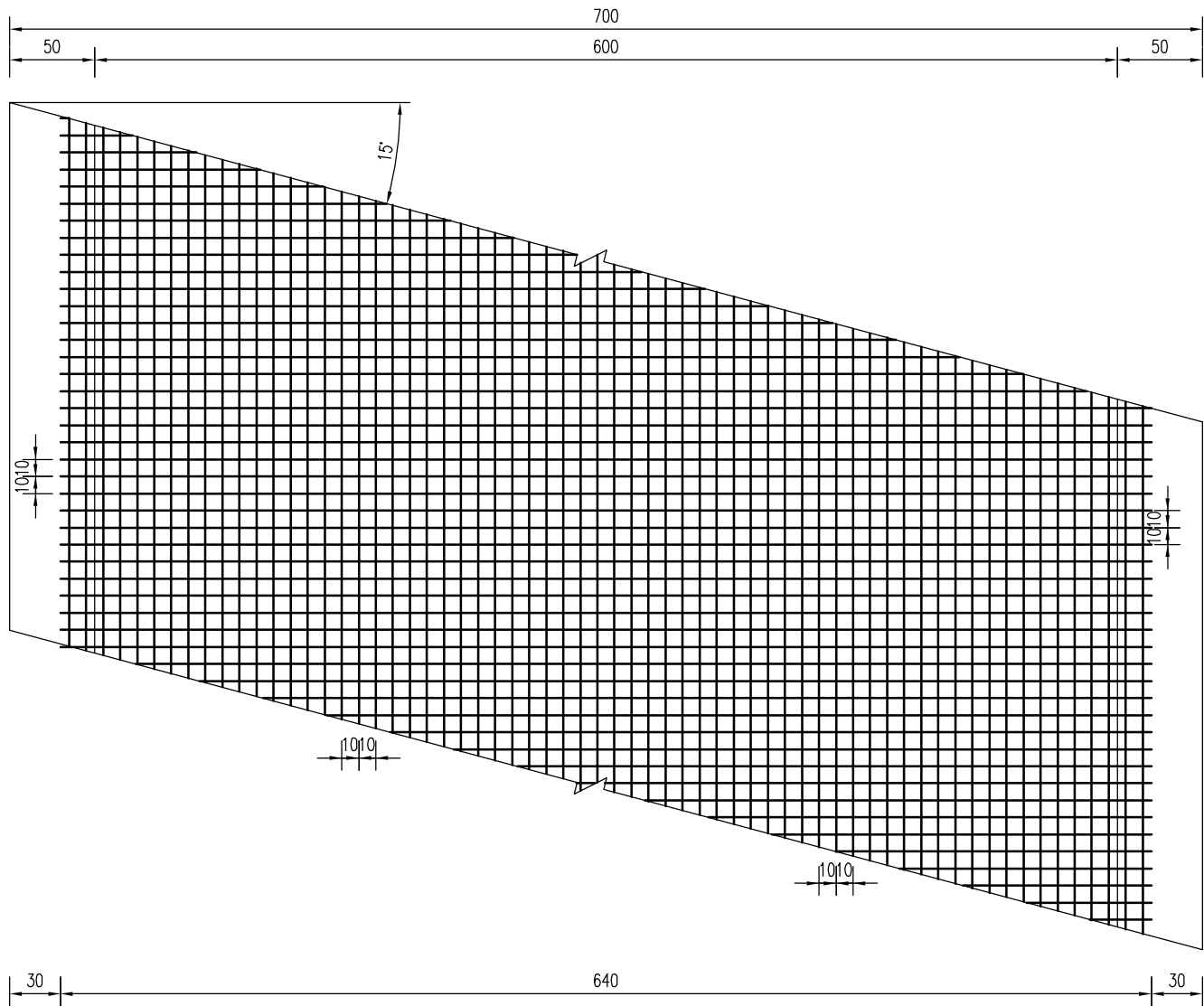
桥面铺装钢筋网平面
