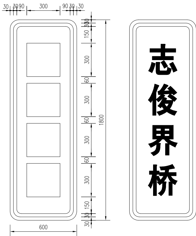
桥名牌标志
