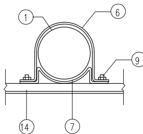
II-II
