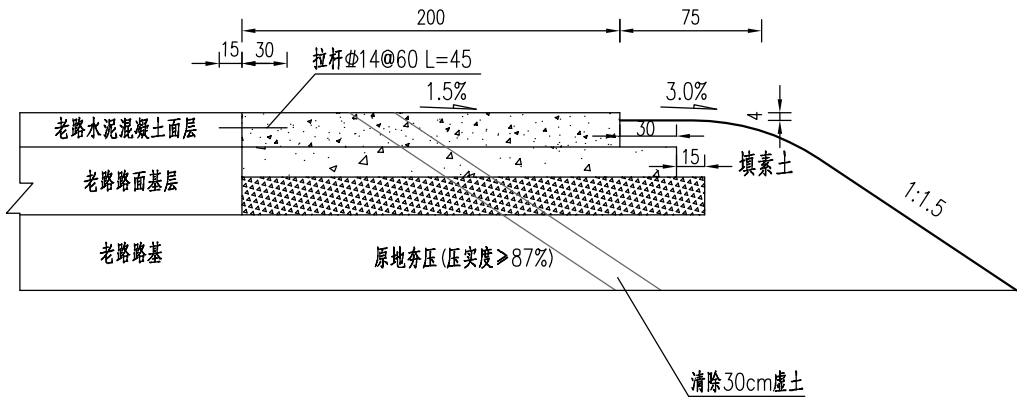
拼宽侧路肩边部构造图
