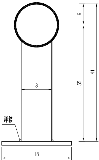
钢板大样 1:5
