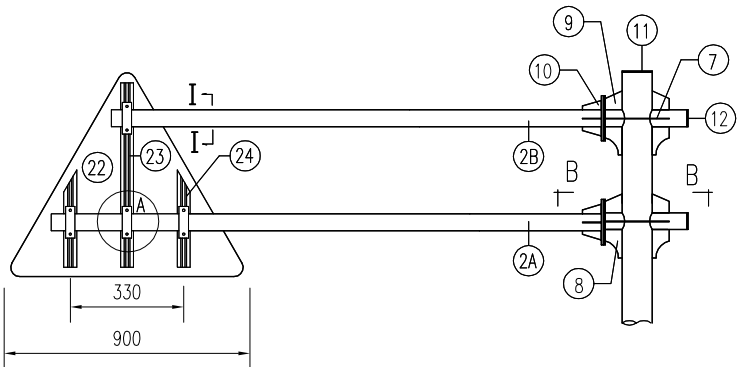
立柱法兰平面
