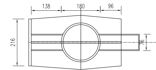
B-B剖面
