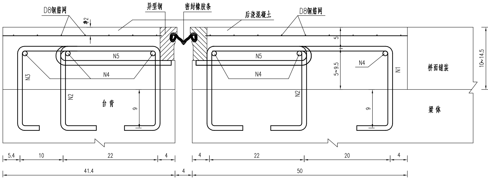
伸缩缝构造正立面
