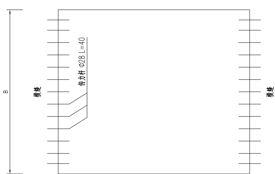
换板设计图
