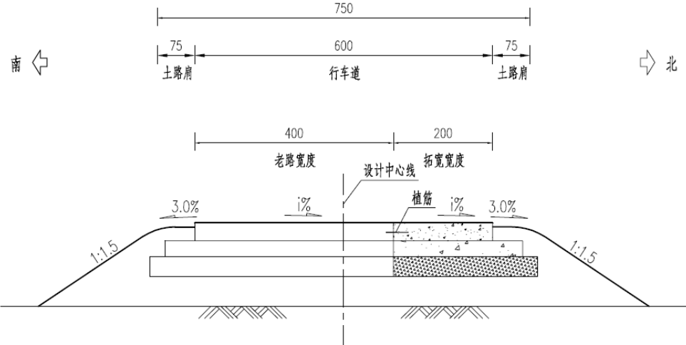
路基标准横断面图
