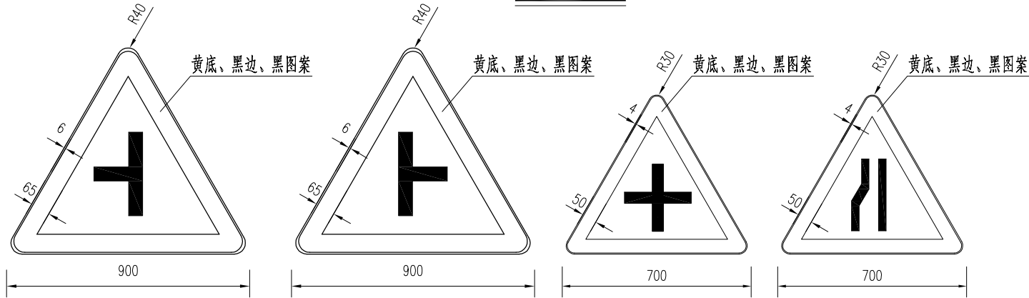
警告标志
