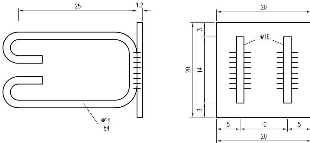
预埋件B大样 1:5
