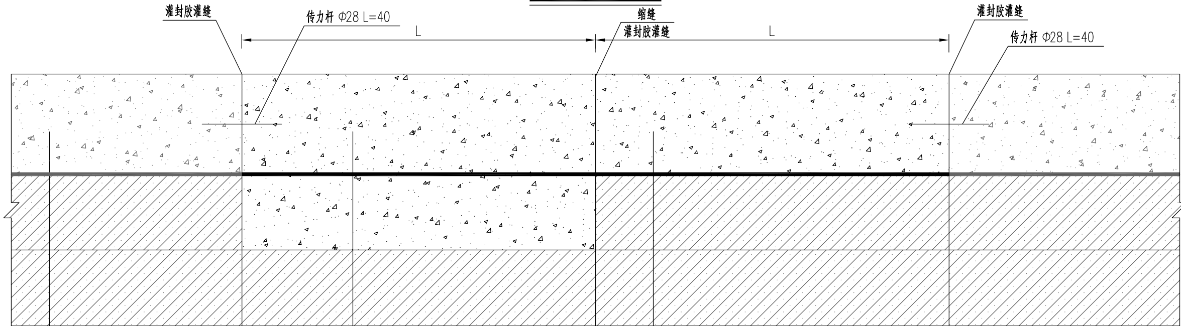
基层挖补示意图
