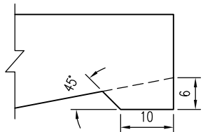
滴水檐A大样
