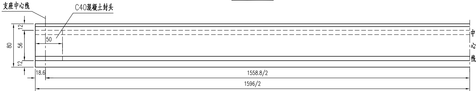
1/2立面 1:40
