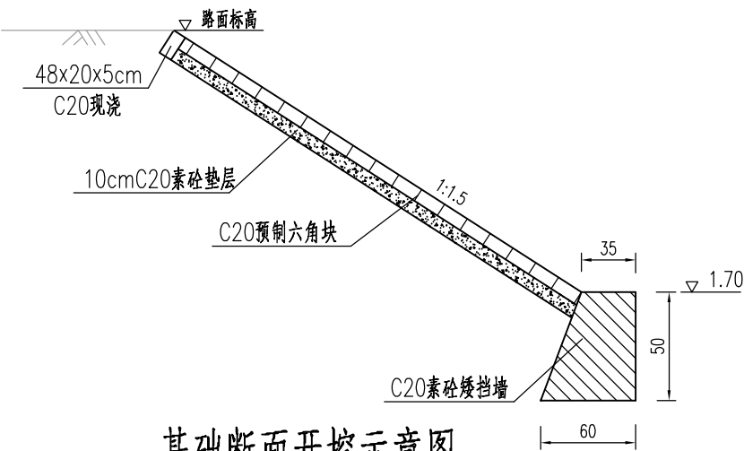
台后铺砌结构示意图 1:50
