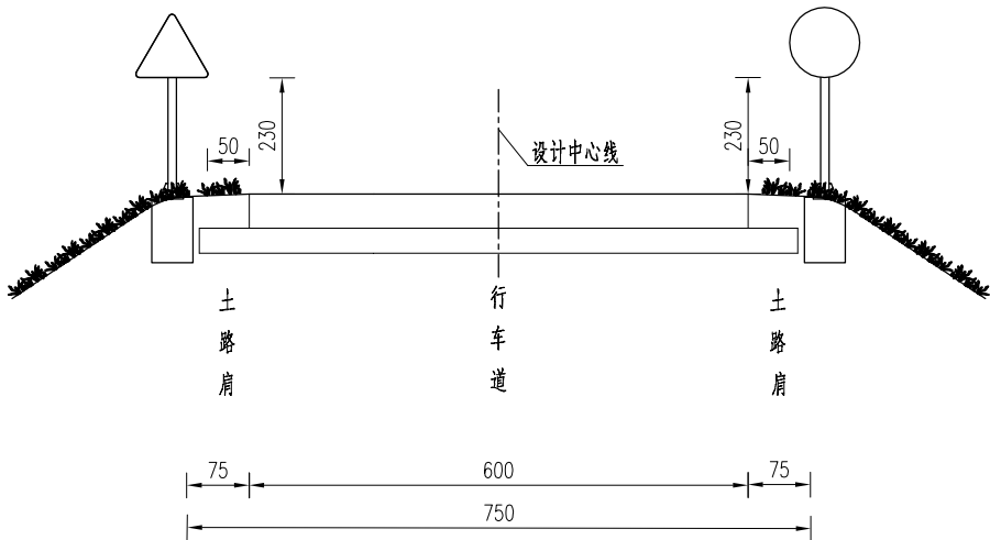
安全设施标准横断面图
