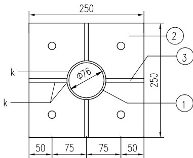
A大样
