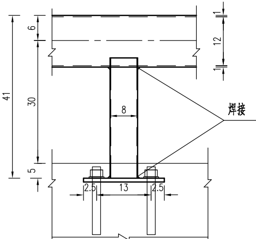
A-A 1:10
