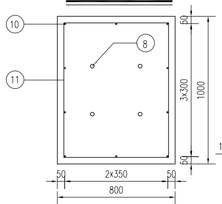
基础钢筋立面
