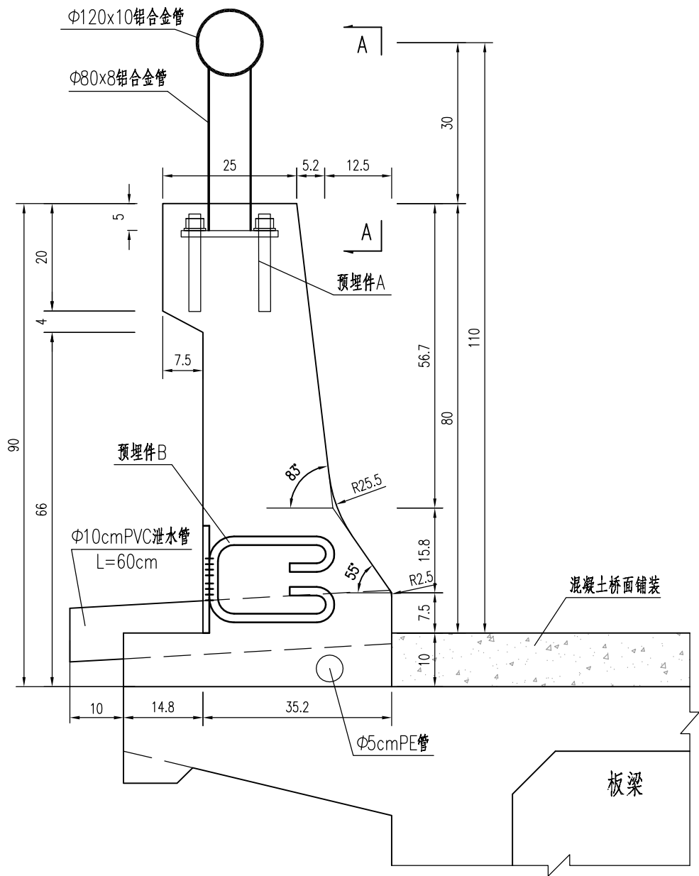
组合式护栏横断面 1:10
