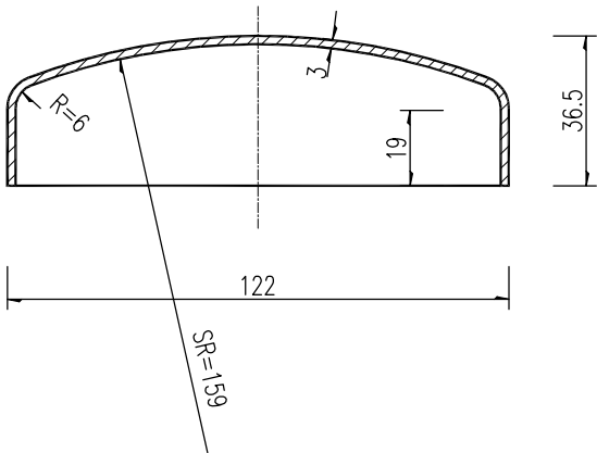
帽盖
