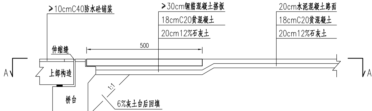
A-A
