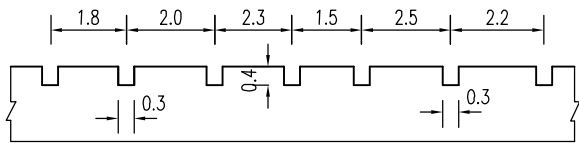
桥面刻槽大样
