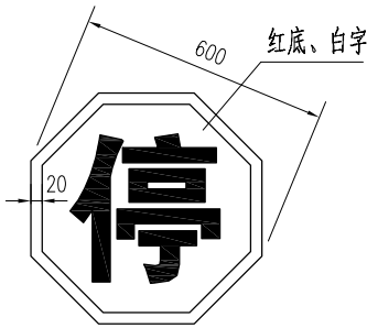
停车让行标志
