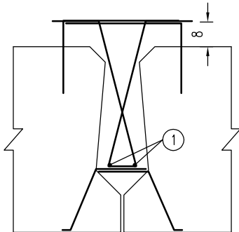
铰缝钢筋施工大样
