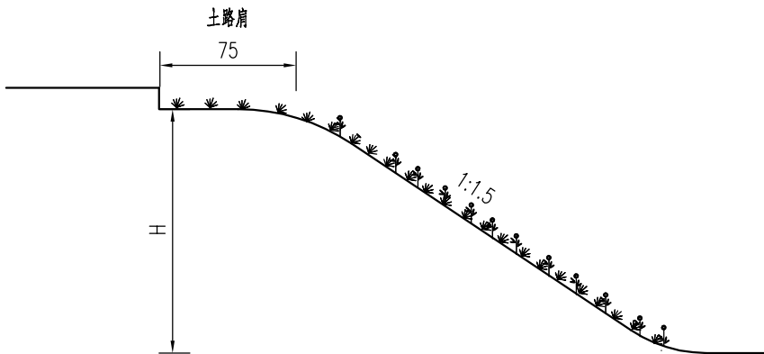
铺草皮护坡剖面
