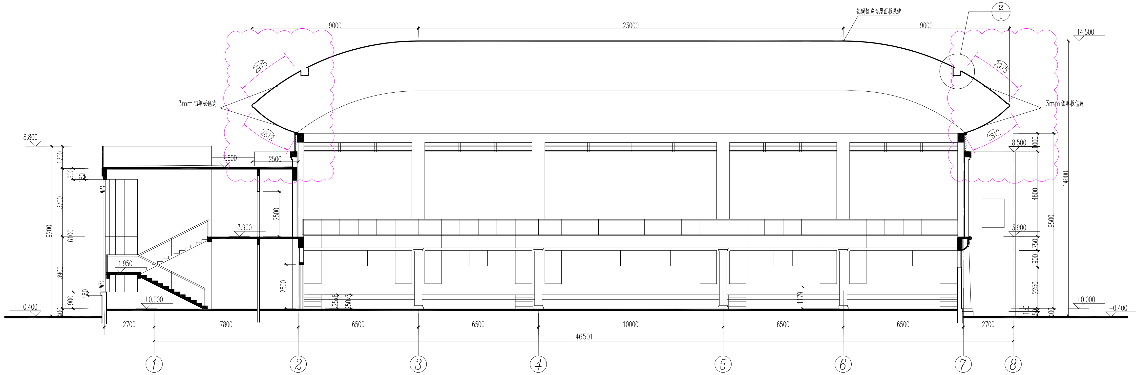
A-A剖面图 1:100
