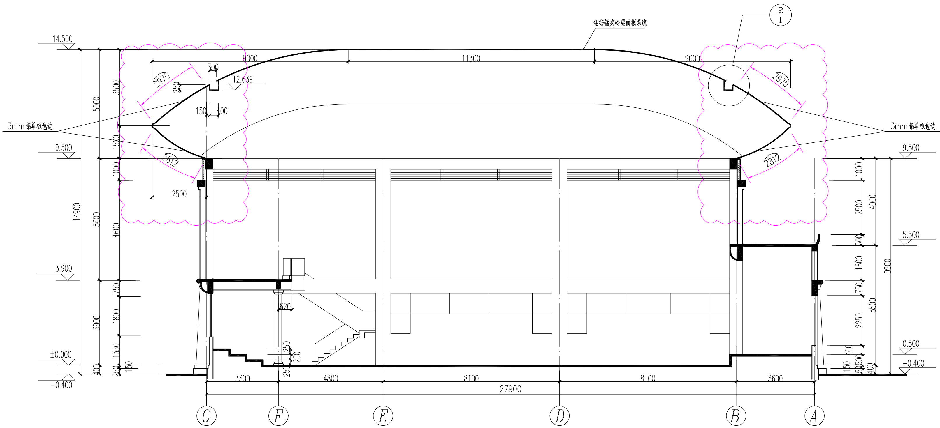
B-B剖面图 1:100
