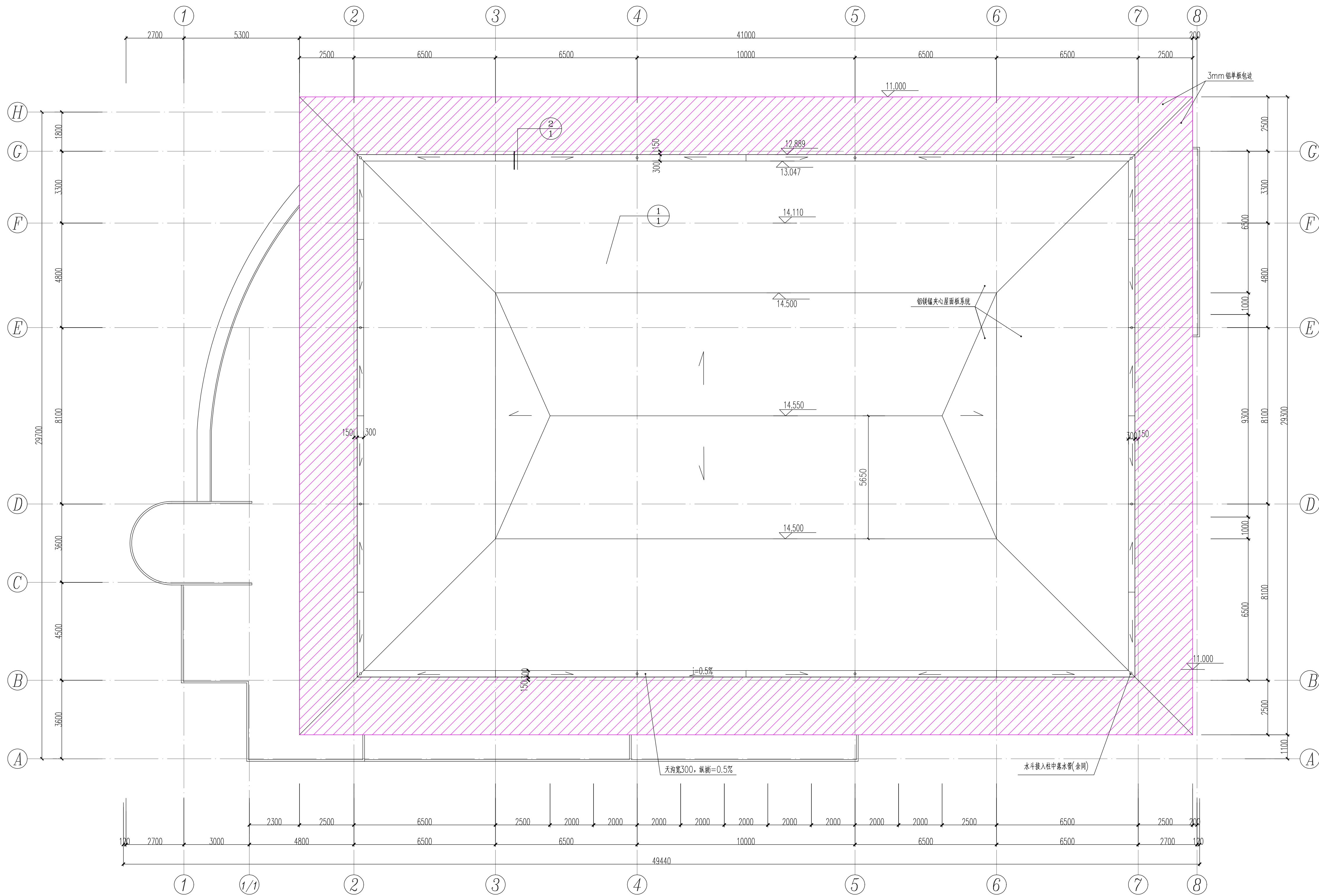
改造后屋顶平面 1:100
