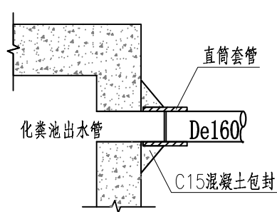
化粪池接出水管大样图
