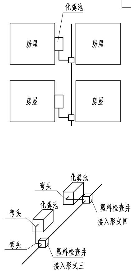
化粪池接出形式示意图 (二)
