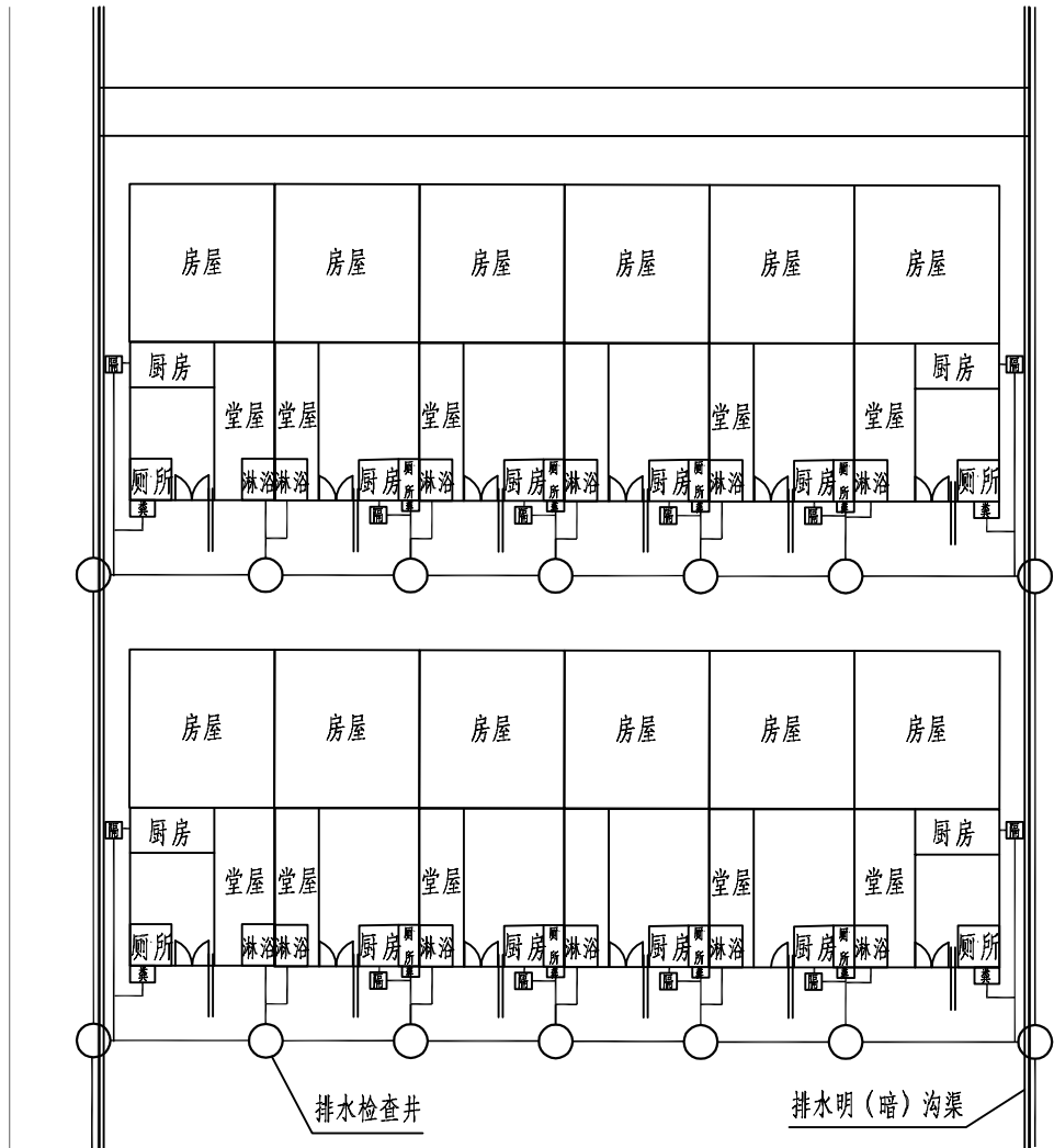
生活污水口接出形式示意图
