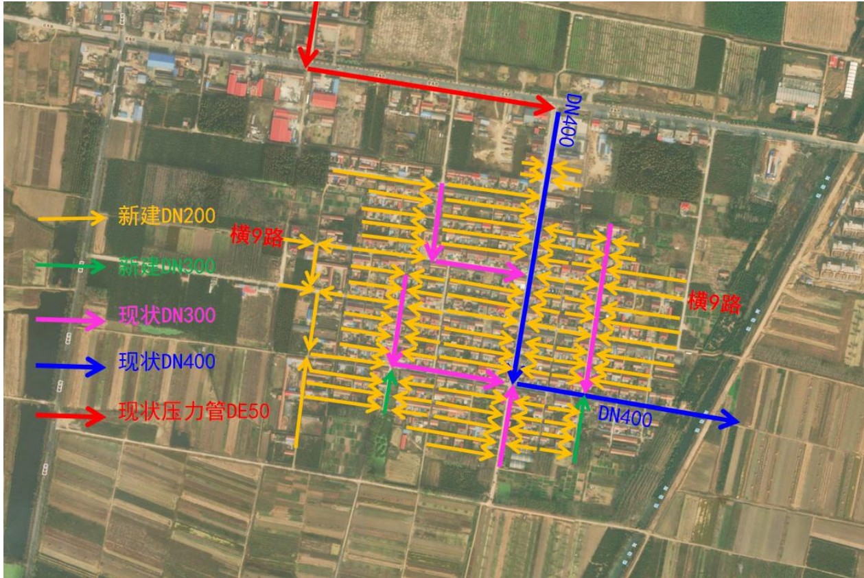
图 4-1 设计污水管线走向图
