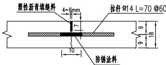
横向缩缝传力杆构造图
