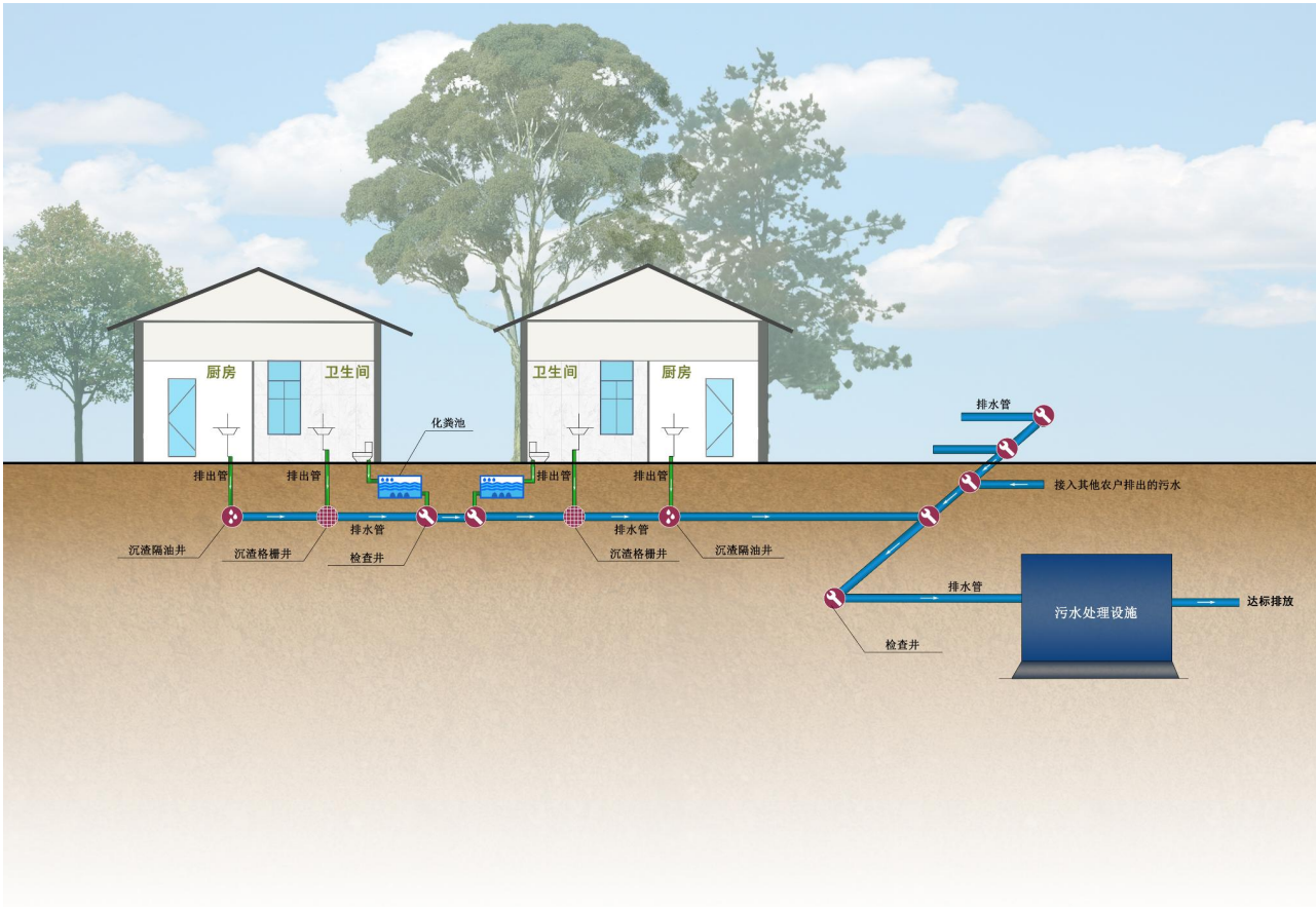
图 4-2 接户原理图
