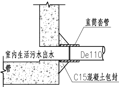
室内污水出水管大样图
