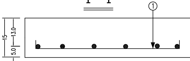
I - I
