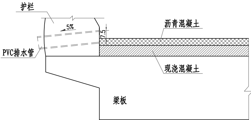
泄水管
