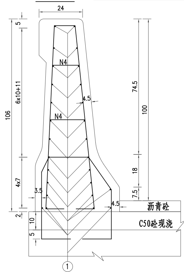
钢筋立面 1:12.5
