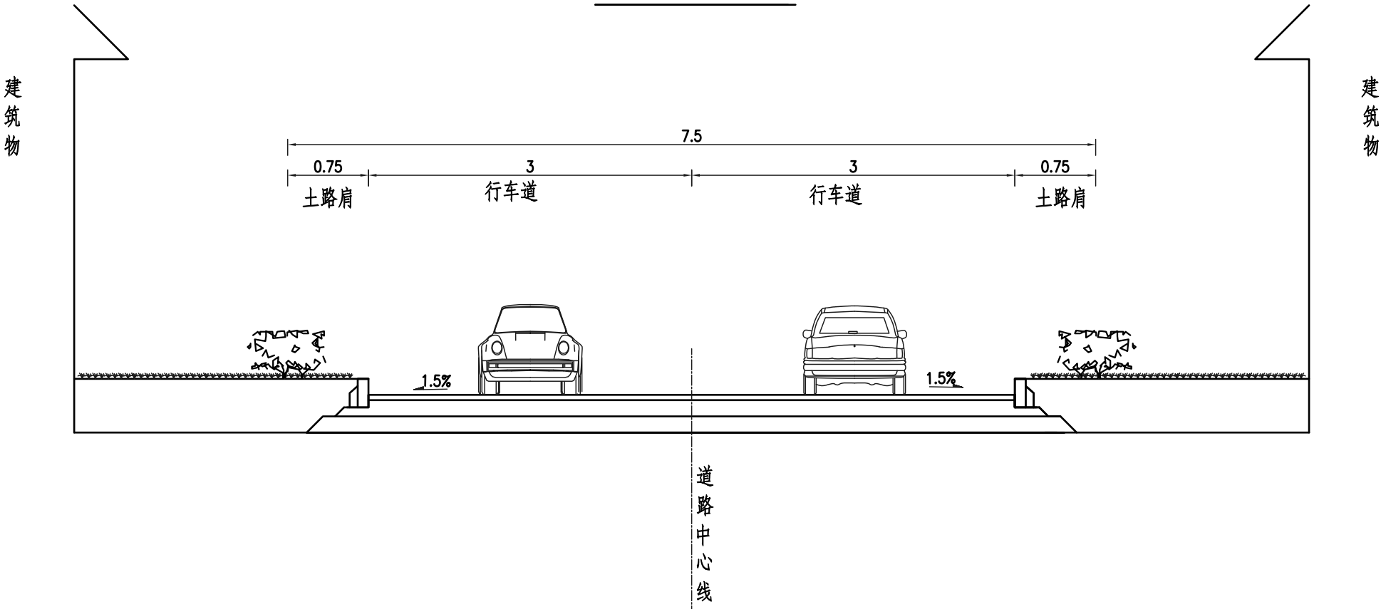
路肩防护设计图
