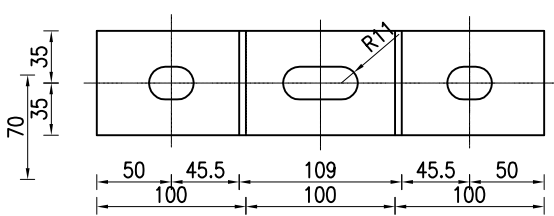
托架立面图
