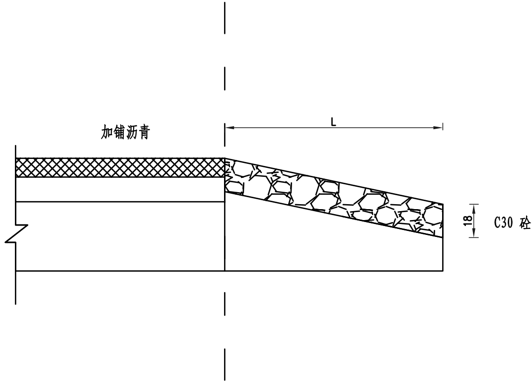
沿线地坪搭接示意图
