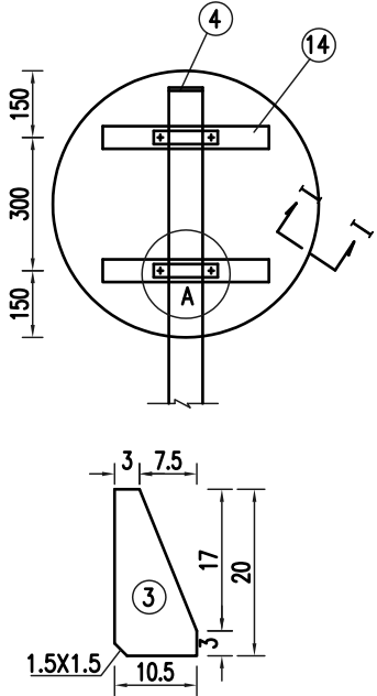
标志板背面
