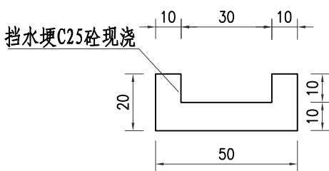
泄水槽
