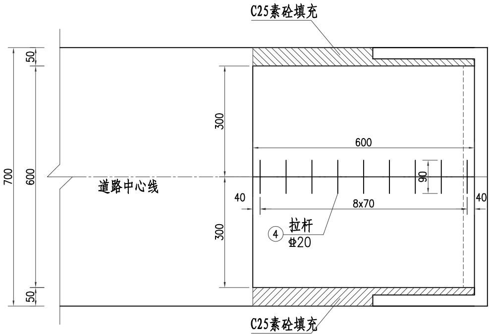
搭板平面
