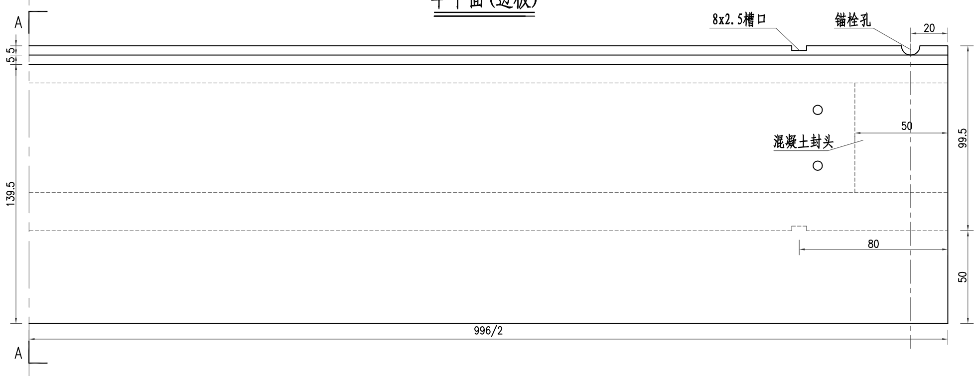
半平面 (边板)
