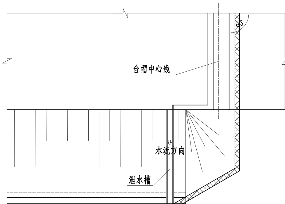
锥坡平面
