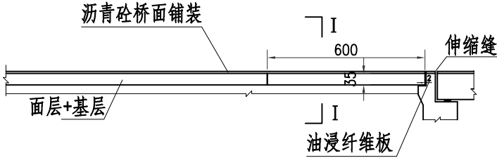
搭板立面
