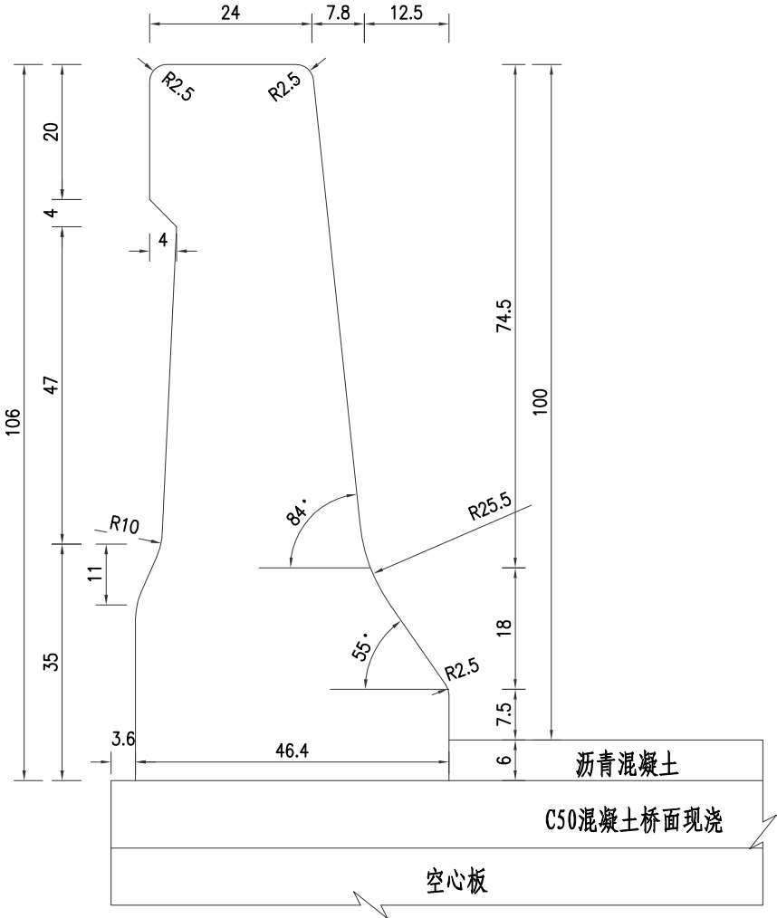
墙式护栏 1:10
