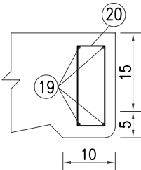
滴水檐大样
