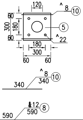
底座法兰平面
