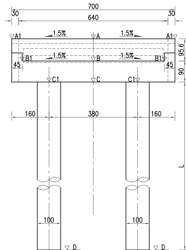
立面 1:100
