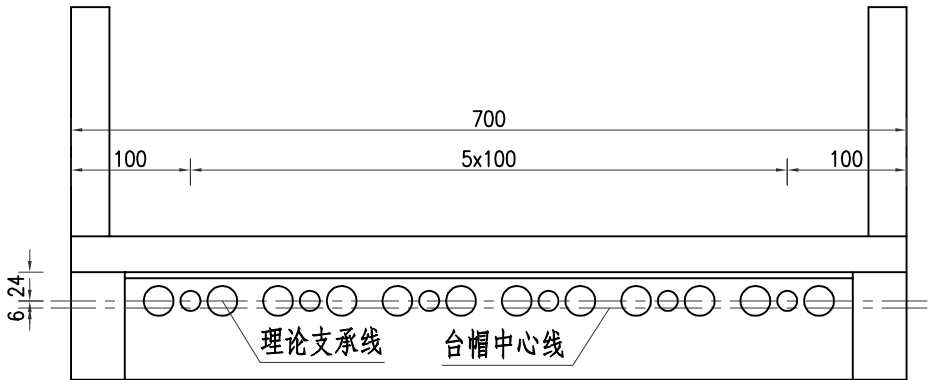
锚栓布置平面图
