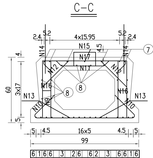
预应力筋有效长度
