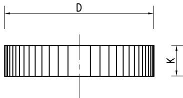
支座立面图
