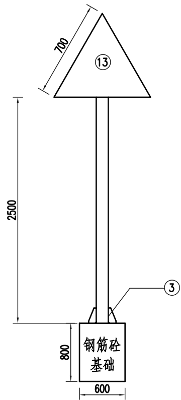
立面图
