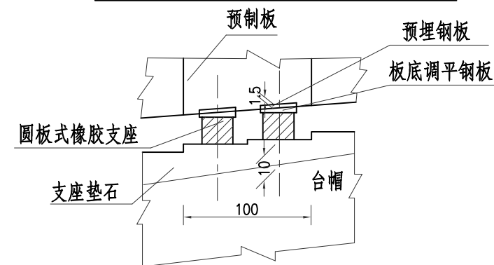
台帽顶支座布置示意图(横桥向)
