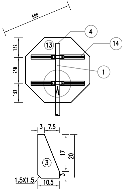
标志板背面
