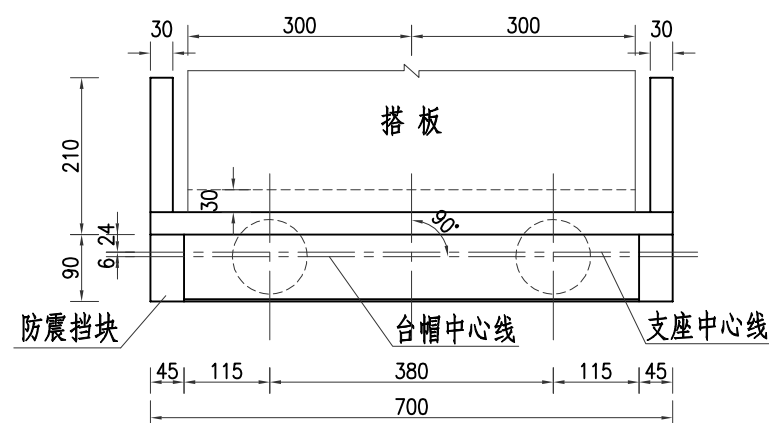
平面 1:100
