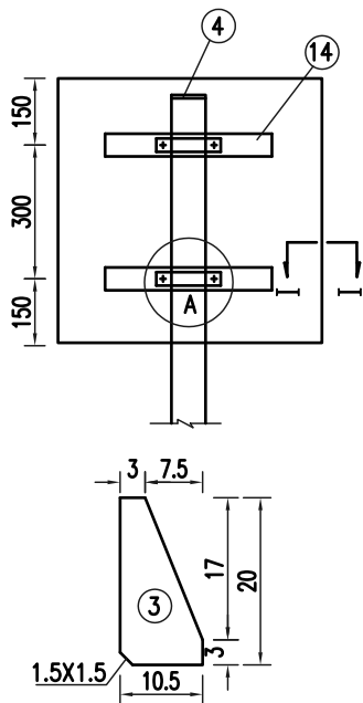
标志板背面
