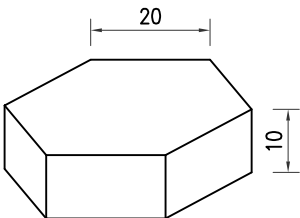
C25水泥砼预制实心六角块大样
