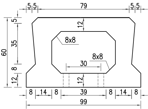
边板
