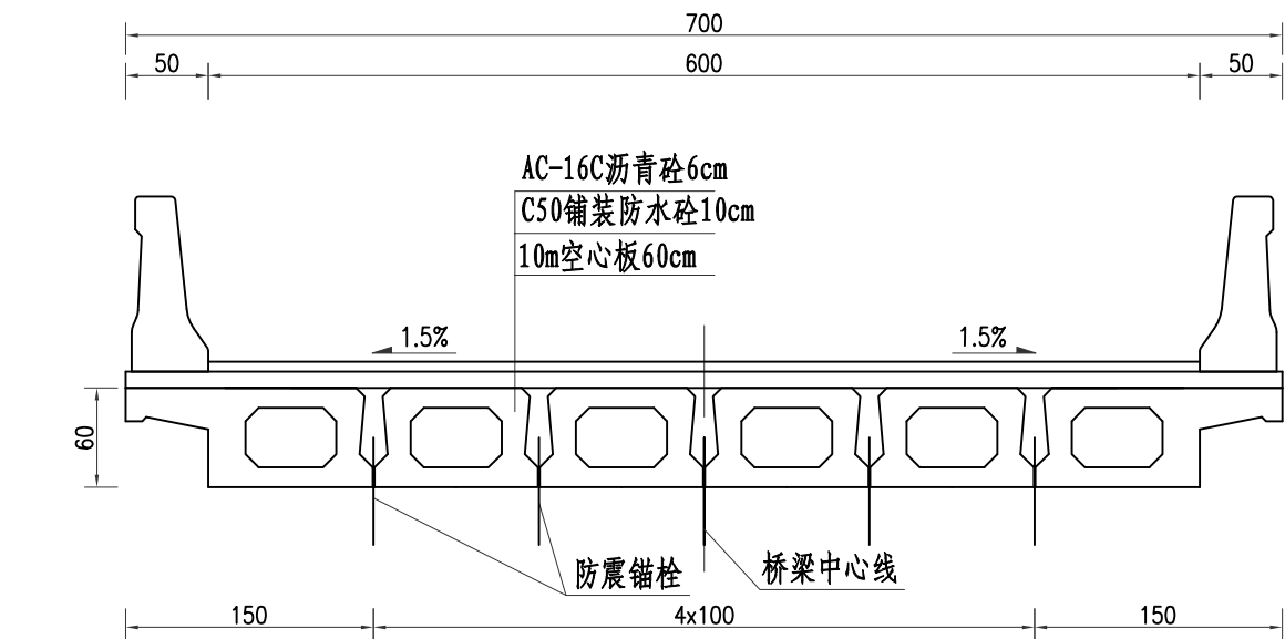
横断面
