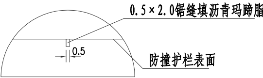
假缝大样 1:10
