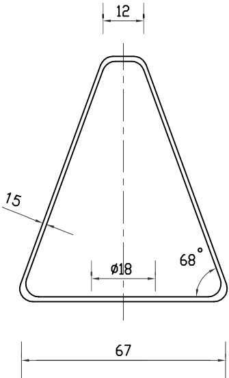
侧面图
