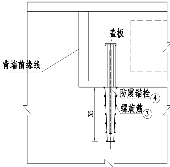
台帽锚栓孔布置图
