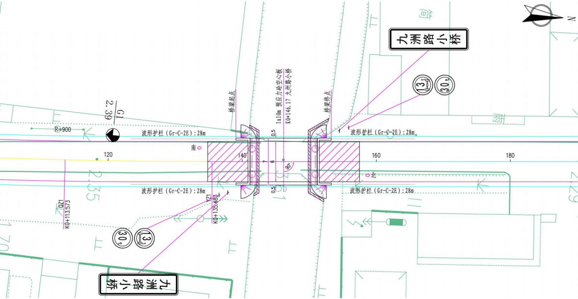
桥位布置方案
