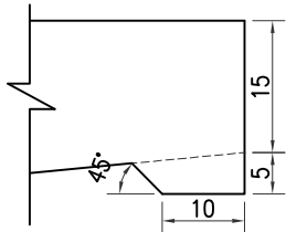
滴水檐大样
