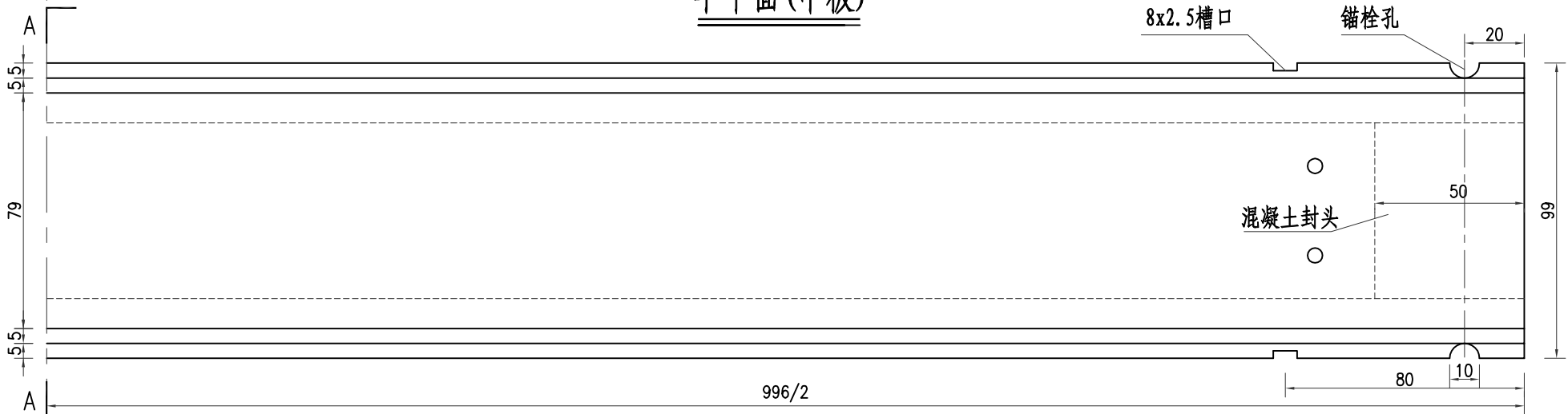
半平面 (边板)
