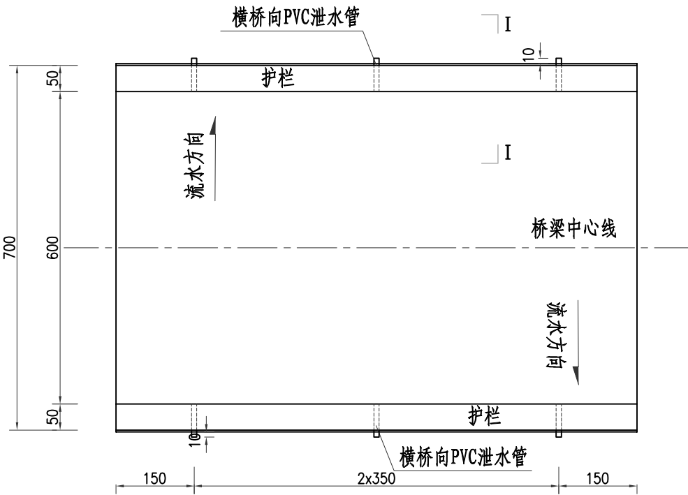
排水管平面布置图
