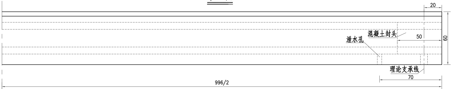
半立面
