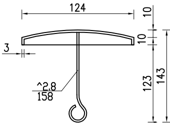
A大样
