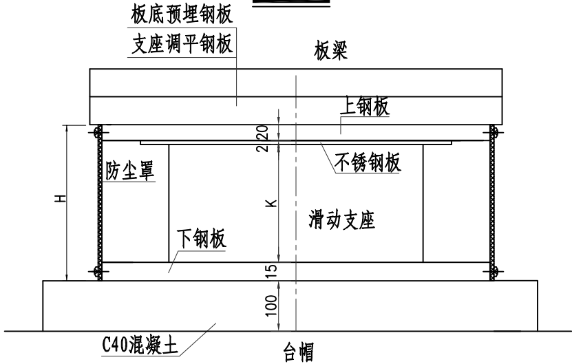
A大样
