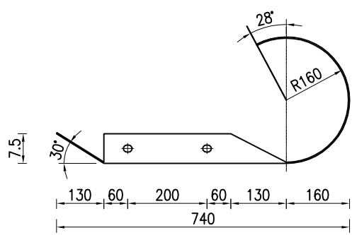
路侧护栏端头平面图 (AD型)
