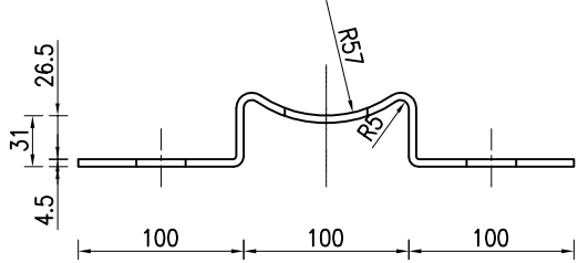
托架平面图
