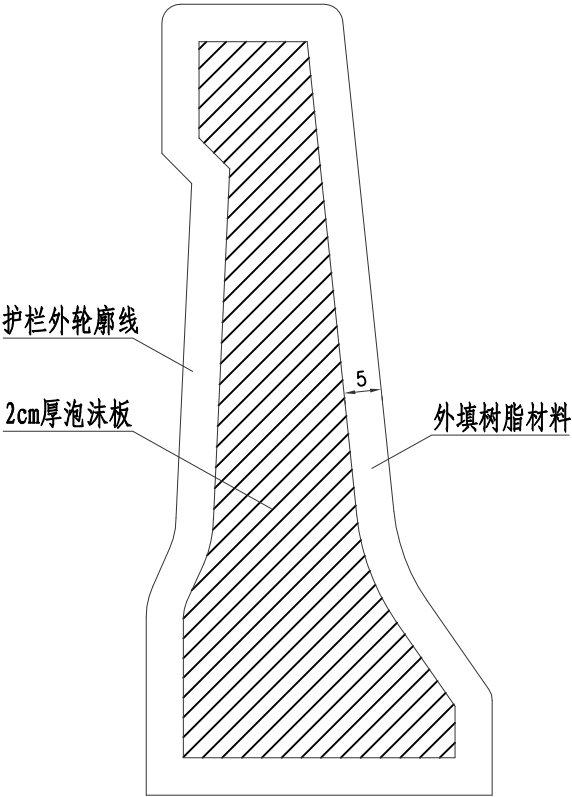
假缝大样 1:10
