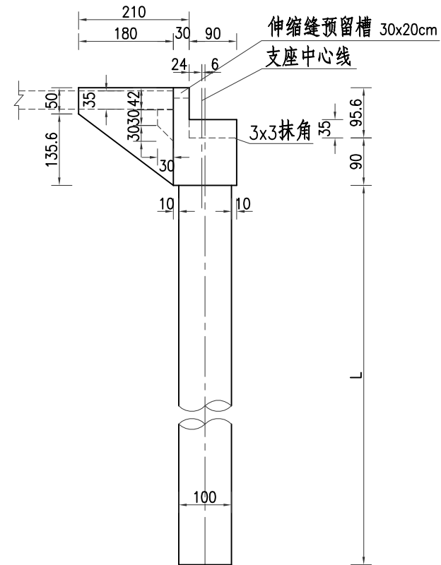
侧面图 1:100
