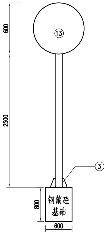
立面图
