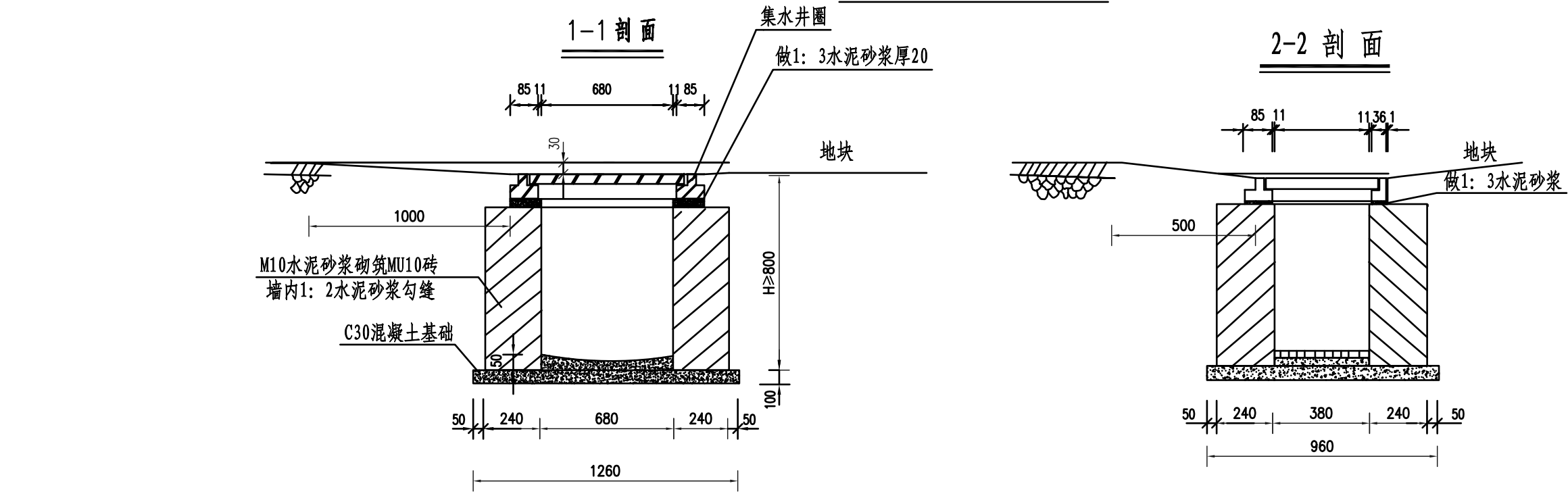
集水井及雨水管设计图
