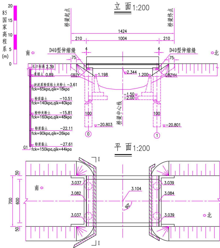
桥型布置方案
