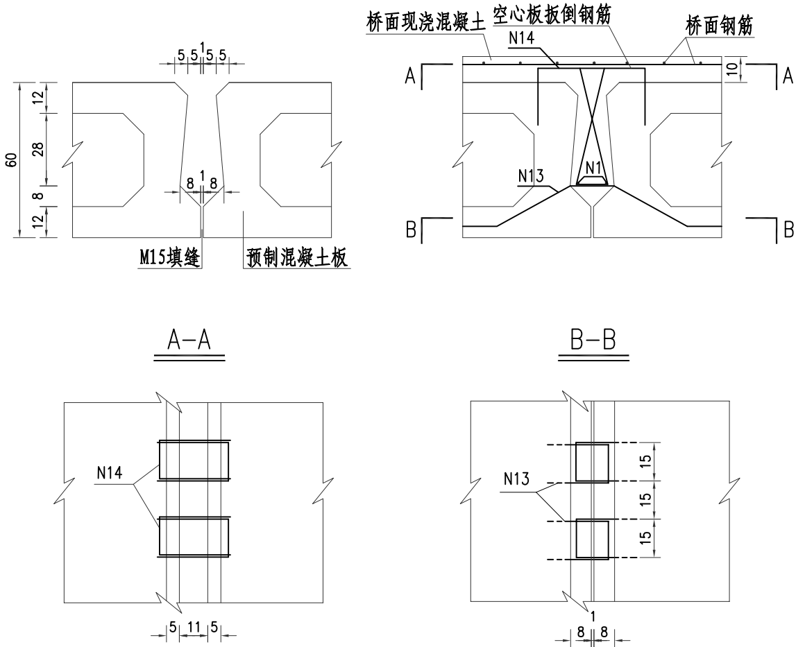
铰缝大样
