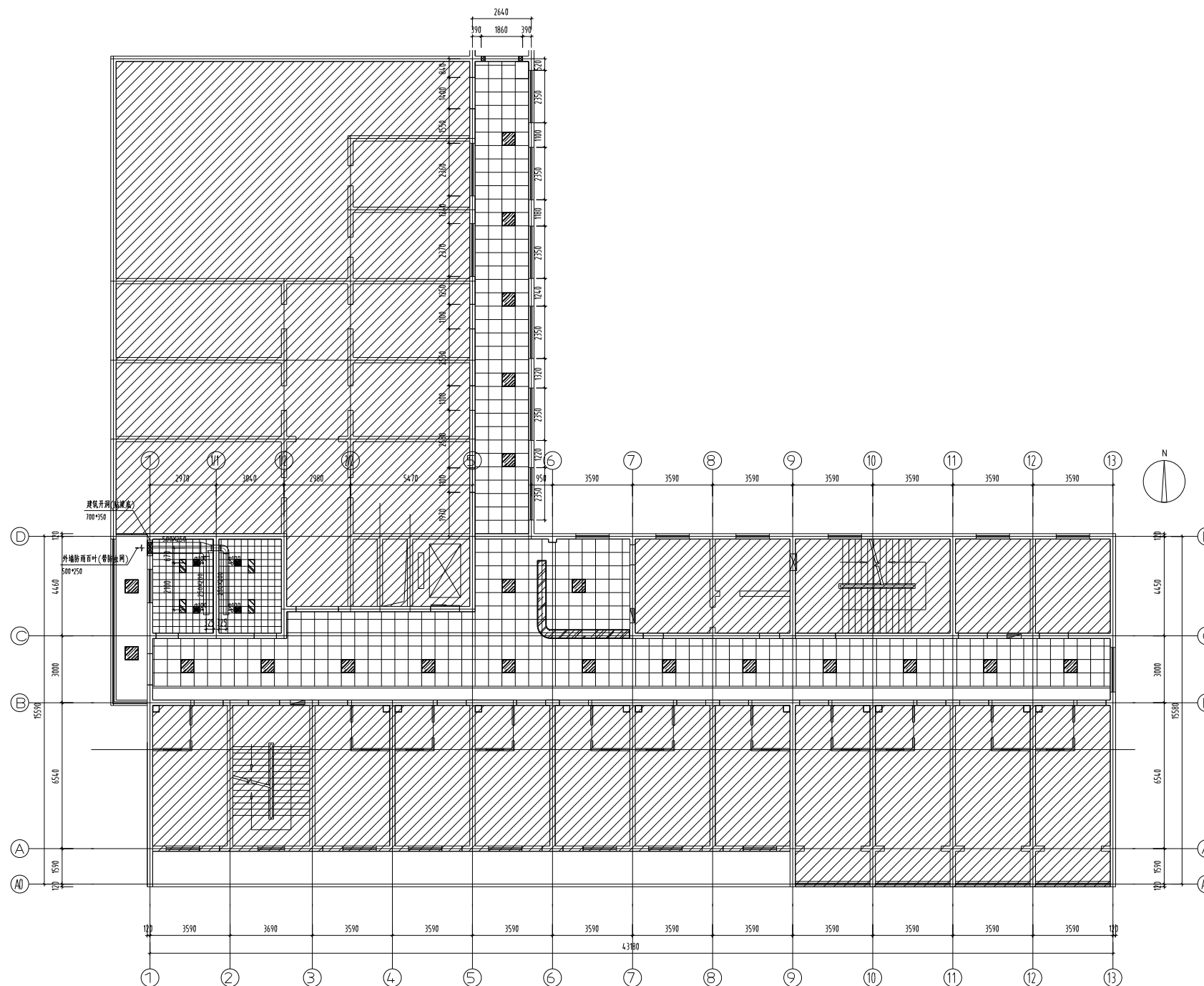
二层通风平面图1:100
