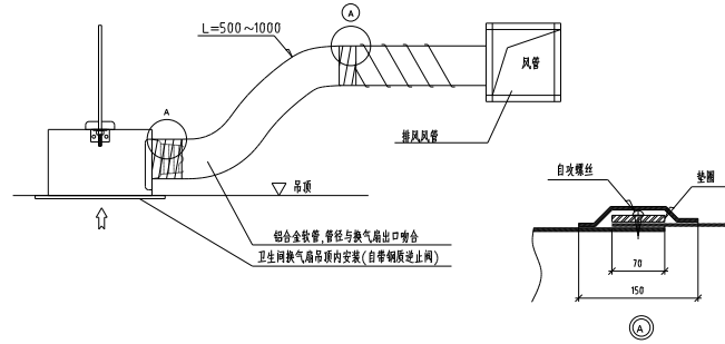
吊顶式排气扇接管示意
