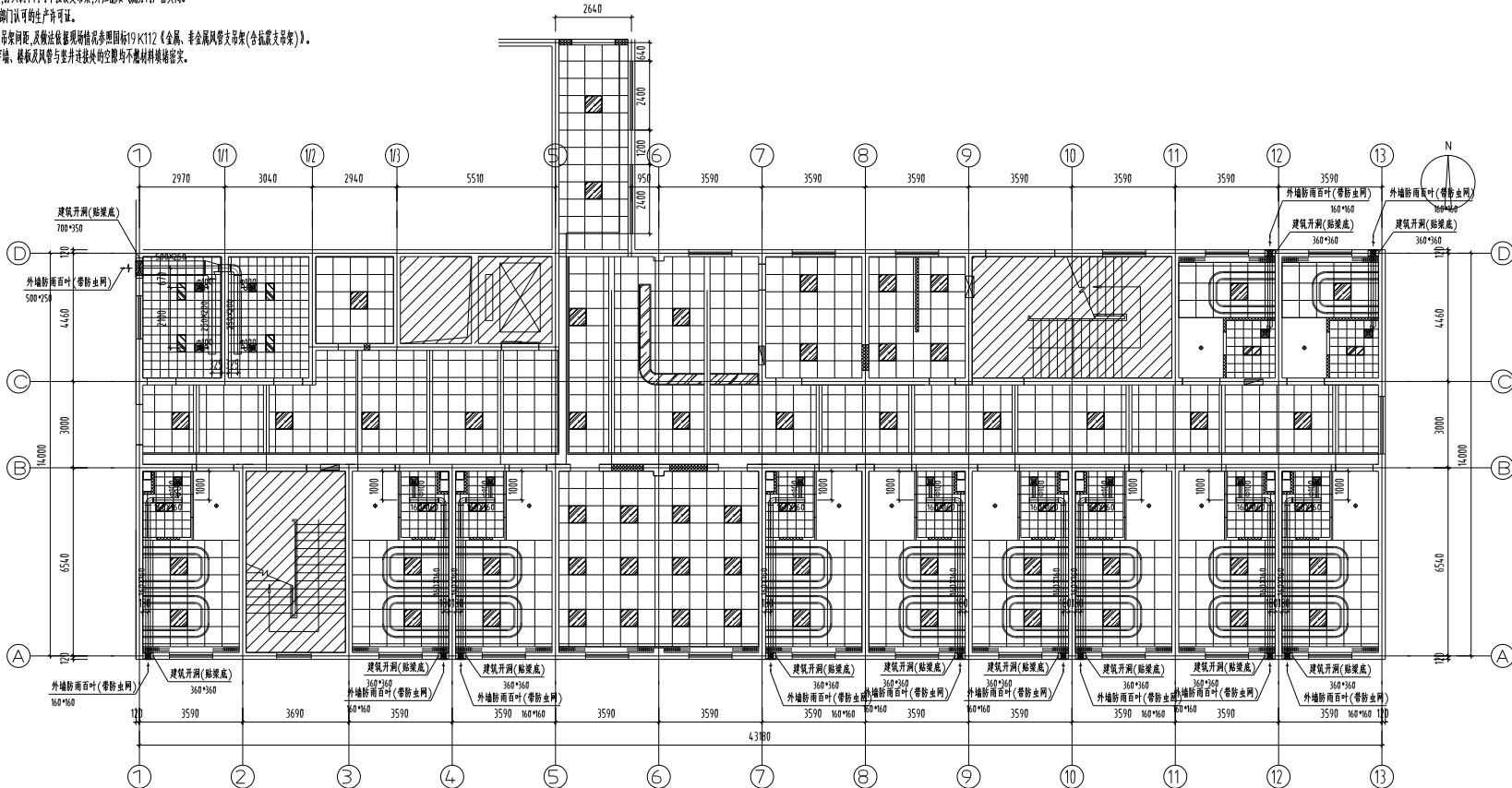
一层通风平面图 1:100
