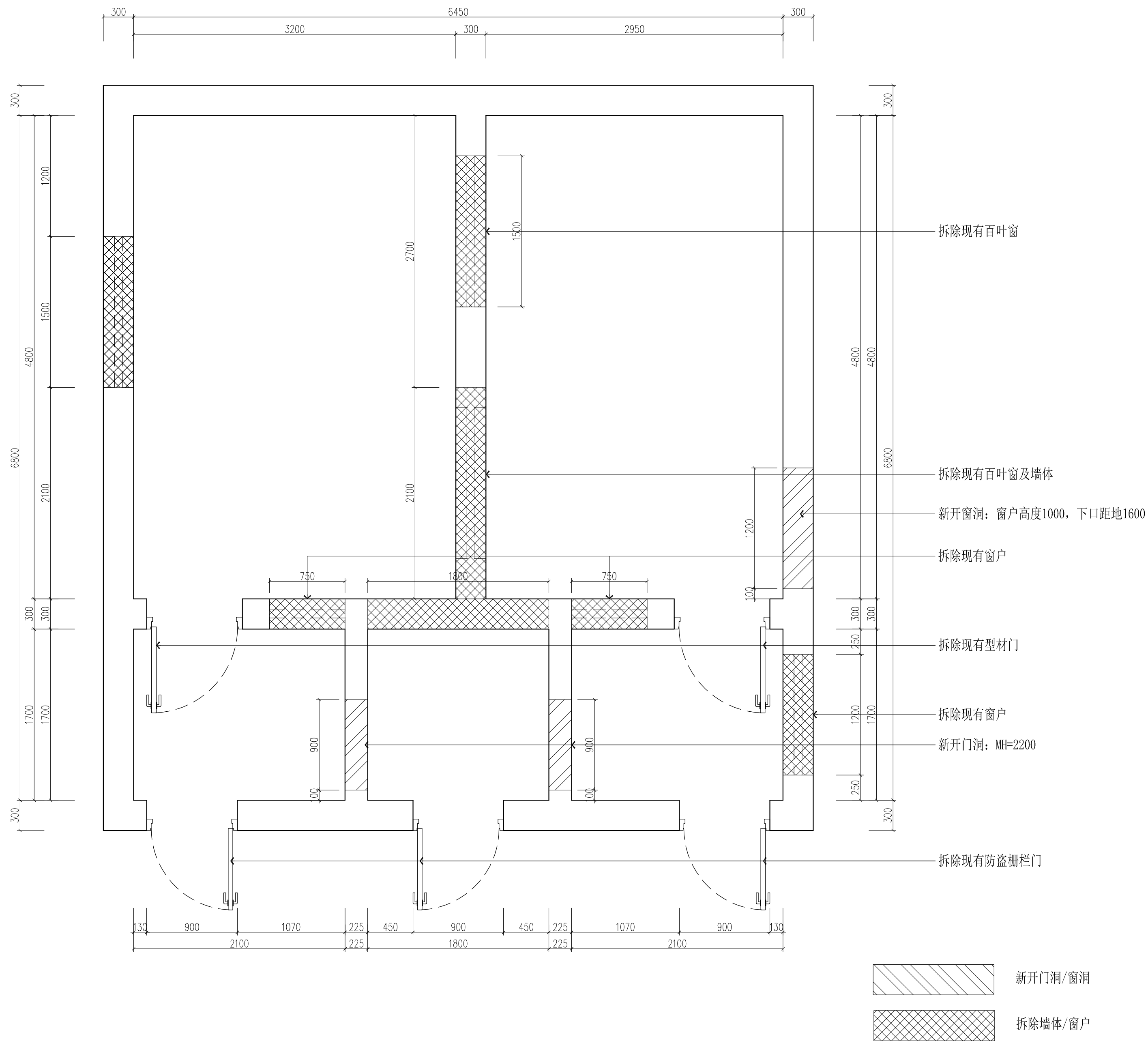
P02 P-02 墙体拆除放样图 SCALE:1/40
