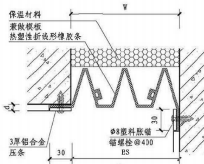
A系列外墙嵌平型变形缝
