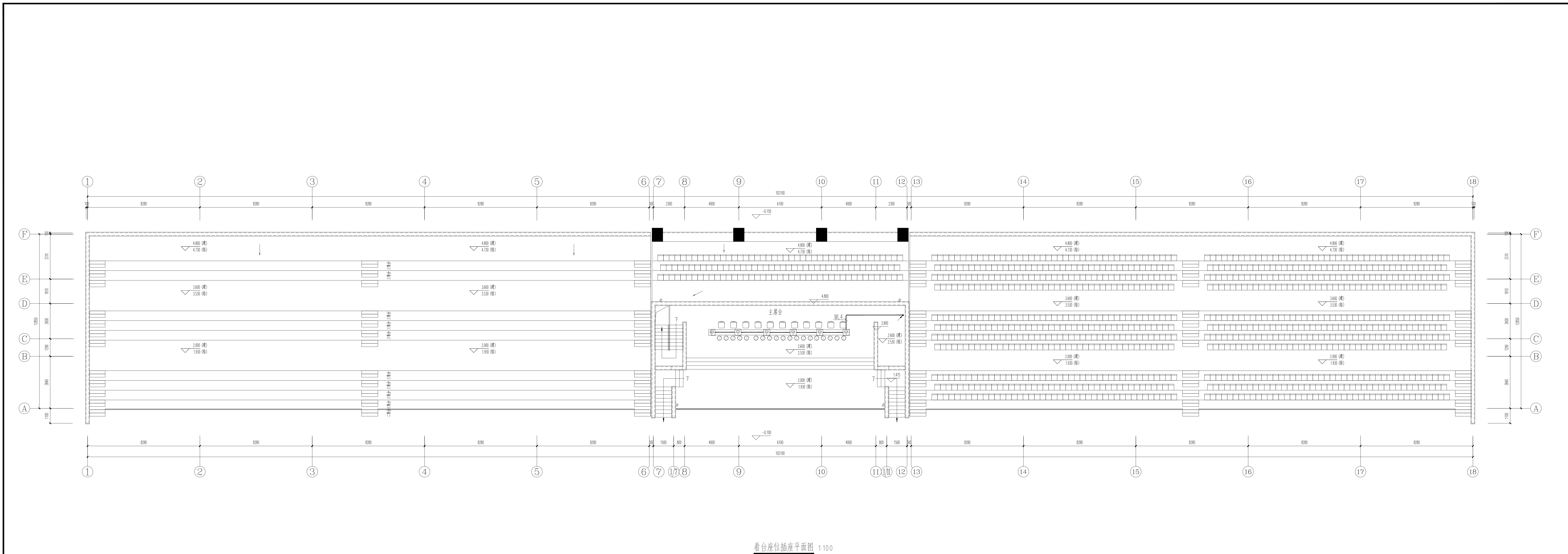
看台座位插座平面图 1:100
