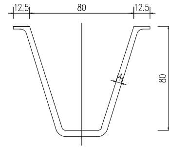
80渠道板断面尺寸 1:20
