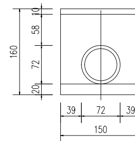
上、下游立面图 1:50
