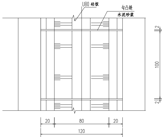
80 渠道平面图 1:20
