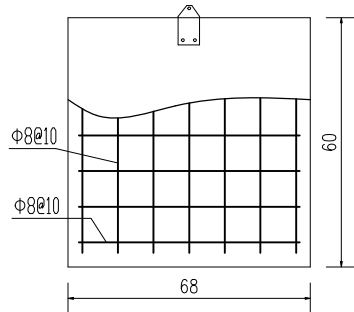
闸门构造 1:15 板厚5cm
