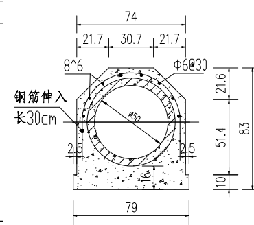
涵管断面图 1:25
