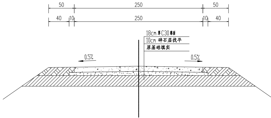
新建2.5m 宽水泥路断面（有路基）1:30
