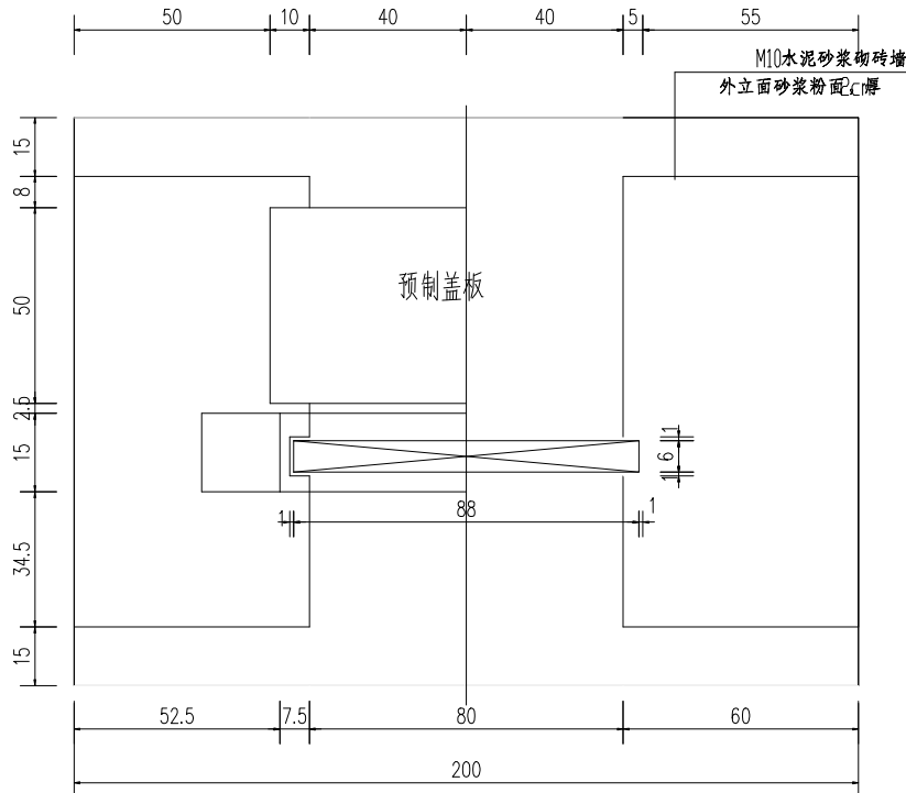
平面图 1:15
