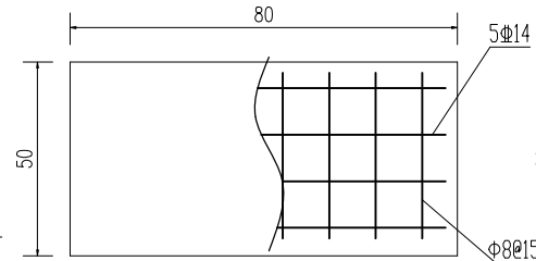
预制盖板尺寸 1:15 板厚10cm
