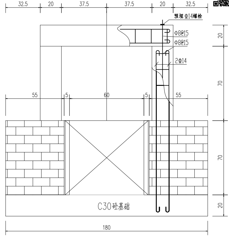
立面图 1:15
