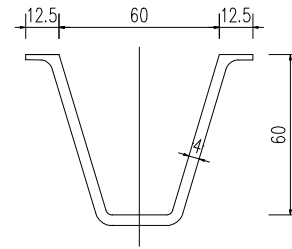
60渠道板断面尺寸 1:20
