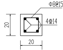
梁结构 1:15
