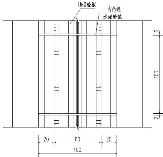
60渠道平面图 1:20
