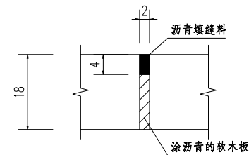
横向胀缝构造 1:30
