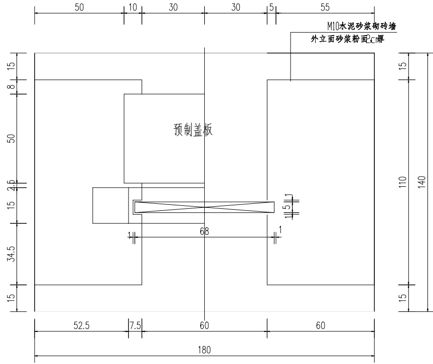
平面图 1:15
