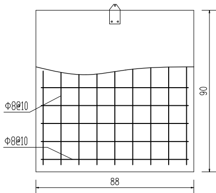
闸门构造 1:15 板厚6cm
