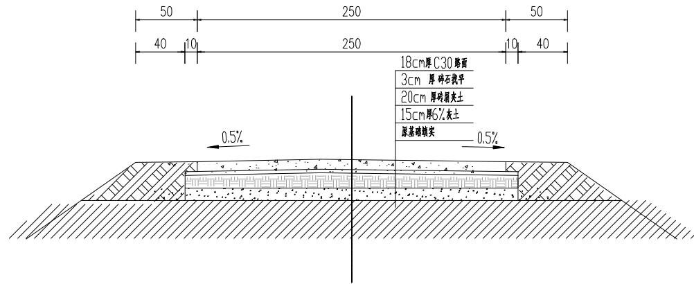
新建2.5m 宽水泥路断面（无路基）1:30
