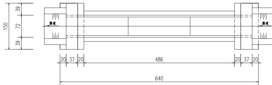
平面图 1:50
