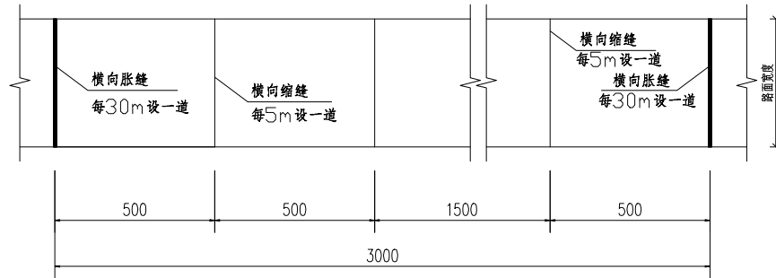
水泥路面横向胀缩缝设置 1:30
