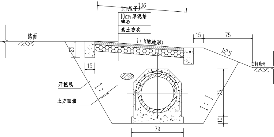
下田涵横断面图 1:25
