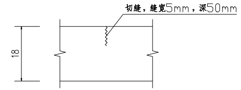
横向缩缝构造 1:30
