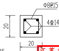
柱结构 1:15
