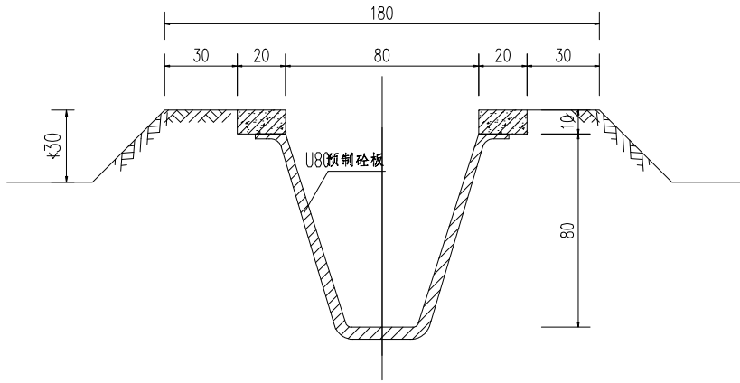
80渠道断面图 1:20
