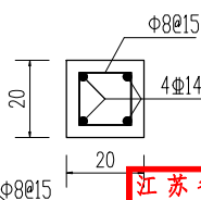
柱结构
