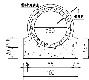
涵管接缝图 1:30
