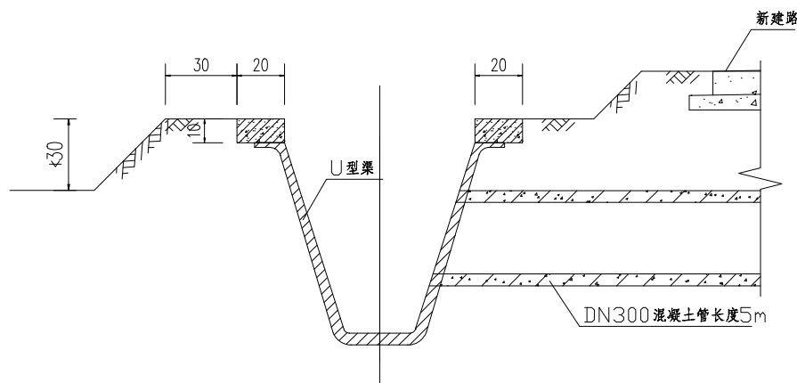
穿路放水管结构图
