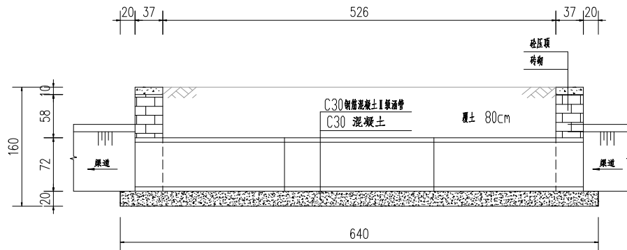
纵剖面图 1:50
