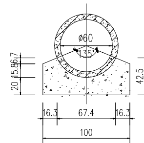
涵管断面 1:30
