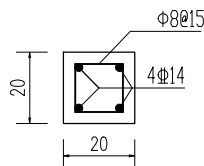
梁结构 1:15
