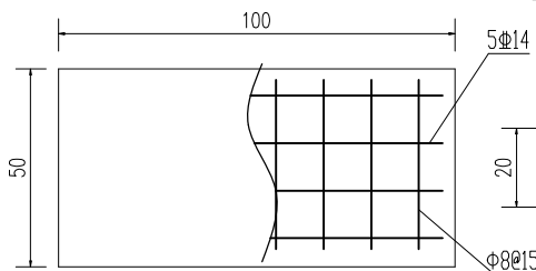
预制盖板尺寸 1:15 板厚10cm
