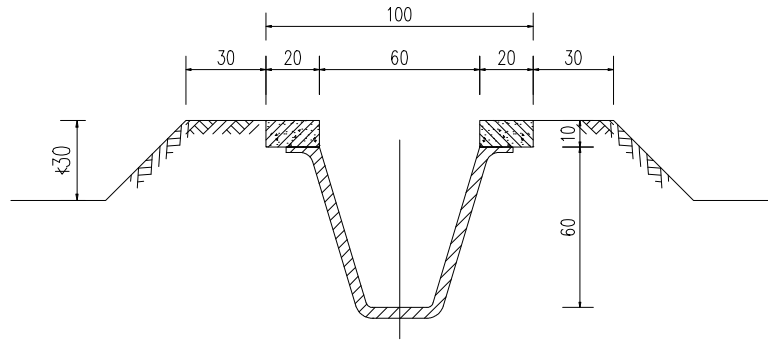
60渠道断面图 1:20
