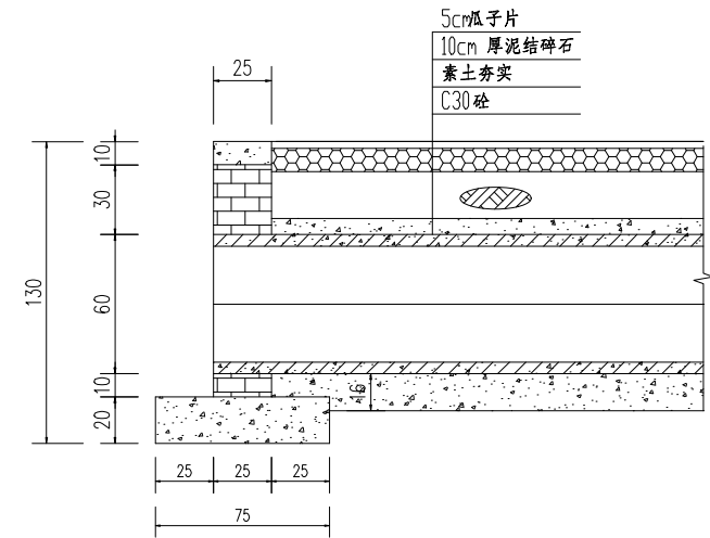
下田涵纵断面图 1:25
