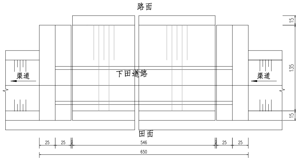
下田涵横断面图 1:25
