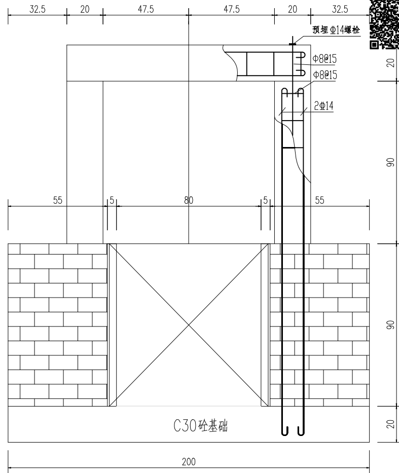
立面图 1:15
