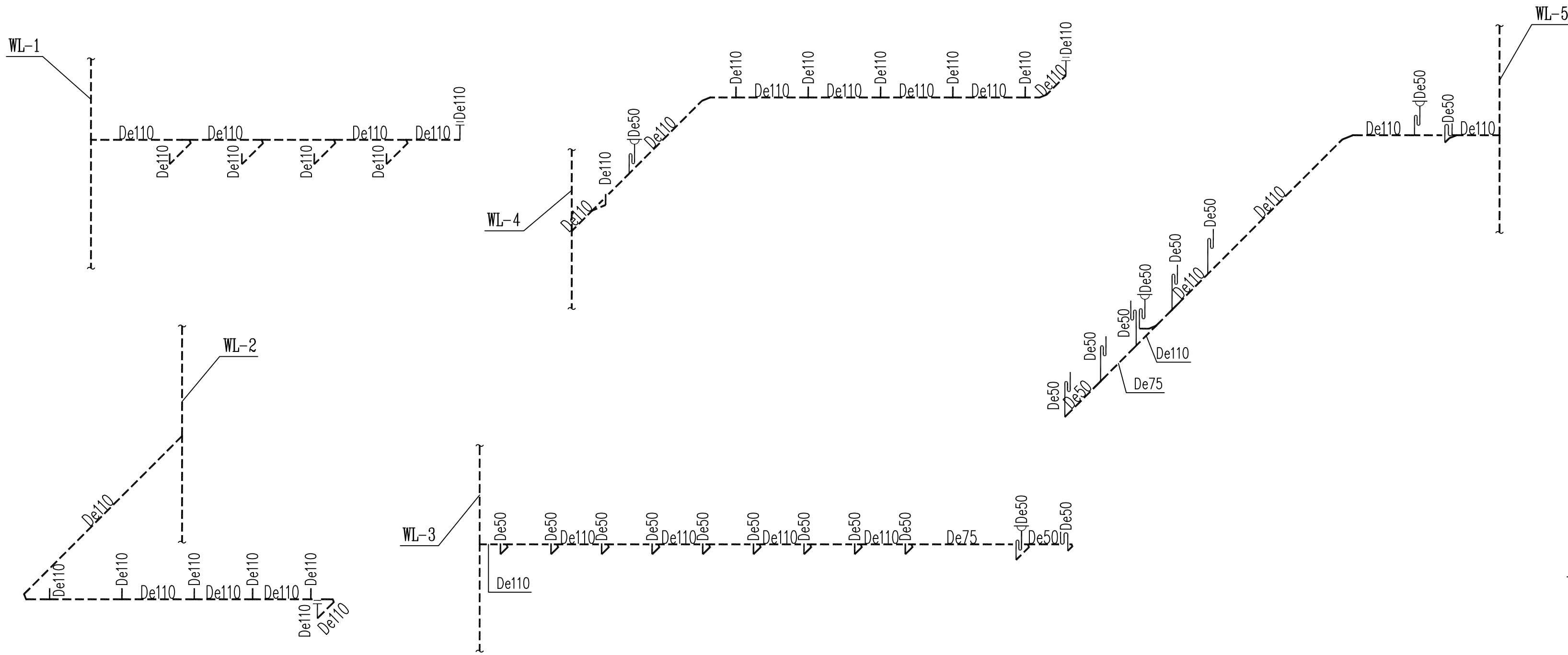
卫生间排水支管
