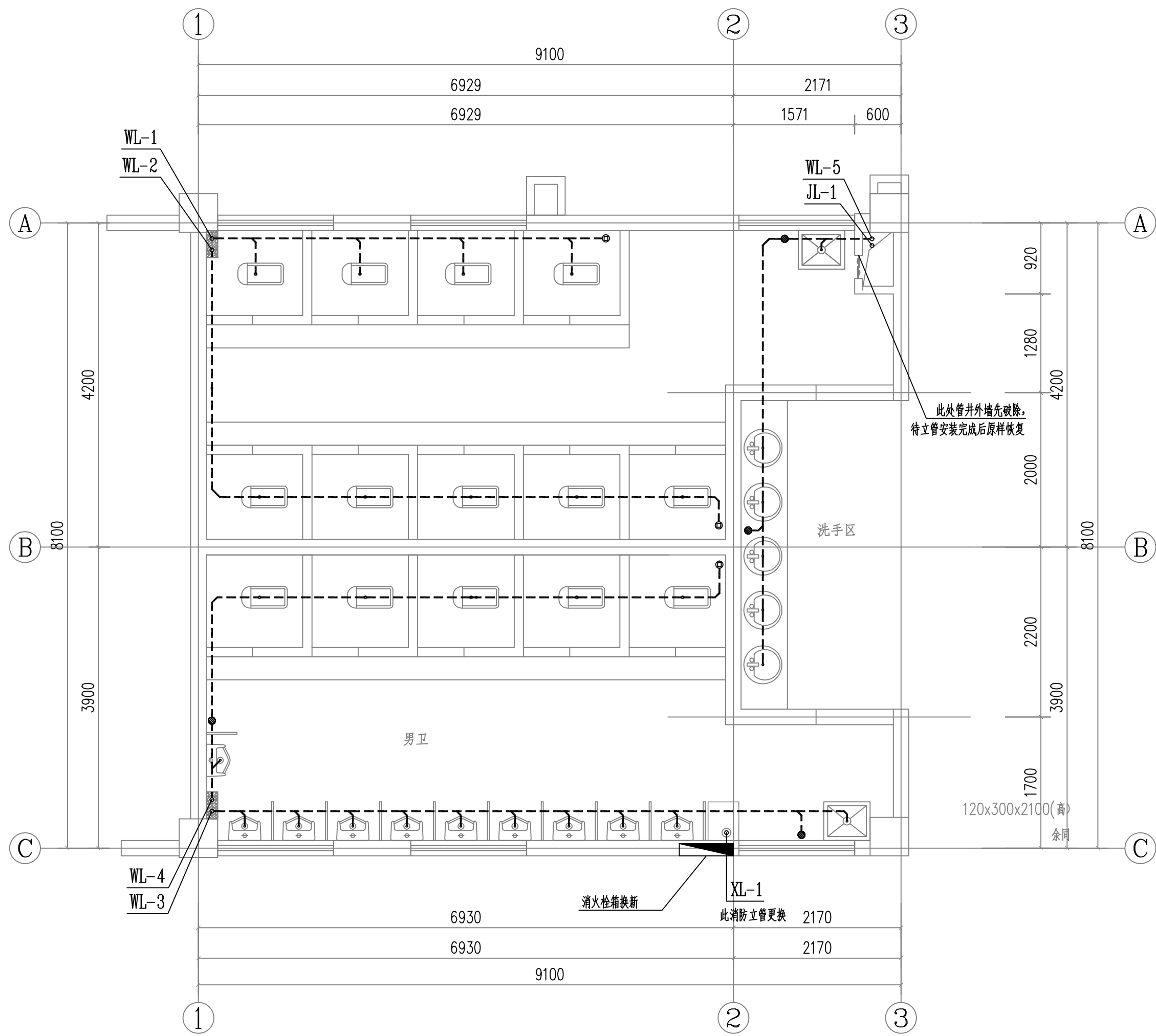
教学楼卫生间改造后排水平面图 1:50
