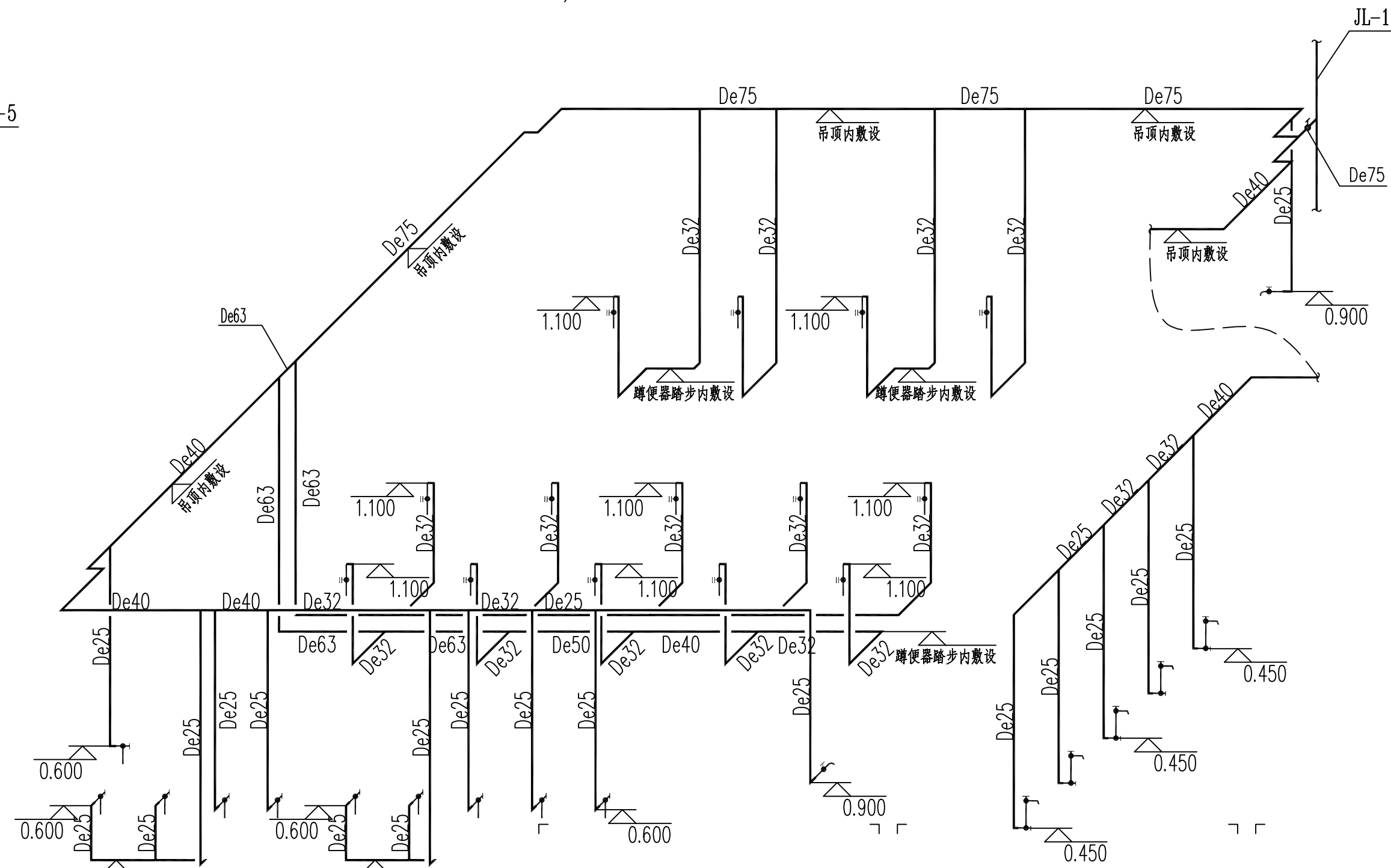
卫生间给水支管
