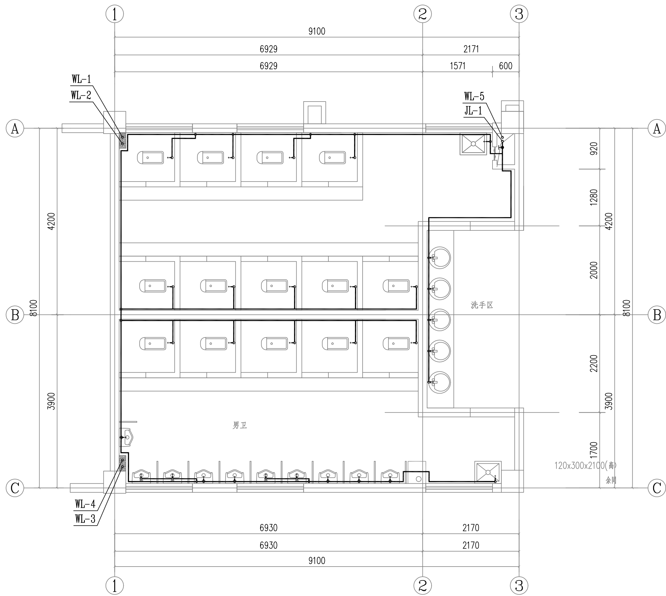
教学楼卫生间改造后给水平面图 1:50
