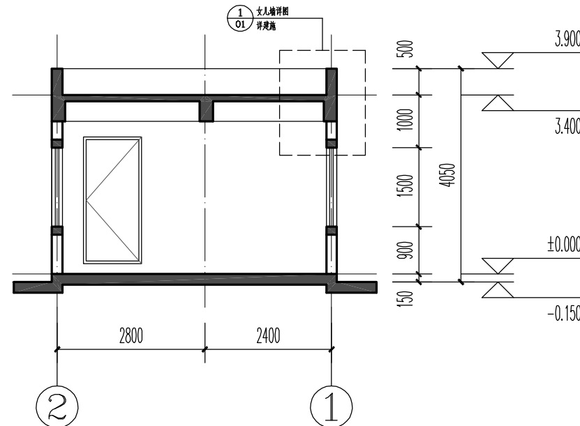
1-1剖面图 1:100
