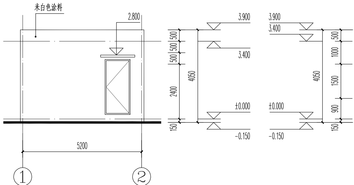
1~2轴立面图 1:100
