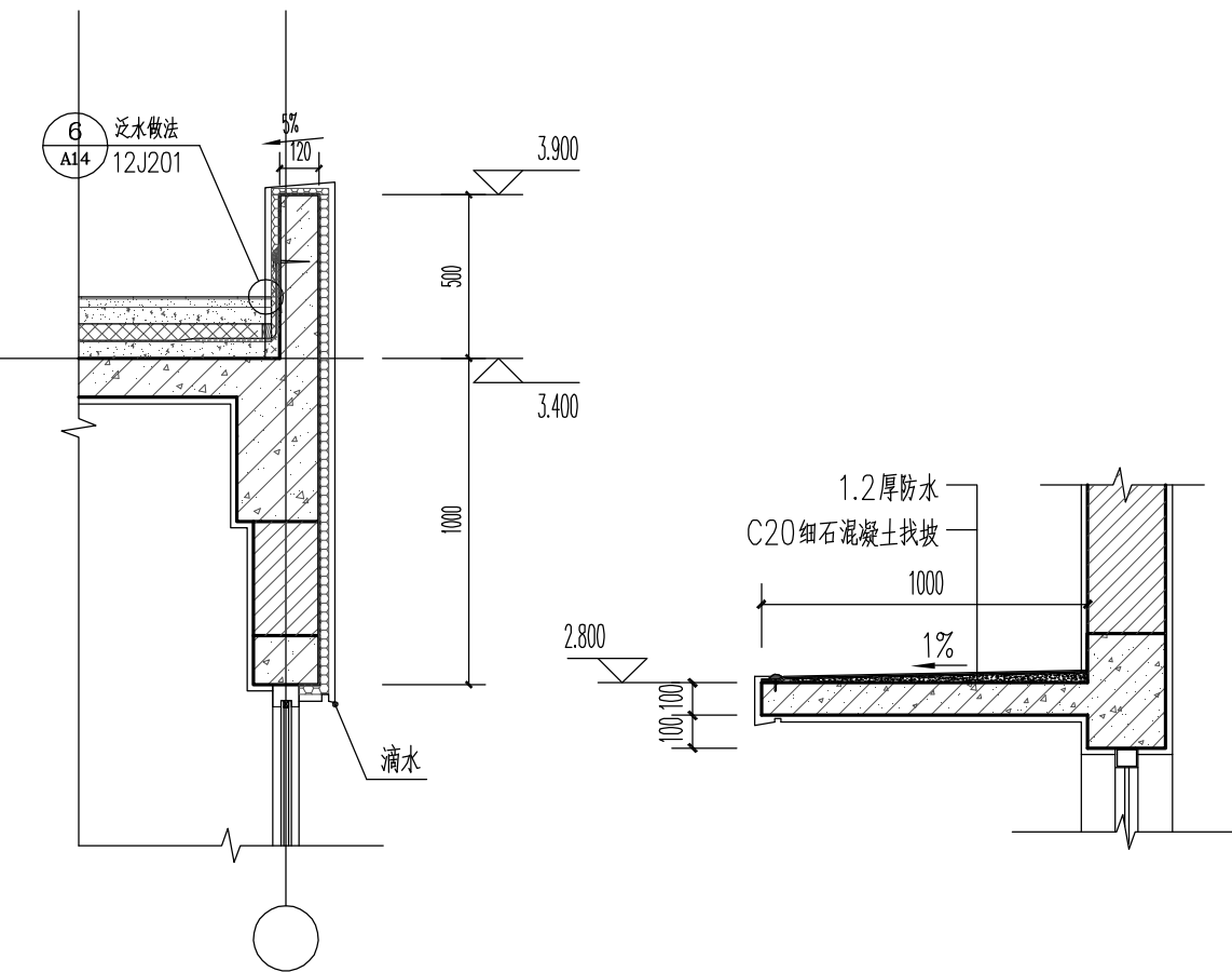
2 土建雨篷 1:25
