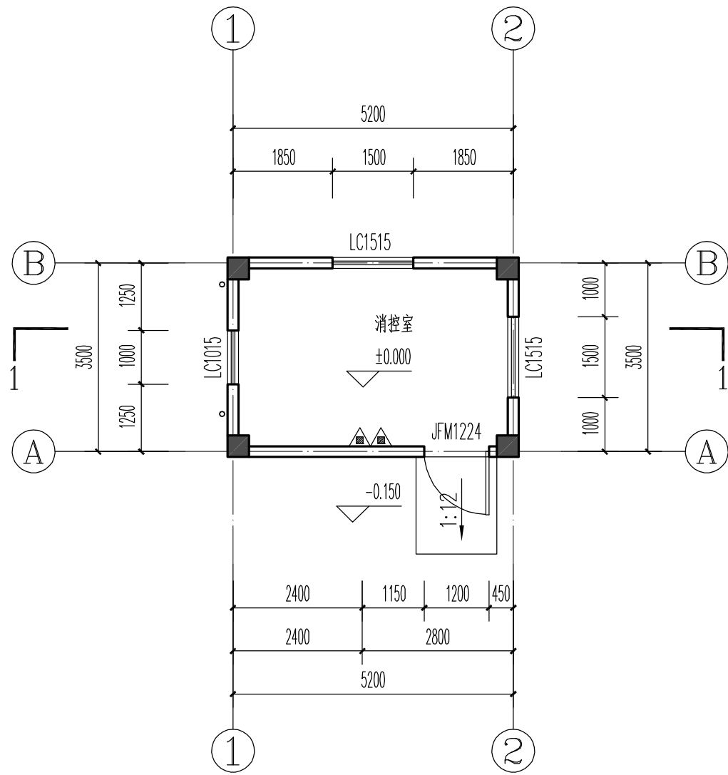
一层平面图 1:100
