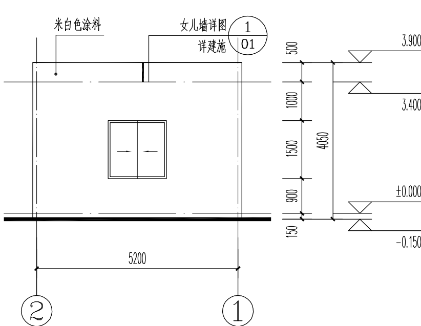
2~1轴立面图 1:100
