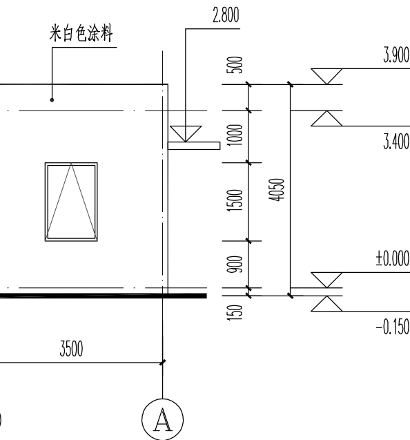
B~A轴立面图 1:100
