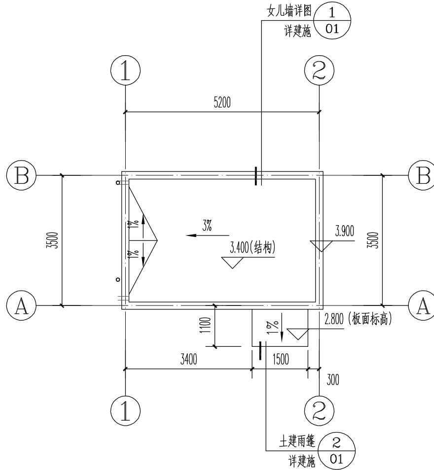
屋顶层平面图 1:100
