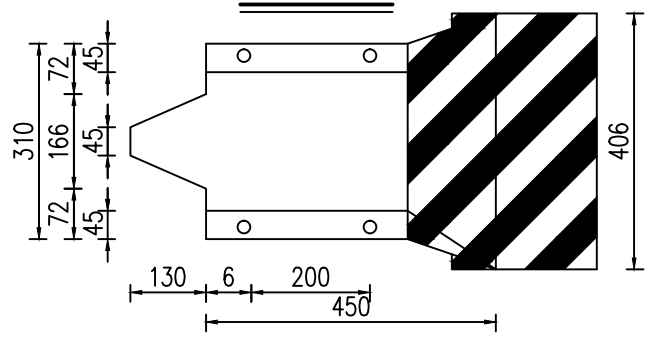
端头大样图
