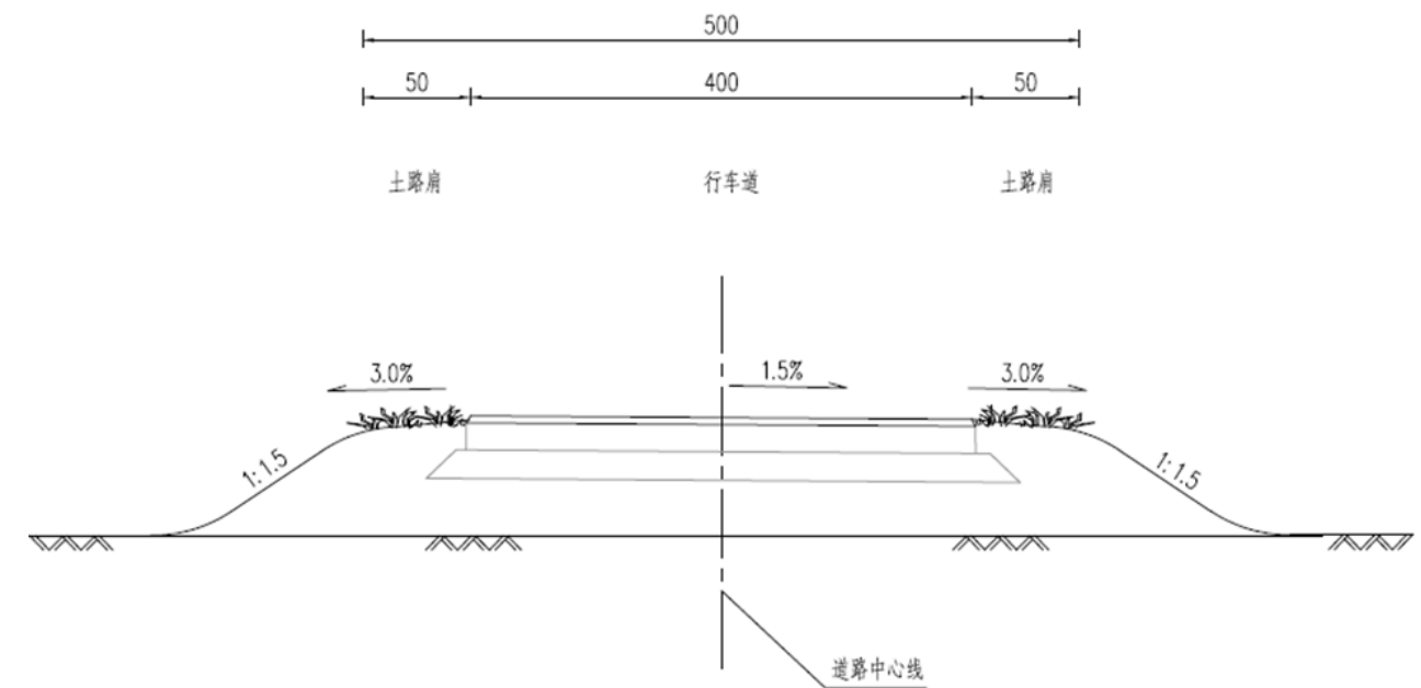
图 1 路基标准横断面图
