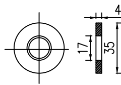
垫片
