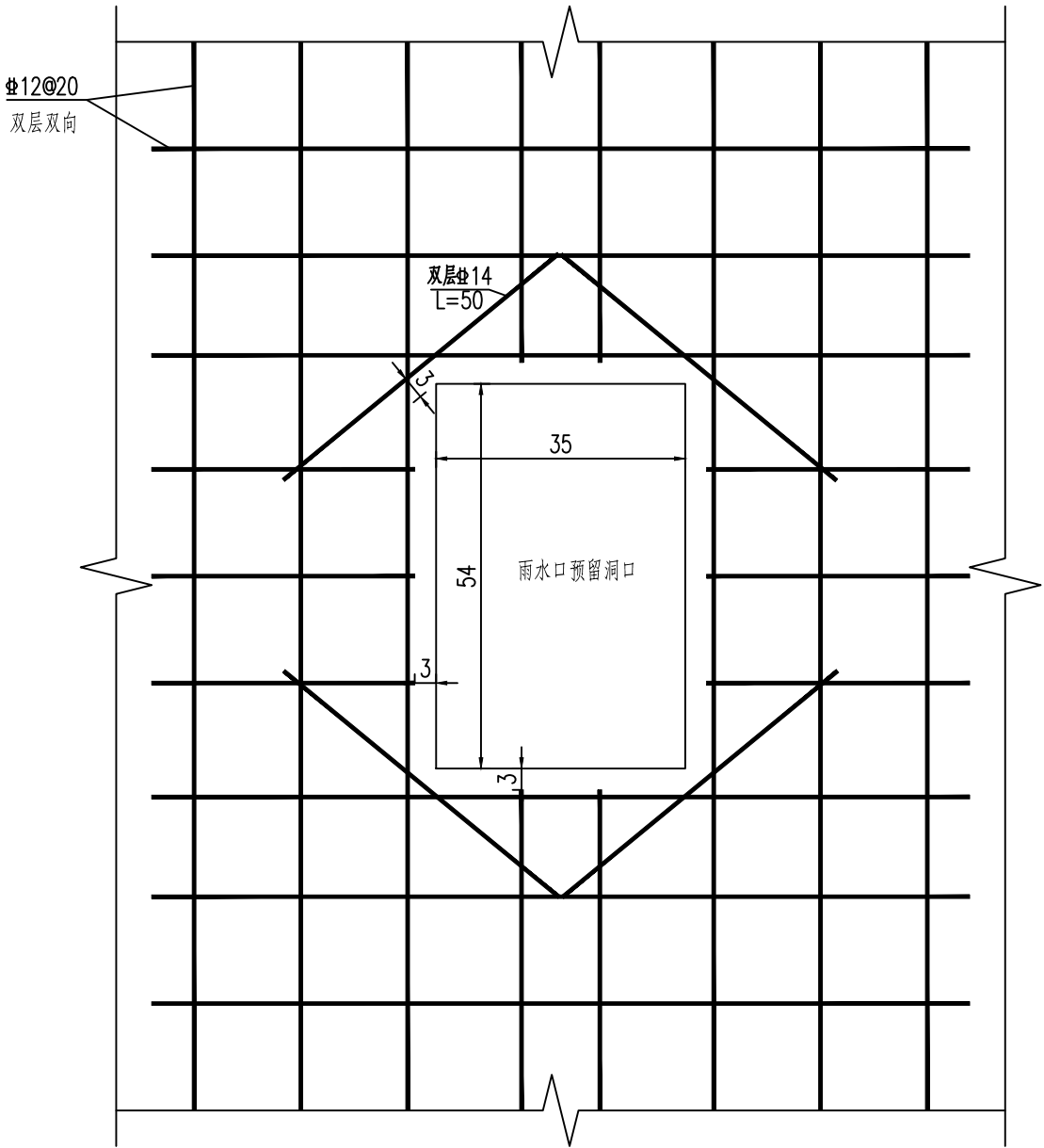
洞口加强筋大样图一
