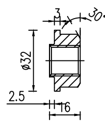
防盗螺母
