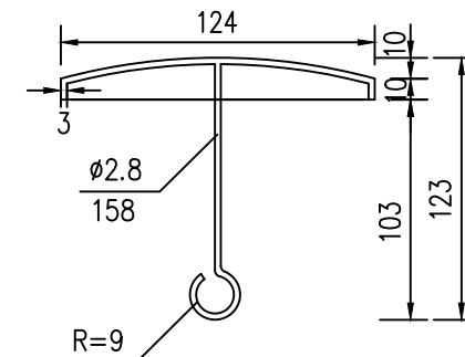
A大样
