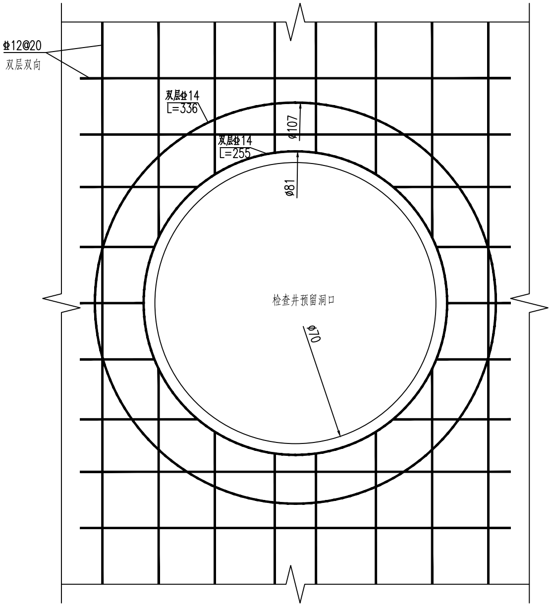
洞口加强筋大样图二
