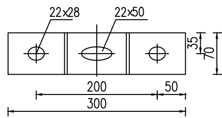
托架大样图
