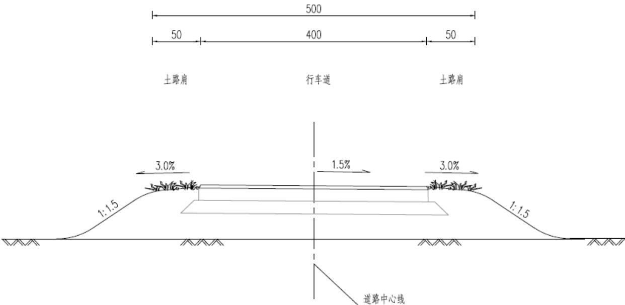
图 15 路基标准横断面图
