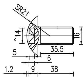
拼接螺栓
