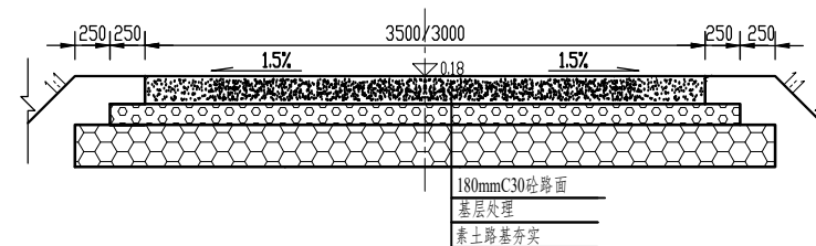
砵道路标准断面图
