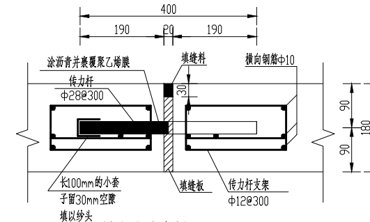
六 横向胀缝大样图 1:10
