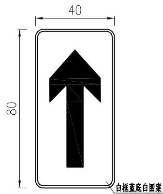
单行道标志 1:20
