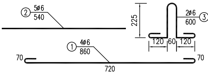
井盖钢筋大样 1:10
