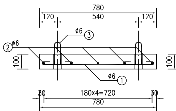
井盖钢筋侧面 1:15
