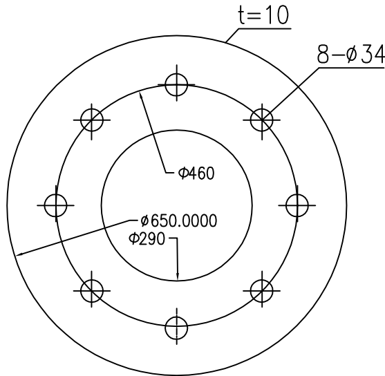
螺栓大样图
