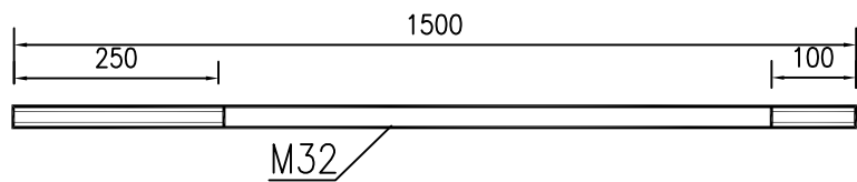
螺栓大样图
