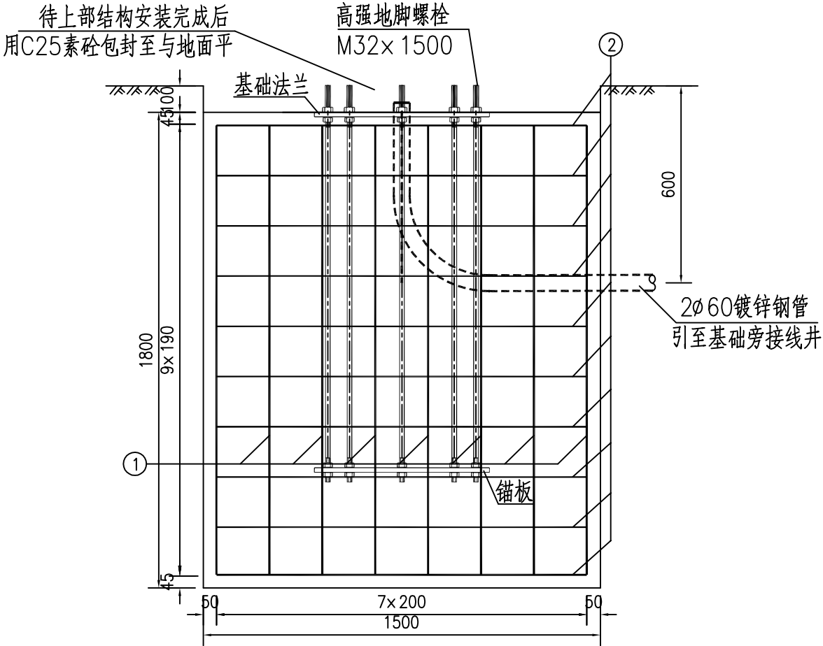
侧面图
