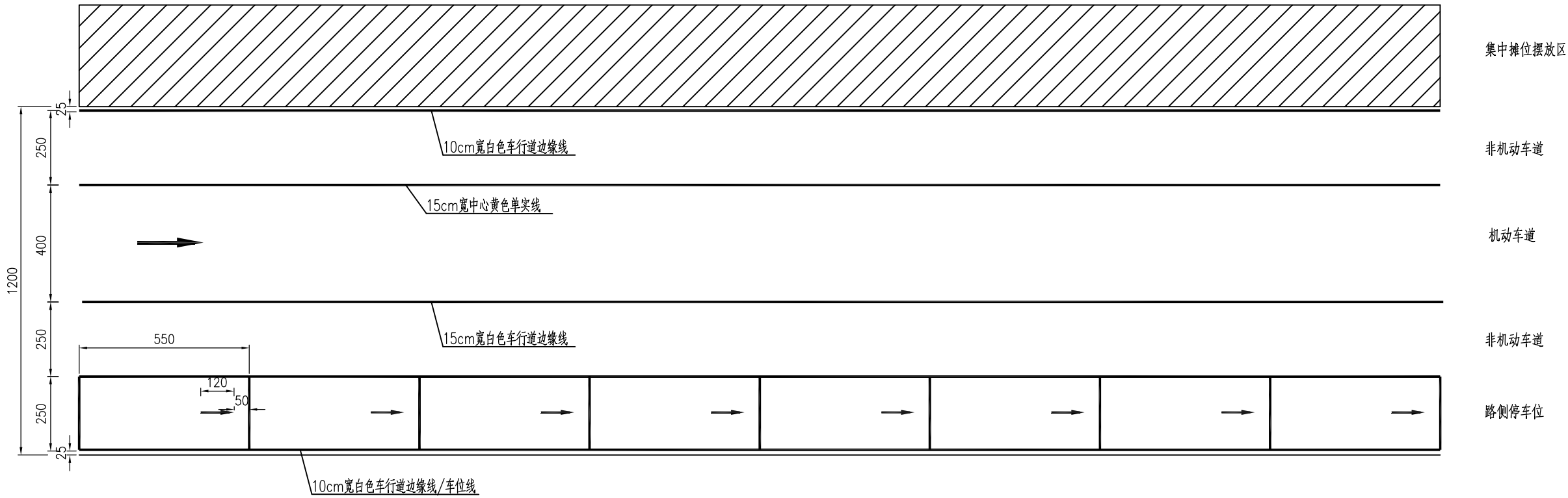
标线一般布置图
