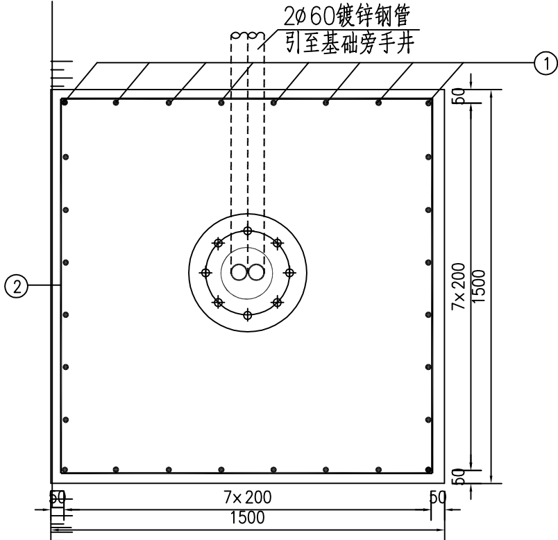
平面图
