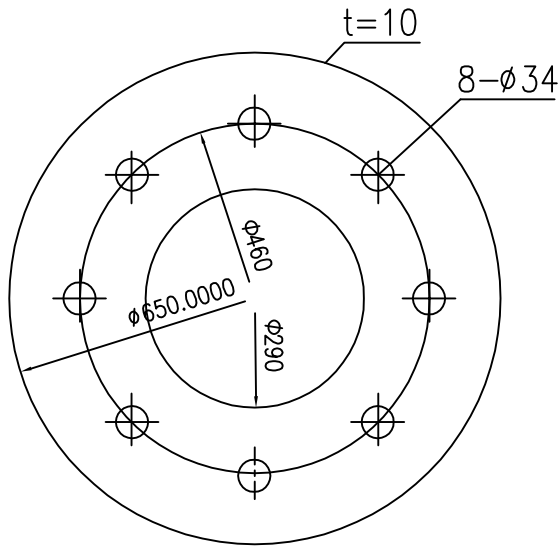
螺栓大样图
