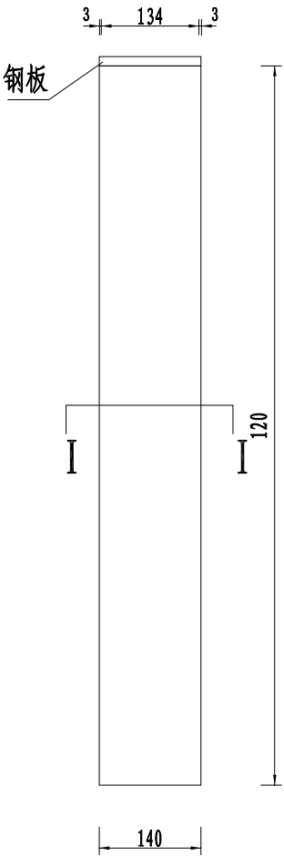
警示桩
