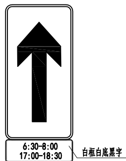
限时单行道标志 1:20
