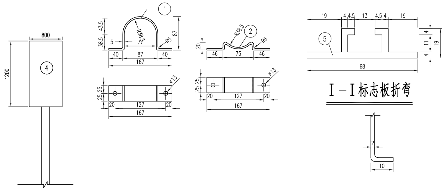
抱箍截面
