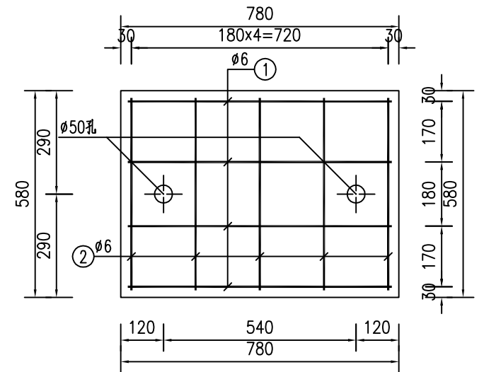
井盖钢筋平面 1:15
