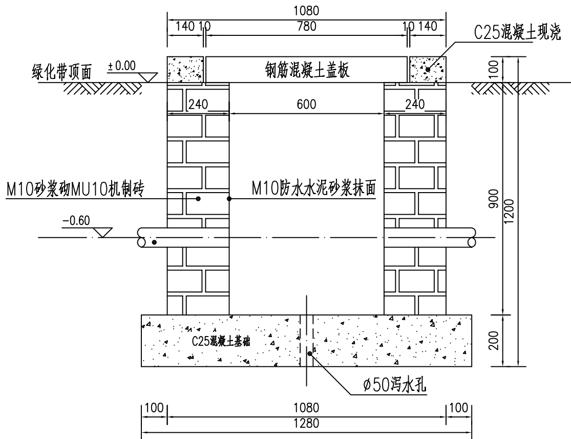
手井立面 1:15
