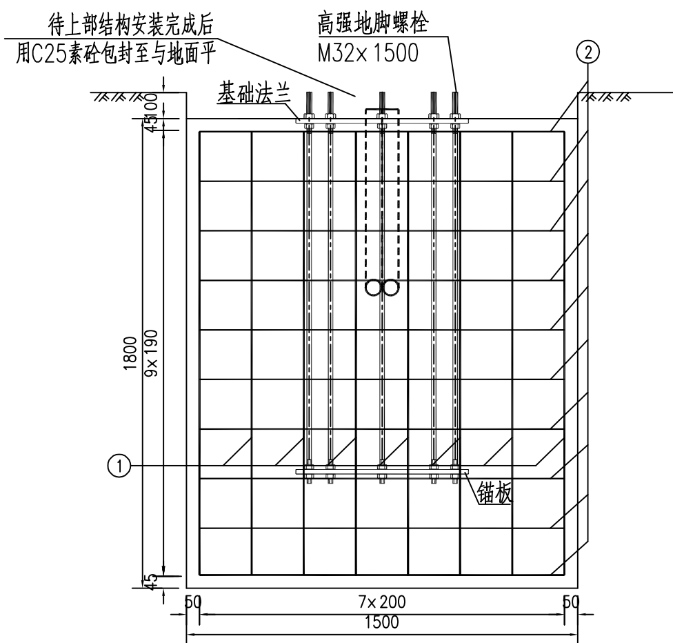
立面图
