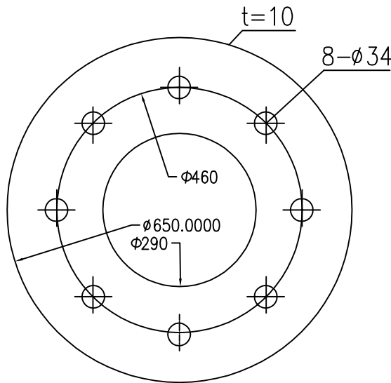
螺栓大样图
