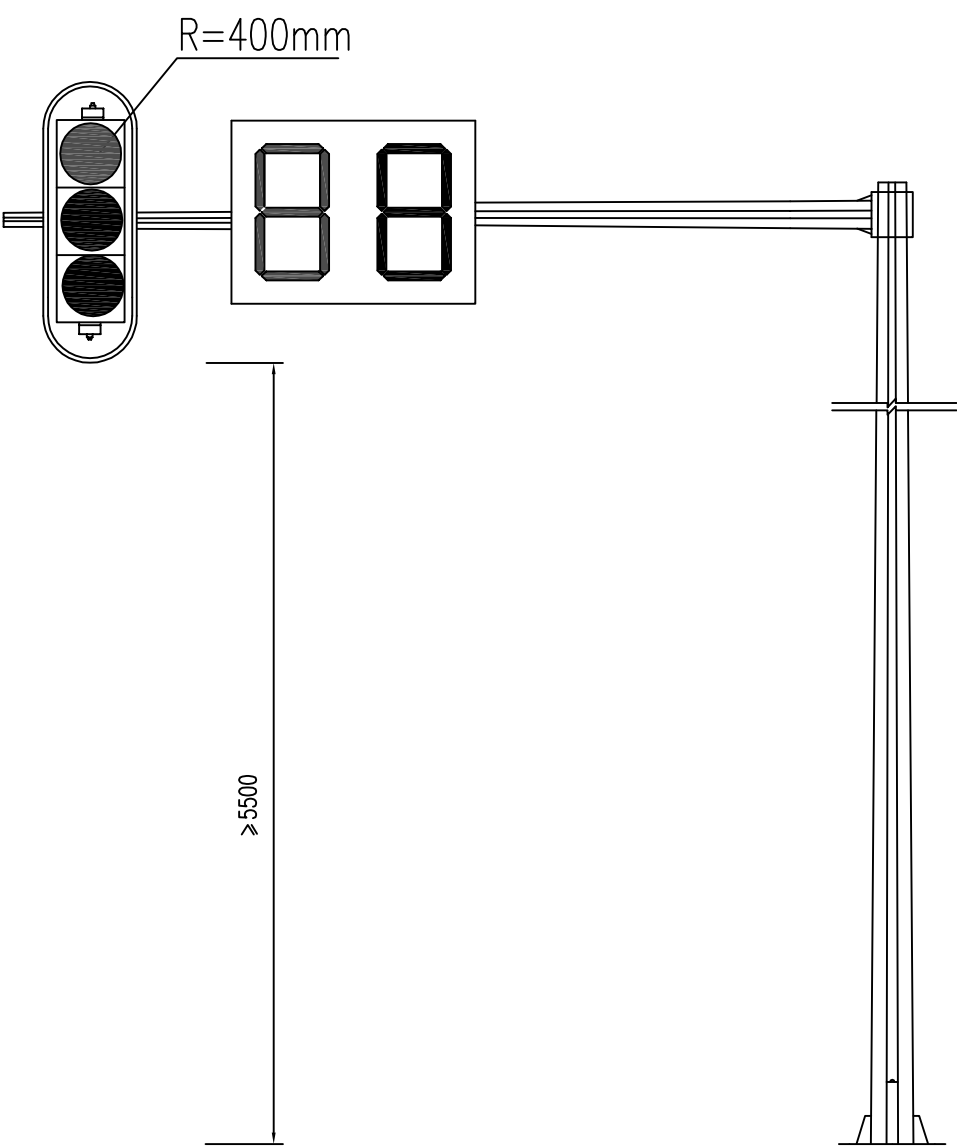
机动车道信号灯灯盘设置示意图（直行）
