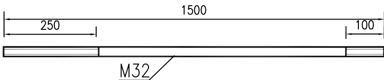
螺栓大样图
