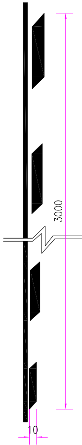
车行道纵向减速标线渐变段 (cm)
