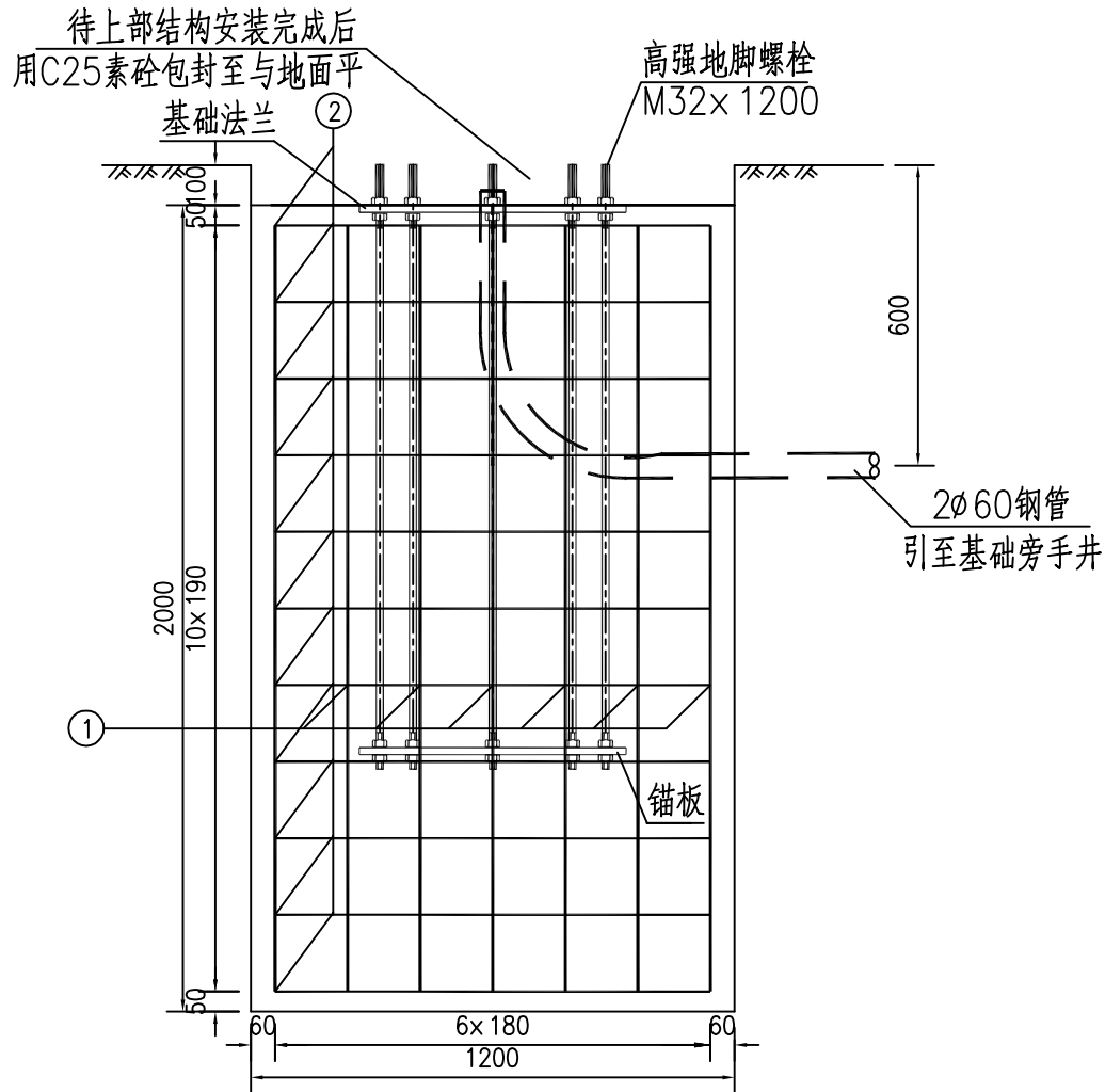
侧面图
