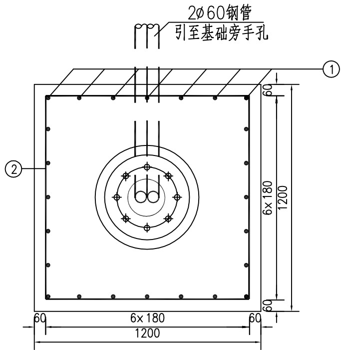
平面图
