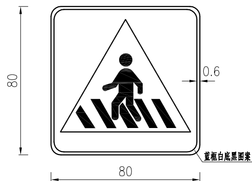
人行横道标志 1:20
