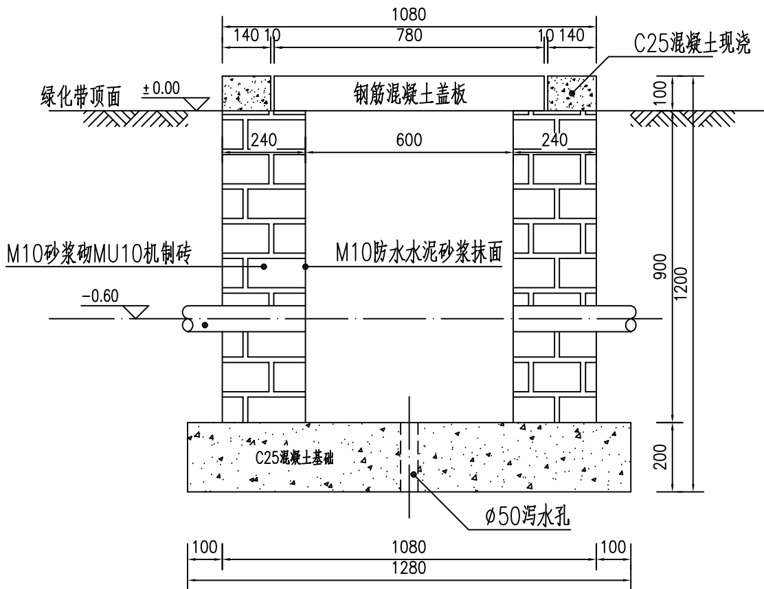
手井立面 1:15
