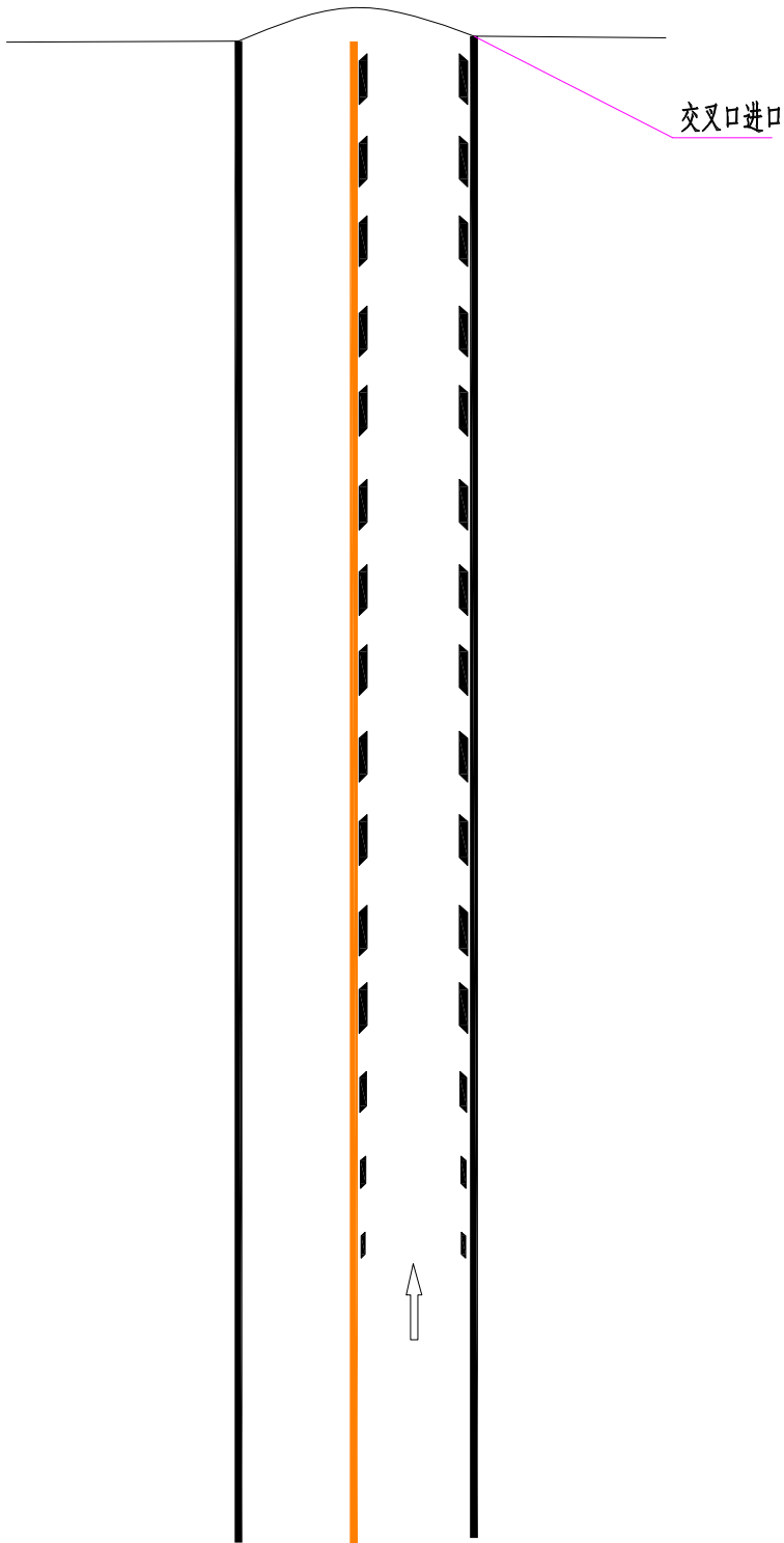
车行道纵向减速标线设置示例 (cm)
