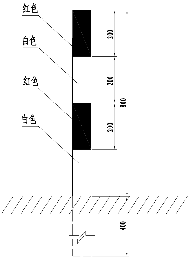
警示桩
