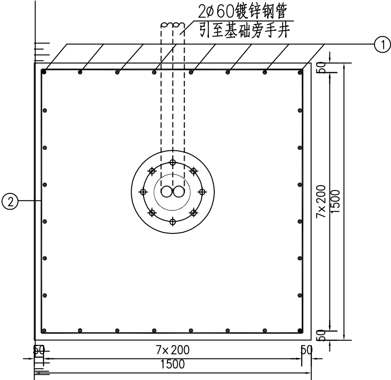
平面图
