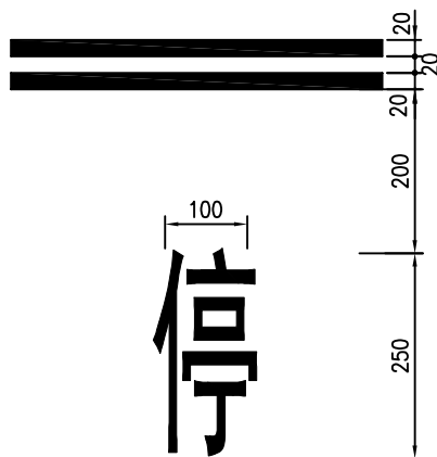
停车让行线大样图 比例 1:100
