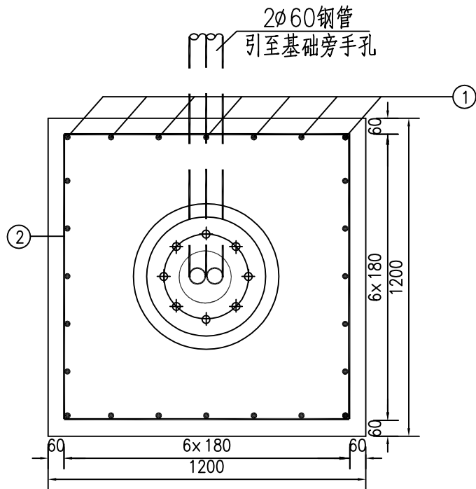
平面图
