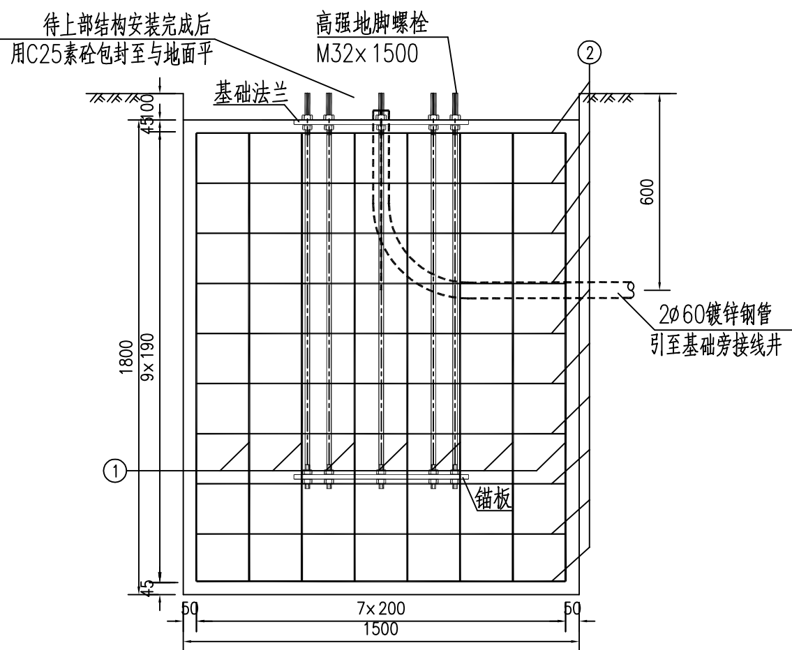
侧面图
