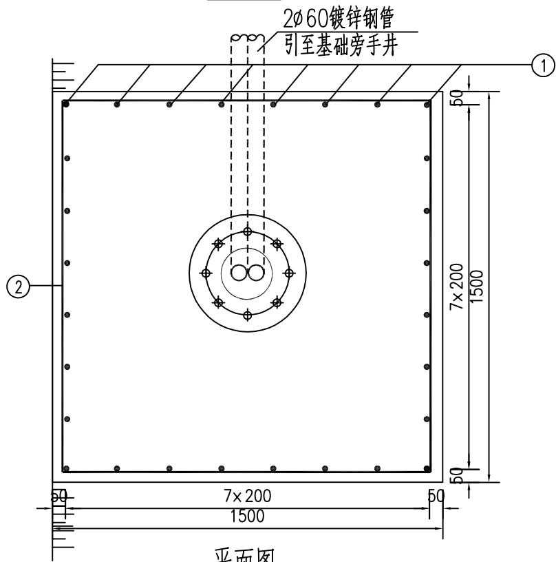
平面图
