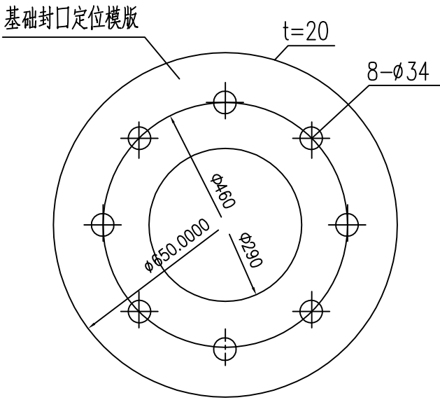
底座法兰盘平面图
