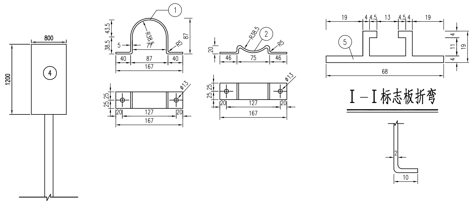
抱箍截面
