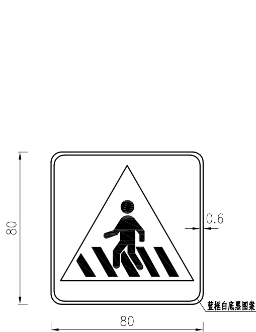
人行横道标志 1:20
