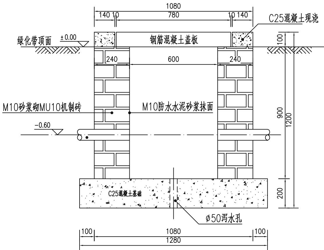
手井立面 1:15
