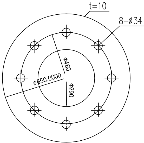
锚板大样图
