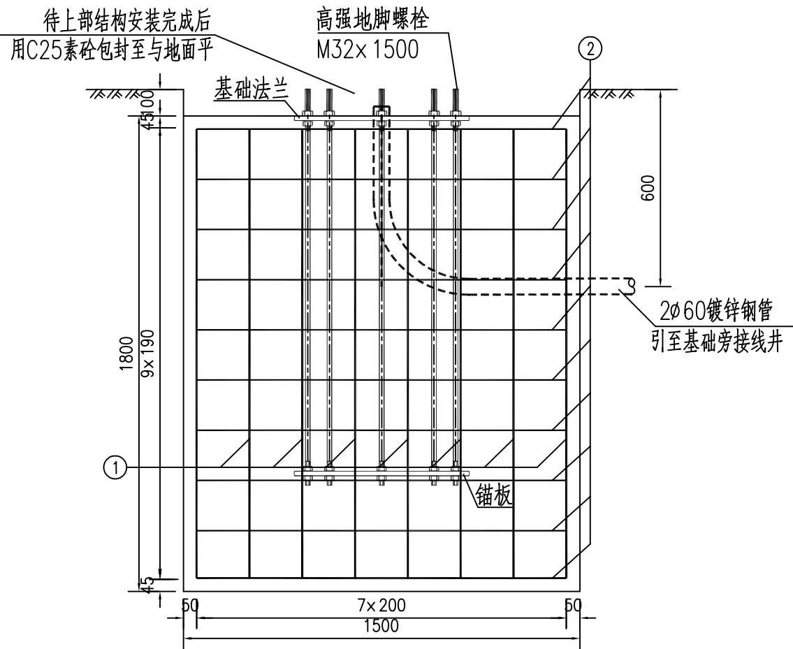
侧面图
