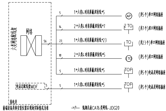
手术部综合布线系统图
