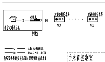
手术部医护对讲系统图
