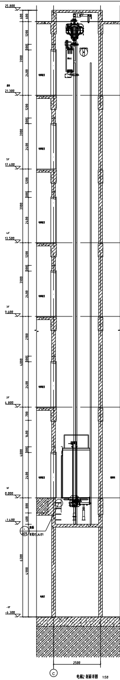
电梯2 剖面详图 150
