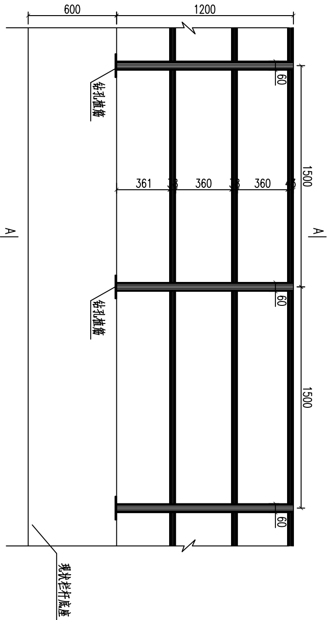
栏杆大样图 1:50
