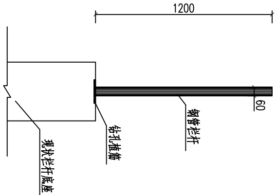
A-A 1:50
