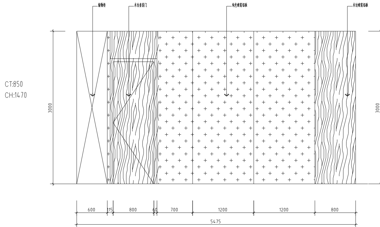
一层、二层招待室立面图
