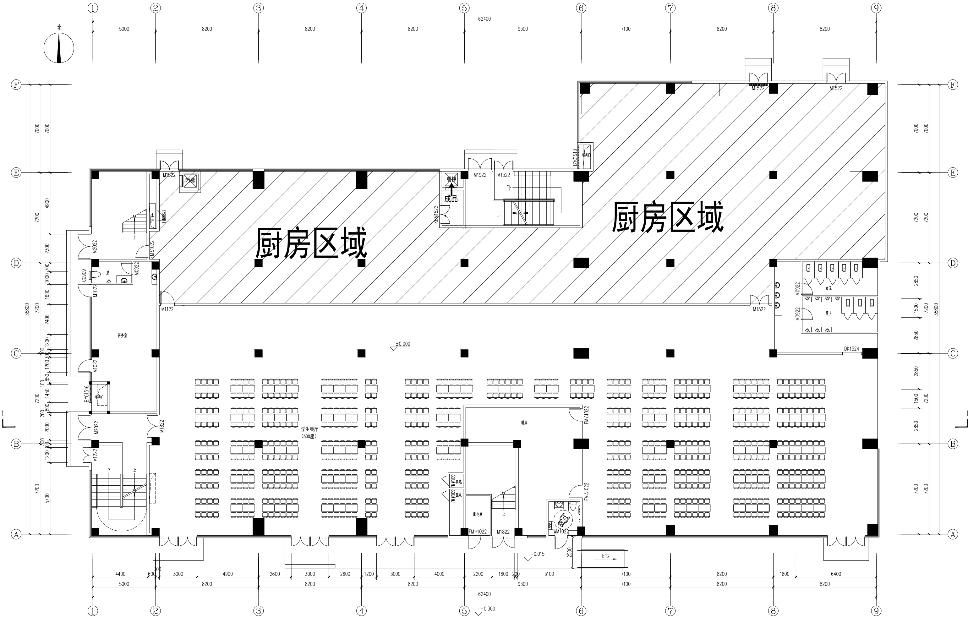
一层平面图 1:100
