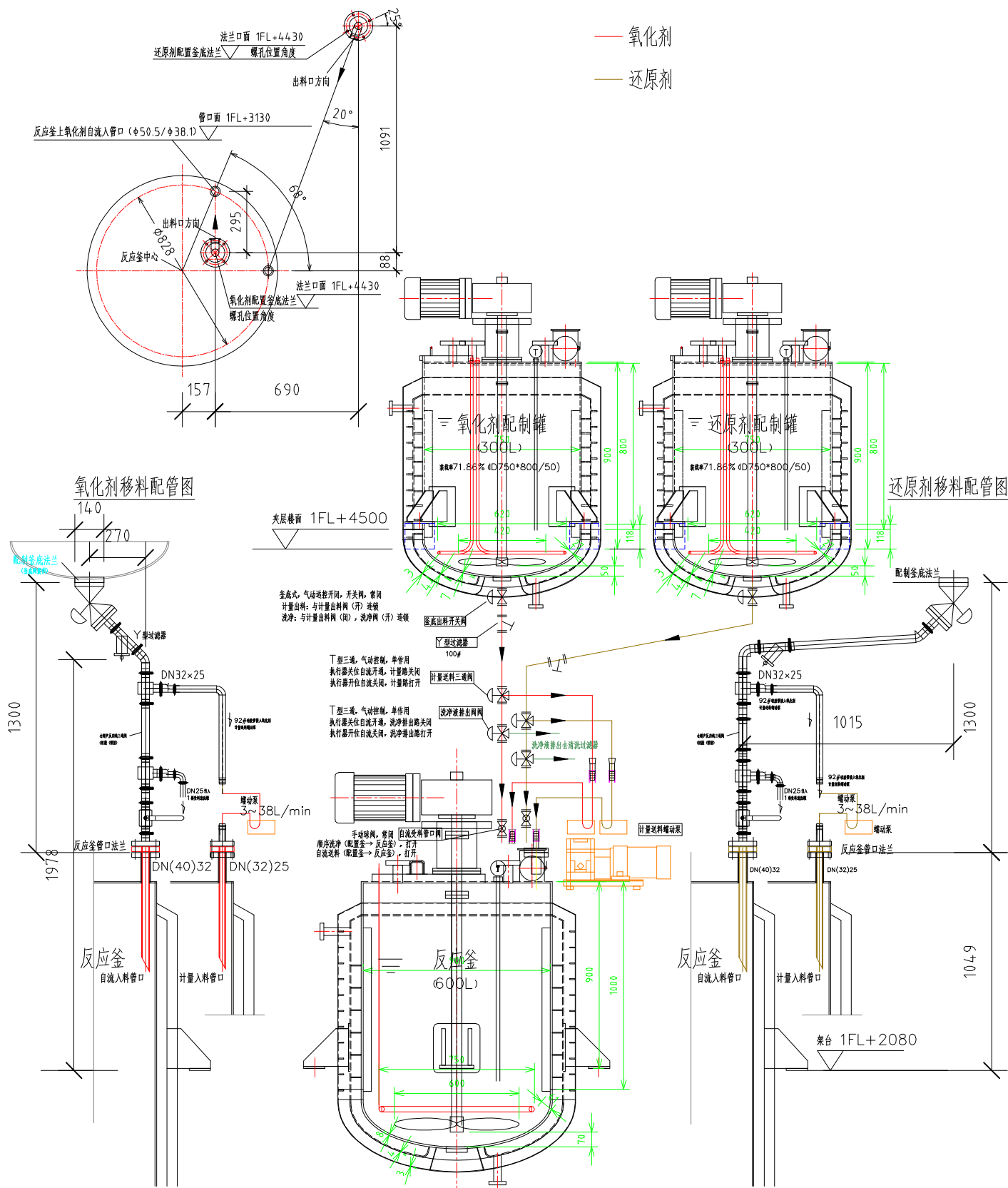
附件1 3：配制釜~反应釜 物料移送操控工艺示意图
