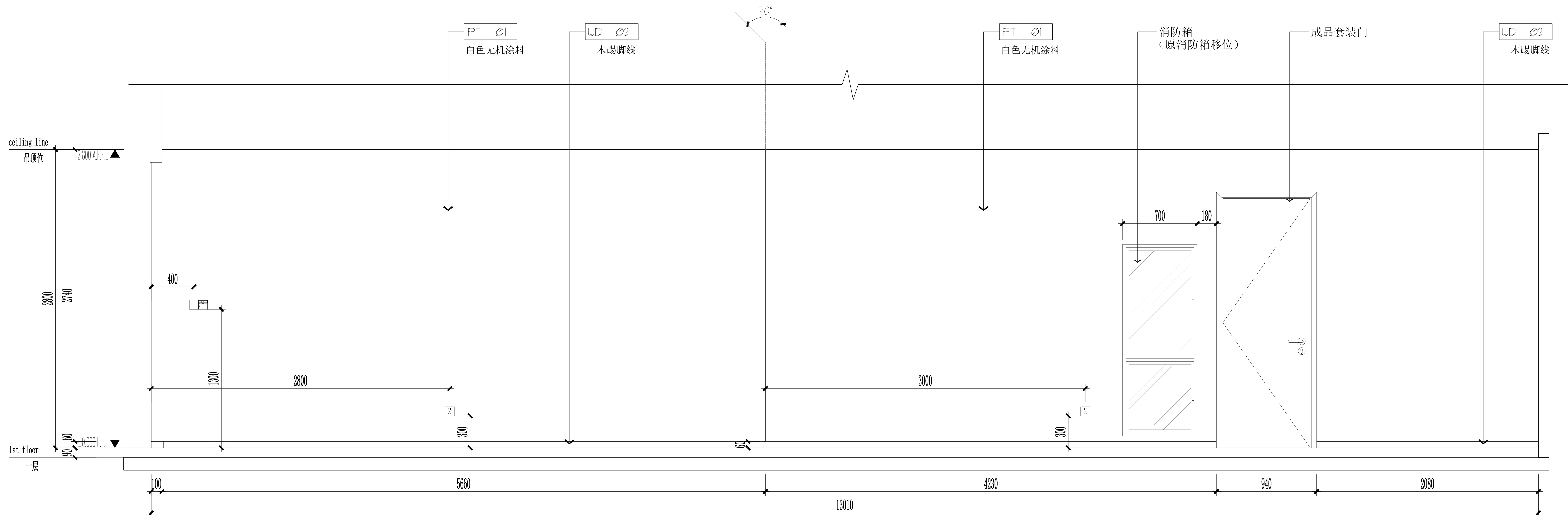
09 ELEVATION 3Q-P-12 接待区过道立面图 SCALE 1:30
