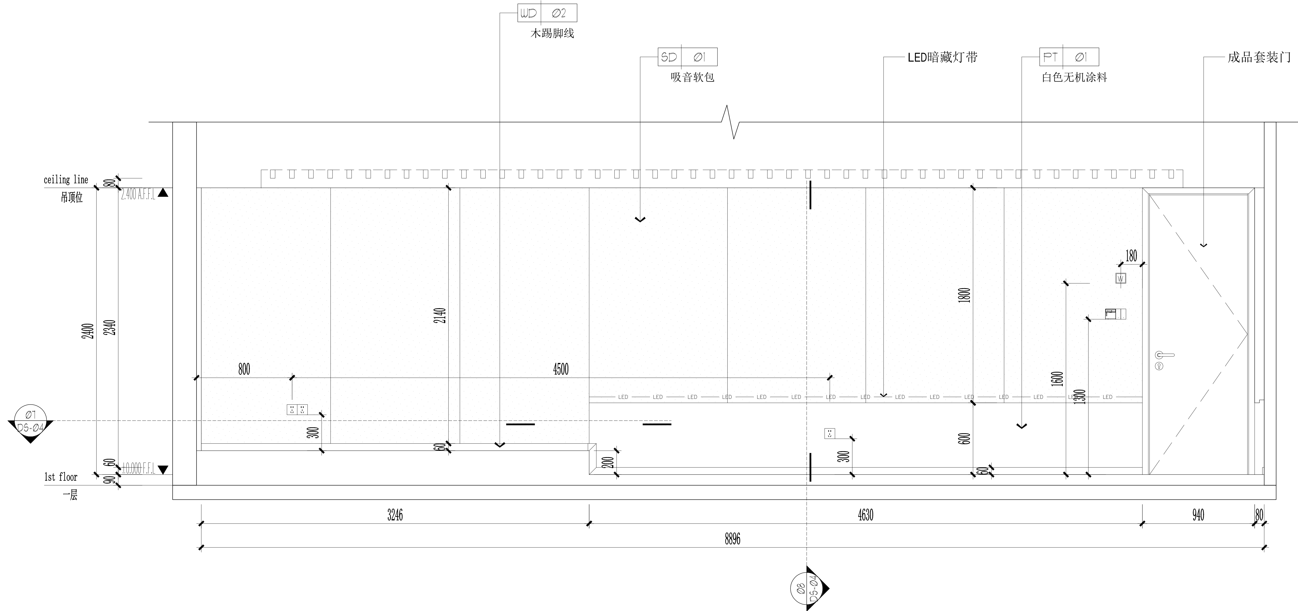
05 3Q-P-12 ELEVATION 多功能教室立面图 SCALE 1:30
