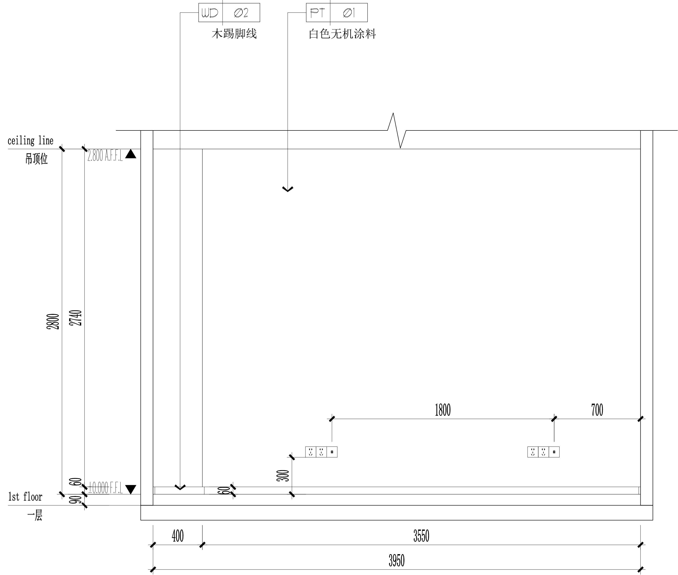
15 3Q-P-12 办公室立面图 SCALE 1:30
