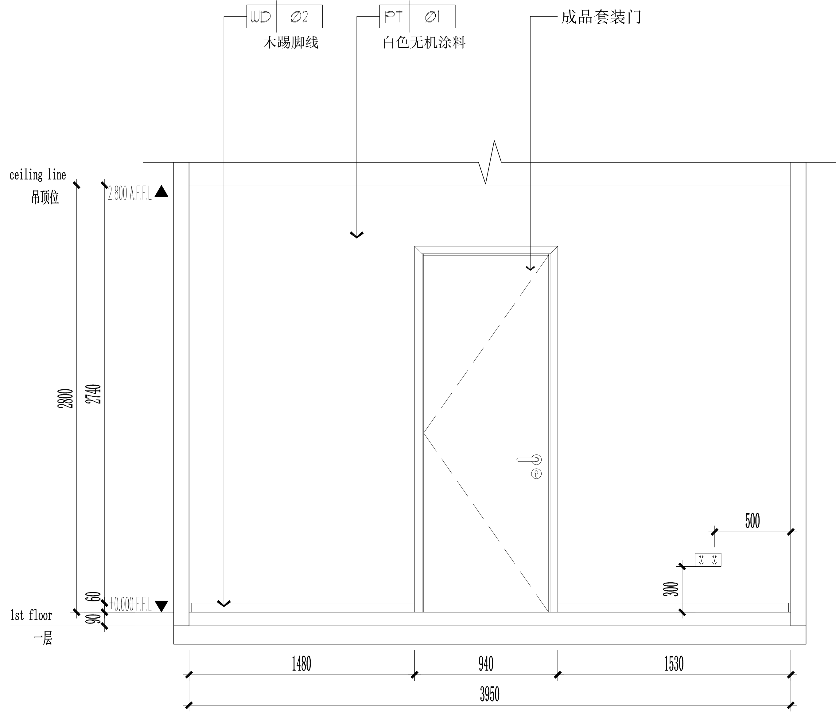
13 3Q-P-12 办公室立面图 SCALE 1:30
