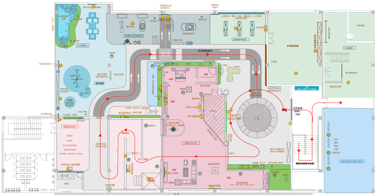
本项目整体平面图
