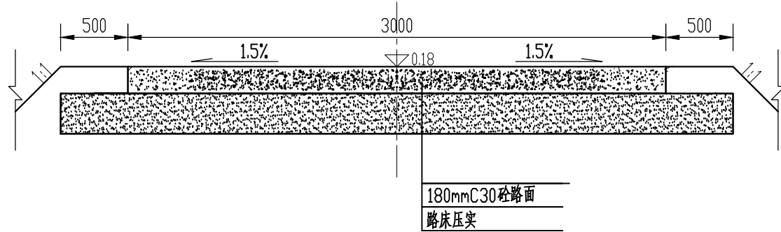
砼道路标准断面图
