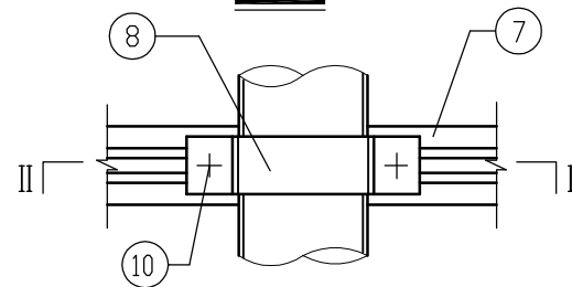
A大样
