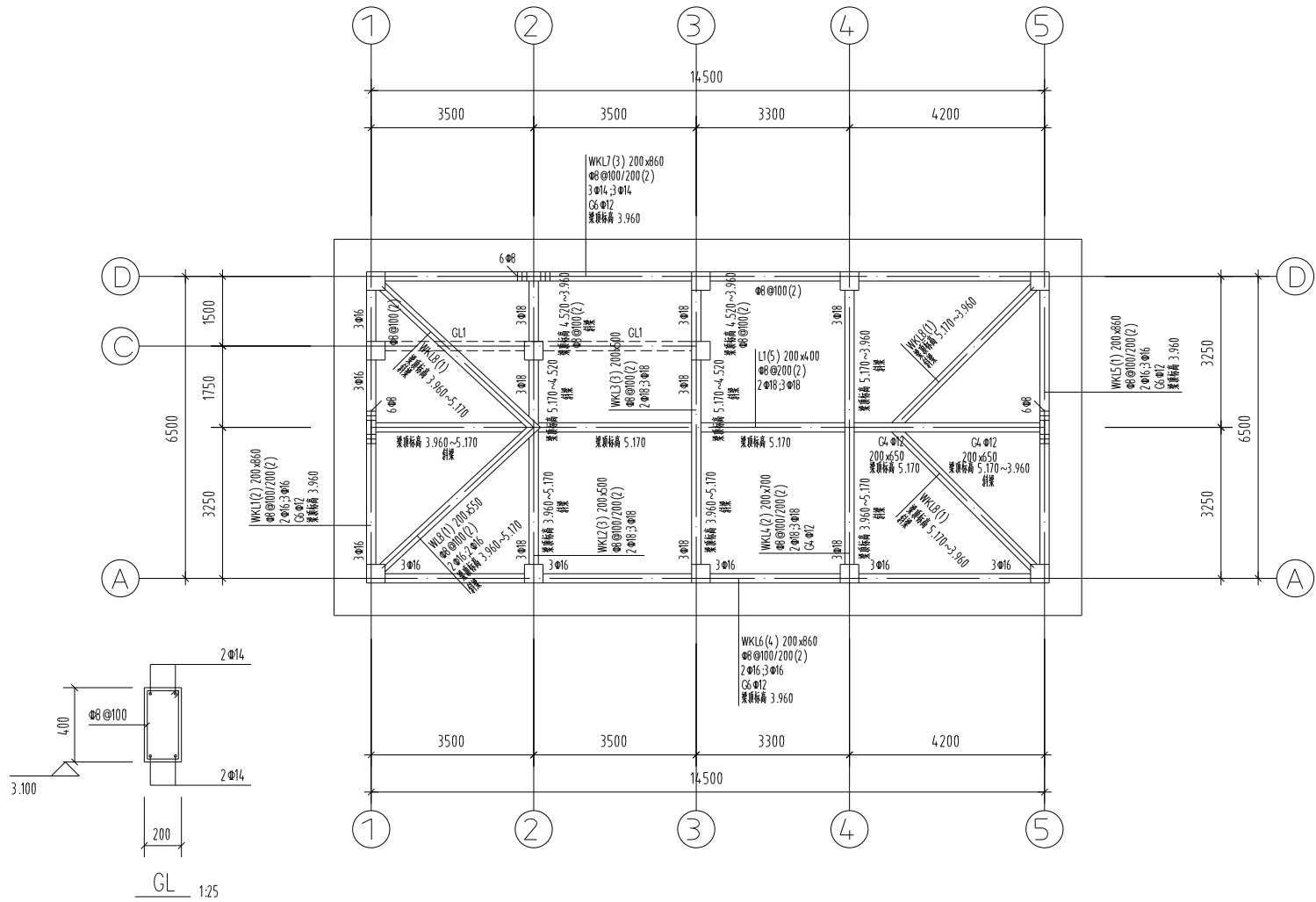
一层屋面框架梁结构布置图
