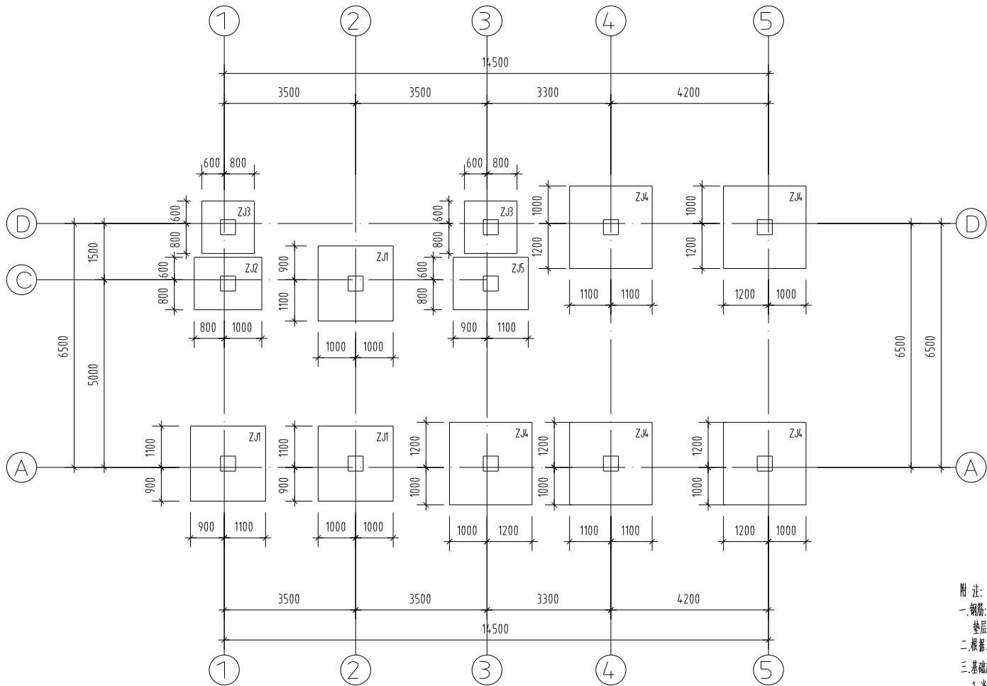
基础平面图 1:100
