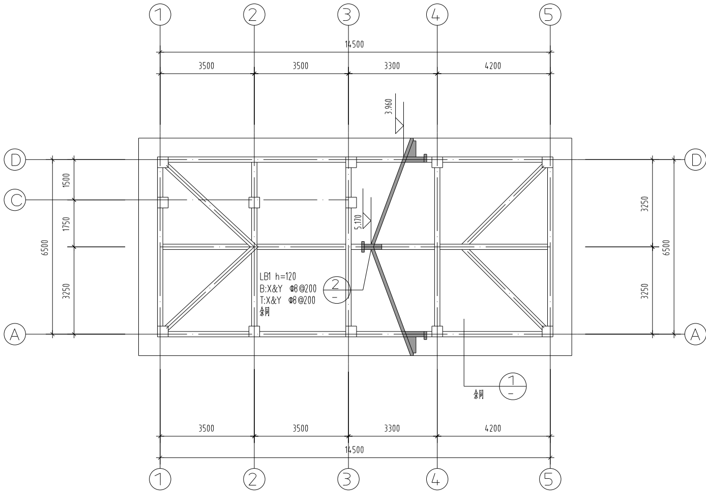
一层屋面现浇板结构布置图
