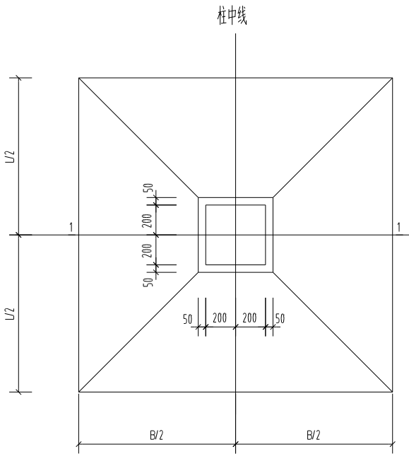
ZJ1~ZJ5 基础平面 1:25
