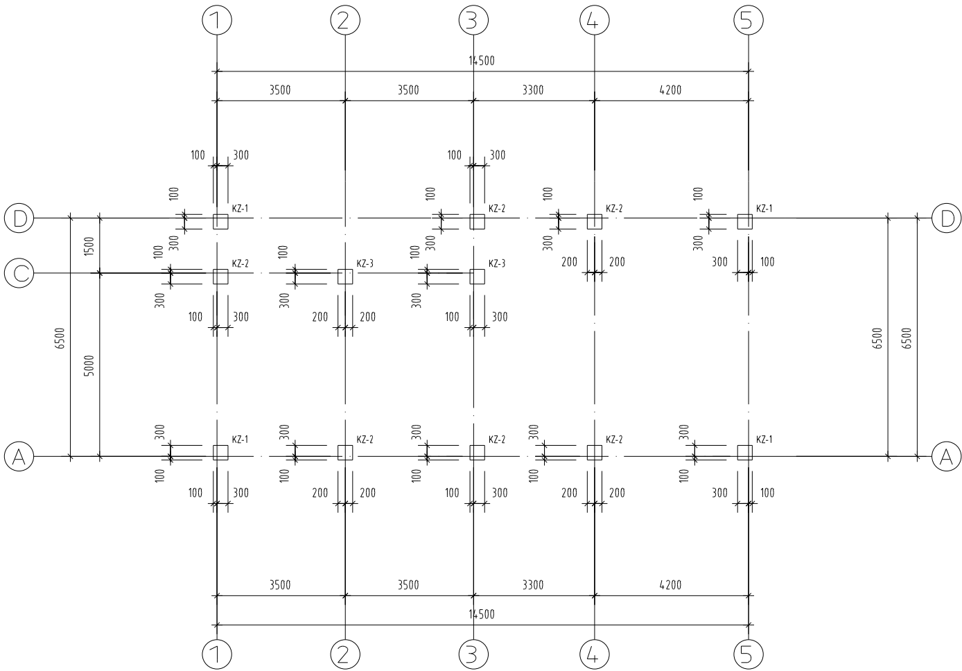
框架柱结构布置图
