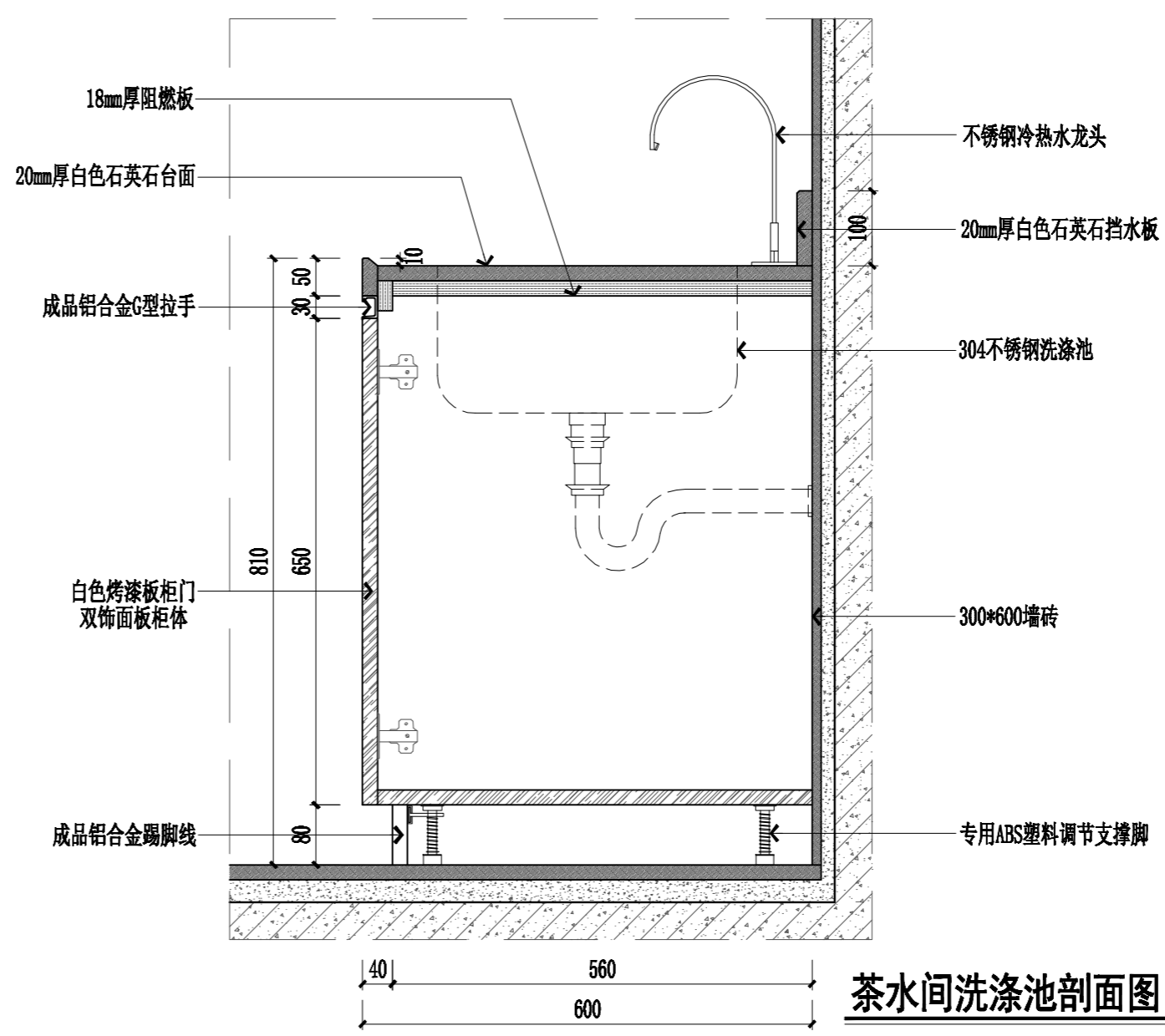
行政楼洗手槽剖面图 1:8
