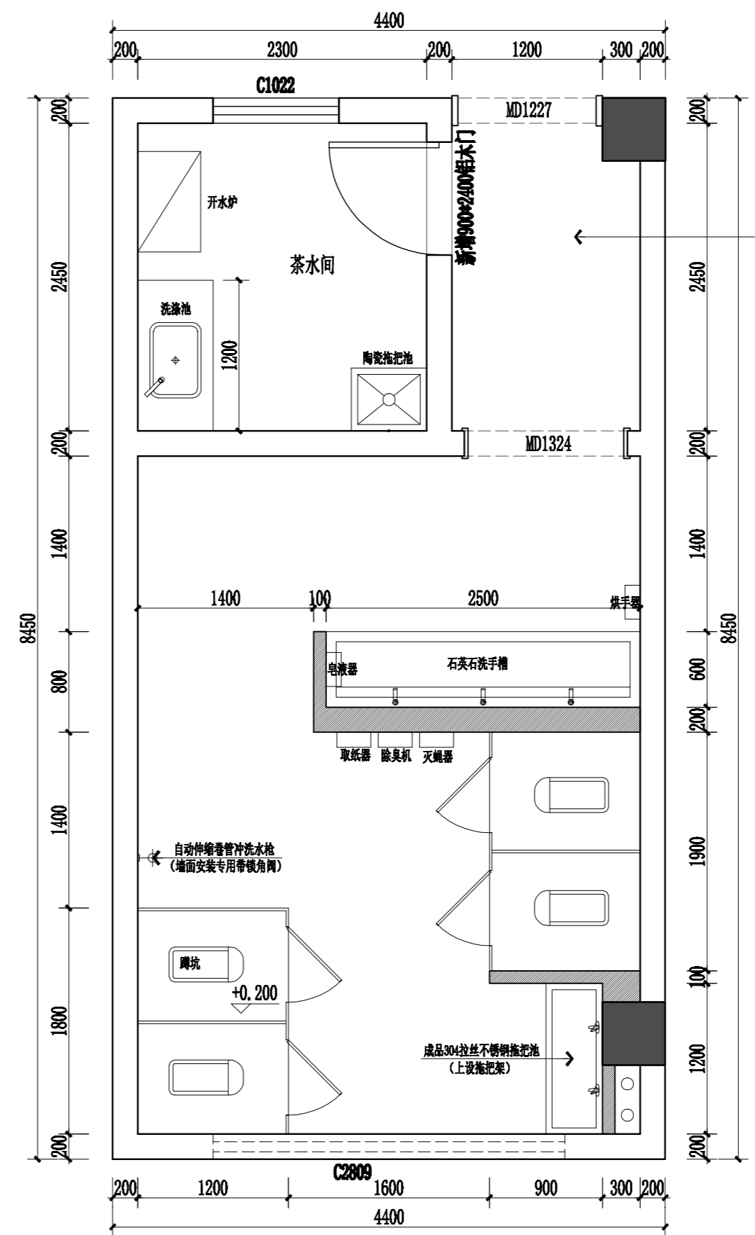
行政楼二层卫生间改造平面图 1:40
