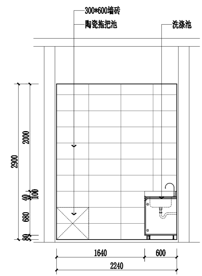
行政楼三层卫生间B立面图 1:40
