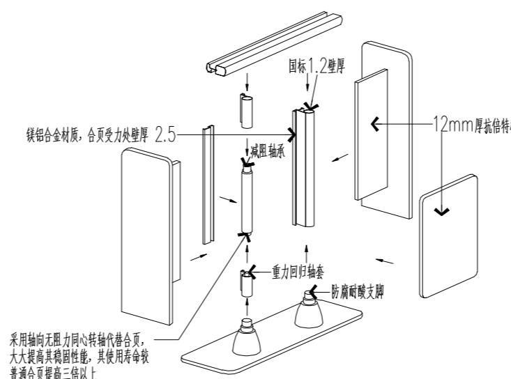
圆立柱隔断配件装配示意图
