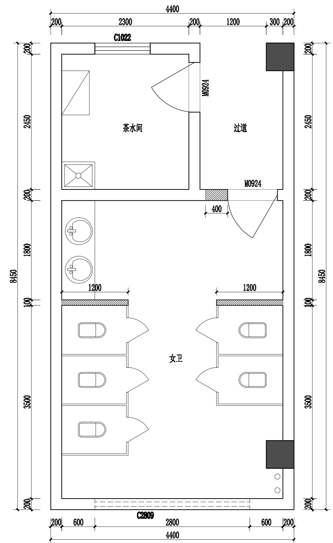
行政楼二层卫生间原始平面图 1:40 层高3800mm, 原吊顶标高2900mm
