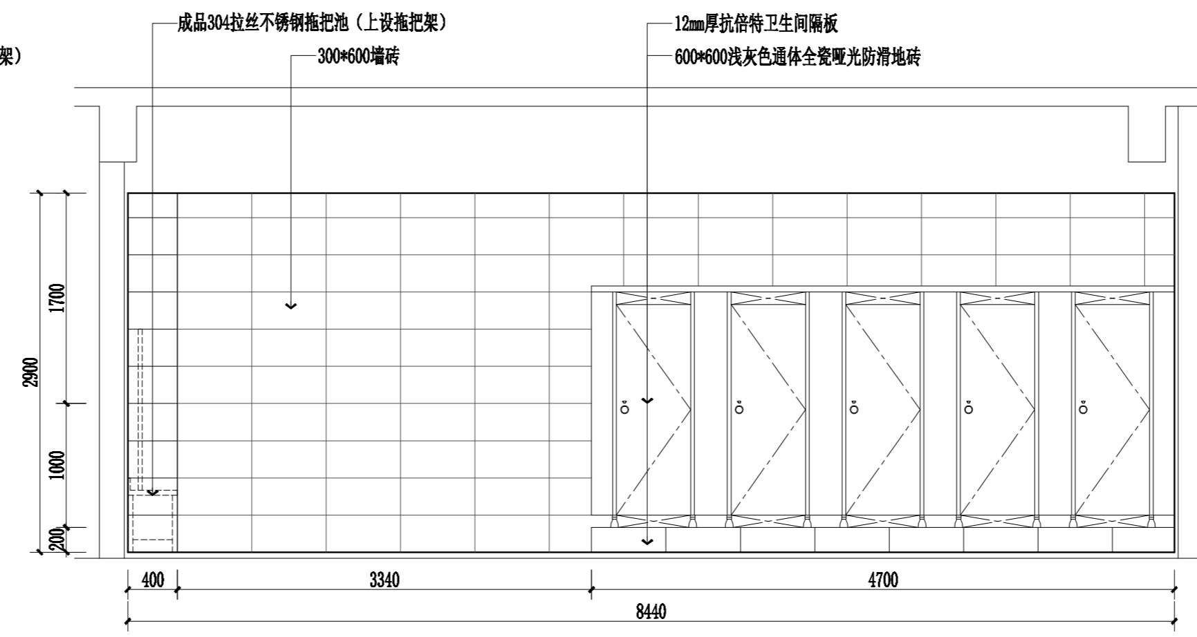
教学楼A一至四层卫生间C立面图 1:40
