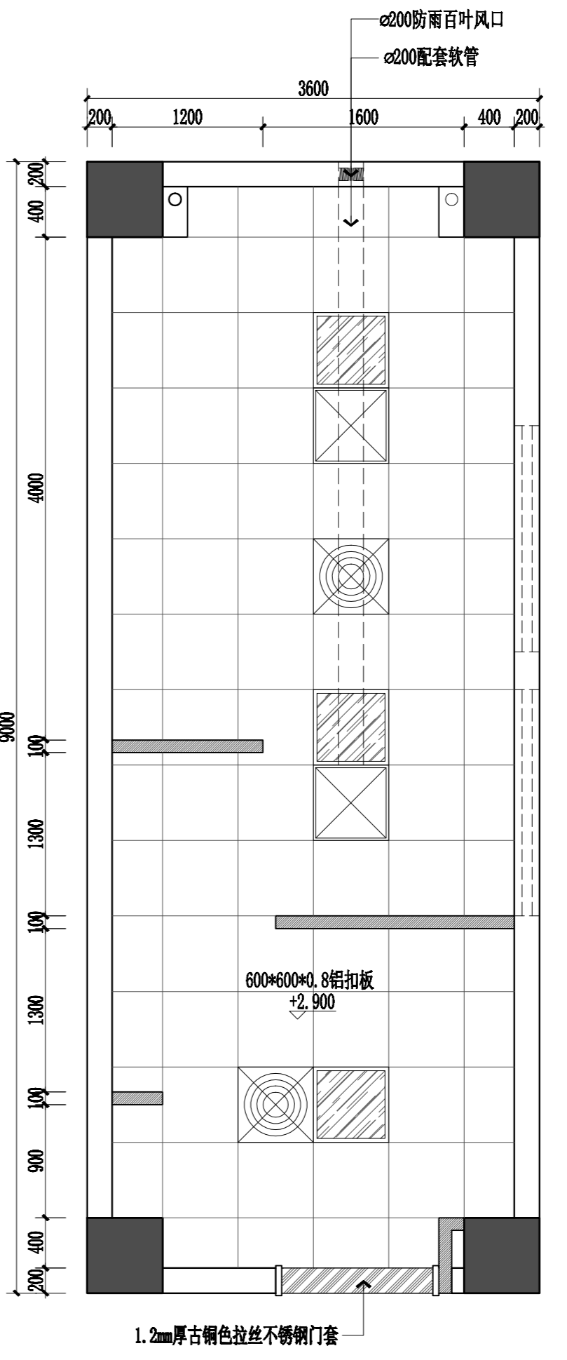
实验楼二至四层男厕顶面布置图 1:40
