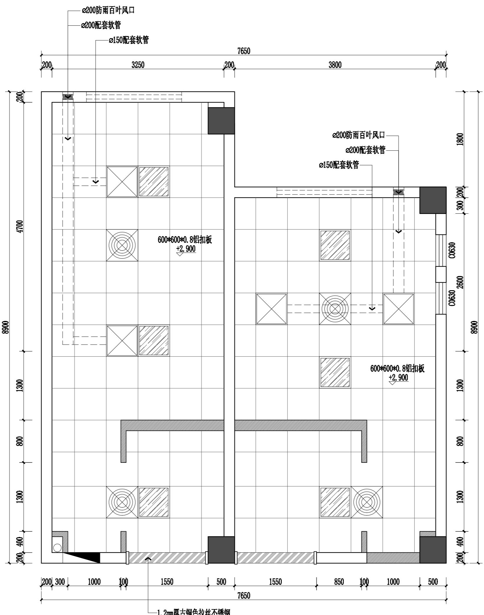
教学楼A一至四层卫生间顶面布置图 1:40
