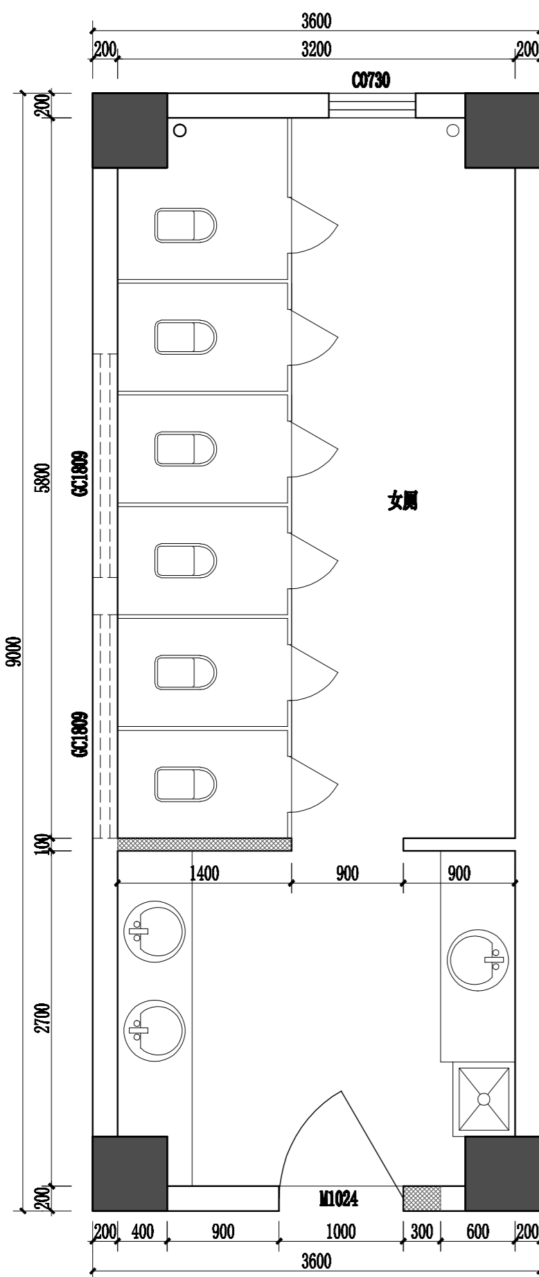
实验楼二至四层女厕原始平面图 1:40 层高3800mm, 原吊顶标高2900mm
