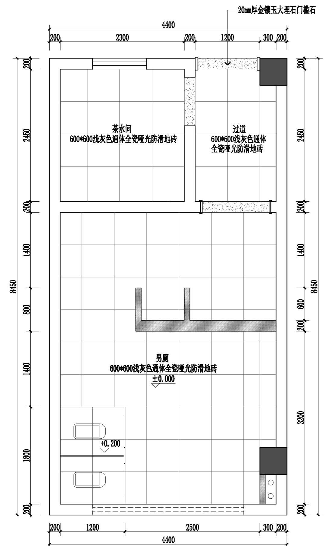
行政楼三层卫生间地面材质图 1:40
