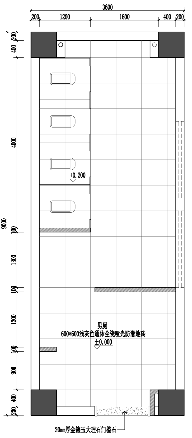
实验楼二至四层男厕地面材质图 1:40
