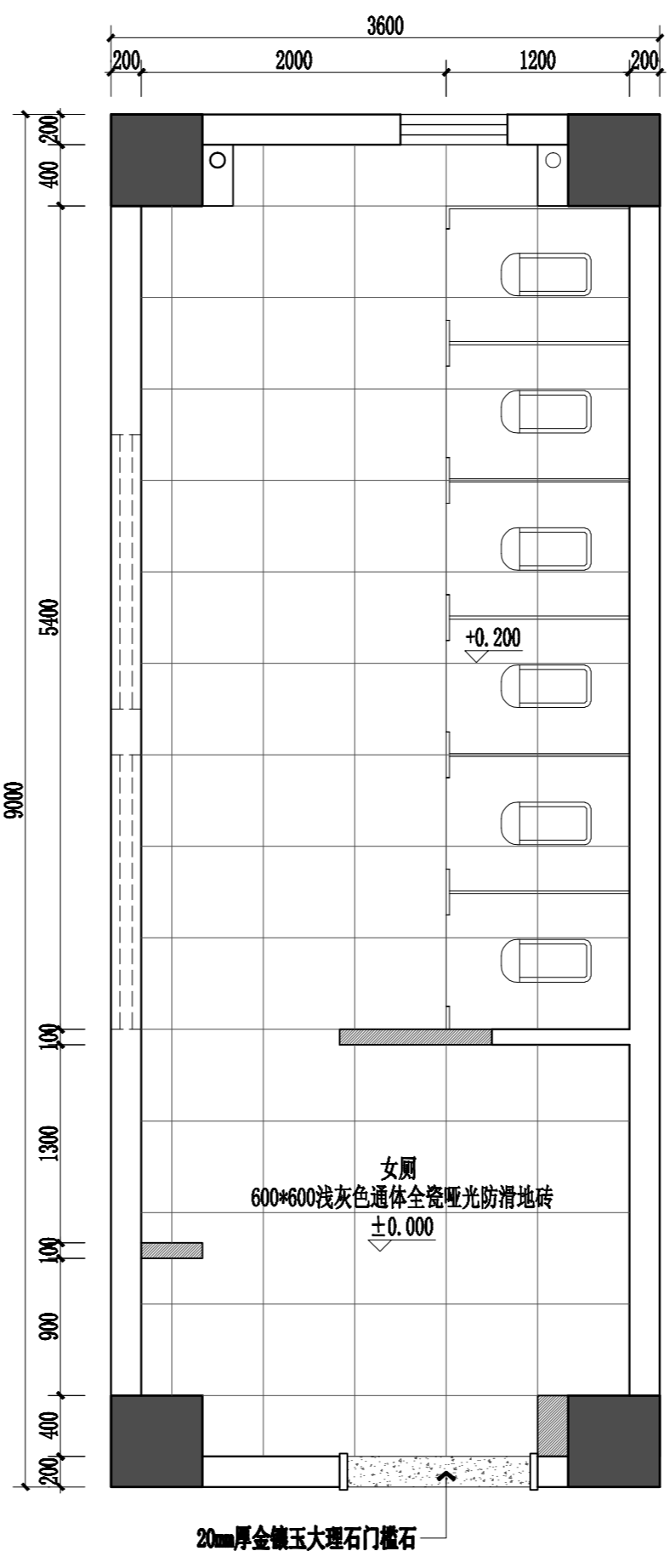
实验楼二至四层女厕地面材质图 1:40
