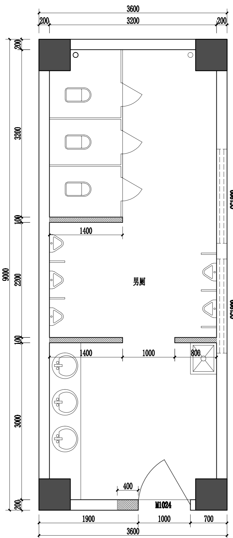
实验楼二至四层男厕原始平面图 1:40
