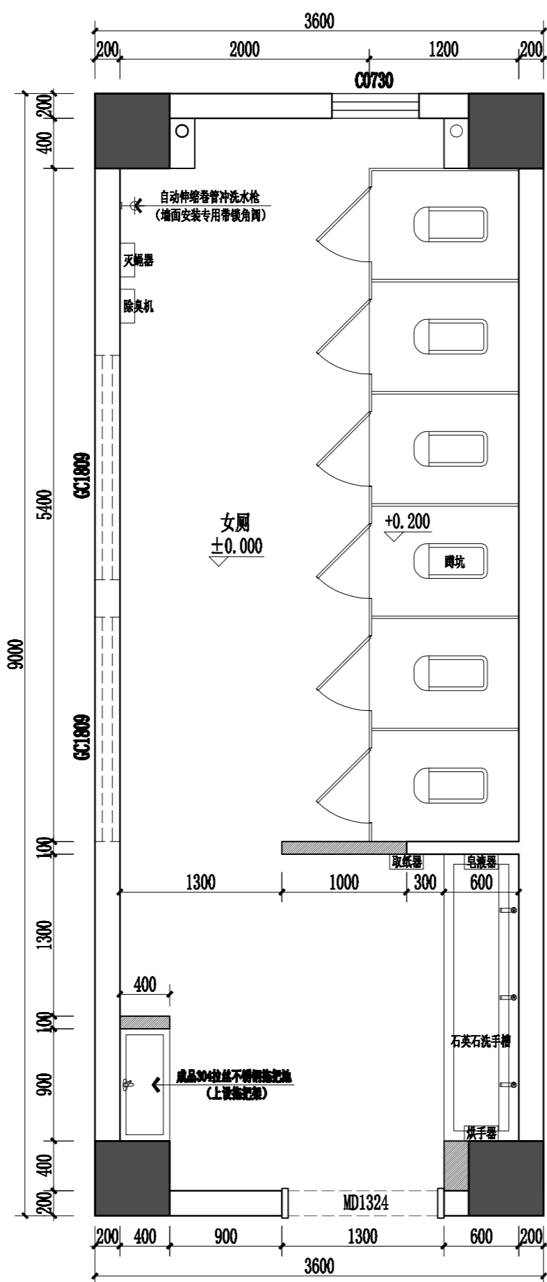
实验楼二至四层女厕改造平面图 1:40
