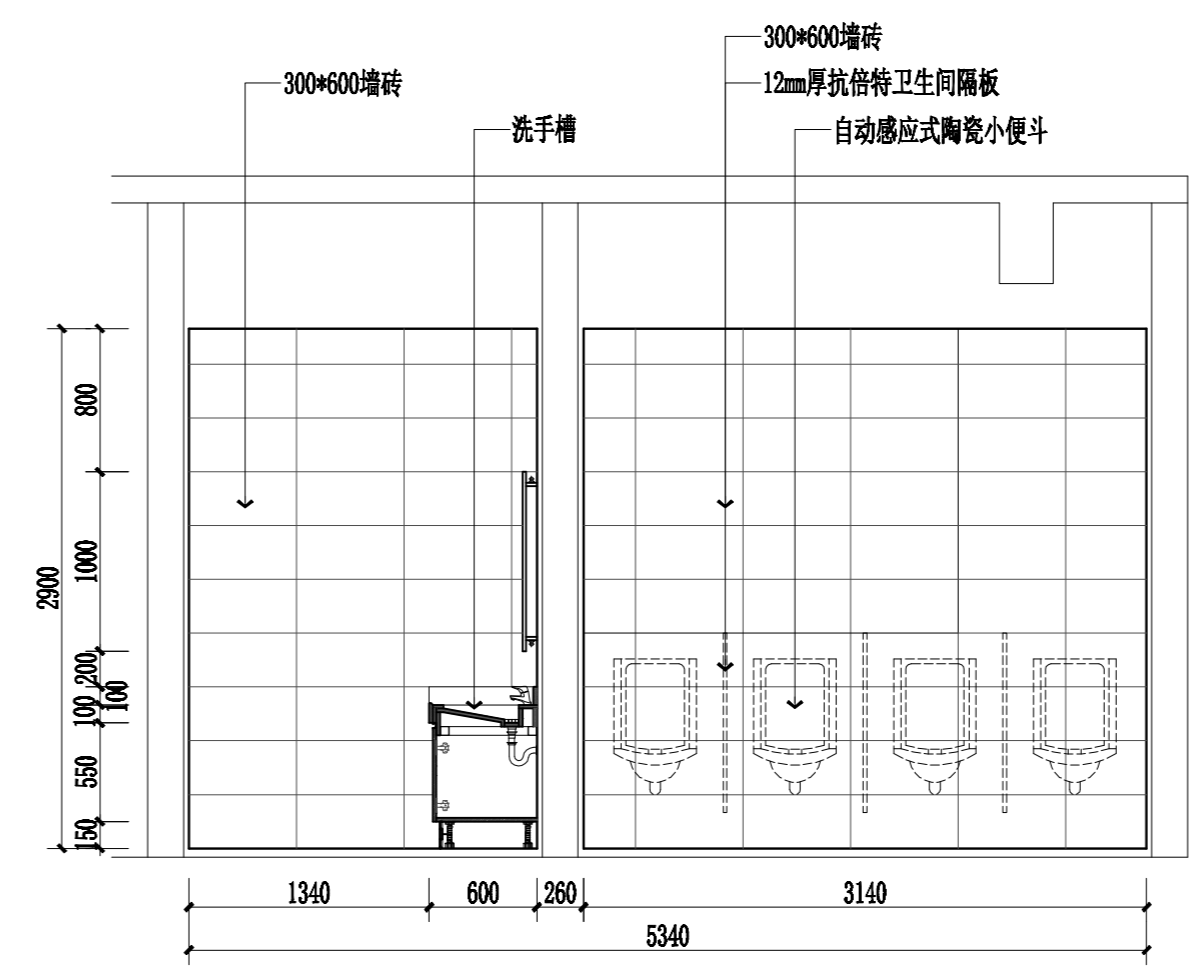
行政楼三层卫生间E立面图 1:40
