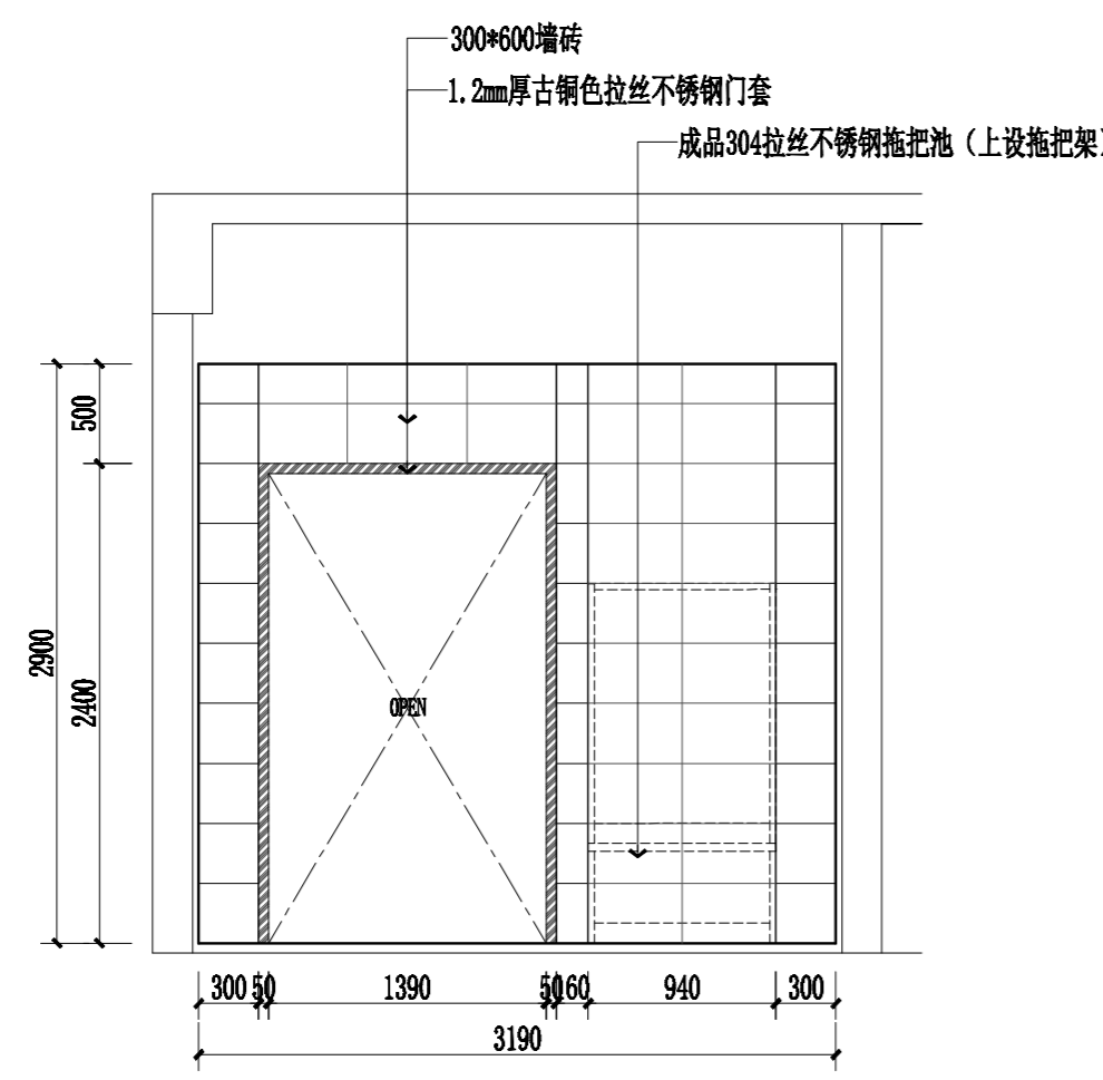
教学楼A一至四层卫生间A立面图 1:40
