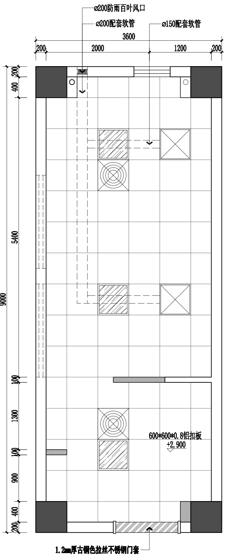
实验楼二至四层女厕顶面布置图 1:40
