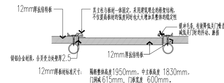
圆立柱隔断配件剖面图
