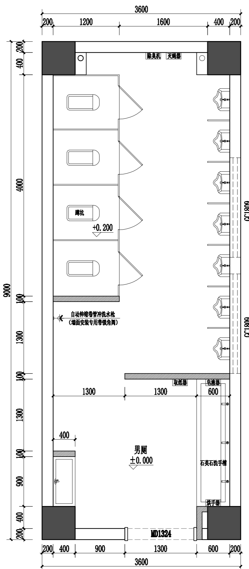
实验楼二至四层男厕改造平面图 1:40
