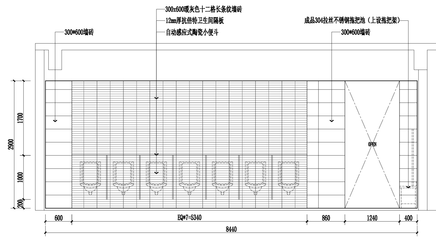
教学楼A一至四层卫生间D立面图 1:40
