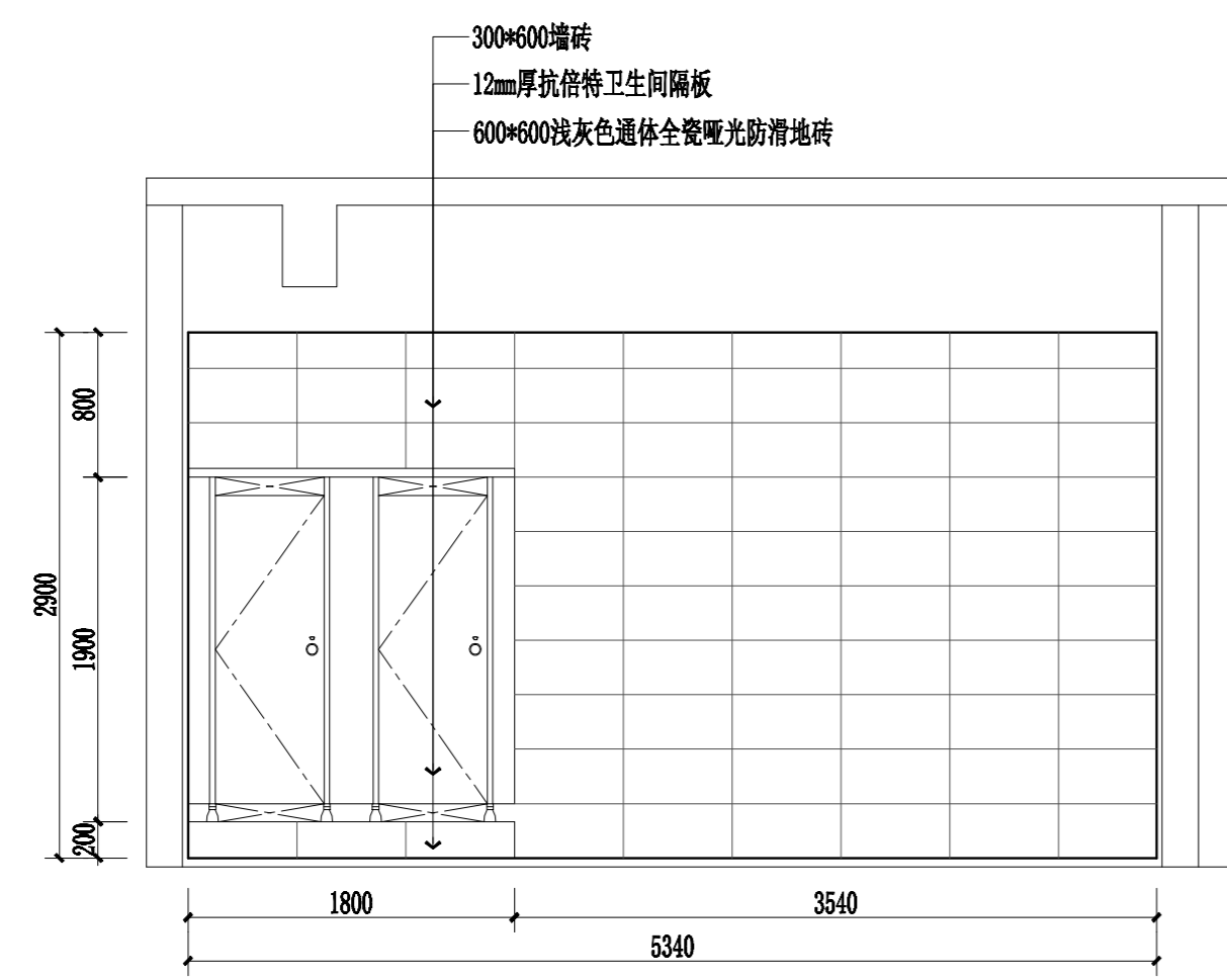
行政楼三层卫生间D立面图 1:40
