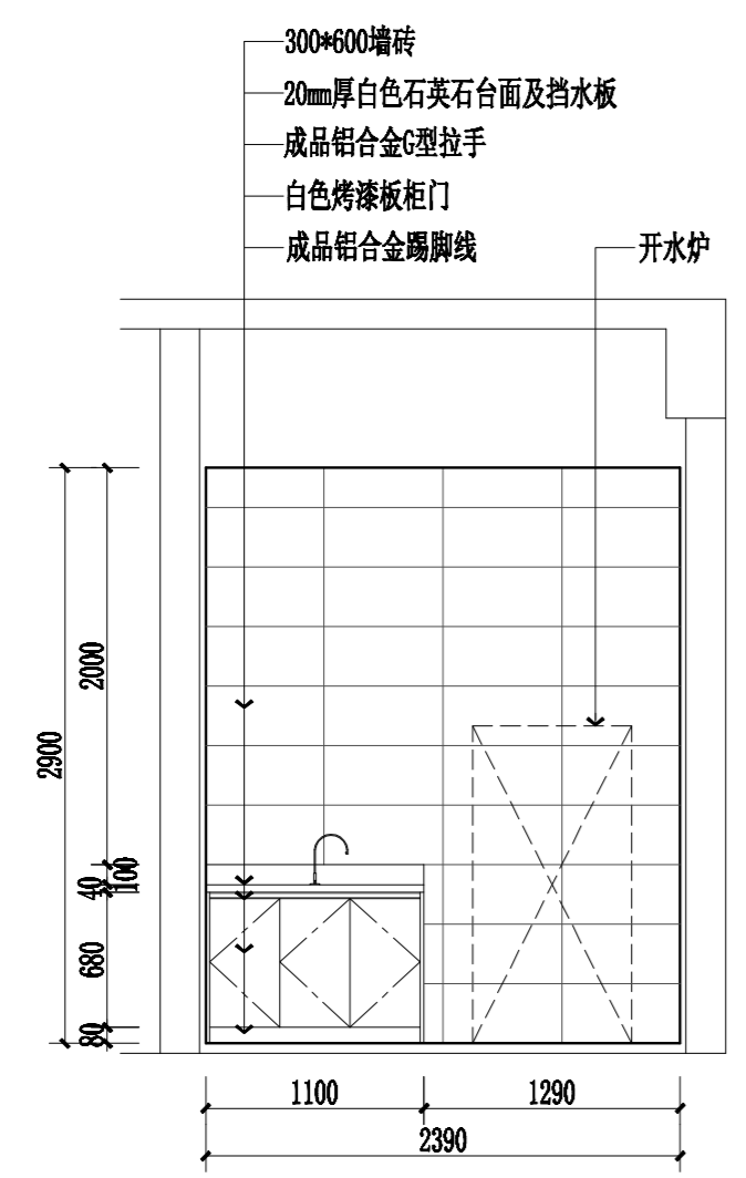
行政楼三层卫生间A立面图 1:40
