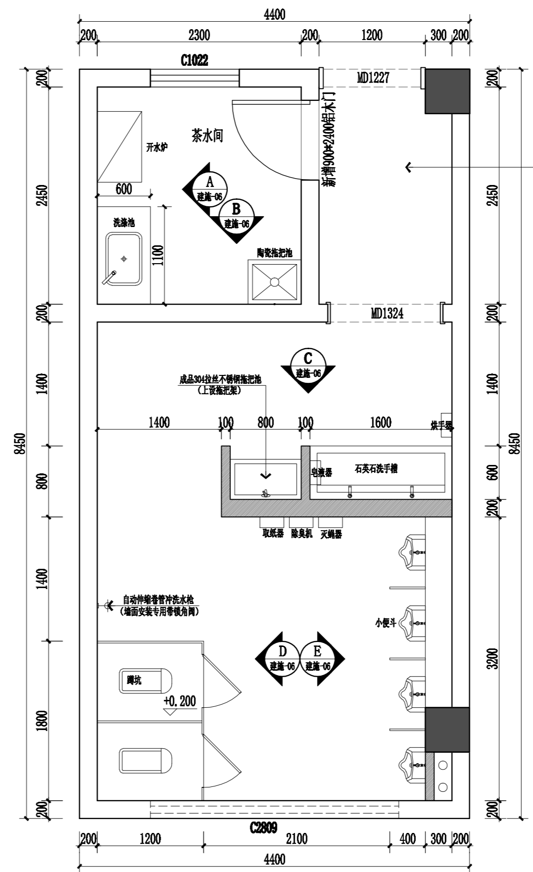
行政楼三层卫生间改造平面图 1:40
