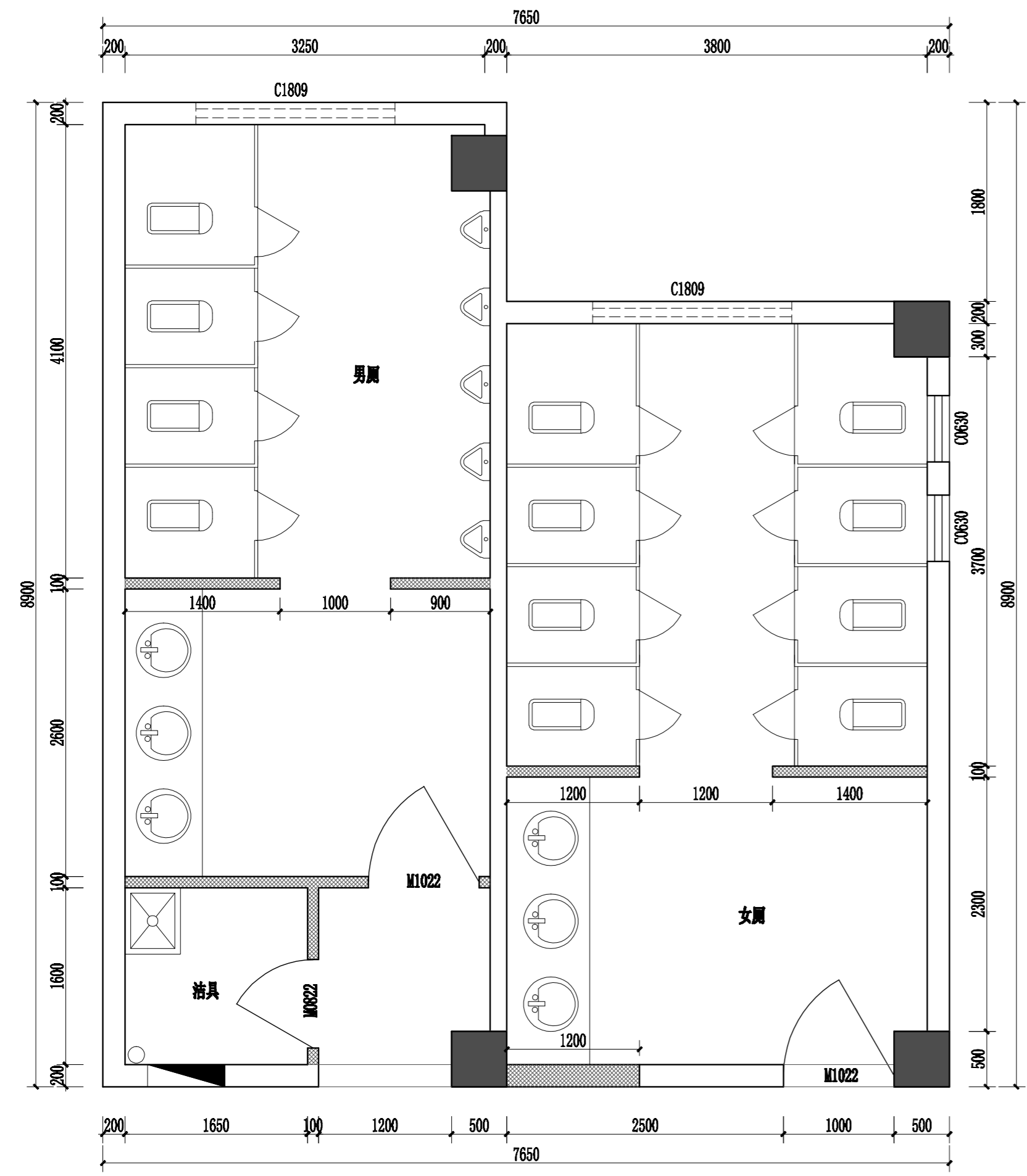
教学楼A一至四层卫生间原始平面图 1:40
