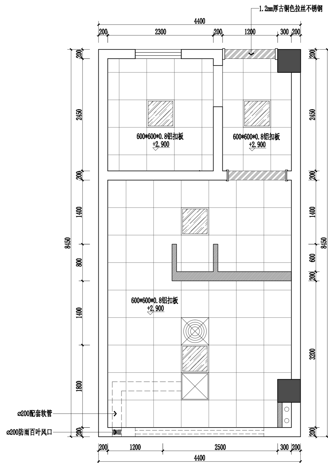
行政楼三层卫生间顶面布置图 1:40
