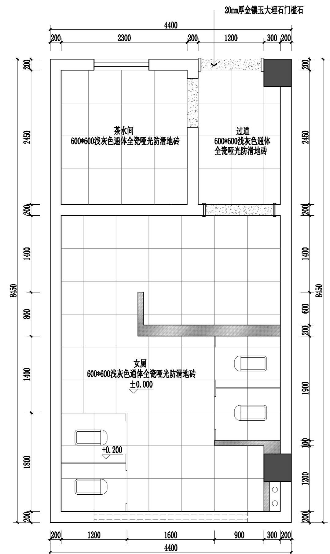
行政楼二层卫生间地面材质图 1:40
