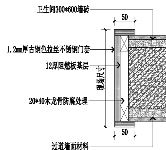
不锈钢门套剖面图 1:5
