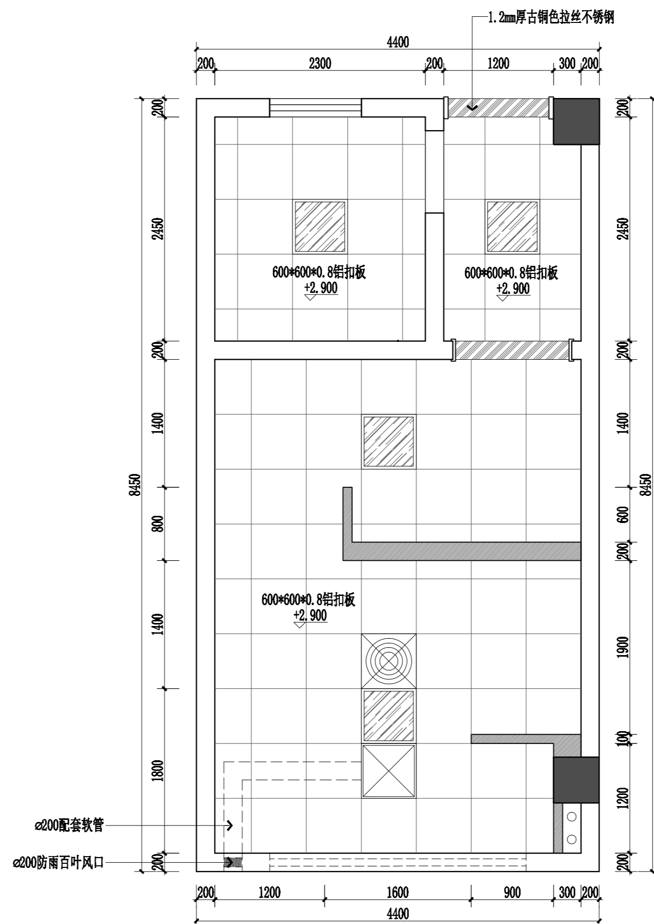
行政楼二层卫生间顶面布置图 1:40
