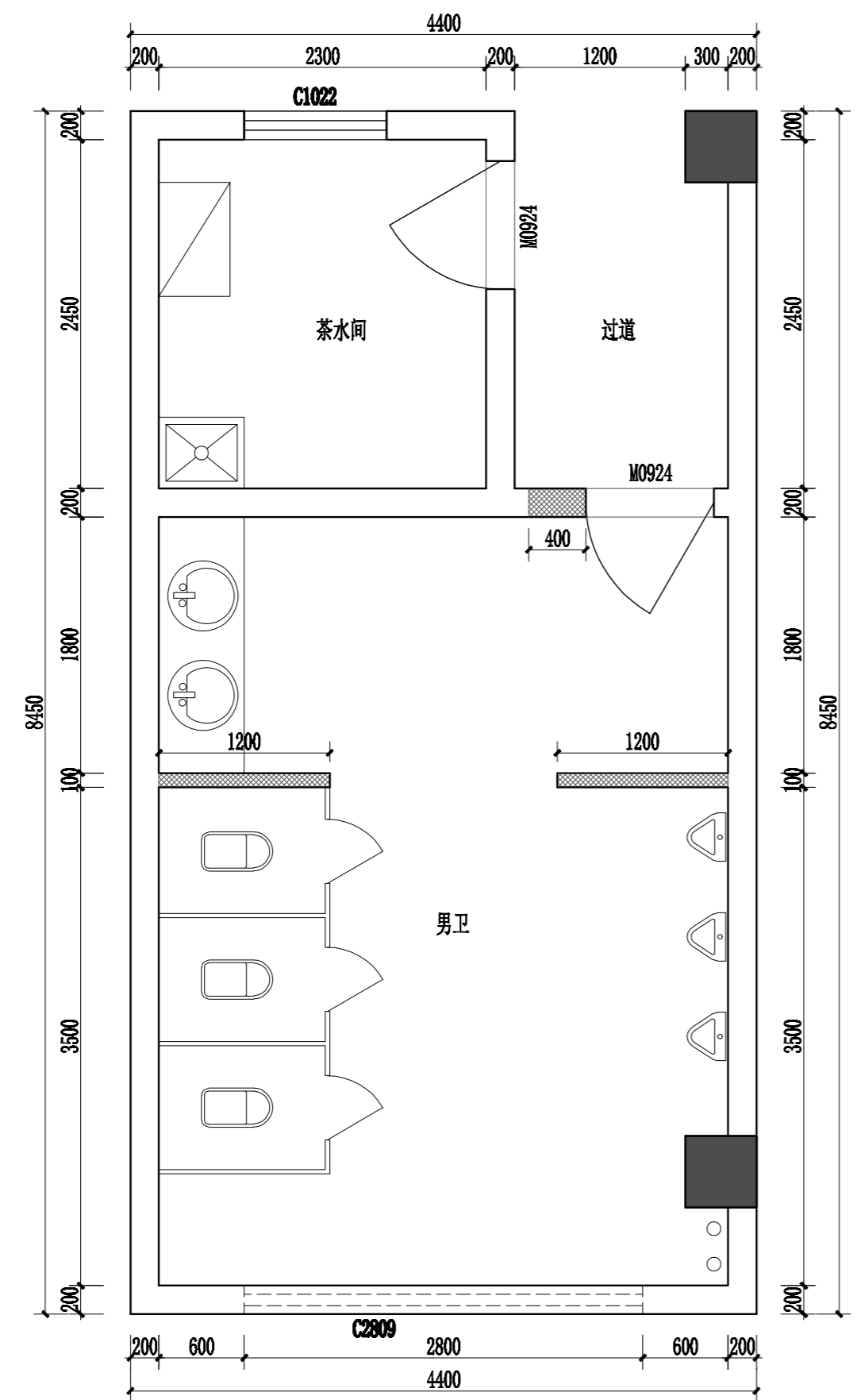
行政楼三层卫生间原始平面图 1:40 层高3800mm, 原吊顶标高2900mm
