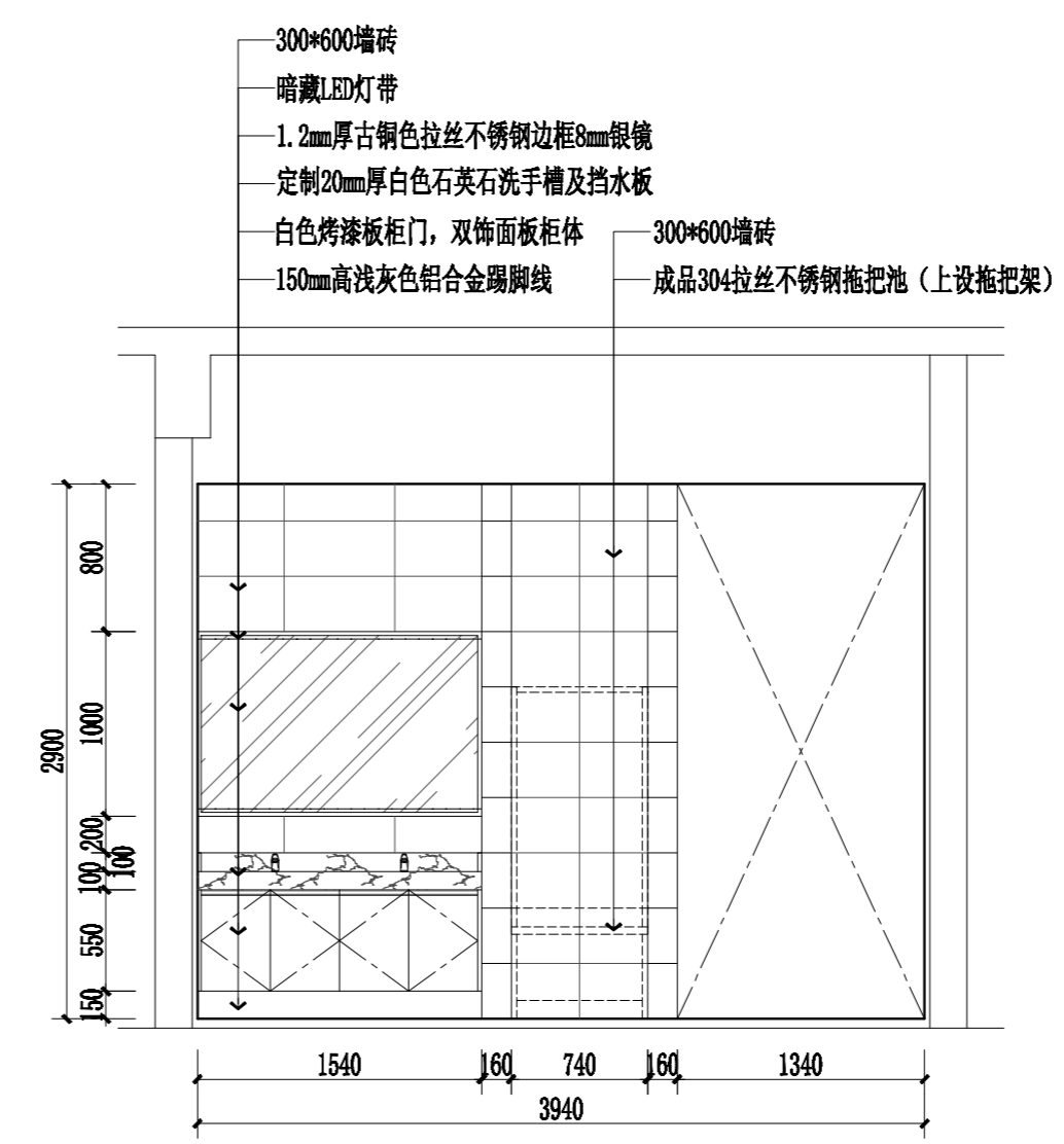
行政楼三层卫生间C立面图 1:40
