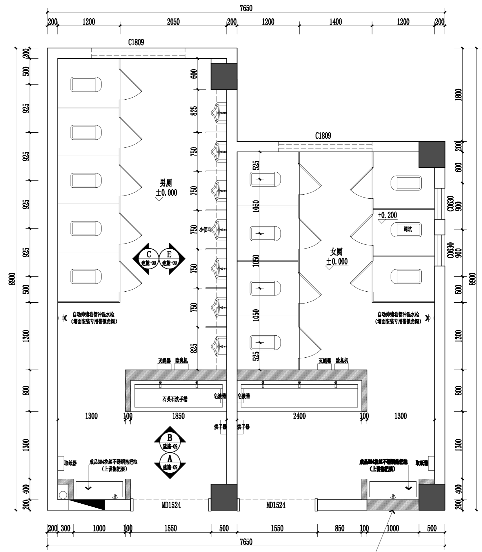
教学楼A一至四层卫生间改造平面图 1:40
