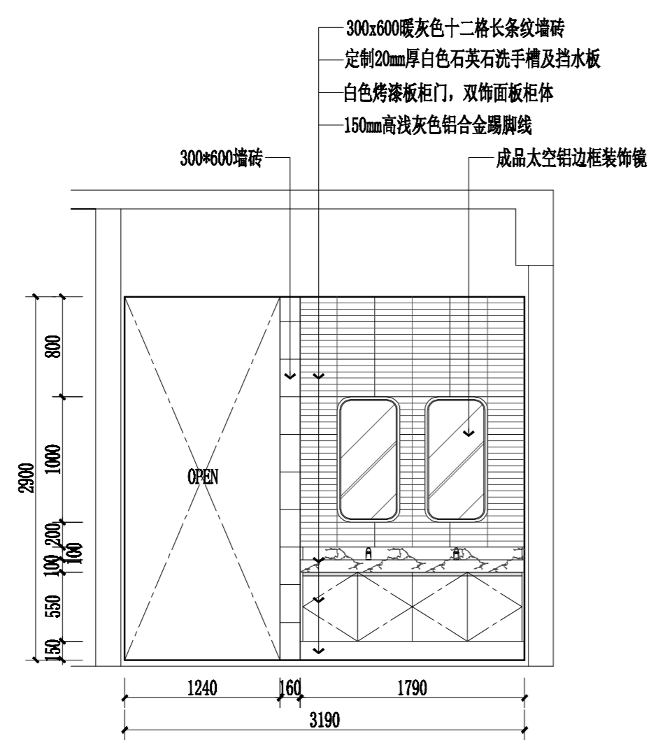
教学楼A一至四层卫生间B立面图 1:40
