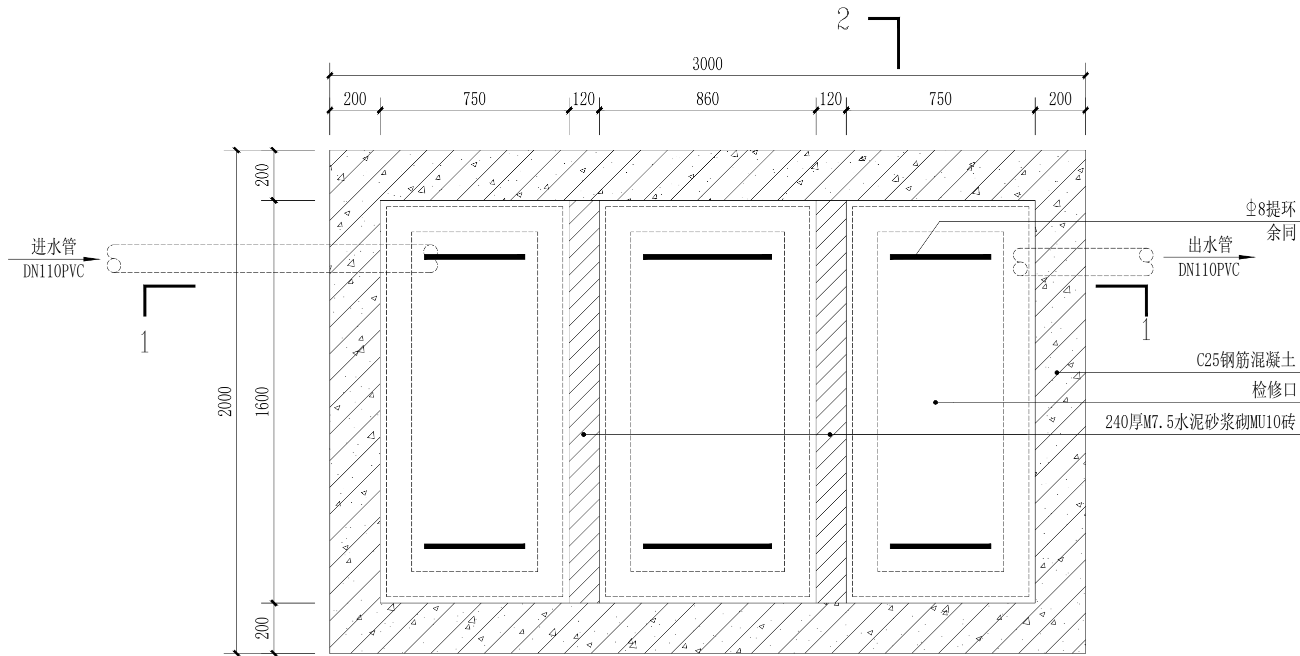
化粪池平面图 1:15
