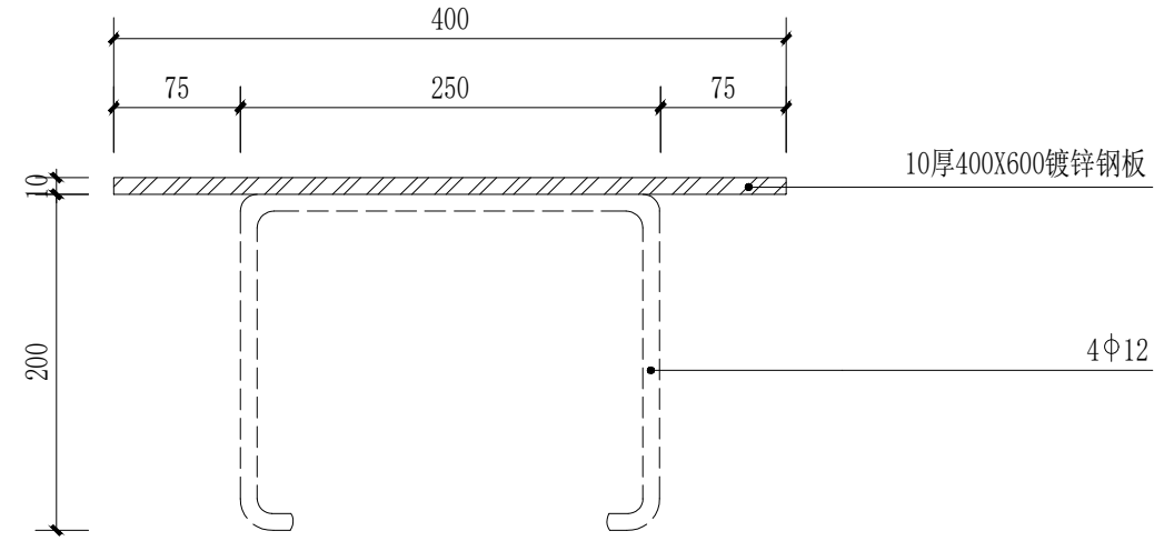
预埋件立面图 1:5
