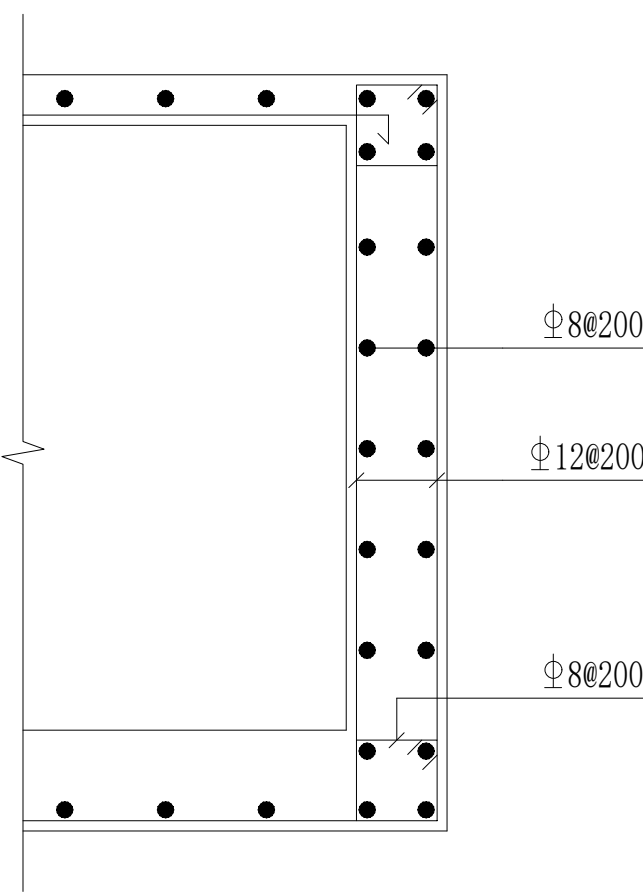
a-a剖面图 1:15
