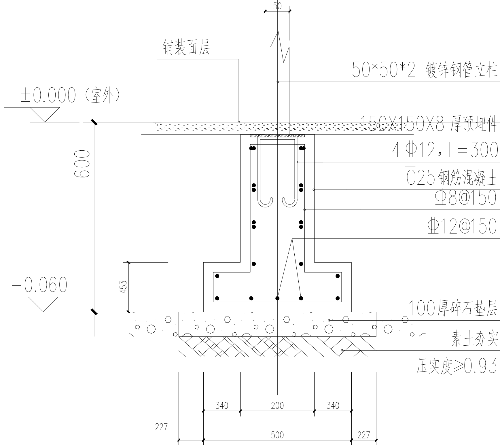
1-1剖面图 1:20
