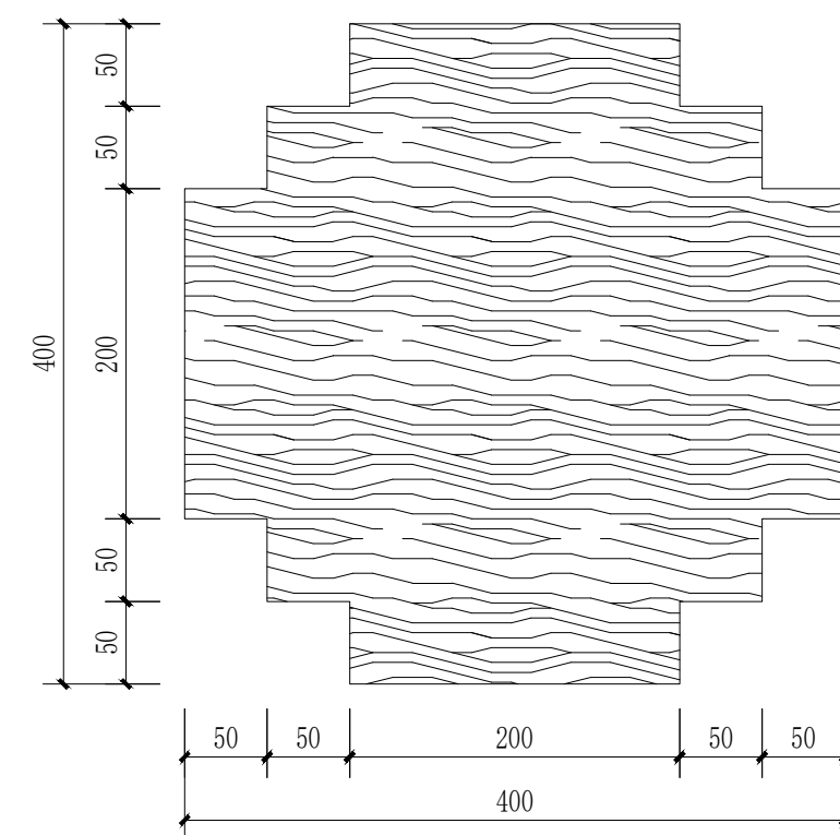
防腐木柱截面 1:5
