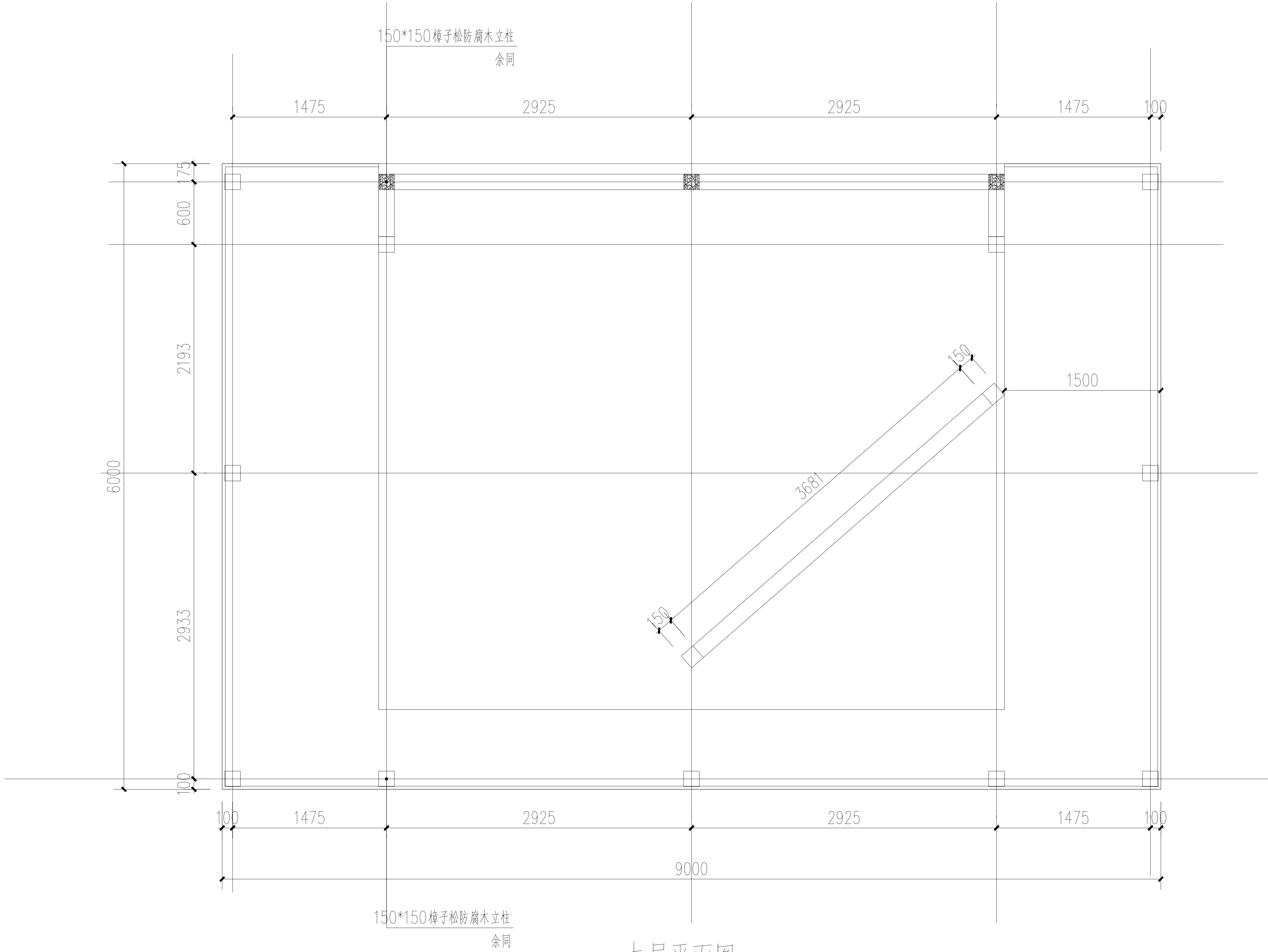
木屋平面图 1:20
