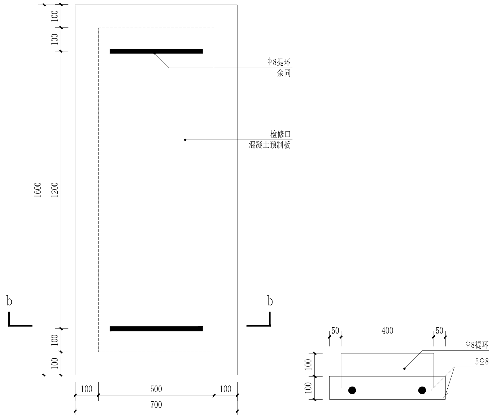
检修口大样图 1:10
