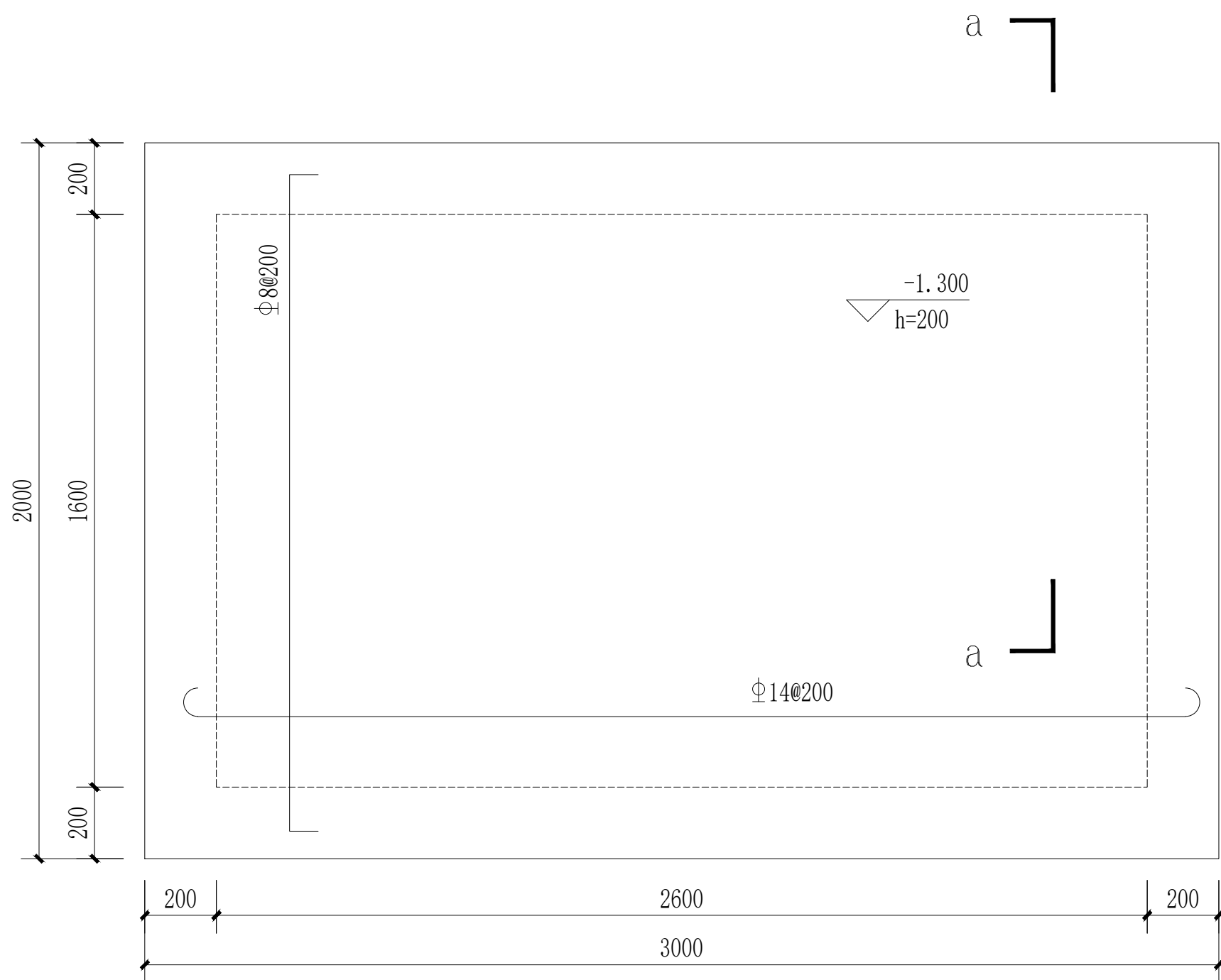
化粪池结构布置平面图 1:15
