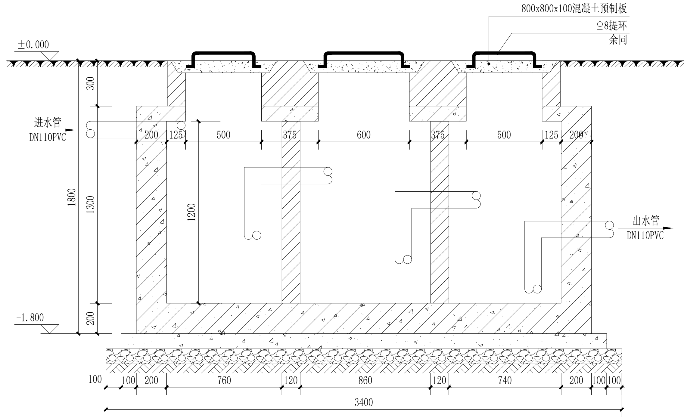
1-1剖面图 1:15
