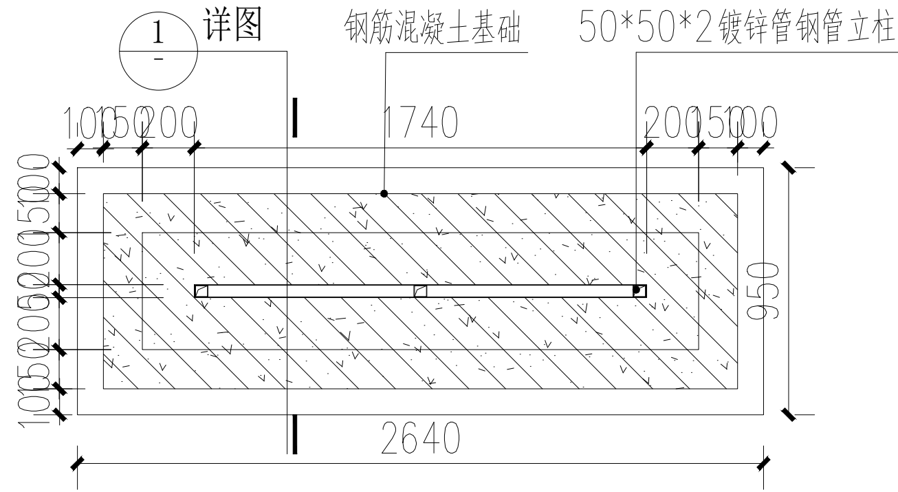
基础平面图 1:20
