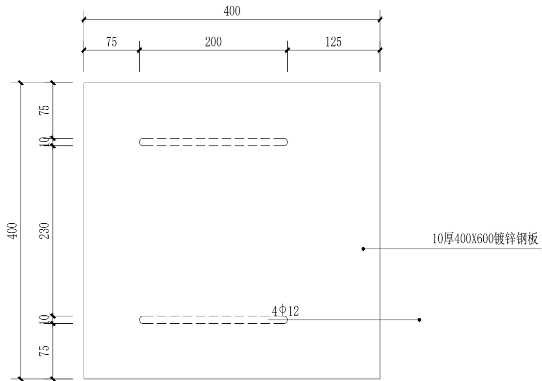
预埋件平面图 1:5
