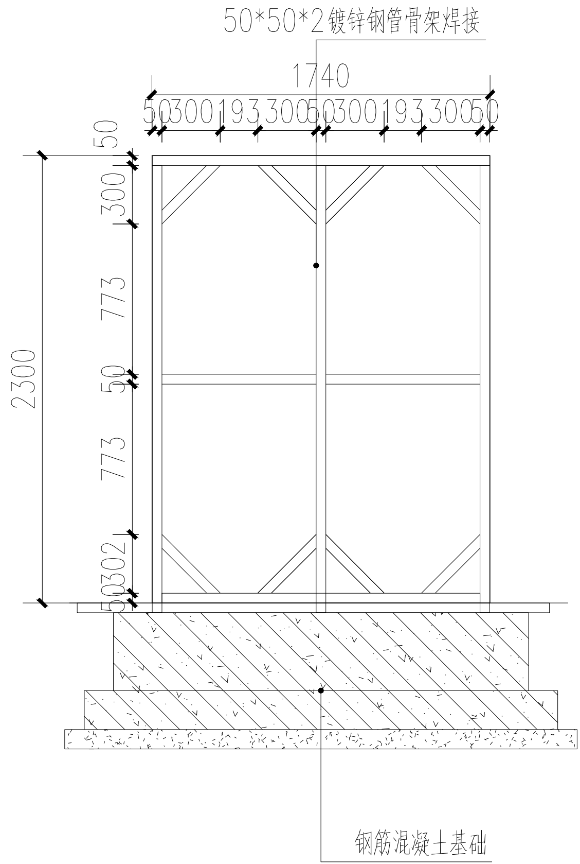
横剖面图 1:20
