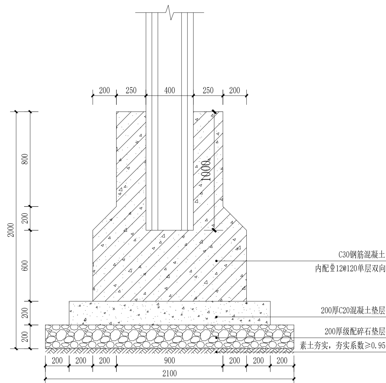
柱基础做法 1: 20
