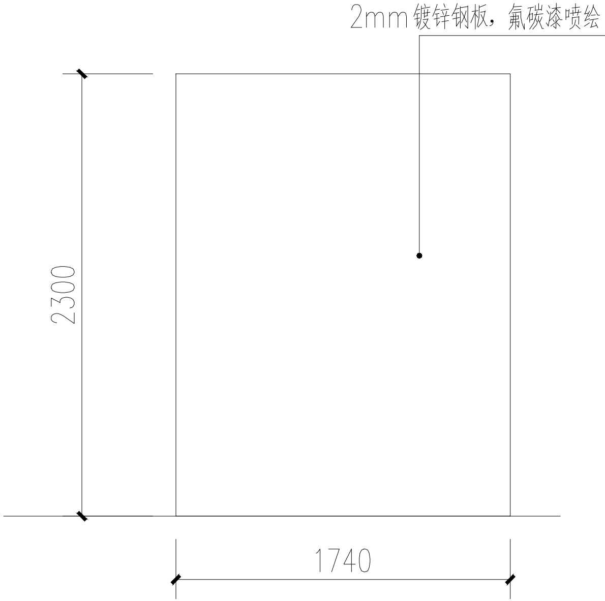
正立面图 1:20
