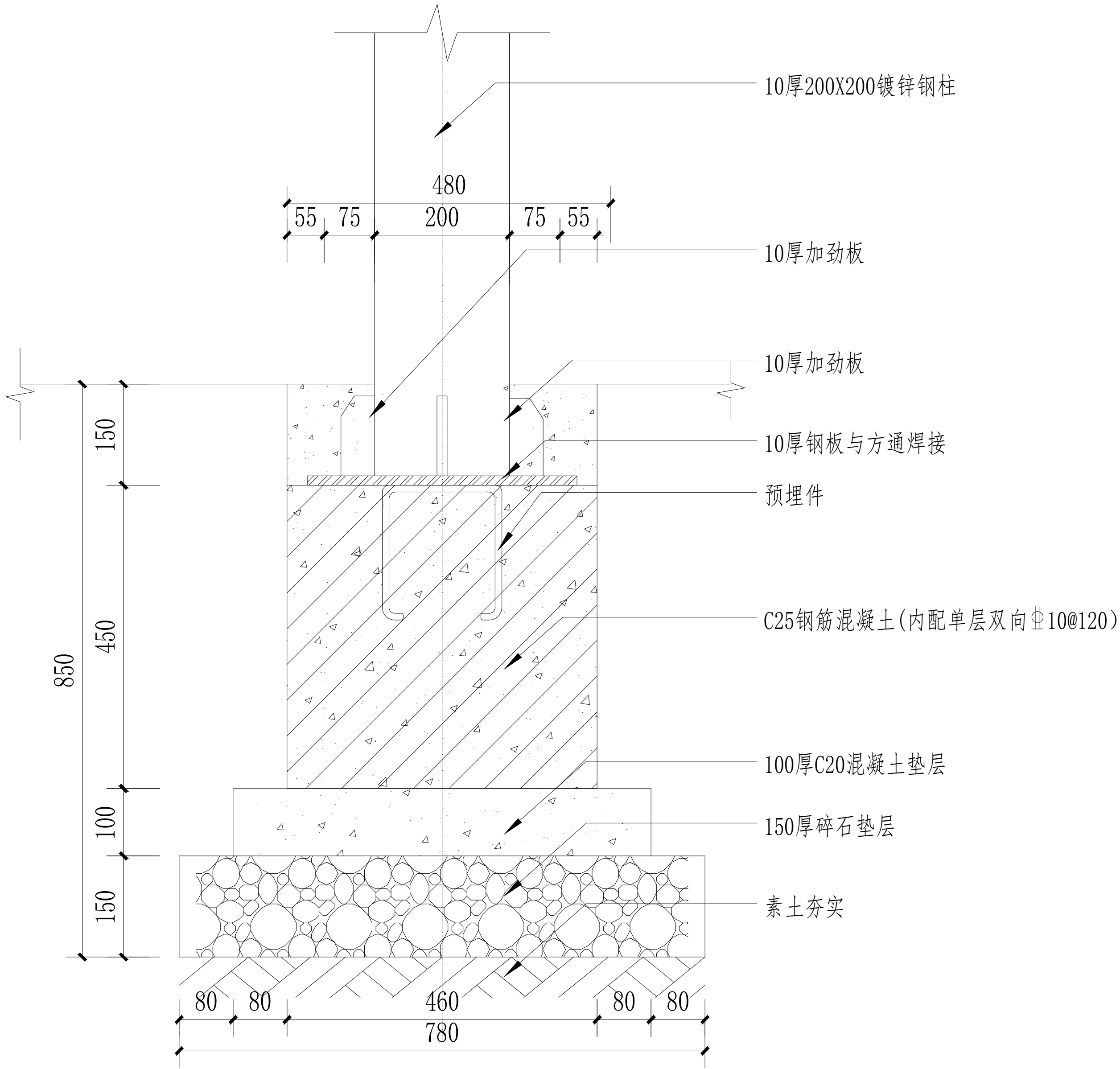
卫生间柱基础 1:5
