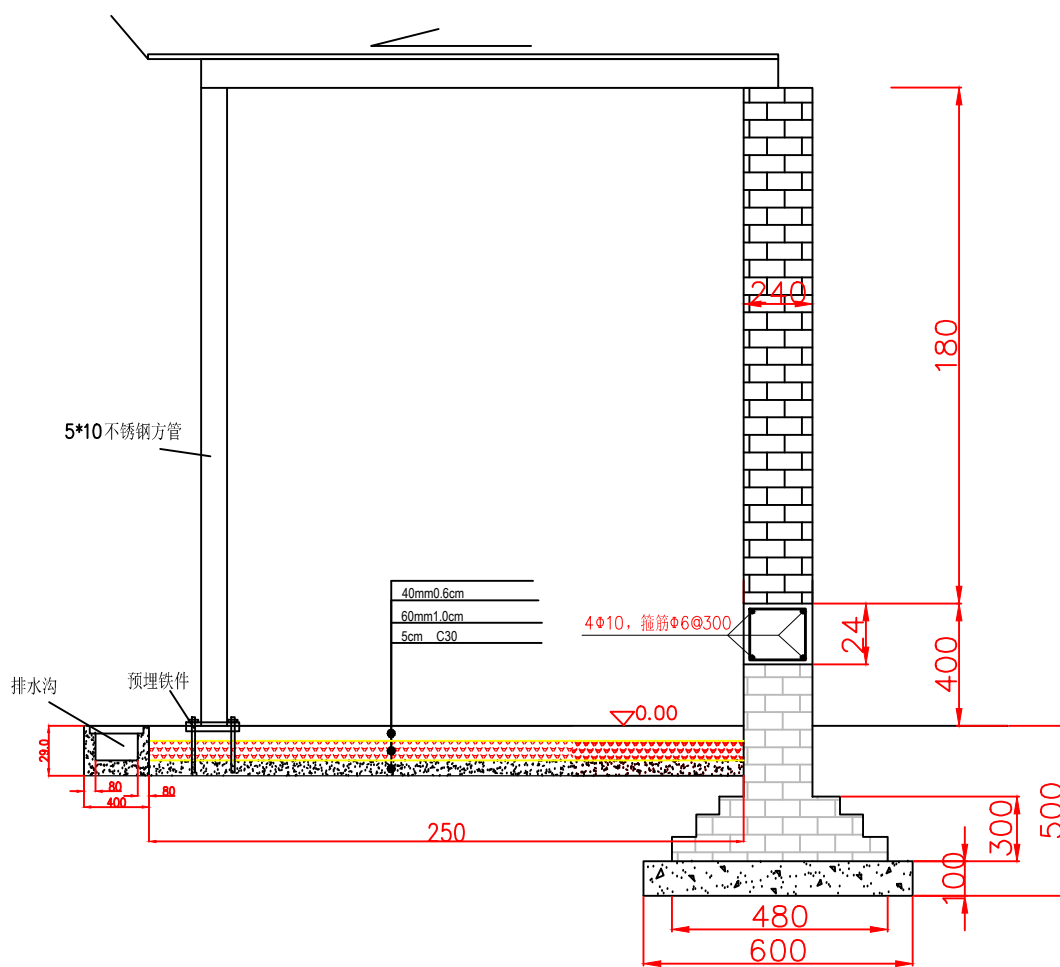
基础大样图
