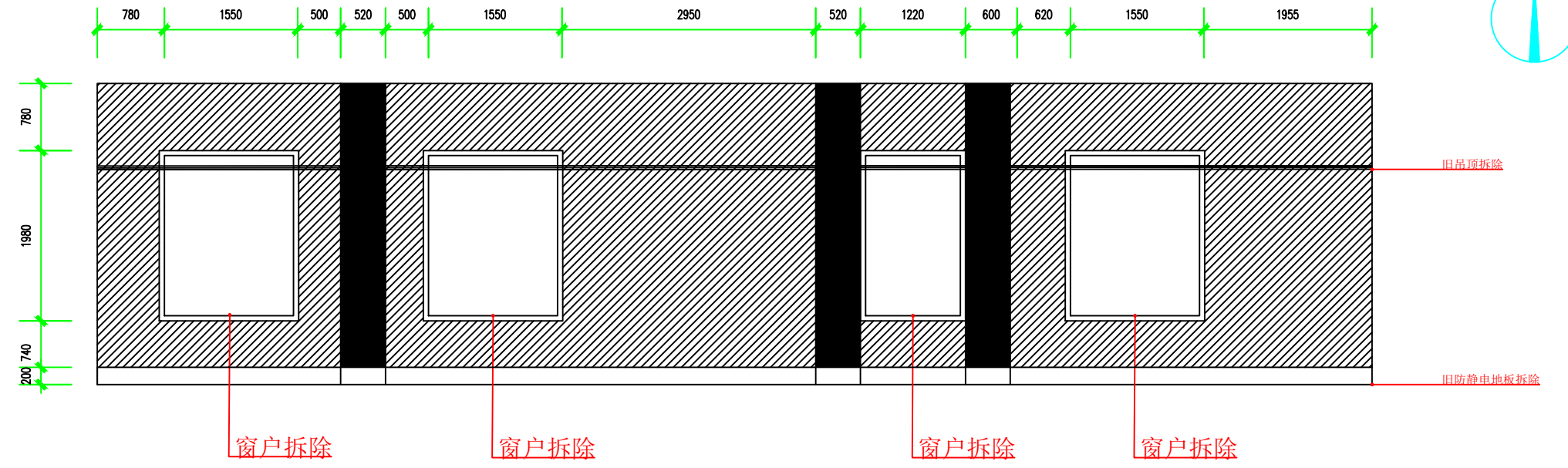
北侧墙面现状立面图
