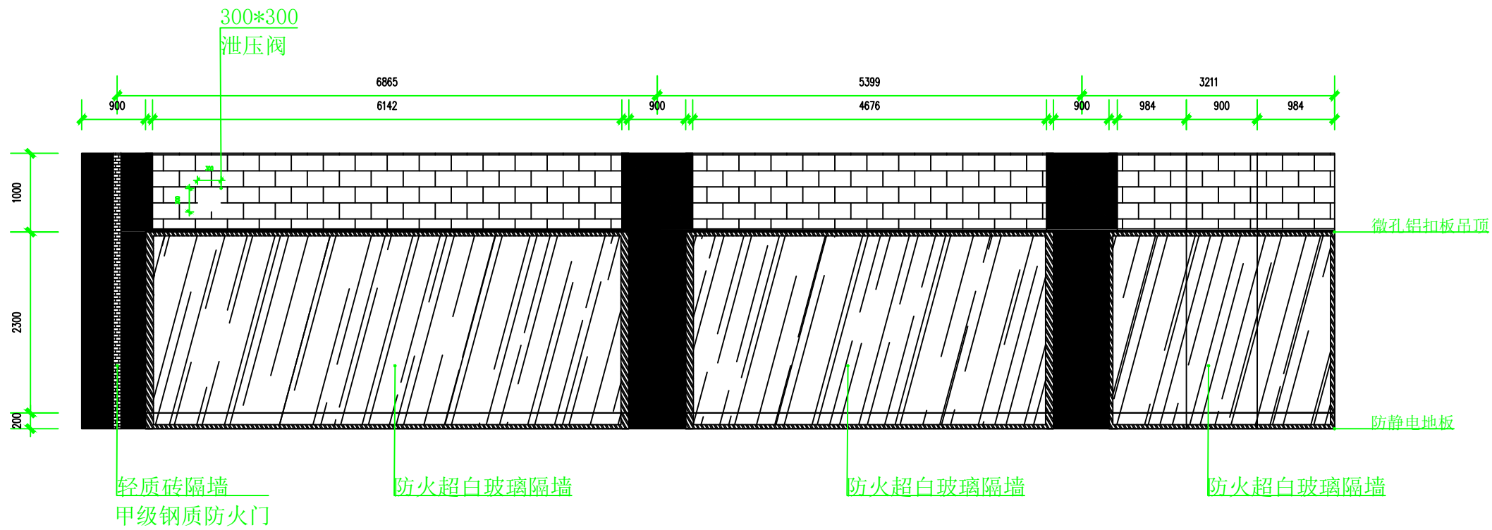
南側墙面装修立面图
