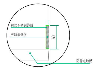
踢脚线做法大样图
