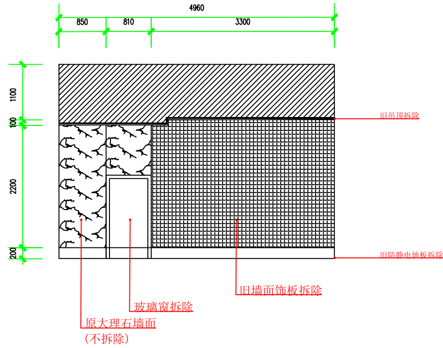
东侧墙面现状立面图
