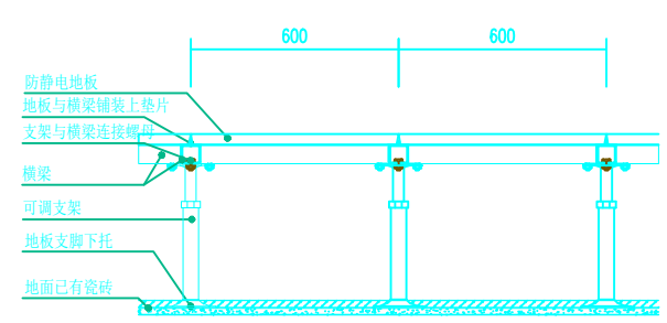
防静电地板铺装立面图
