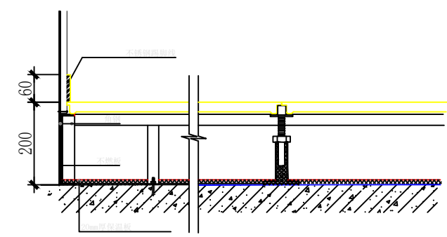
地面铺设剖面图
