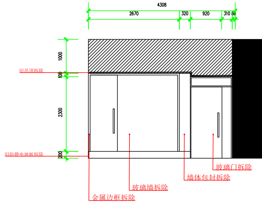
西側墙面现状立面图
