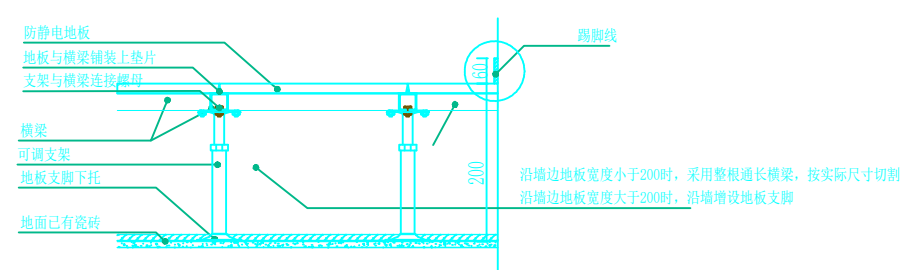
防静电地板沿墙支撑立面图
