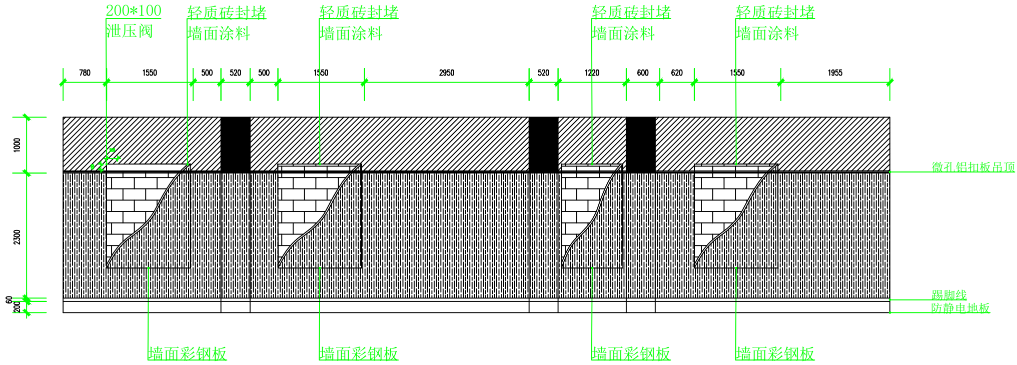
北侧墙面装修立面图
