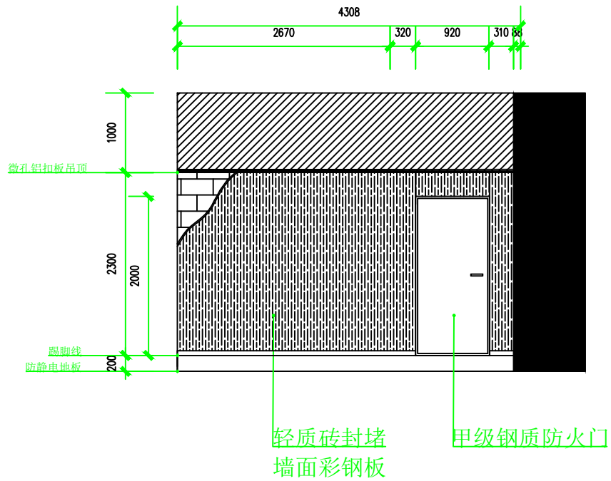
西側墙面装修立面图
