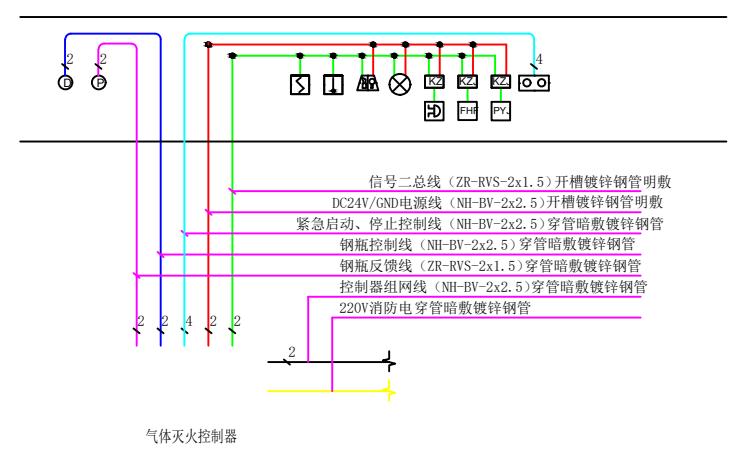
柜式七氟丙烷气体灭火装置电气控制原理图
