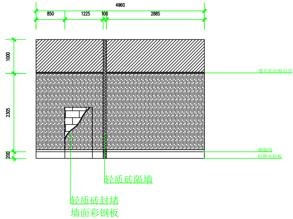
东侧墙面装修立面图
