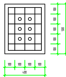
平面配筋
