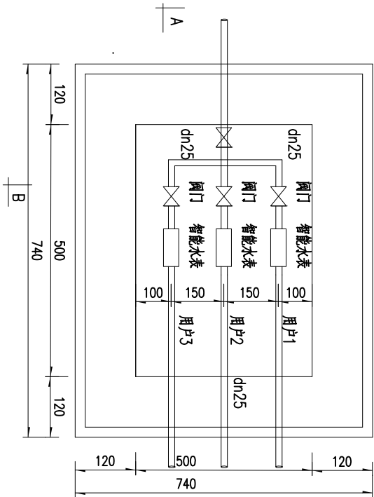
入户水表井平面图 (2-3户)
