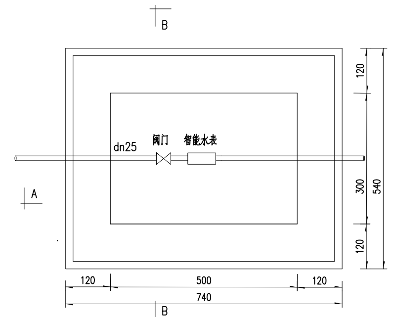
入户水表井平面图（单户）
