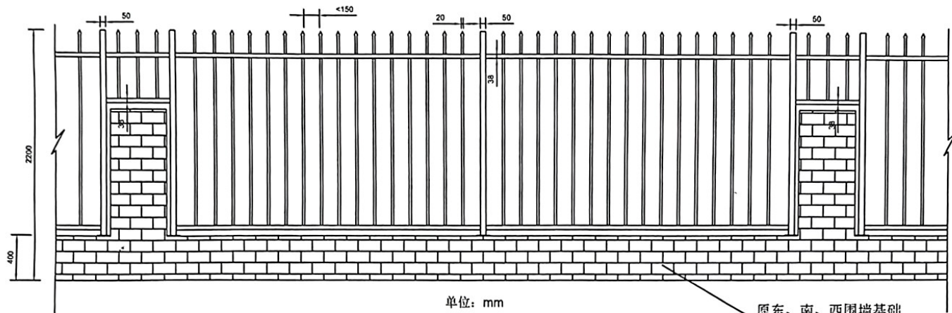
宜陵地涵上游安全维护设施 (C型)
