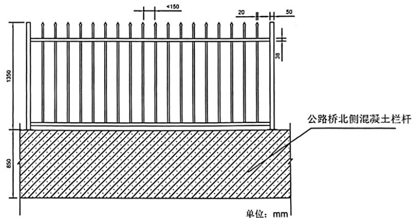
宜陵地涵上游安全维护设施 (C型)
