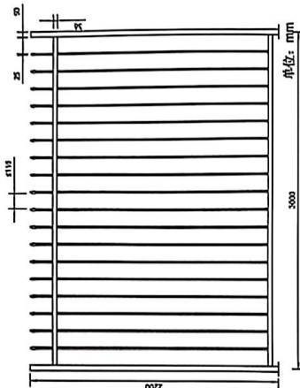
一站上游高水闸东侧至进水闸上游左岸翼墙安全围护设施（D型）
