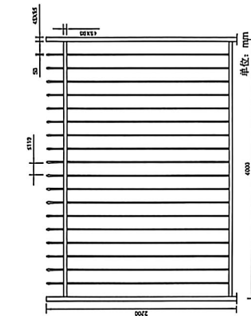
东闸北岸头至进水闸下游左岸翼墙安全围护设施（G型）
