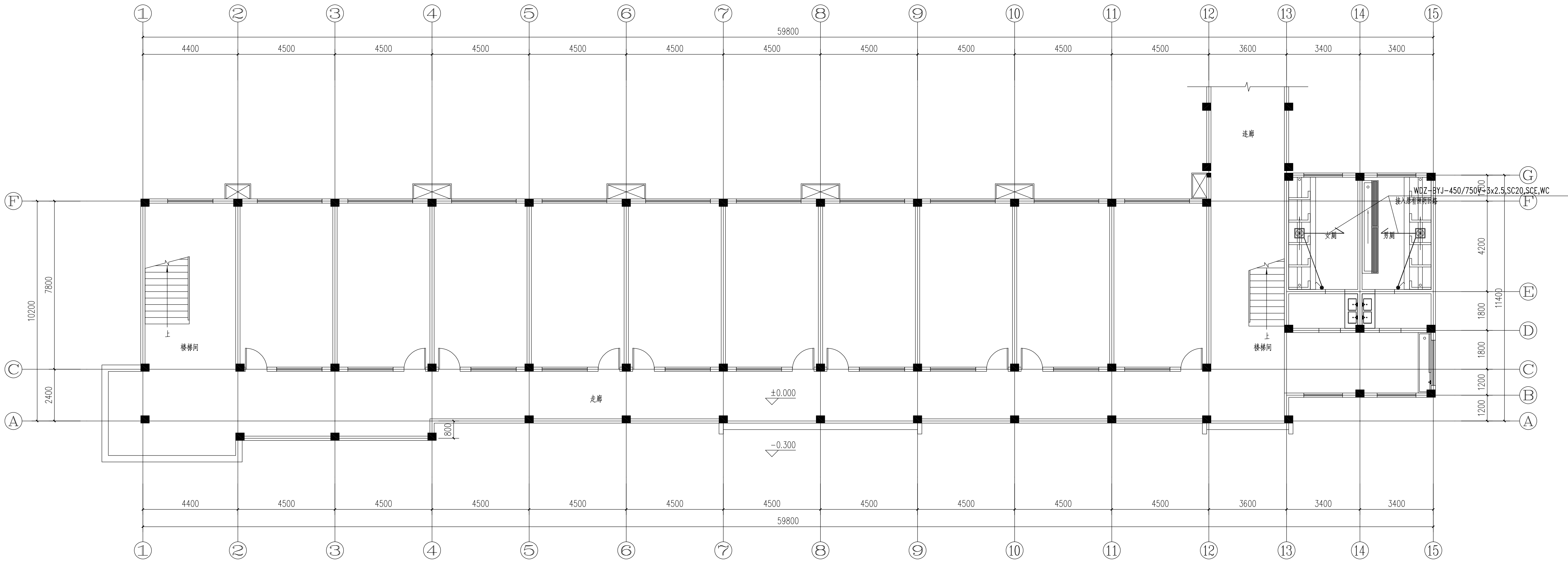
至善楼一~五层厕所配电平面图 1:100
