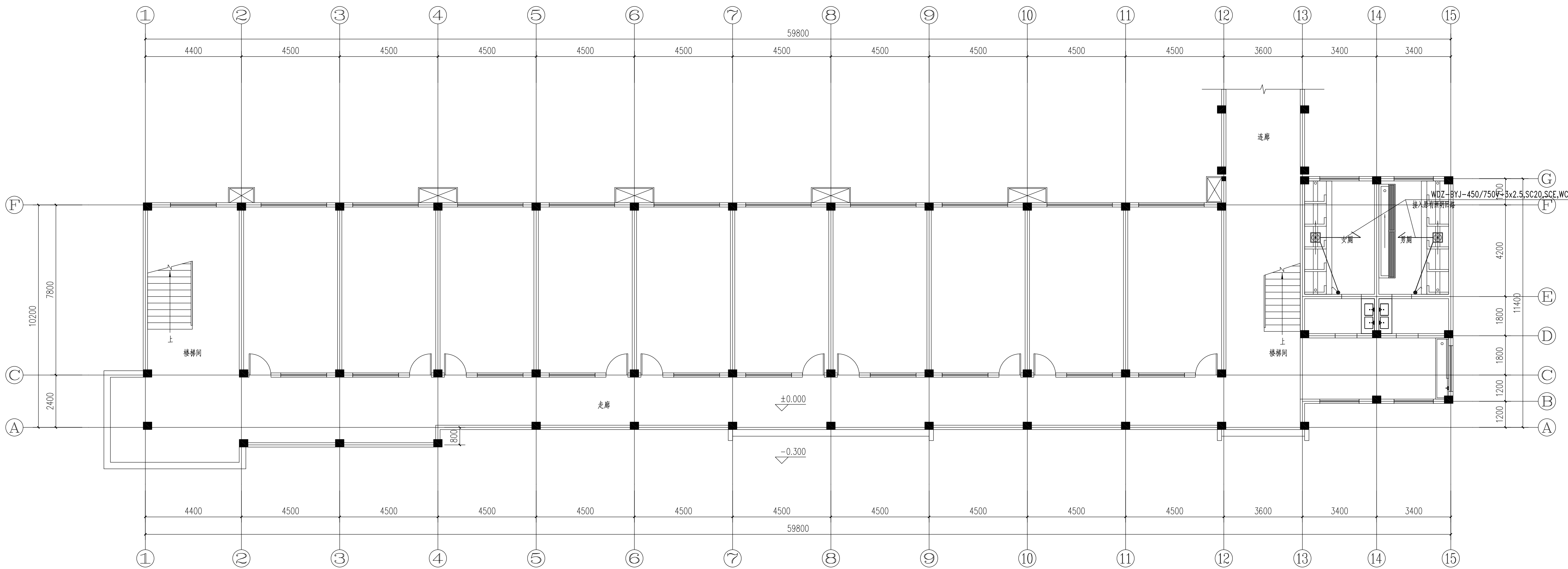
正心楼一~五层厕所配电平面图 1:100
