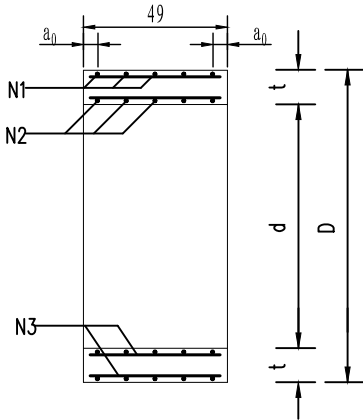
管节纵断面
