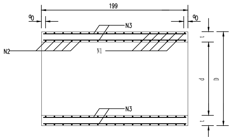
管节纵断面
