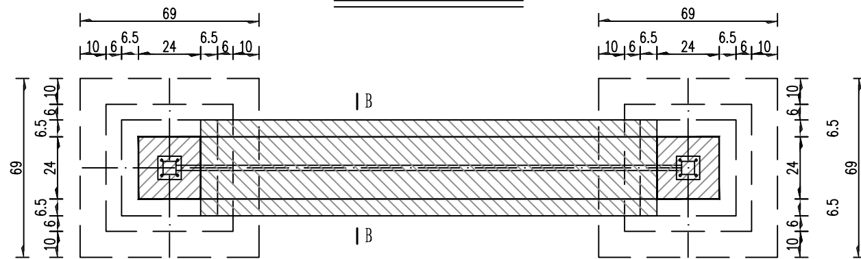
围墙基础平面大样
