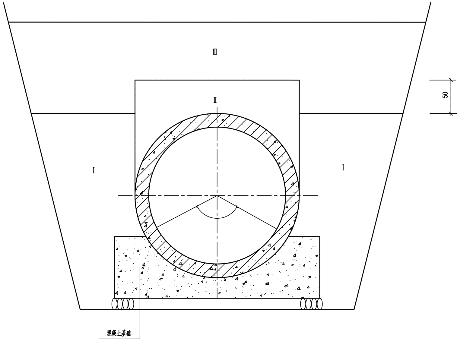
钢筋混凝土管沟槽回填大样图
