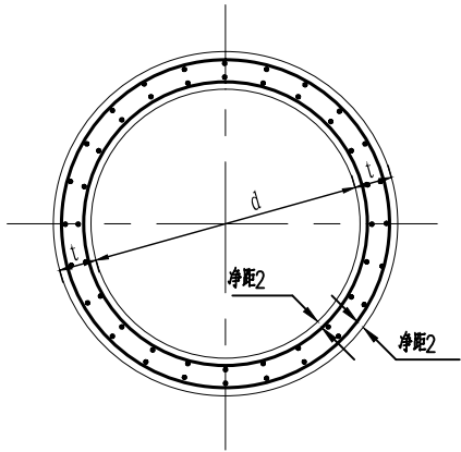
管节横断面
