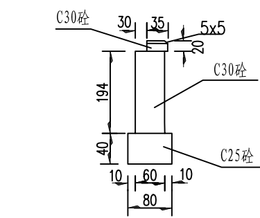
端墙
