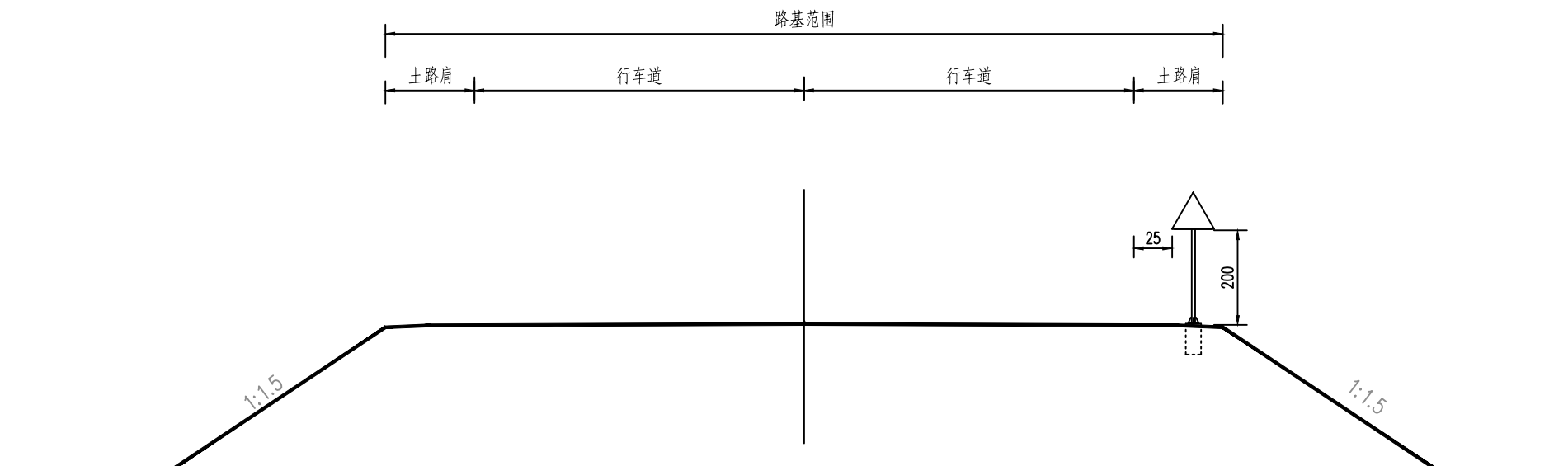
安全设施横断面图
