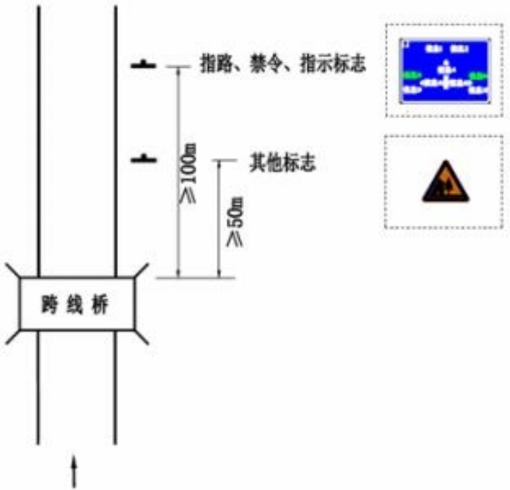
标志间距
