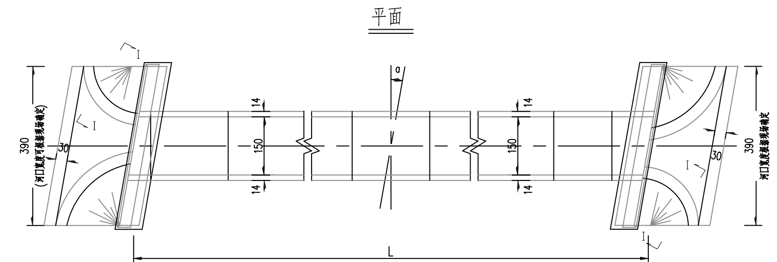
端墙
