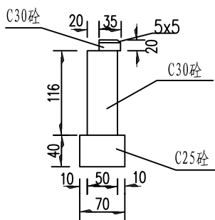
端墙
