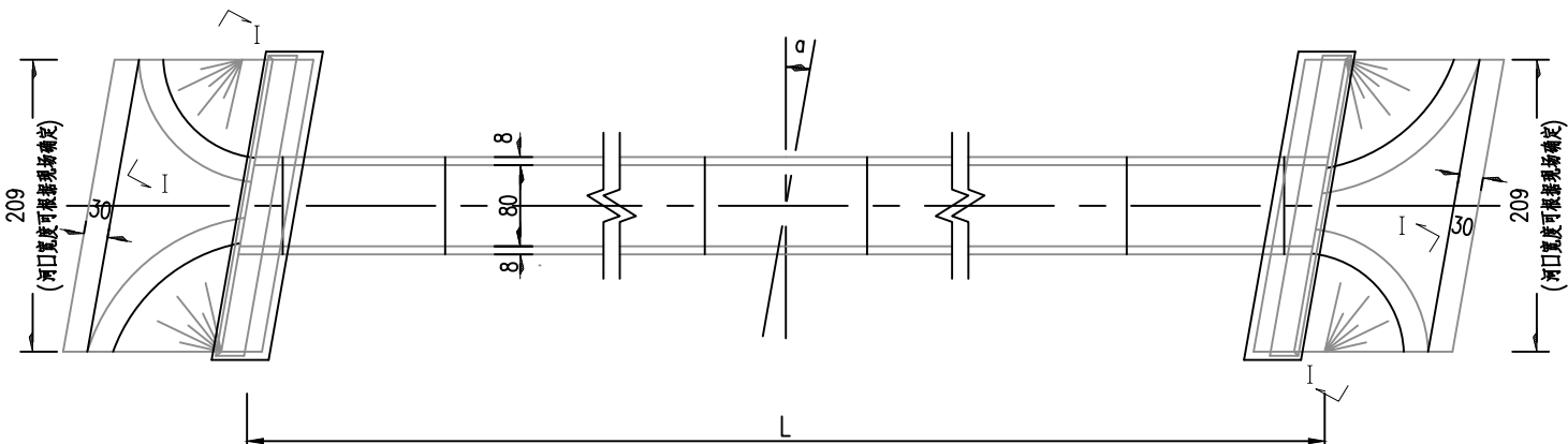
平面
