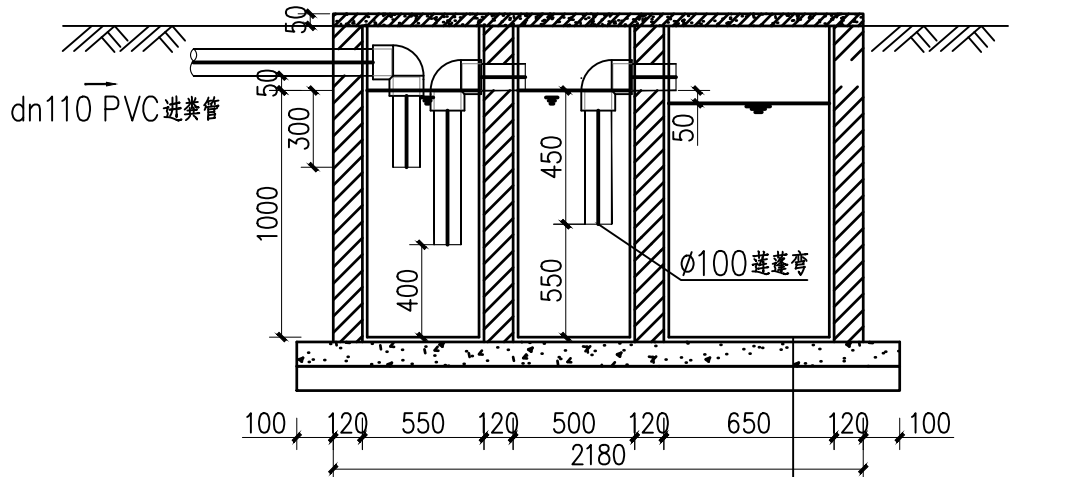
三格式化粪池剖面图
