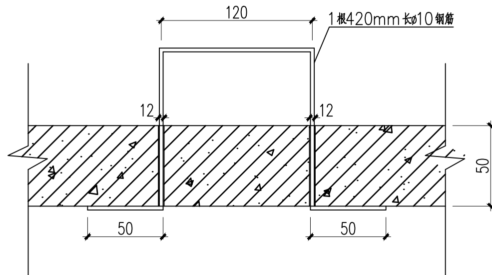
把手大样图
