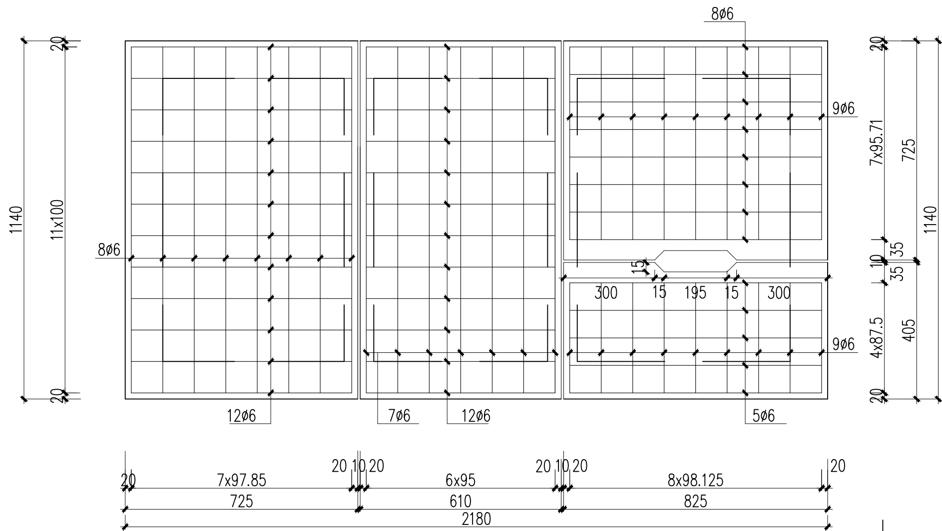
顶板配筋图
