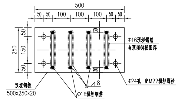
预埋钢板大样图 1:12.5
