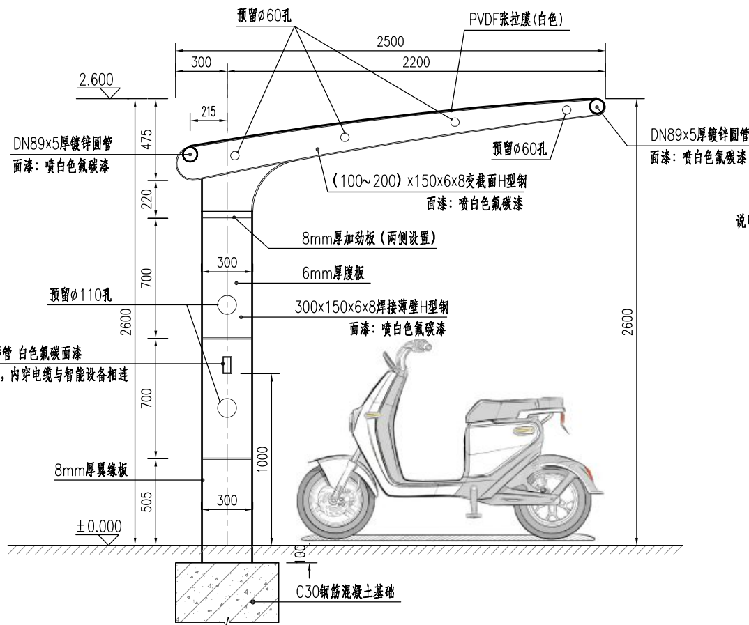
车棚剖面图 1:30
