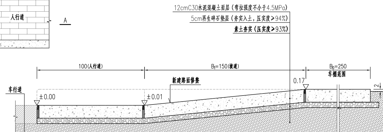
出入口纵剖面 (C-C) 1:20
