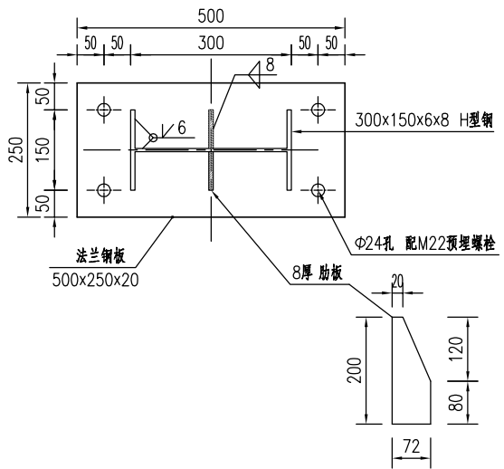
C-C剖面图 1:25
