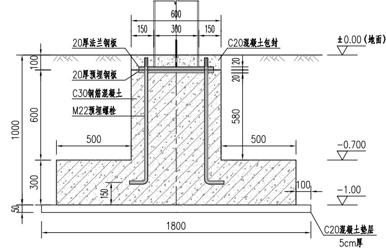
A-A剖面图 1:25
