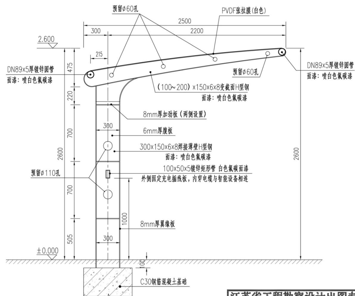
图 5-1 车棚剖立面图 (
