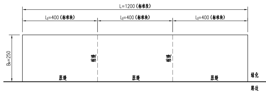
类型(B) 板块划分平面图
