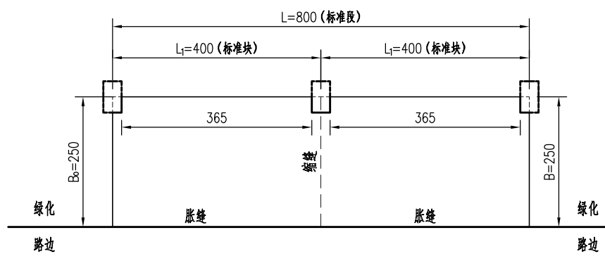
类型(A) 板块划分平面图
