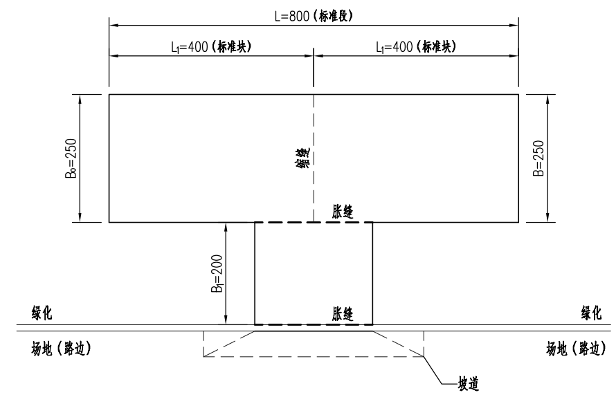
其他类型板块划分平面图
