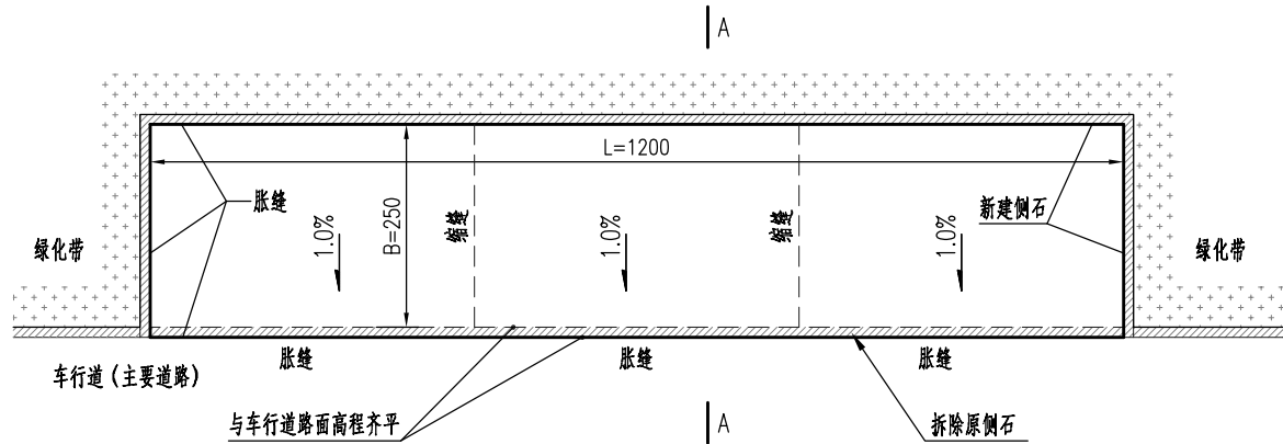
类型 (B) 停车棚平面
