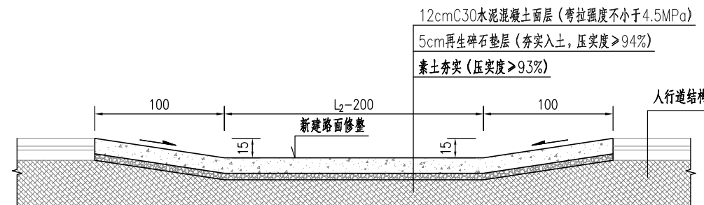
人行道双面坡剖面 (A-A) 1:40
