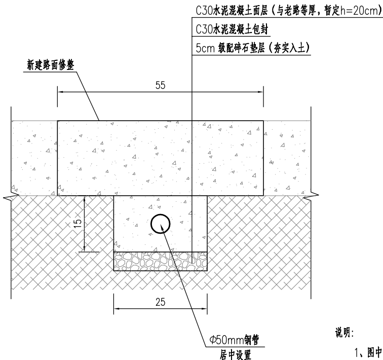
掘路修复路面结构设计图 1:10 适用于: 电缆管线过路情况
