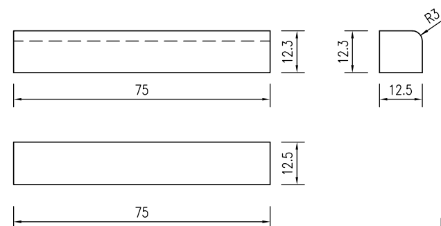
Y2侧石构造 1:15
