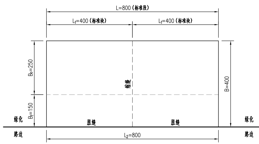
类型(C)、(D)板块划分平面图
