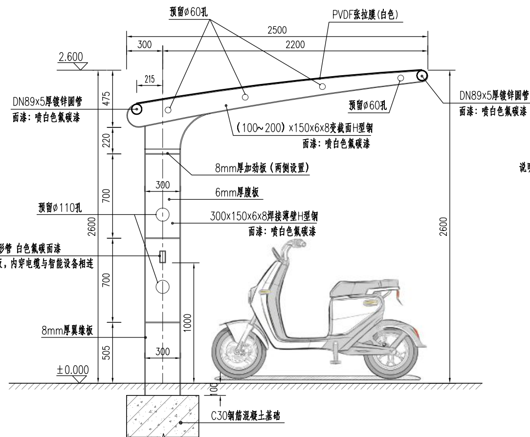
车棚剖面图 1:30
