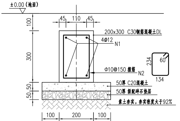
地梁配筋图 (DL) 1:12.5
