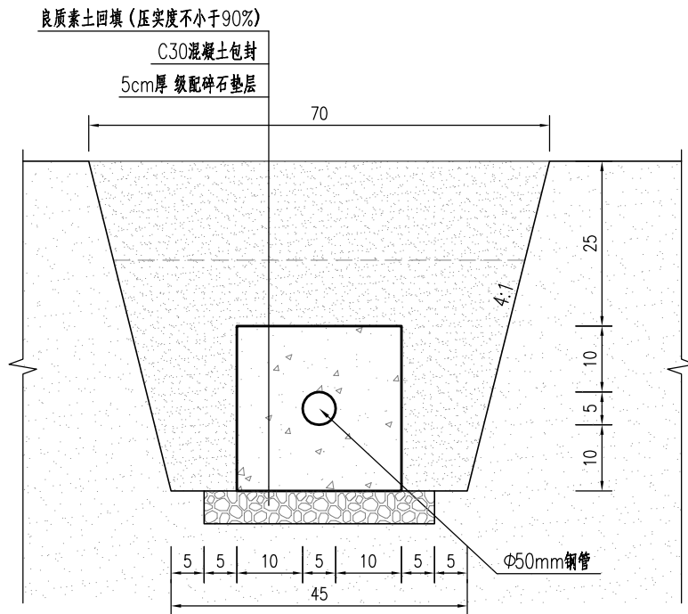
绿化带填挖修复结构设计图 1:10 适用于范围: 电缆在绿化带范围
