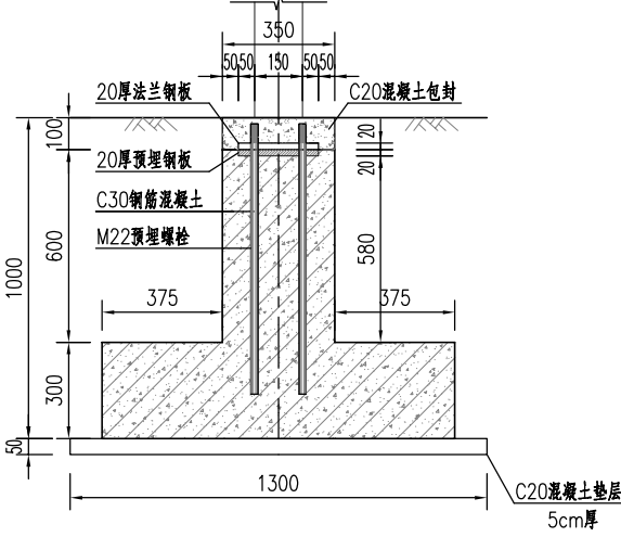
C-C剖面图 1:25
