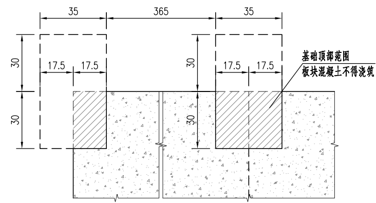
基础顶部预留安装空间示意图
