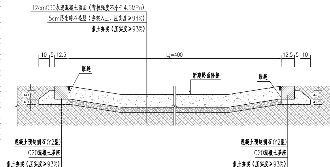
出入口纵剖面 (C-C) 1:20
