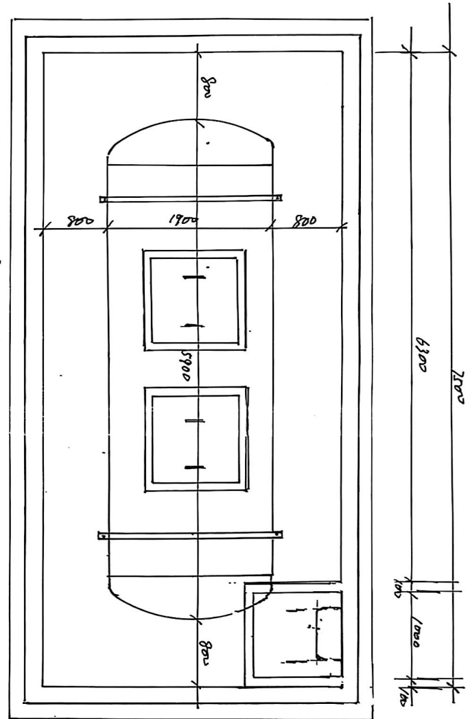
15m²油罐间尺寸图
