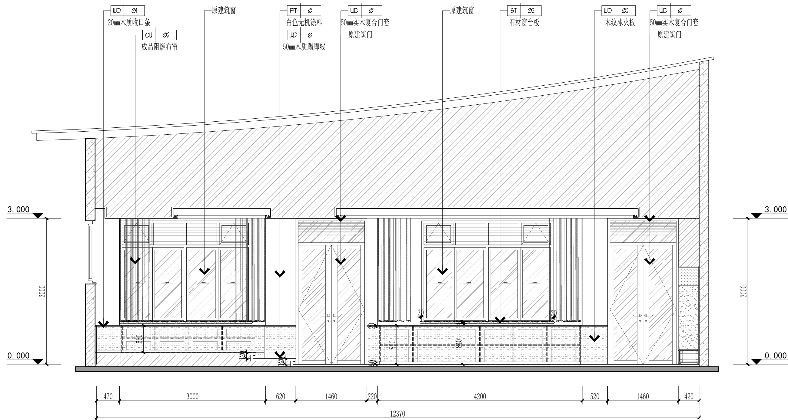
E25 ELEVATION 夹城里A规划幼儿园三层阅览室立面图 SCALE: 1/50
