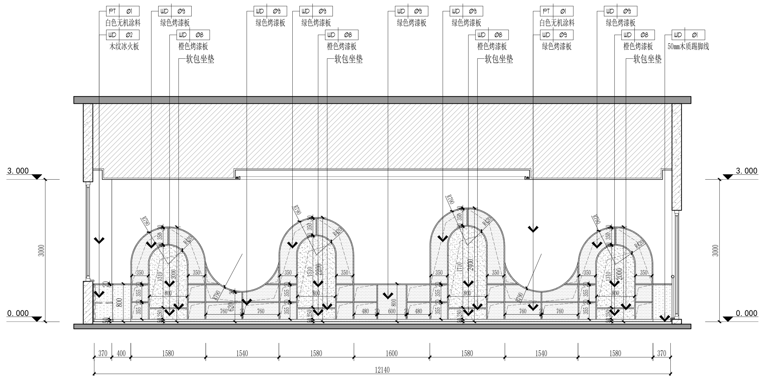
E26 ELEVATION 夹城里A规划幼儿园三层阅览室立面图 SCALE: 1/50
