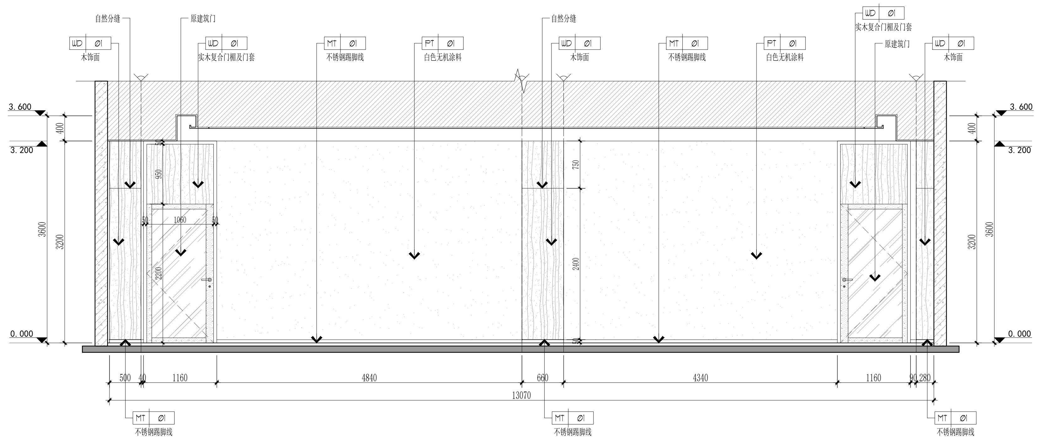
E04 ELEVATION 夹城里B规划幼儿园三层党团会议室立面图
