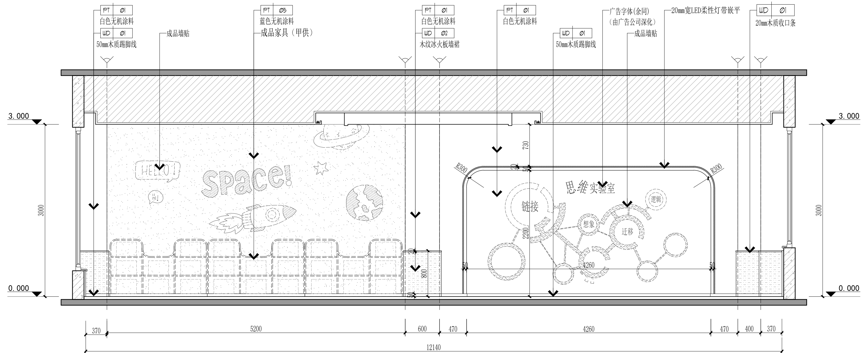
夹城里A规划幼儿园二层科发教室立面图
