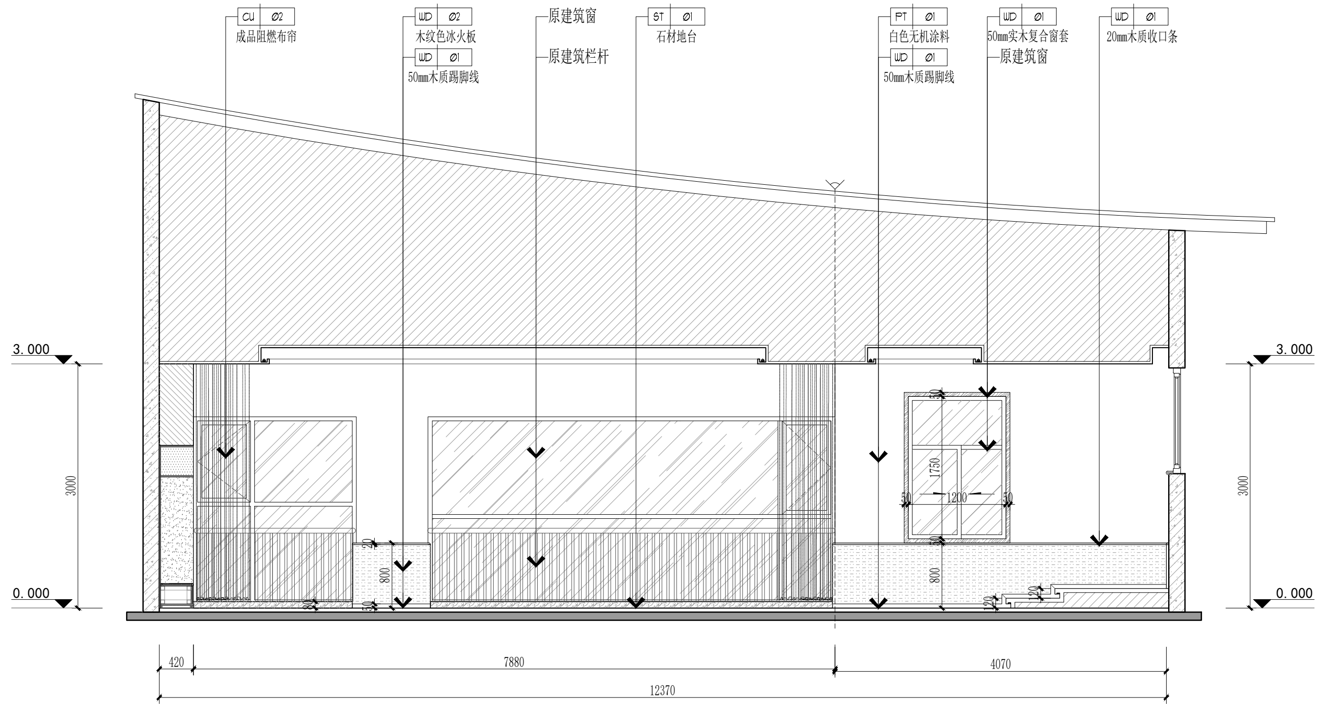
夹城里A规划幼儿园三层阅览室立面图
