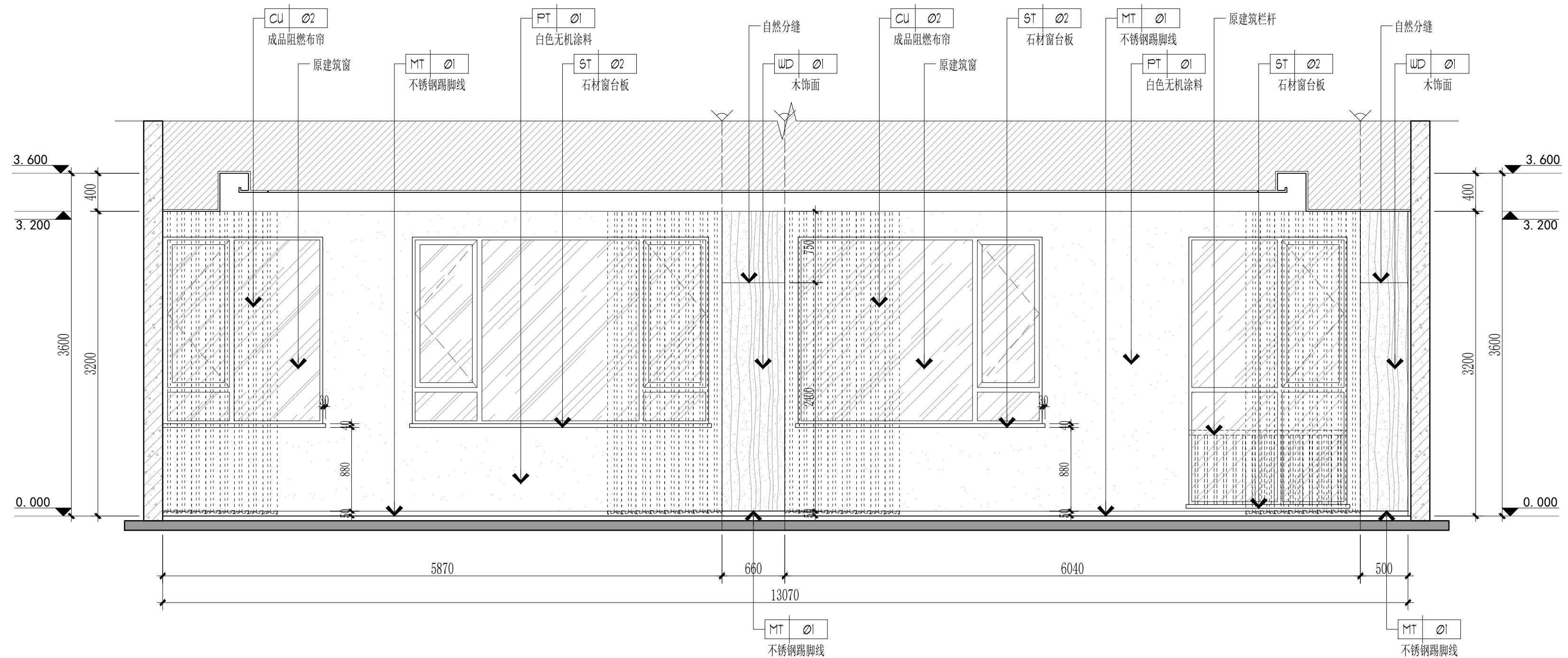
E02 ELEVATION 夹城里B规划幼儿园三层党团会议室立面图
