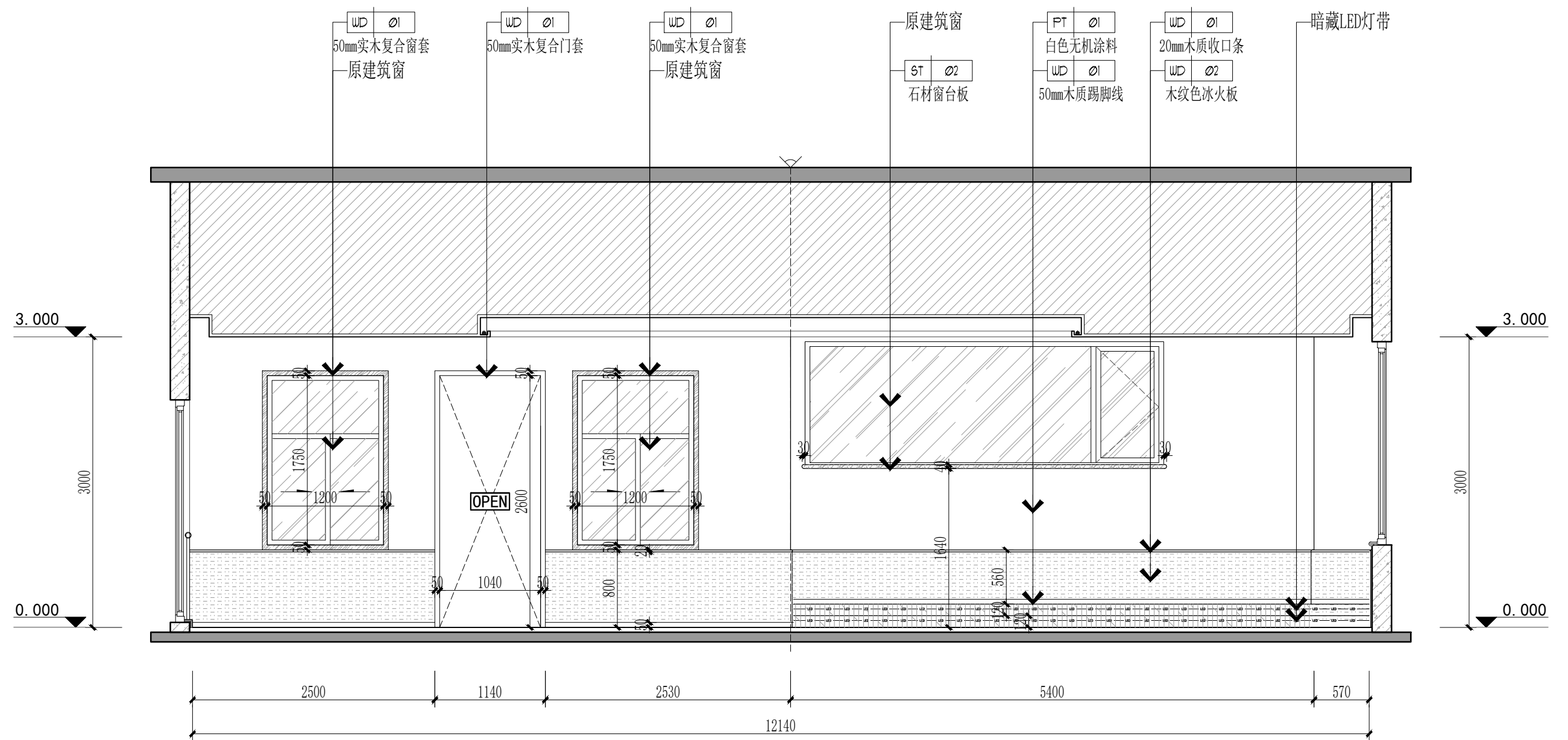
夹城里A规划幼儿园三层阅览室立面图
