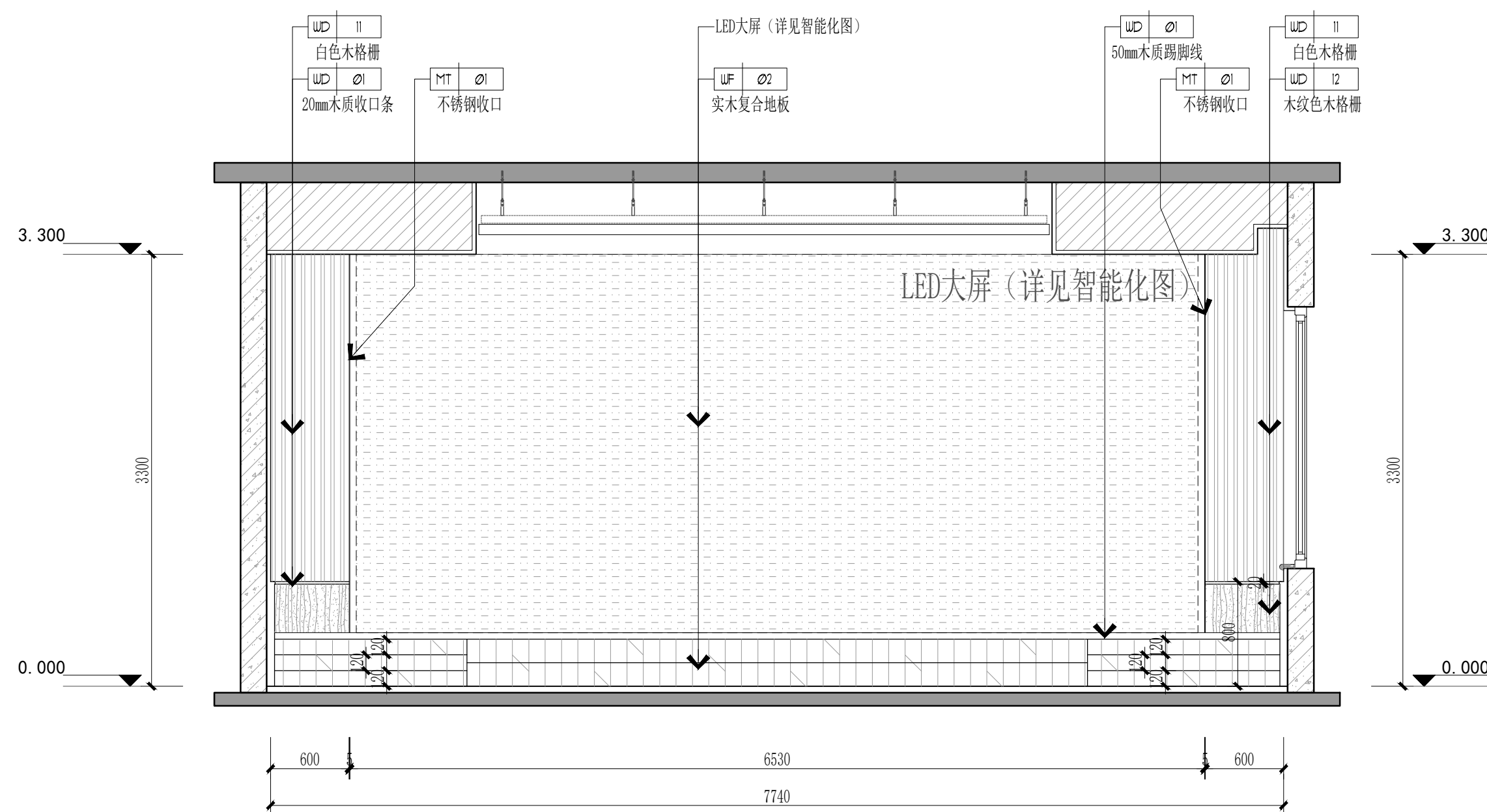
夹城里A规划幼儿园三层报告厅立面图
