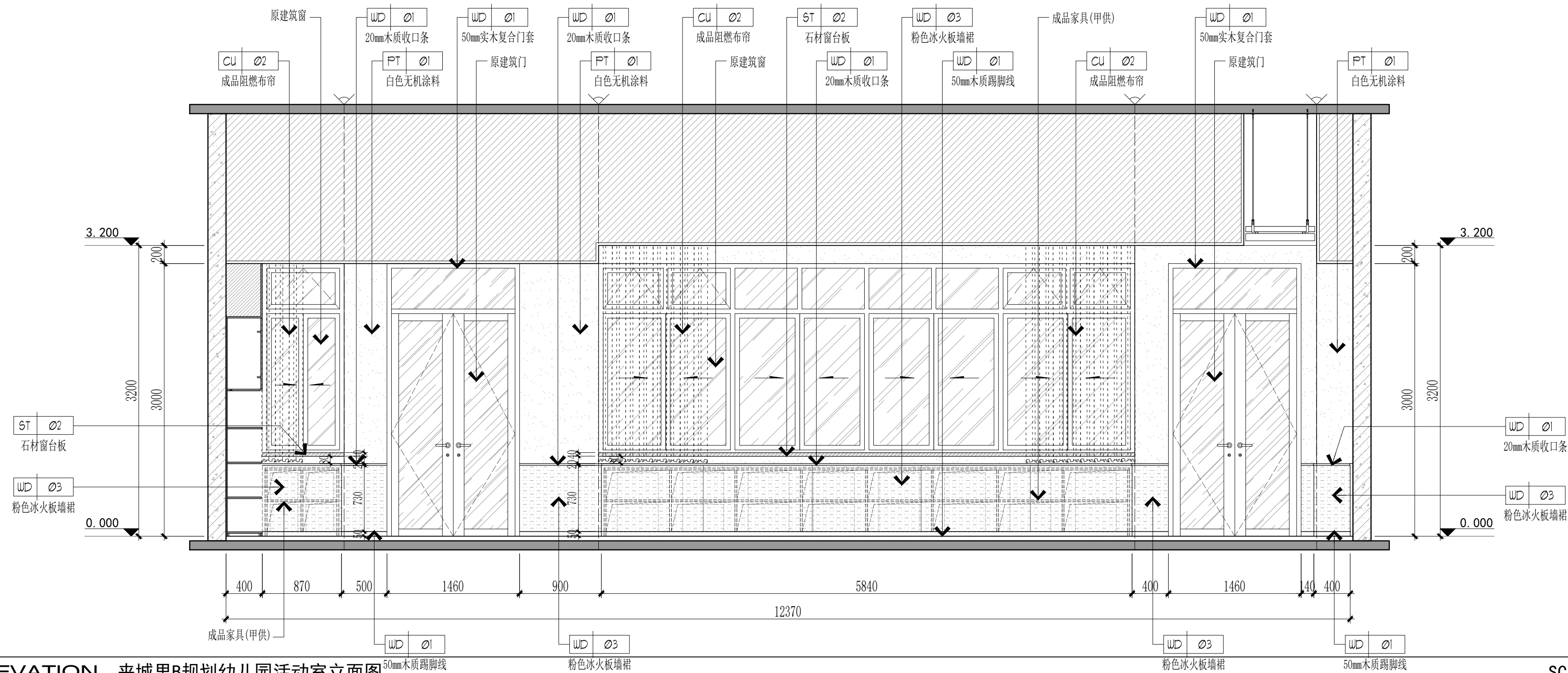
E03 ELEVATION 夹城里B规划幼儿园活动室立面图 SCALE: 1/40
