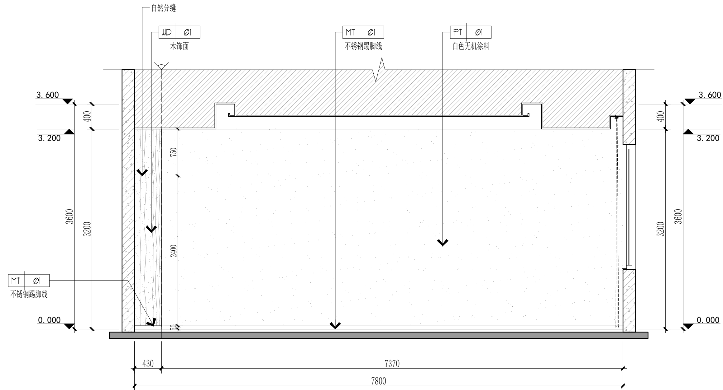
E01 ELEVATION 夹城里B规划幼儿园三层党团会议室立面图
