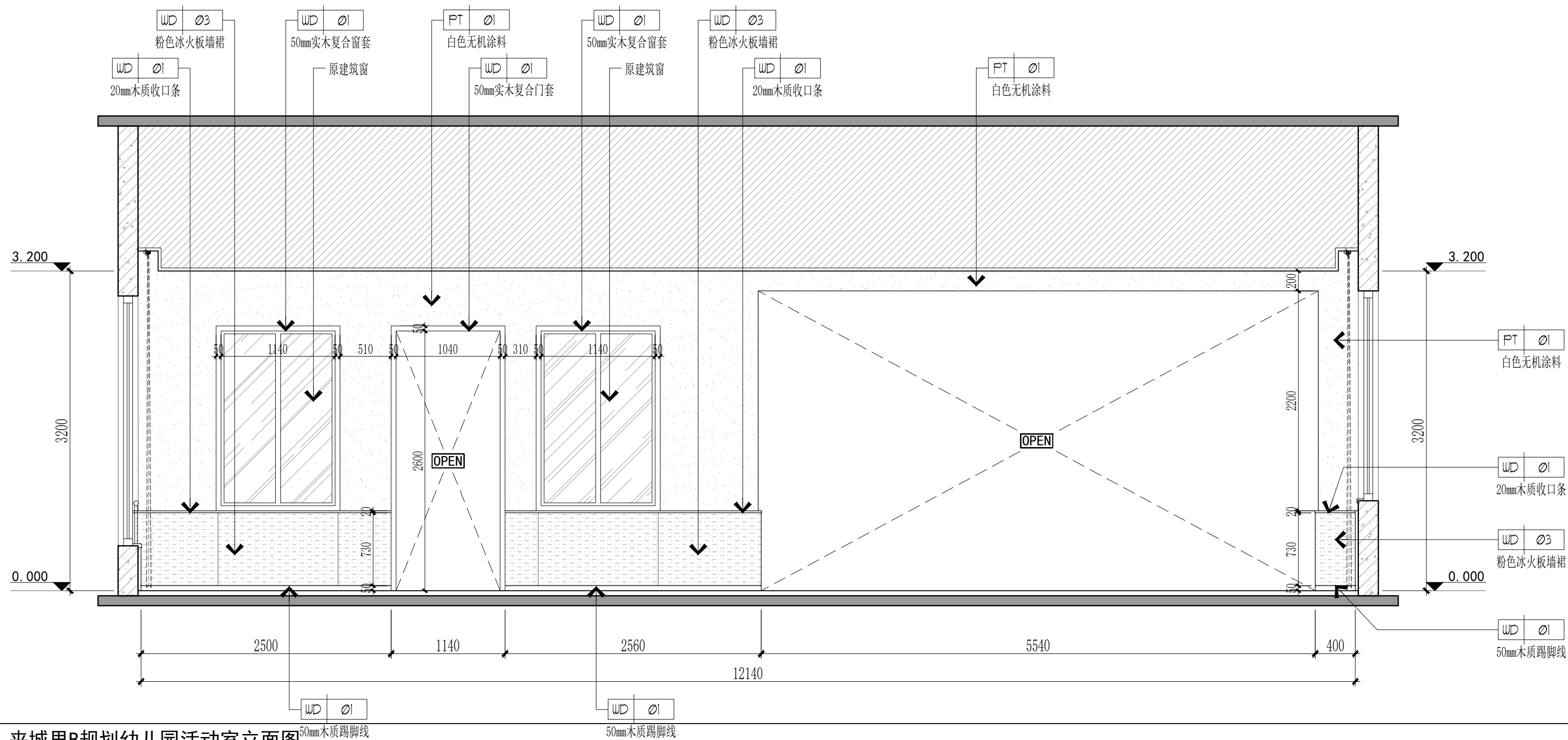
E02 ELEVATION 夹城里B规划幼儿园活动室立面图
