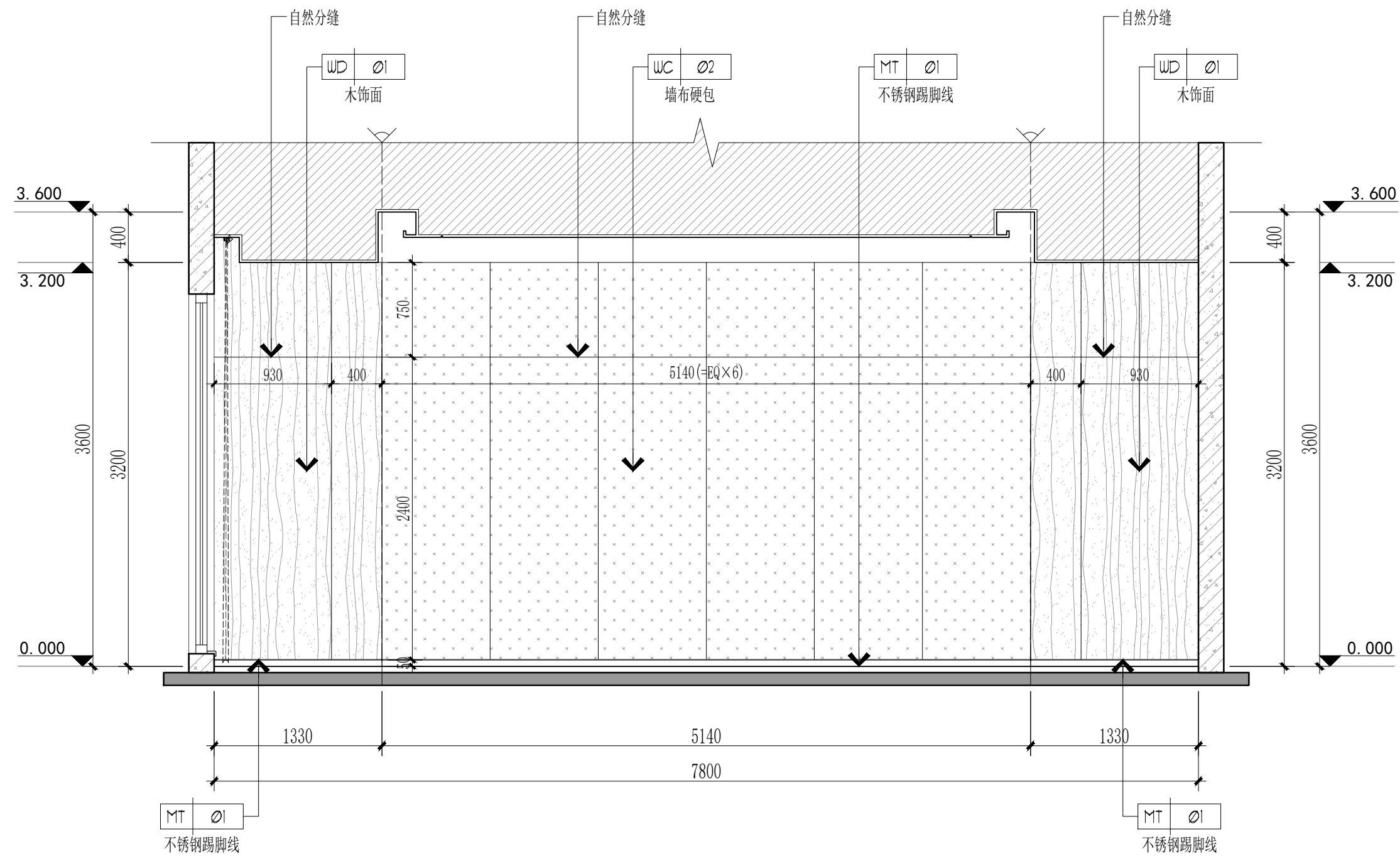
E03 ELEVATION 夹城里B规划幼儿园三层党团会议室立面图
