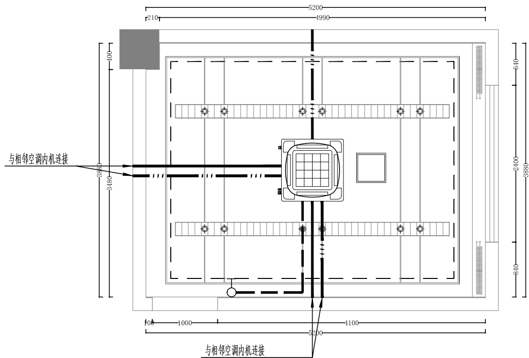
三层贵宾休息室空调平面图 1:25
