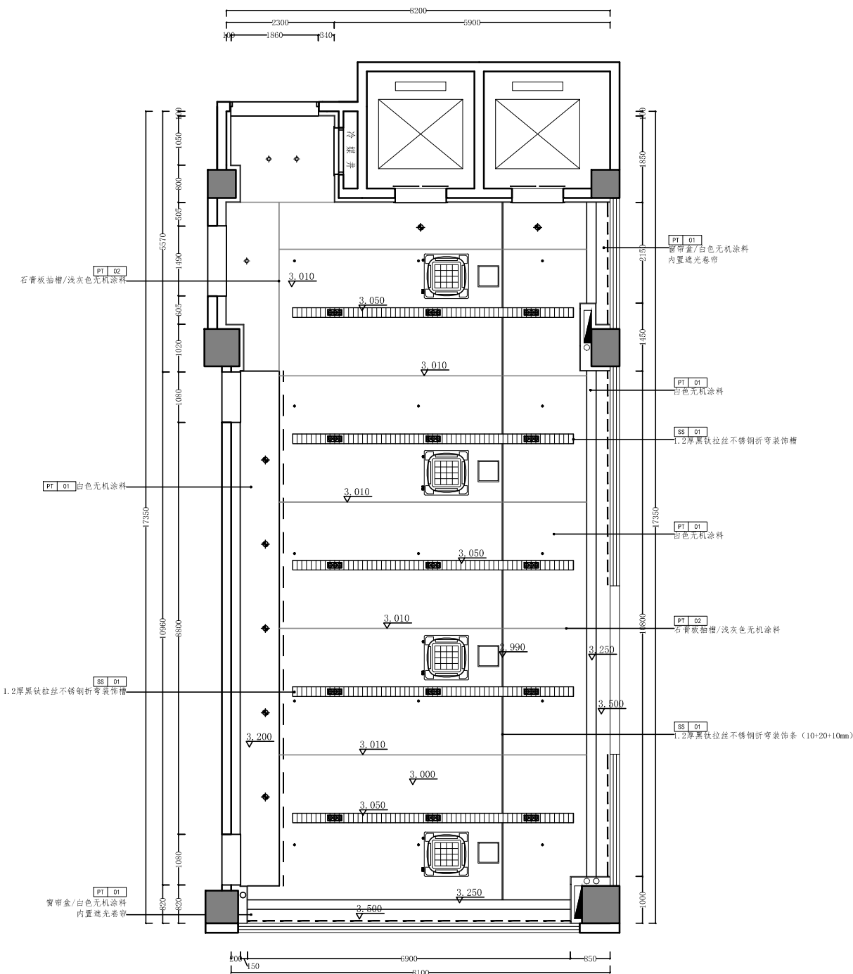
一层门厅顶面布置图 1:50
