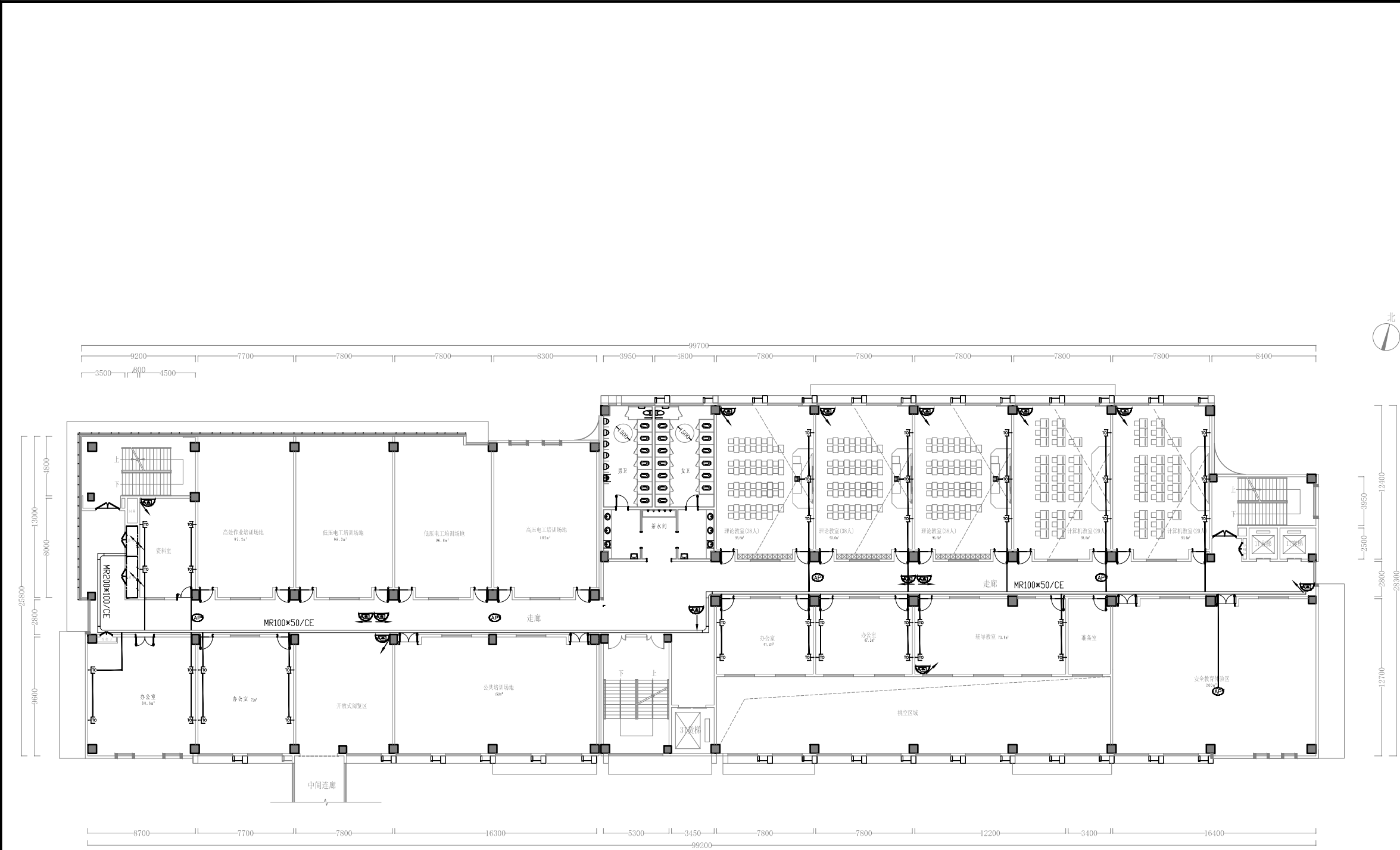
二层监控、网络平面图 1:160
