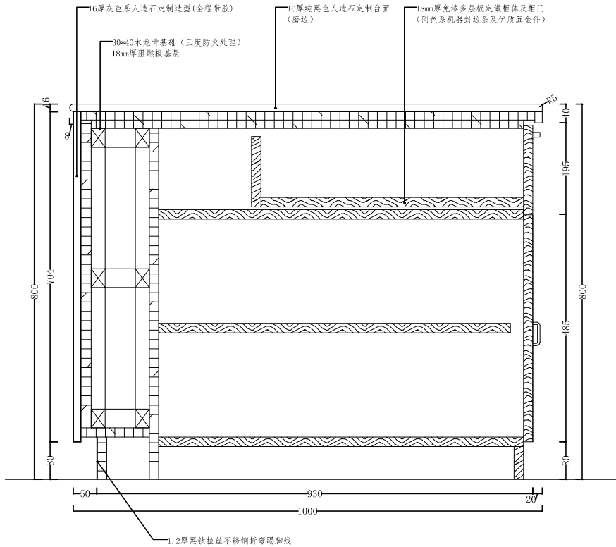
一层门厅服务台b-b剖面图 1:10
