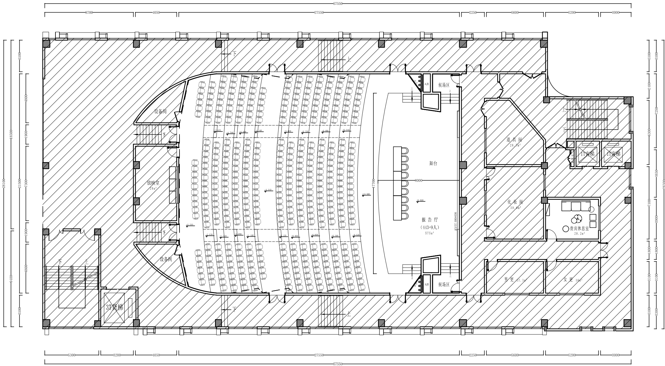
三层平面布置图 1:100
