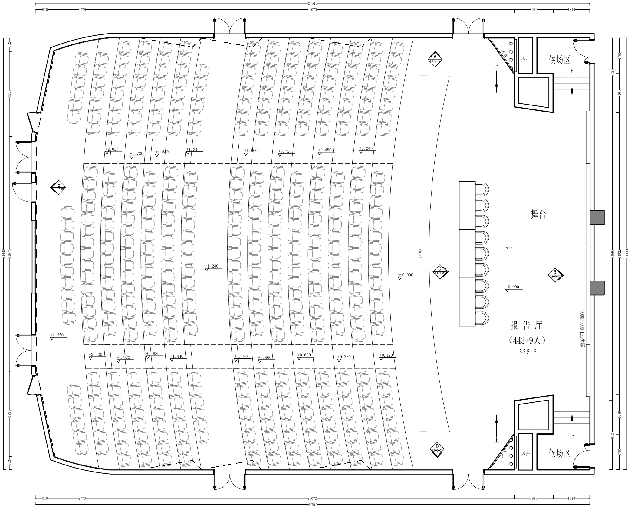
三层大报告厅平面索引图 1:50
