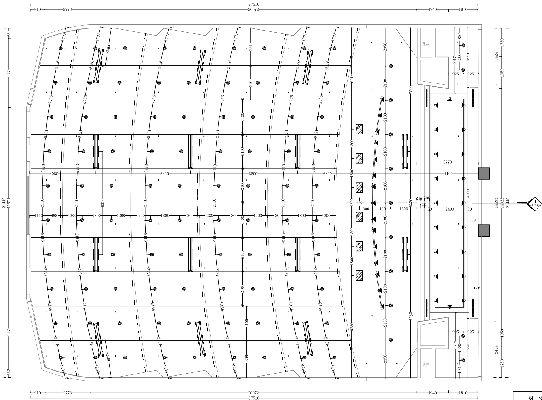
三层大报告厅灯具定位图 1:60
