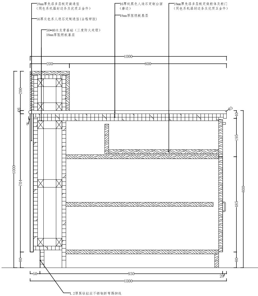
一层门厅服务台a-a剖面图 1:10
