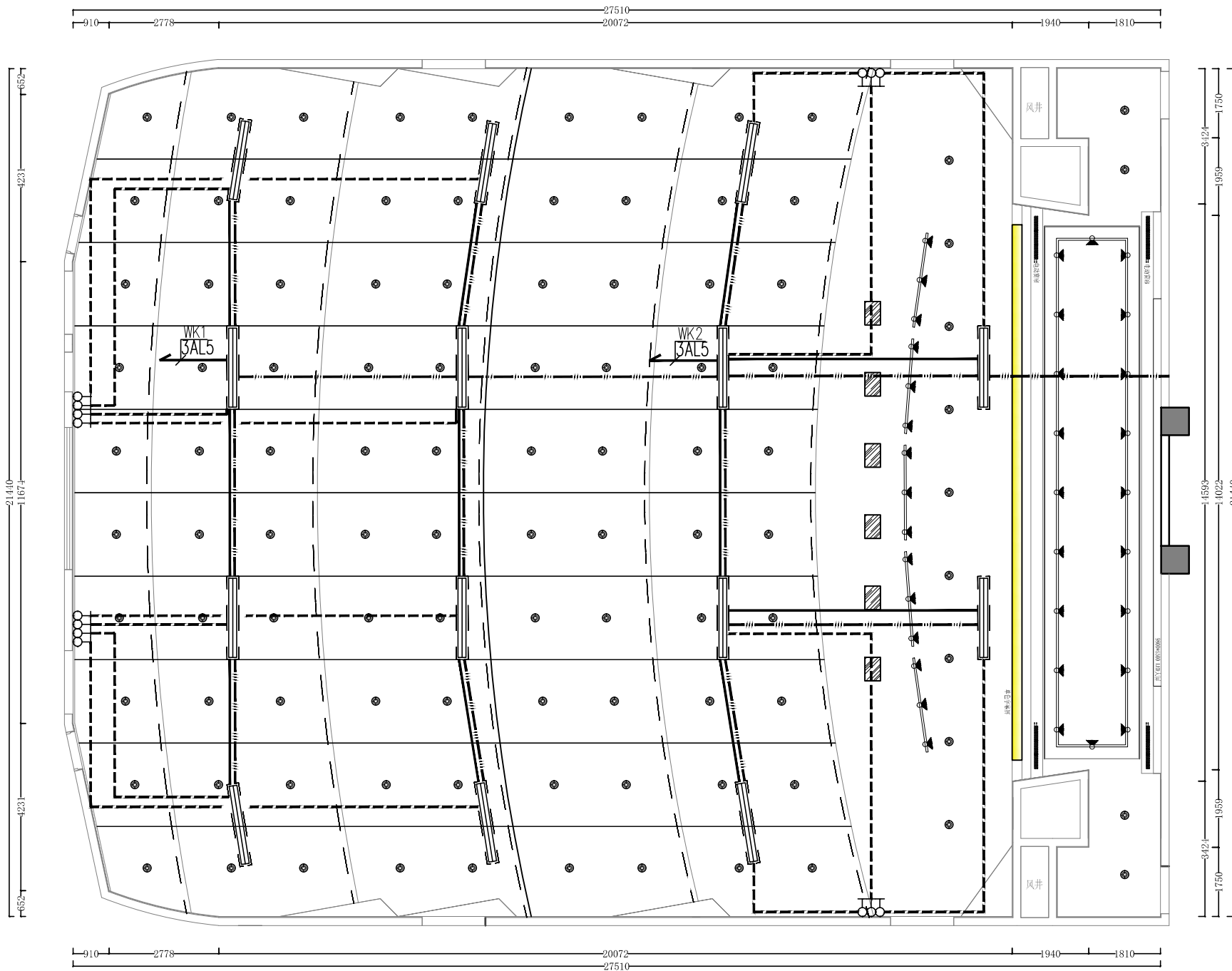
三层大报告厅空调平面图 1:60
