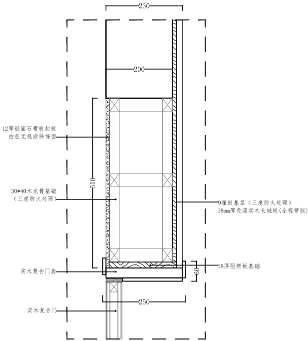
H JT-2-01 三层贵宾休息室C立面节点图 1:10
