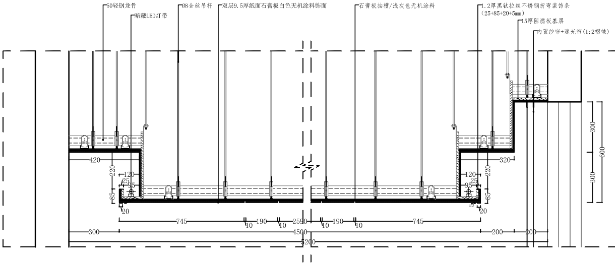
6 JT-2-01 三层贵宾休息室吊顶剖面图 1:10
