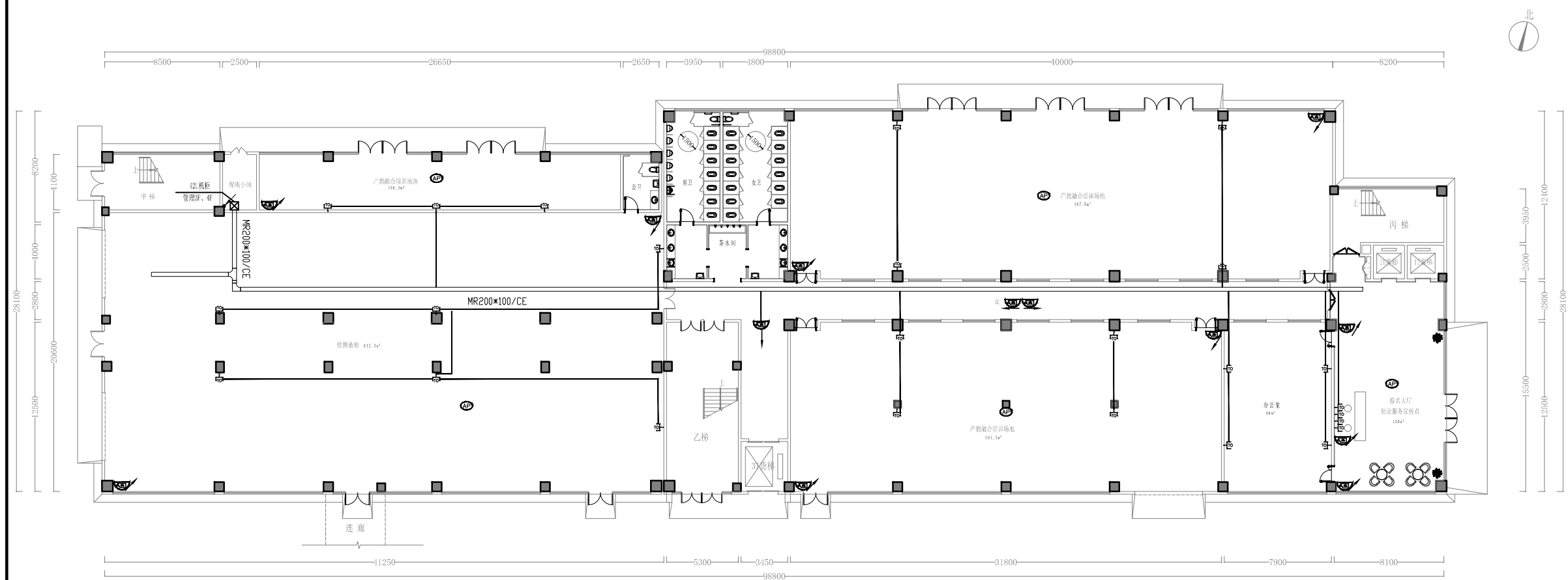
一层监控、网络平面图 1:160
