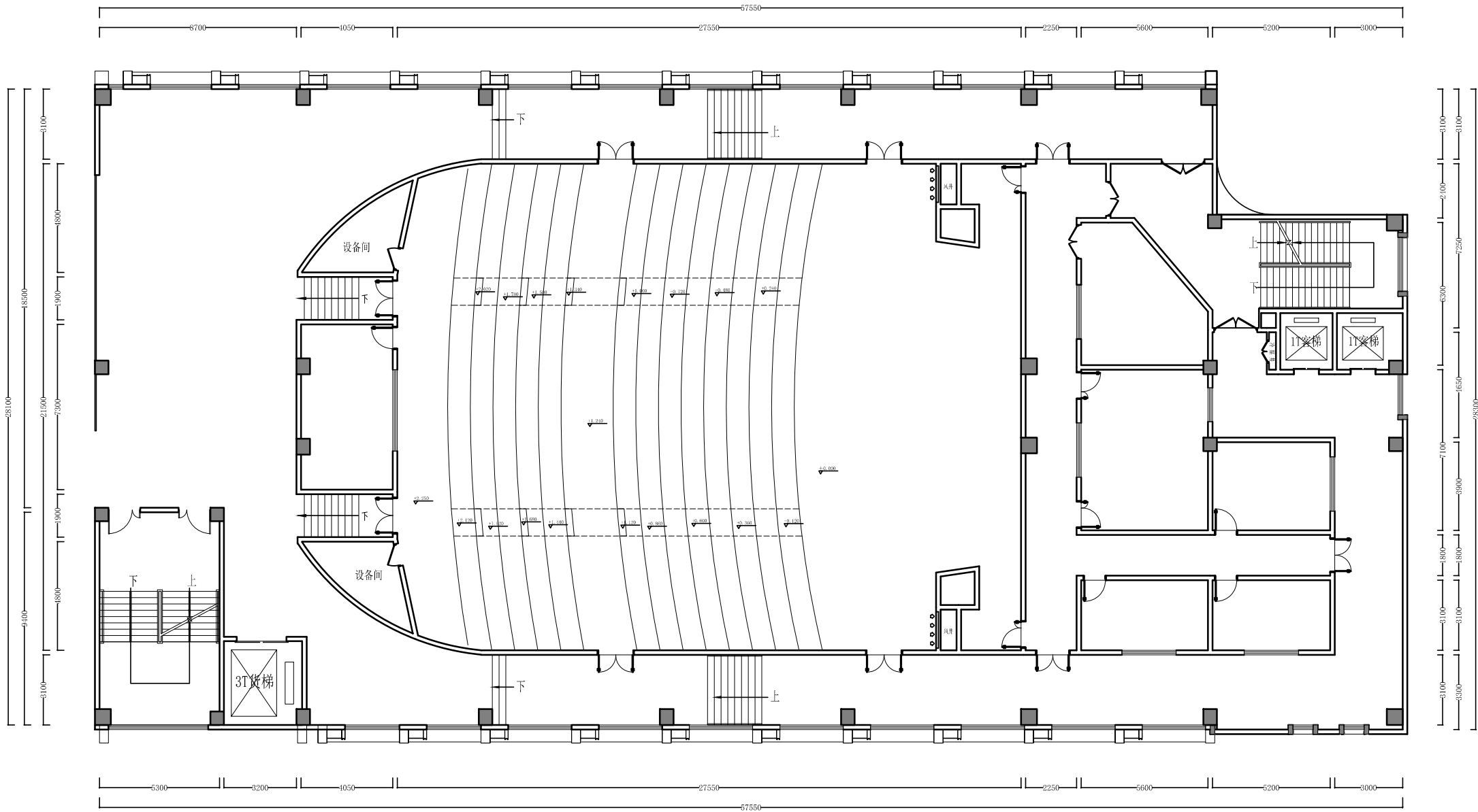
三层原始平面图 1:100
